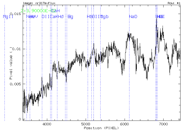
FIG. G.17 : Spectre de SN 2000bt obtenu le 8 Avril 2000 au WHT.
