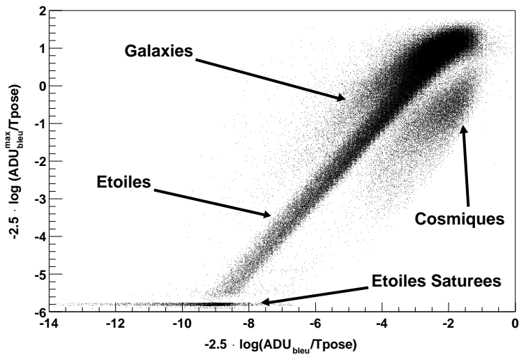
FIG. 8.1 : Les différents objets présents sur les images EROS dans le plan brillance de surface S_{B_{eros}} en fonction de la magnitude \tilde{B}_{eros} , pour un sous-ensemble de 23 champs de 1999 dans la bande B_{eros} . La bande rectiligne correspondant aux étoiles vérifie la relation (8.7). Au-dessus, pour une brillance de surface plus faible à flux égal, ce sont les galaxies. En-dessous, on a les cosmiques.
