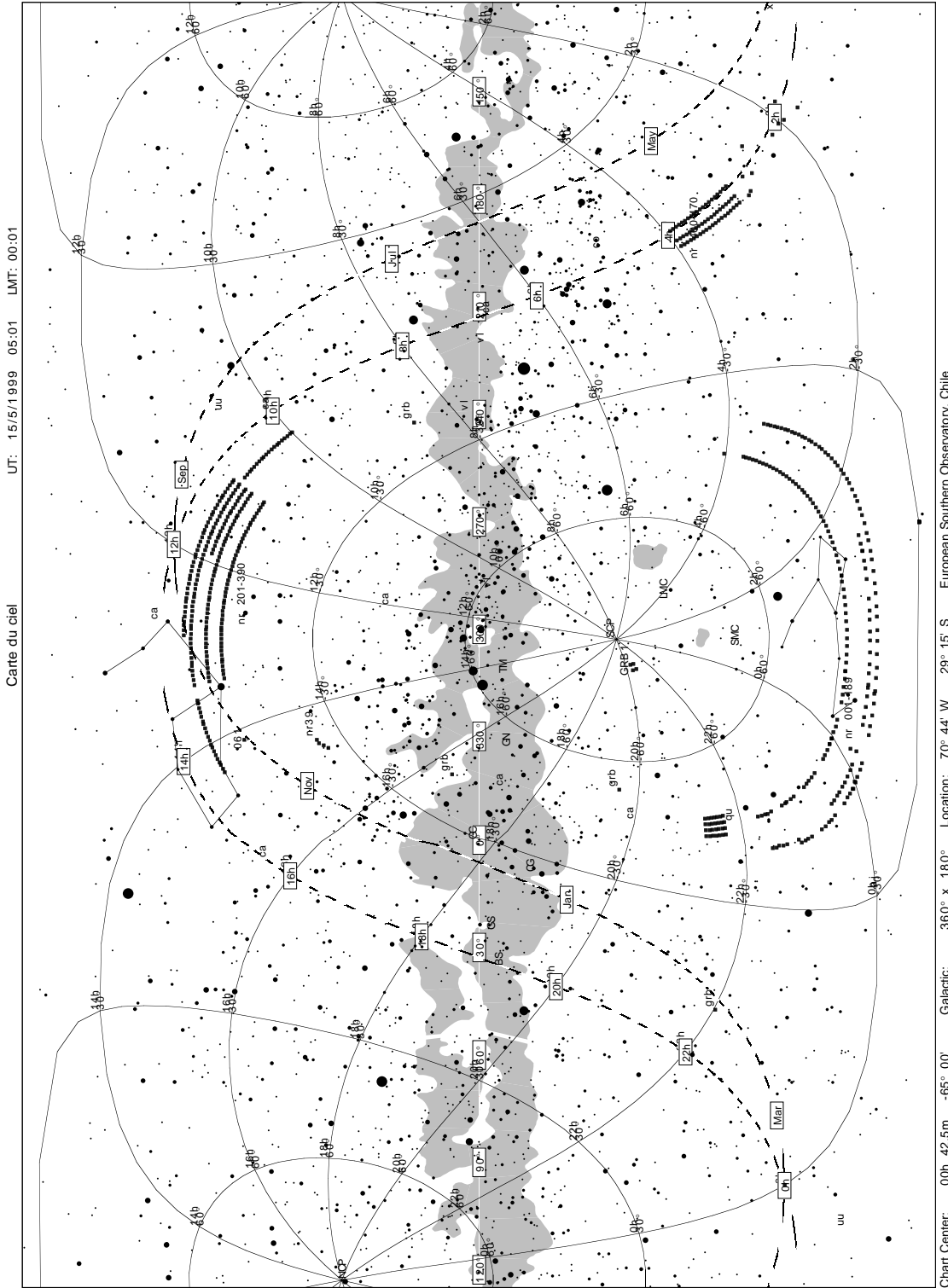
FIG. 7.16 : Positionnement des champs de recherche de supernova en coordonnées galactiques, représentés par des petits carrés noirs. Les champs qui ont servi aux recherches de 1999 et 2000, visibles au printemps, sont ceux de l'hémisphère nord galactique.
