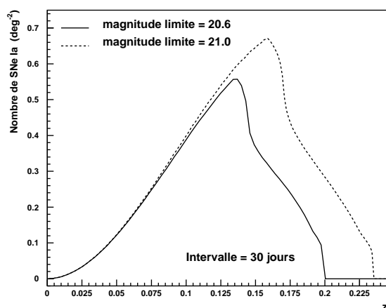
FIG. 8.34 : Distribution des supernovæ en décalage spectral pour deux valeurs de la magnitude limite, correspondant à des temps de pose de 300 secondes et 600 secondes pour EROS. Le seuil en décalage spectral augmente d'environ 20%, ce qui correspond au doublement du temps de pose. L'intervalle de temps entre la découverte et la référence est de 30 jours. La coupure en magnitude apparente de la galaxie hôte est 19.
