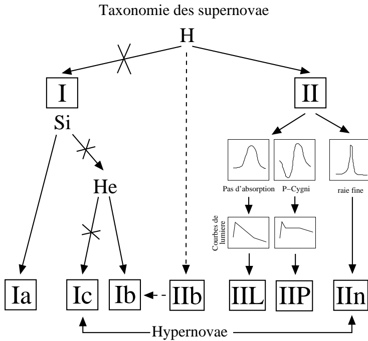
FIG. 1.1 : La classification détaillée des supernovæ nécessite non seulement l'identification de certaines caractéristiques dans les spectres, mais aussi une analyse fine de l'évolution de la luminosité, des spectres et des profils des raies. Ce diagramme montre que la classification repose sur la présence (ou l'absence) de certaines raies dans le spectre (principalement le spectre photosphérique) – pour les différents « type I » – mais aussi sur la forme de la courbe de lumière ainsi que sur le profil de certaines raies – pour les différents « type II » (d'après Cappellaro & Turatto 2000).
