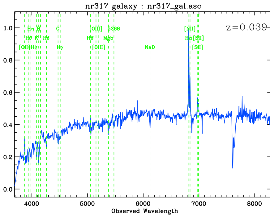
FIG. G.18 : Spectre de la galaxie hôte de SN 2000bt obtenu le 8 Avril 2000 au WHT.
