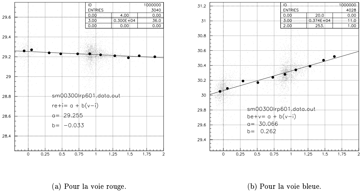
FIG. D.4 : Exemples d'ajustements du terme de couleur en utilisant les étoiles d'Ogle superposées au catalogue de référence EROS pour un CCD d'un champ du SMC.
