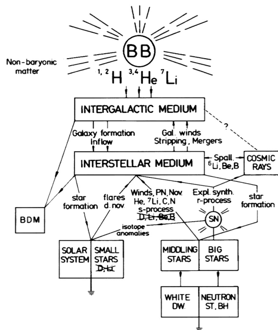
FIG. 5.6 : Illustration d'un scénario d'évolution chimique de l'Univers. Tiré de Pagel (1997).
