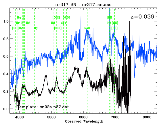
FIG. G.16 : Spectre de SN 2000bt obtenu le 8 Avril 2000 au WHT.
