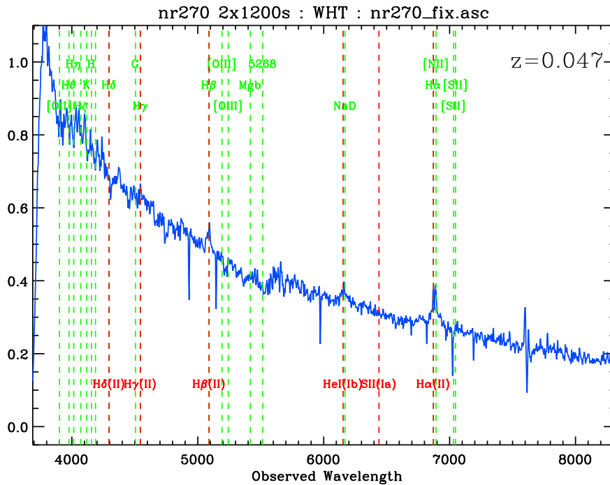
FIG. G.19 : Spectre de SN 2000bu obtenu le 9 Avril 2000 au WHT.
