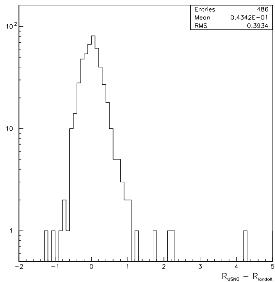
FIG. C.4 : Histogramme de R_{\text{USNO}} - R_{\text{Landolt}} montrant là encore une importante dispersion.
