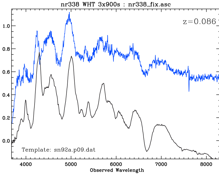
FIG. G.23 : Spectre de SN 2000bx obtenu le 8 Avril 2000 au WHT.
