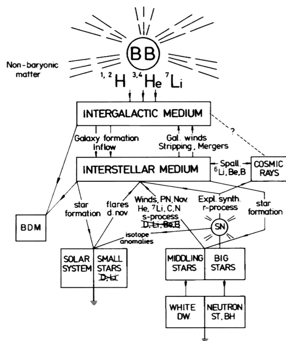
FIG. 5.6 : Illustration d'un scénario d'évolution chimique de l'Univers. Tiré de Pagel (1997).
