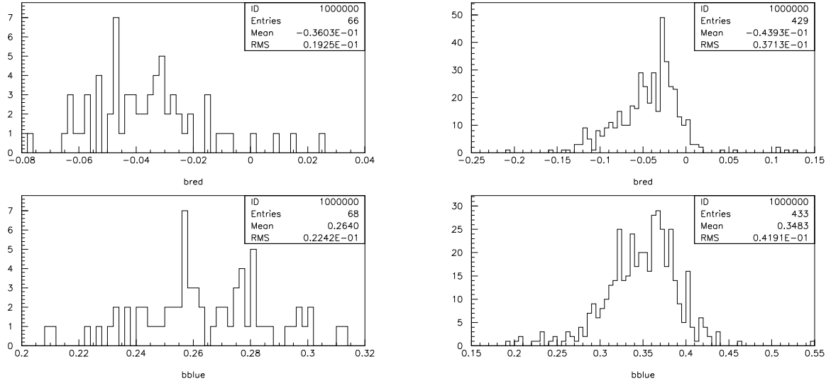
(a) Histogramme du terme de couleur pour la voie rouge (en haut) et pour la voie rouge (en bas) déterminé avec le catalogue Ogle.
