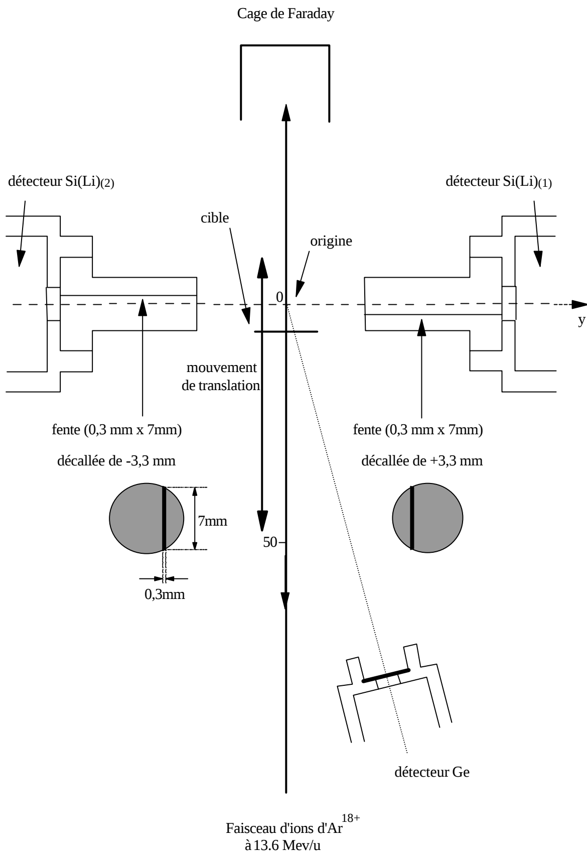
Figure II-12 : Dispositif expérimental.
