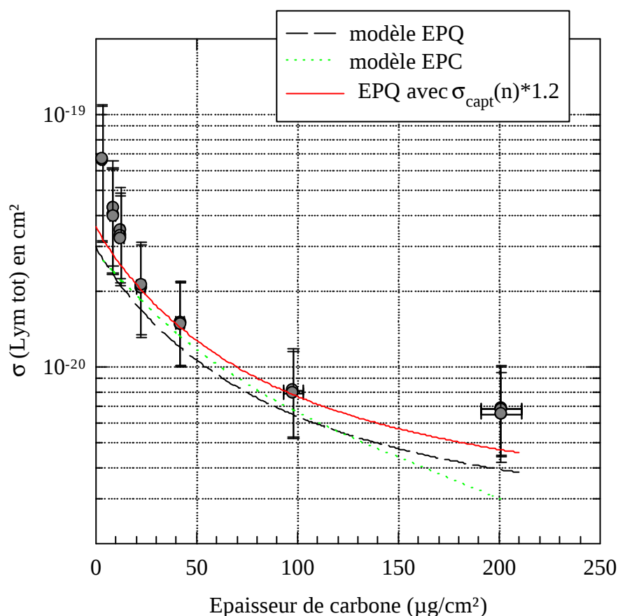
Figure V-31 : Comparaison de l'évolution de la section efficace totale d'émission Lyman de l' \text{Ar}^{17+} ( v_p=23 ua) en fonction de l'épaisseur de carbone avec les valeurs des modèles EPQ et EPC.
