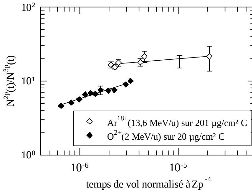
Figure V-8 : Evolution des rapports d'intensités N^{(2p \text{ @} 1s)}(t) / N^{(3p \text{ @} 1s)}(t) avec le temps de vol pour les collisions O^{2+} ( v_p=9 \text{ ua} ) @ C (Can et al, 1987) et Ar^{18+} ( v_p=23 \text{ ua} ) @ C. Le temps de vol est normalisé à Z_p^{-4} .
