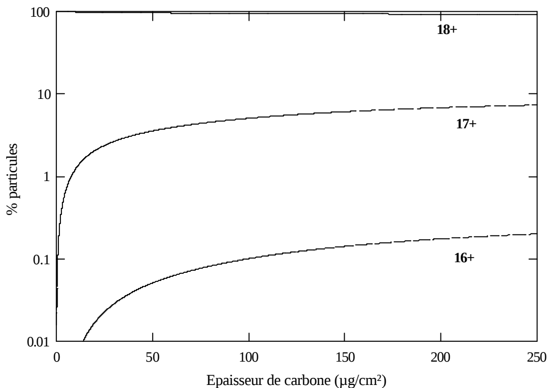
Figure II-11 : Evolution de la distribution d'état de charge pour la collision \text{Ar}^{18+} @ C à 13,6 MeV/u en fonction de l'épaisseur de cible.
