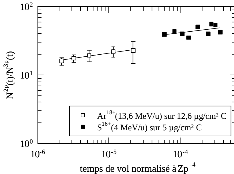
Figure V-9 : Evolution des rapports d'intensités N^{(2p \text{ @} 1s)}(t) / N^{(3p \text{ @} 1s)}(t) avec le temps de vol pour les collisions S^{16+} ( v_p=13 ua) @ C (Rothermel et al, 1983) et Ar^{18+} ( v_p=23 ua) @ C. Le temps de vol est normalisé à Z_p^{-4} .
