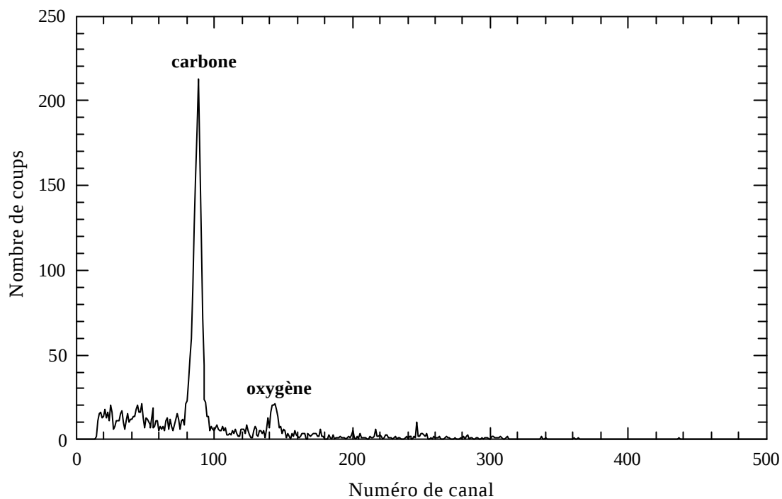
Figure II-5 : Spectre en énergie des particules \alpha rétrodiffusées détectées à 165^\circ pour une cible de 3,5 \mu\text{g}/\text{cm}^2 de carbone.
