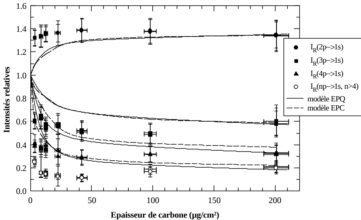
Figure V-25 : Evolution des intensités relatives normalisées des transitions Lyman émises par l' Ar^{17+}(v_p=23 \text{ ua}) avec l'épaisseur de carbone traversée. Les symboles représentent l'expérience et les courbes les modèles décrits au chapitre IV.
