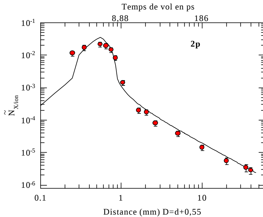
Figure V-4 : Comparaison entre l'évolution expérimentale de l'intensité de la transition Ly\alpha avec le temps de vol obtenue pour une cible de 98 \mu\text{g}/\text{cm}^2 et le modèle EPC corrigé des effets géométriques.
