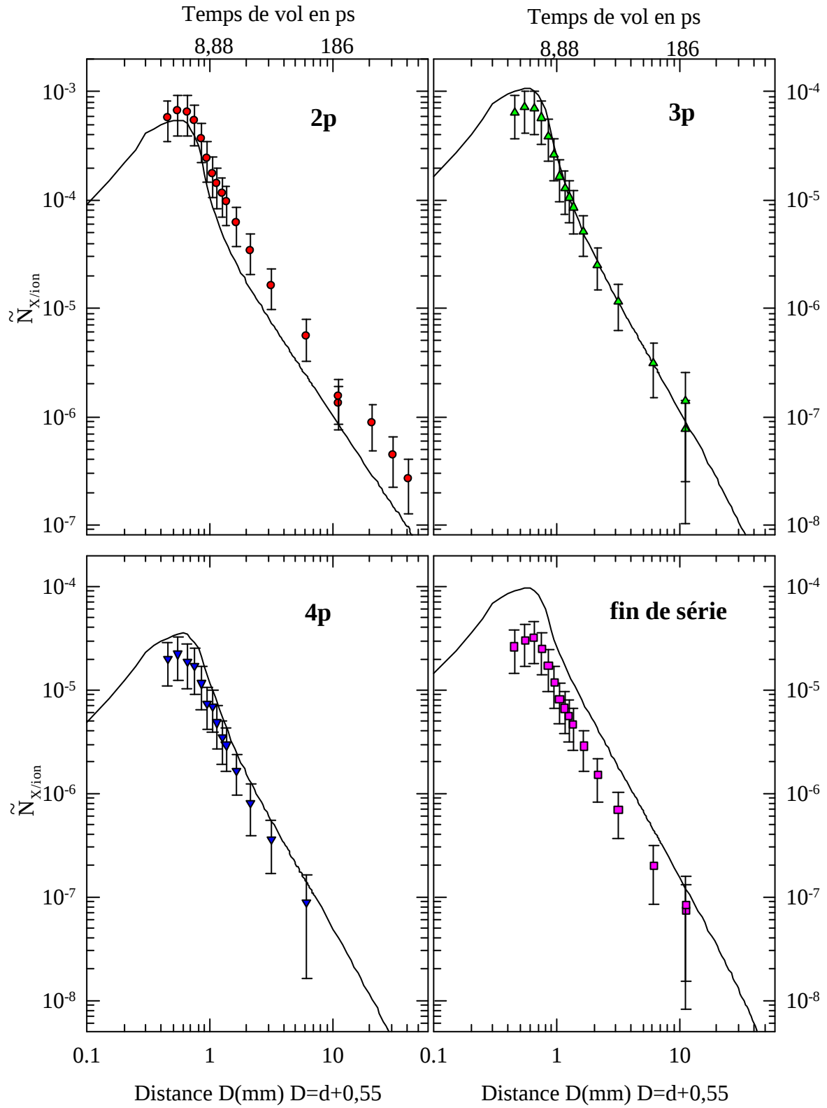
Figure V-17 : Comparaison modèle EPC - expérience.
