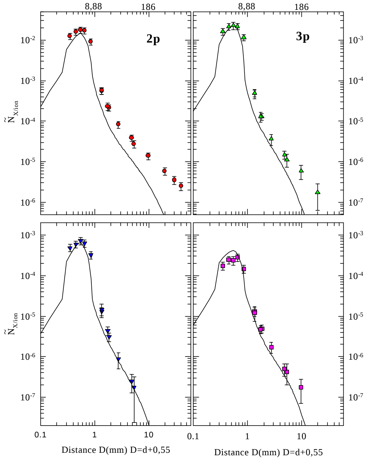
Figure A-Ia-3 : Comparaison modèle EPQ (avec les sections efficaces d'excitation intracouche de type dipolaire augmentées pour n > 5 ) - expérience.
