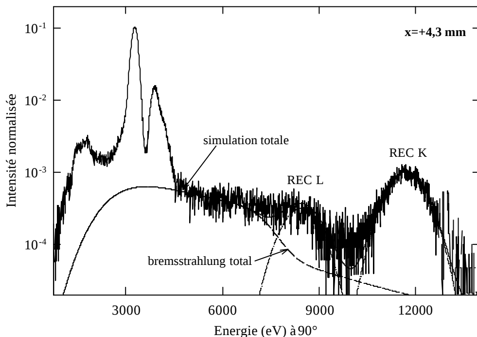
Figure III-5 : Simulation du spectre de bremsstrahlung total et des raies REC-K et REC-L pour un spectre enregistré à 90° avec une cible de 42 µg/cm².
