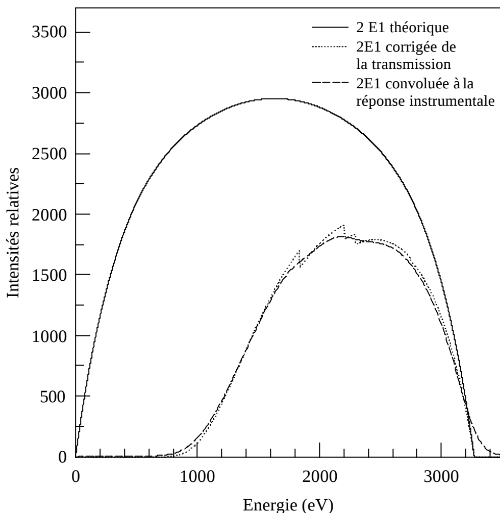
Figure III-7 : Forme spectrale observée par le détecteur Si(Li)(1) de la raie de désexcitation de type 2E1. Comparaison avec la forme spectrale théorique.
