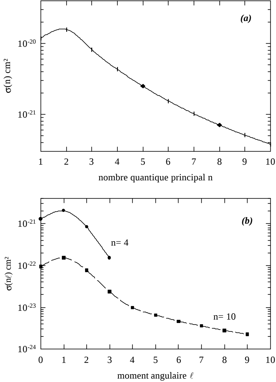
Figure IV-2 : Distributions des sections efficaces de capture pour \text{Ar}^{18+} ( v_p=23 ua) sur C :
