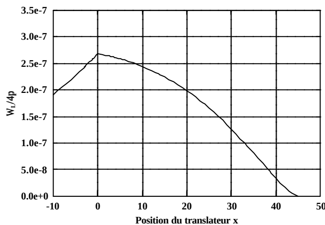
Figure II-23 : Courbe d'évolution de l'angle solide du détecteur Ge en fonction de la position de la cible.
