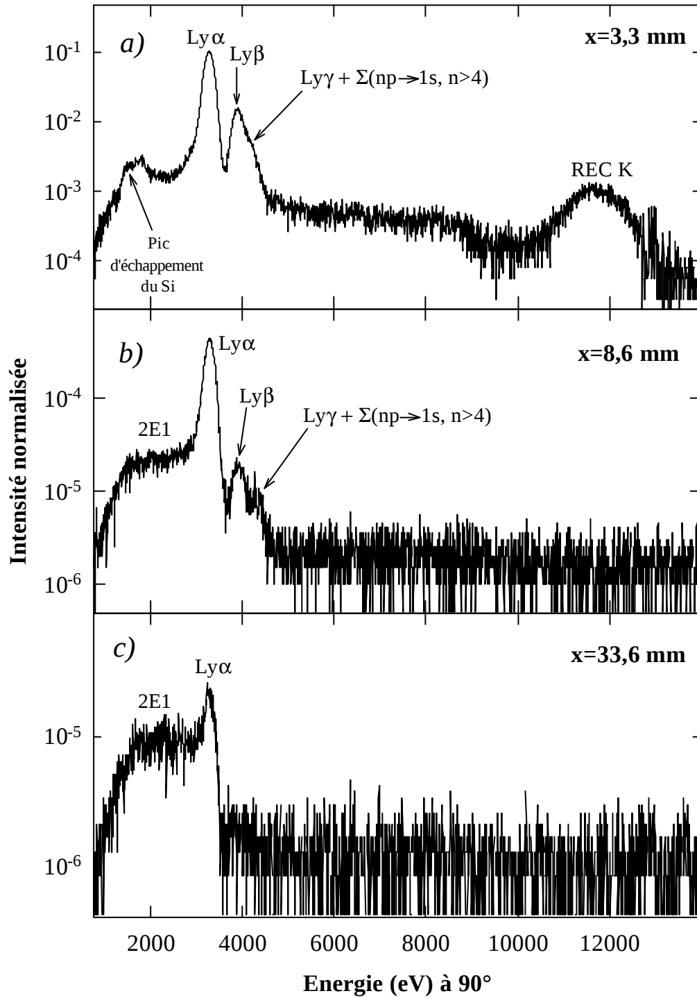
Figure III-1 : Spectres bruts enregistrés par le détecteur Si(Li)(1) (voir montage expérimental) pour une cible de 42 \mu\text{g}/\text{cm}^2 .
