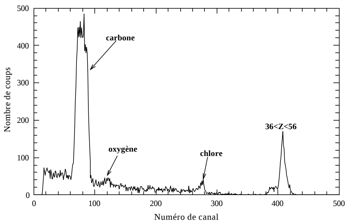
Figure II-6 : Spectre en énergie des particules \alpha rétrodiffusées détectées à 165^\circ pour une cible de 28 \mu\text{g}/\text{cm}^2 de carbone.
