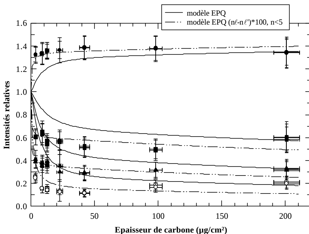
Figure V-28 : Evolution des intensités relatives normalisées des transitions Lyman émises par l' \text{Ar}^{17+} ( v_p=23 ua) avec l'épaisseur de carbone traversée. Pour le modèle EPQ, les sections efficaces d'excitation intracouche dipolaire sont multipliées par 100 pour n=2, 3 et 4 .
