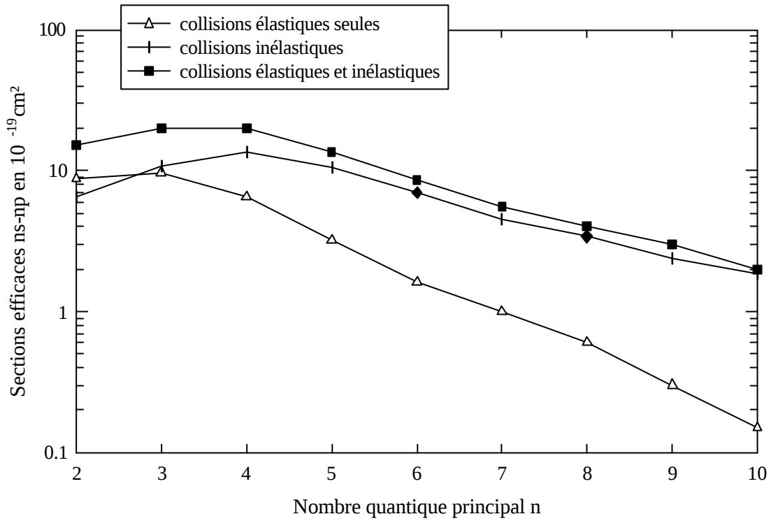
Figure IV-10 : Evolution des sections efficaces d'excitation intracouche ns \rightarrow np de l' Ar^{17+} à v_p=23 ua, extraites du modèle du transport classique (modèle EPC), en fonction du nombre quantique n .
