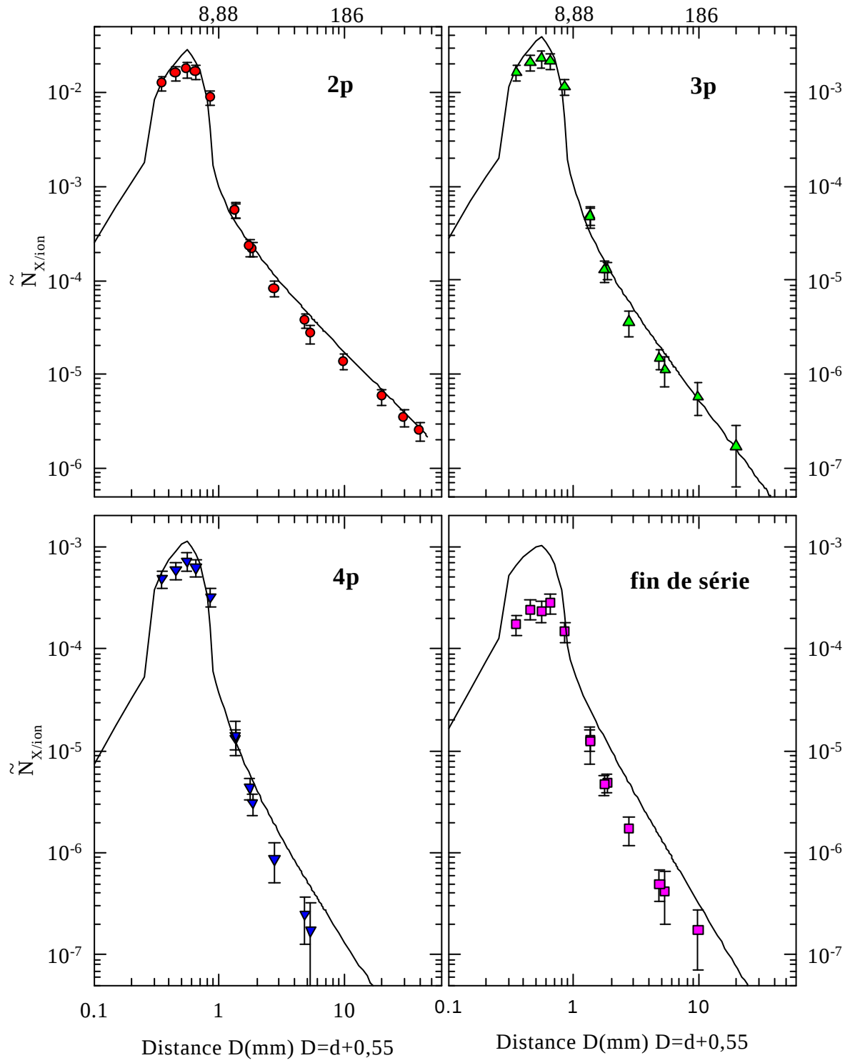
Figure A-Ia-6 : Comparaison modèle EPC - expérience.
