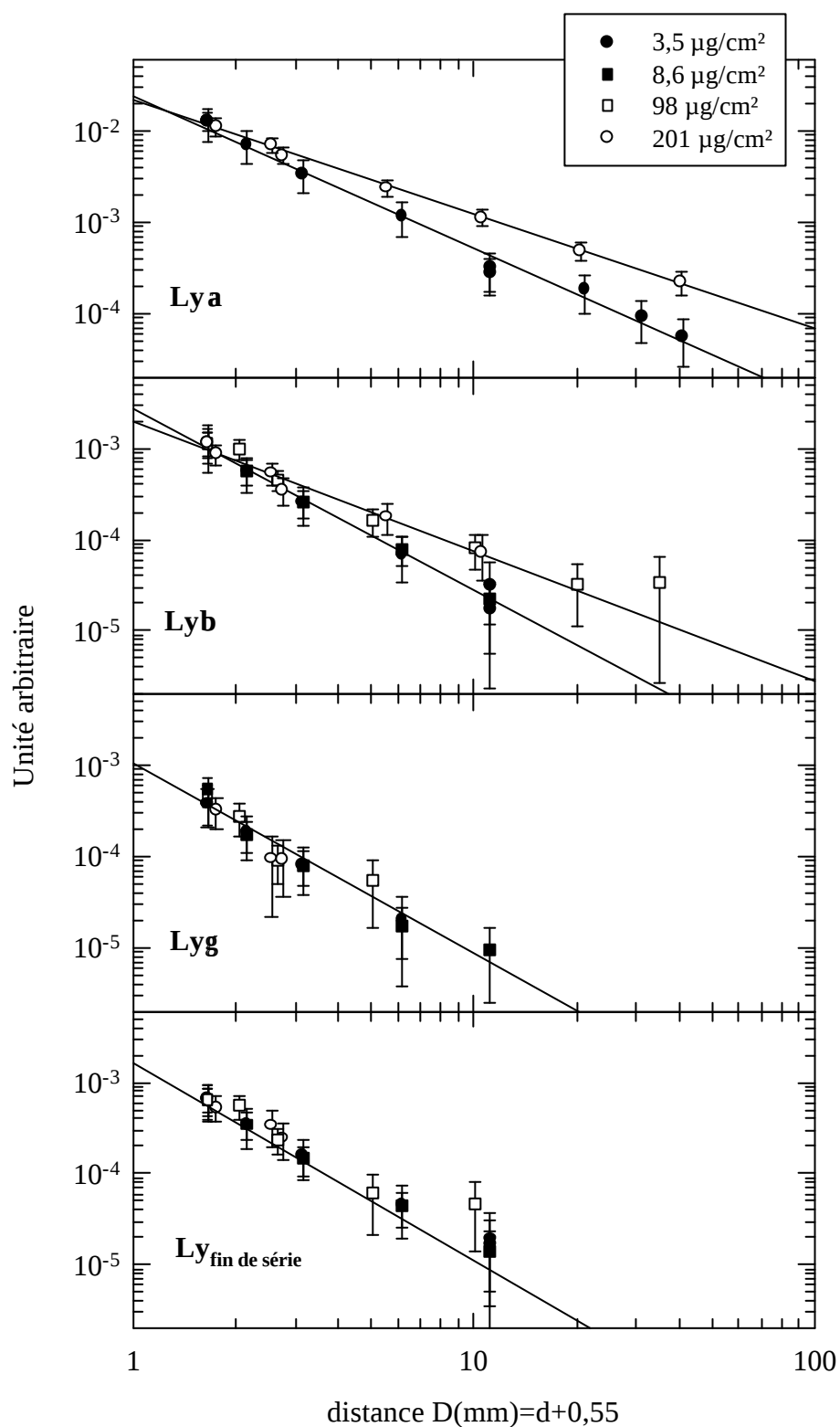
Figure III-20 : Evolution de chaque transition Lyman np observée à partir de d=1,1 mm pour les cibles les plus fines (3,5 et 8,6 \mu\text{g}/\text{cm}^2 ) et pour les cibles les plus épaisses (98 et 201 \mu\text{g}/\text{cm}^2 ). Les points expérimentaux à d=1,1 mm (soit D=1,65 mm) des cibles de 8,6 , 98 et 201 \mu\text{g}/\text{cm}^2 sont normalisés (voir texte).
