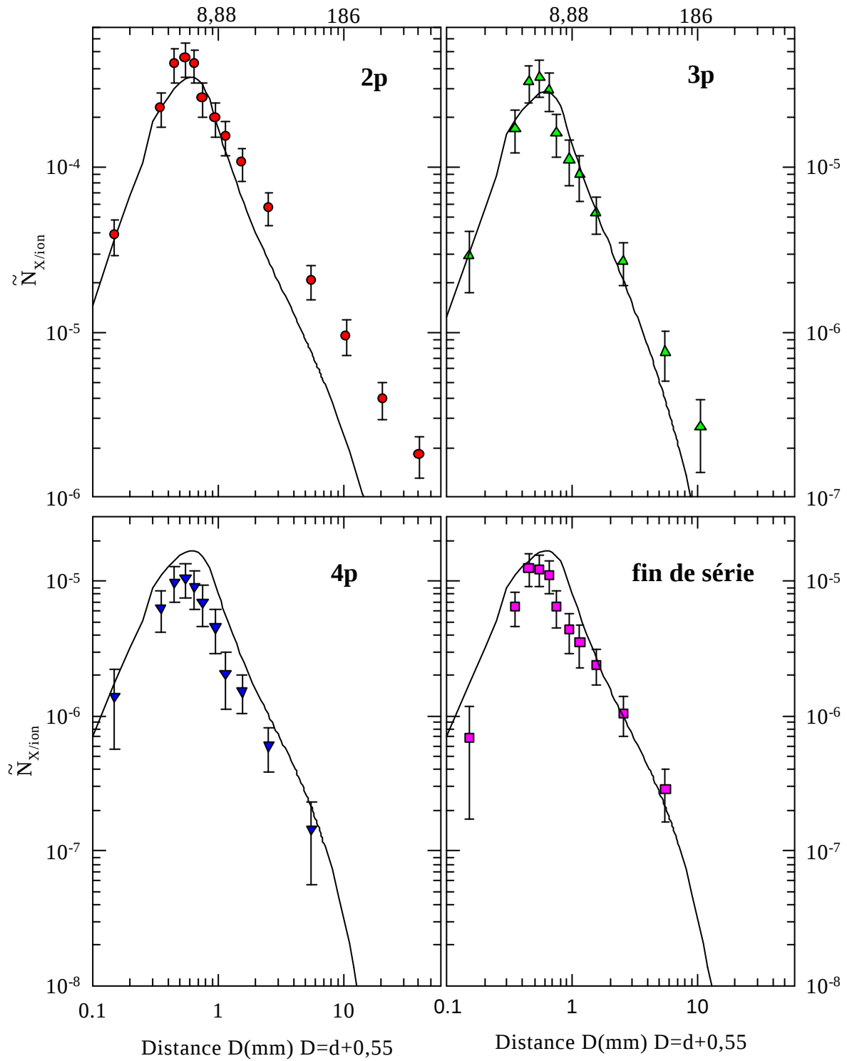
Figure A-Ia-2 : Comparaison modèle EPQ (avec les sections efficaces d'excitation intracouche de type dipolaire augmentées pour n > 5 ) - expérience.
