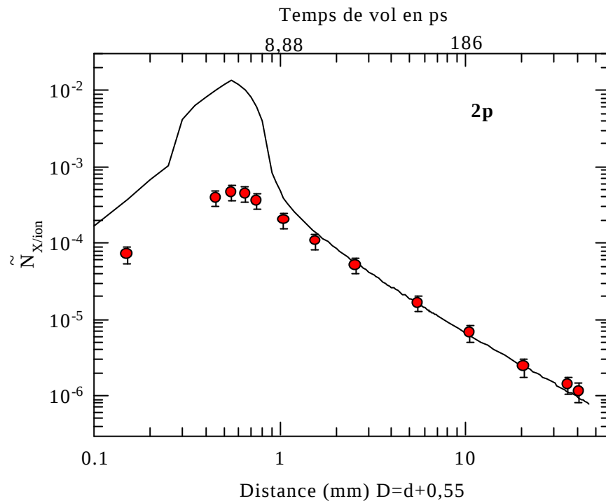
Figure V-5 : Comparaison entre l'évolution expérimentale de l'intensité de la transition Lyman \alpha avec le temps de vol obtenue pour une cible de 12,6 \mu\text{g}/\text{cm}^2 et le modèle EPC corrigé des effets géométriques.
