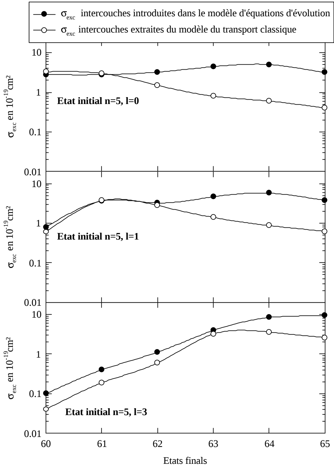
Figure IV-12 : Comparaison des sections efficaces d'excitation intercouche extraites ou introduites dans chacun des deux modèles dans le cas des transitions (n=5, \ell=0) \rightarrow (6\ell') , (n=5, \ell=1) \rightarrow (6\ell') et (n=5, \ell=3) \rightarrow (6\ell') .
