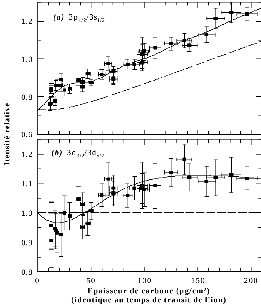
Figure I-7 : Comparaison des modèles avec l'évolution expérimentale des rapports des intensités caractéristiques de (a) 3p_{1/2} \otimes 2s_{1/2}/3s_{1/2} \otimes 2p_{1/2} et (b) 3d_{3/2} \otimes 2p_{3/2}/3d_{5/2} \otimes 2p_{3/2} du Kr^{35+} ( v_p=35 ua) en fonction de l'épaisseur de C. Les modèles sont : (---) modèle collisionnel dans l'espace des phases quantique reflétant l'évolution expérimentale des transitions Lyman ( n\ell \otimes n\ell' augmentées, voir texte) et (—) modèle de réponse collective.
