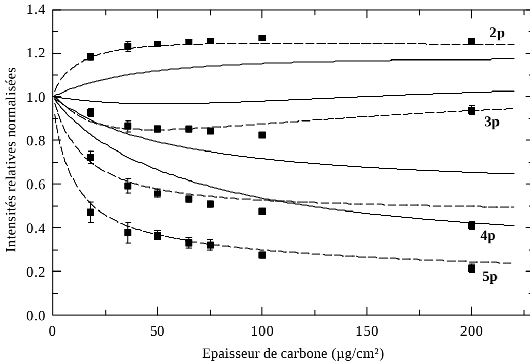
Figure I-6 : Evolution des intensités relatives normalisées des transitions Lyman np @ 1s émises en vol par des ions \text{Kr}^{35+} ( v_p=35 ua) en fonction de l'épaisseur de carbone traversée. Les courbes correspondent au modèle d'équation d'évolution : (—) avec sections efficaces d'ionisation et d'excitation intracouche dipolaires ; (---) avec sections efficaces d'ionisation et sections efficaces d'excitation intracouche dipolaires augmentées (voir texte).
