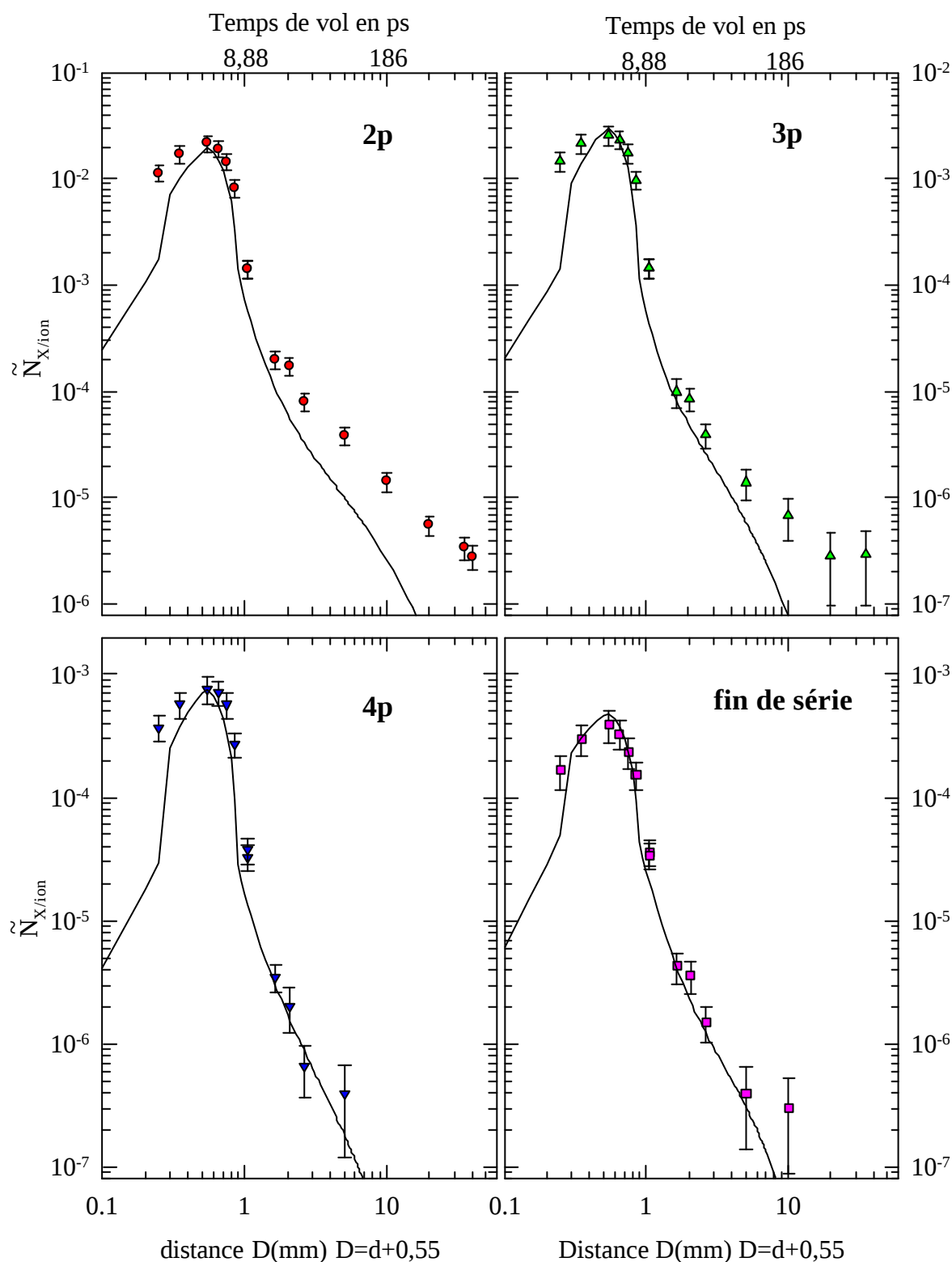
Figure V-15 : Comparaison mod\u00e8le EPQ (avec les sections efficaces d'excitation intracouche de type dipolaire augment\u00e9es pour n > 5 ) - exp\u00e9rience.
