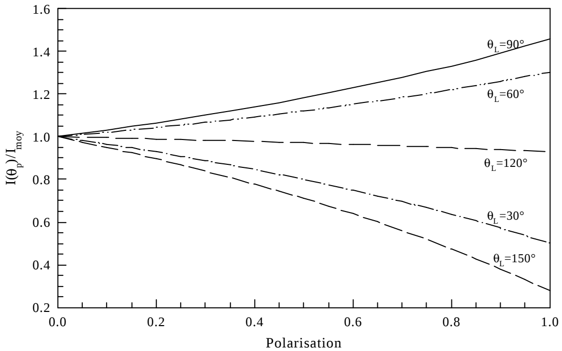
Figure II-14 : Evolution du rapport I(\mathbf{q}_p)/I_{\text{moy}} pour différents angles d'observation en fonction de la polarisation P du rayonnement.
