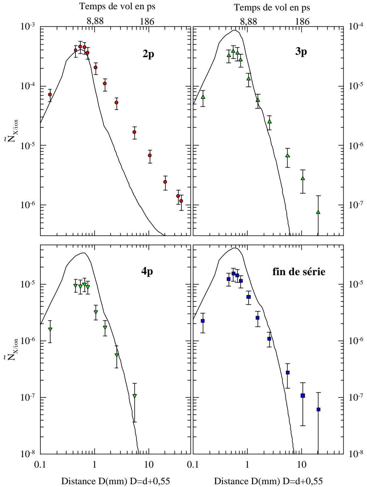
Figure V-11 : Comparaison modèle EPQ - expérience.
