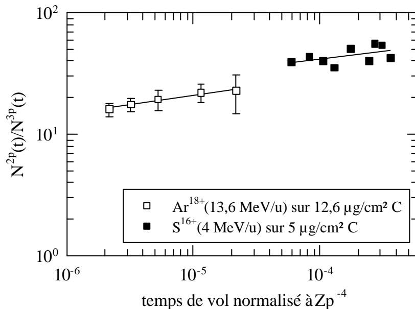
Figure V-9 : Evolution des rapports d'intensités N^{(2p \text{ @s})}(t) / N^{(3p \text{ @s})}(t) avec le temps de vol pour les collisions S^{16+} ( v_p=13 ua) @C (Rothermel et al, 1983) et Ar^{18+} ( v_p=23 ua) @C. Le temps de vol est normalisé à Z_p^{-4} .
