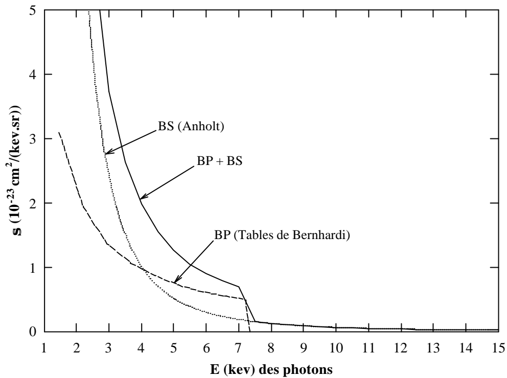
Figure III-3 : Evolution du bremsstrahlung primaire, secondaire et du bremsstrahlung total à 90^\circ en fonction de l'énergie.
