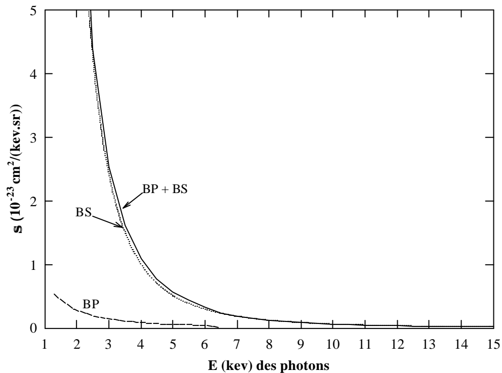
Figure III-4 : Evolution du bremsstrahlung primaire, secondaire et du bremsstrahlung total à 150^\circ en fonction de l'énergie.
