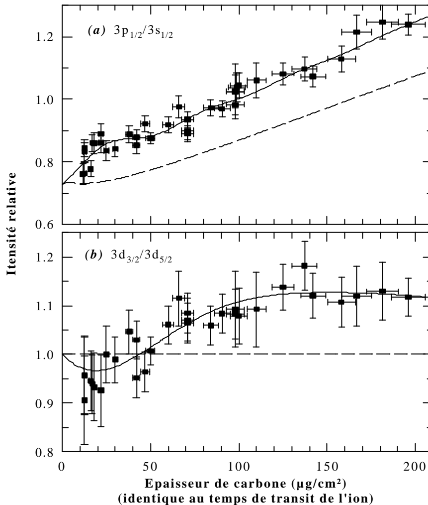
Figure I-7 : Comparaison des modèles avec l'évolution expérimentale des rapports des intensités caractéristiques de (a) 3p_{1/2}/3s_{1/2} et (b) 3d_{3/2}/3d_{5/2} du Kr^{35+} ( v_p=35 ua) en fonction de l'épaisseur de C. Les modèles sont : (---) modèle collisionnel dans l'espace des phases quantique reflétant l'évolution expérimentale des transitions Lyman ( nl/nl' augmentées, voir texte) et (—) modèle de réponse collective.
