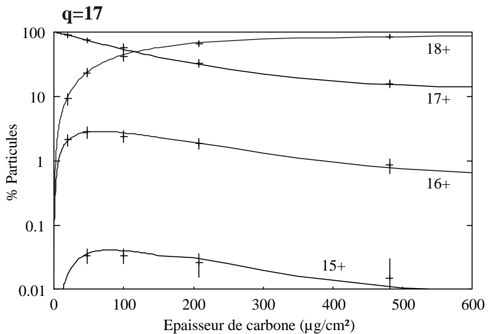
Figure II-10 : Evolution de la distribution d'état de charge pour la collision \text{Ar}^{17+} @ \text{C} à 13,6 MeV/u en fonction de l'épaisseur de cible. Les lignes continues correspondent aux valeurs données par le code ETACHA
