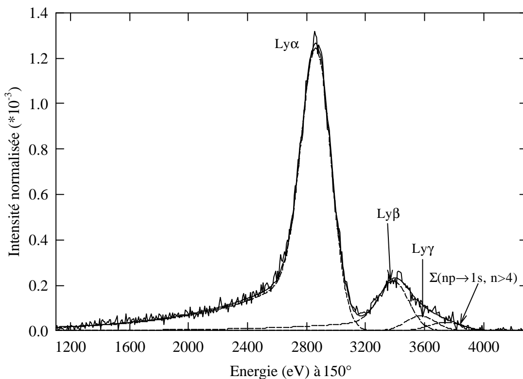
Figure III-11 : Exemple de décomposition d'un spectre enregistré par le détecteur Ge pour une cible de carbone de 42 \mu\text{g}/\text{cm}^2 .
