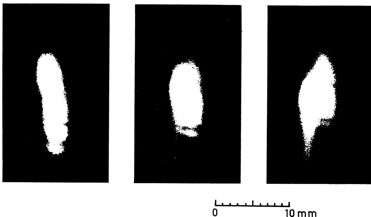
Figure 5 - Coupes du faisceau, 40cm après la fente d'entrée, pour trois valeurs de l'écart en tension entre le collimateur et les plaques défléctrices verticales (Z1, Z2). A gauche, écart maximum ; à droite, écart nul.
