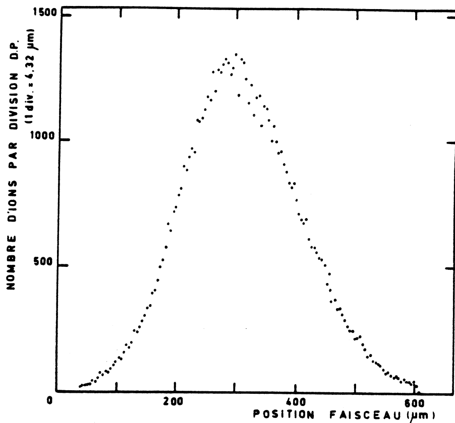
Figure 12 - Structure du faisceau observée au niveau de F.E.. La largeur de ce faisceau à mi-hauteur est de 233μm.
