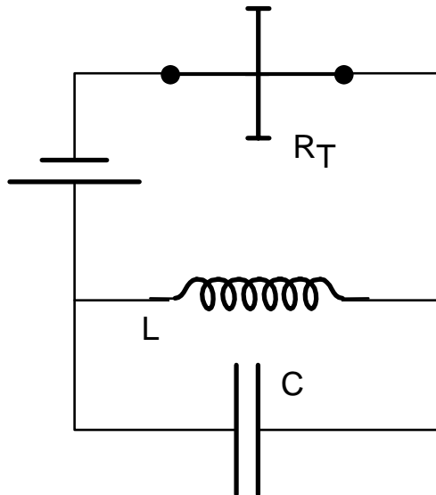
Fig. 5.7. Environnement électromagnétique d’une jonction tunnel connectée à une impédance. La solution de ce cas simple est la brique élémentaire sur laquelle est construite la théorie du blocage de Coulomb.
