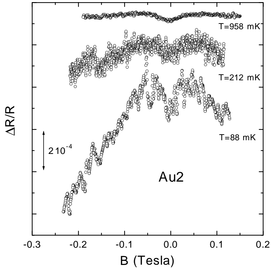
Fig. 3.7. Les échantillons d'or Au1 et Au2 présentent une magnétorésistance négative anormale à basse température pour des champs magnétiques relativement importants par rapport aux corrections de localisation faible. Au-dessus de 1 K cet effet est négligeable.
