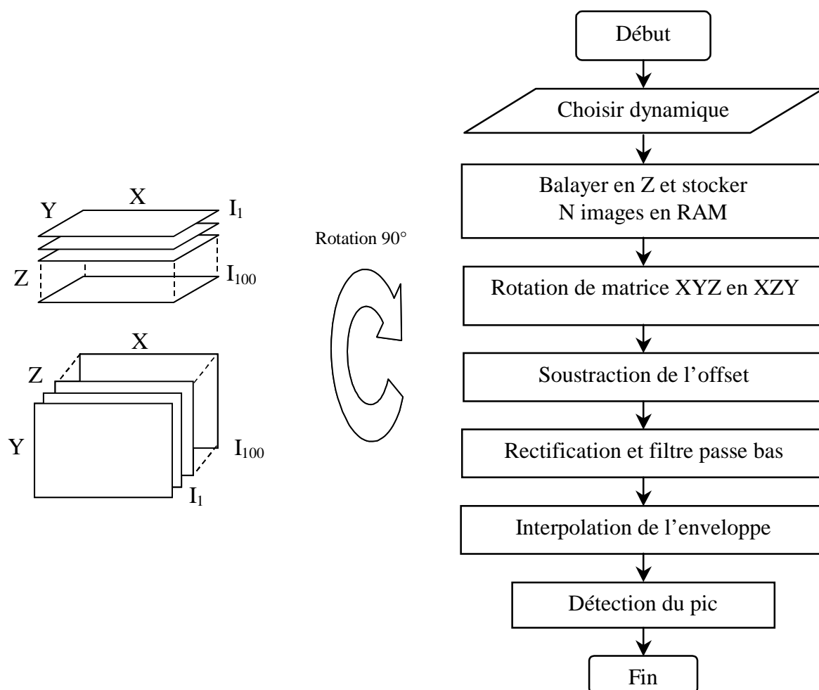
Figure 2.15 : Algorithme de démodulation adapté au traitement d'images sous Labview.
