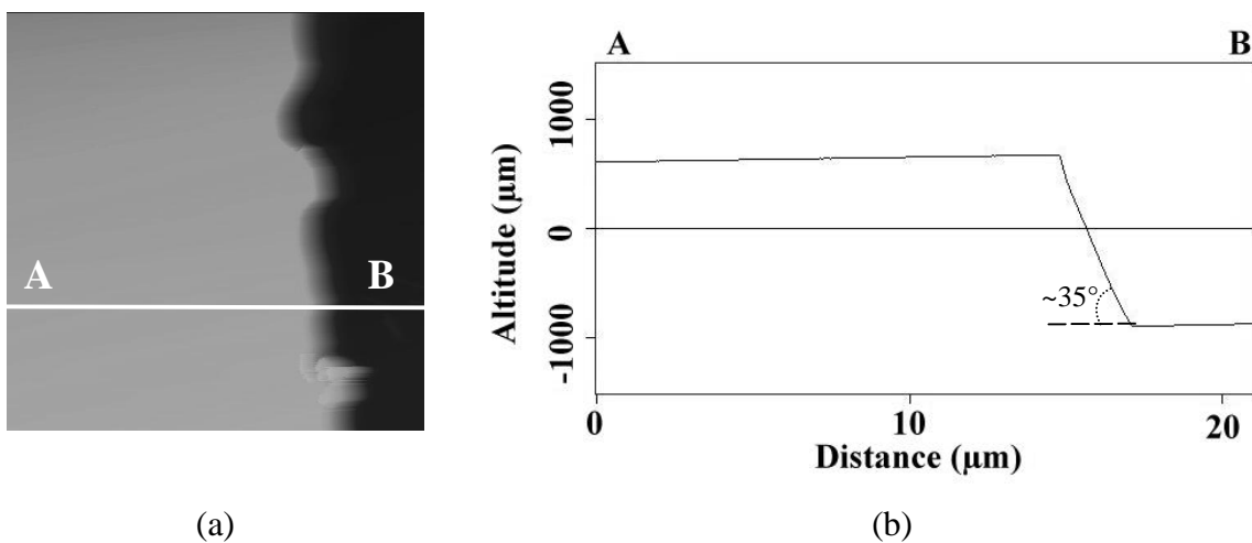
Figure 5.7 : Image (a) et profil (b) AFMI d'une marche en Si 'nue' (échantillon MAR1) ( h=1,56 \mu\text{m} ).
