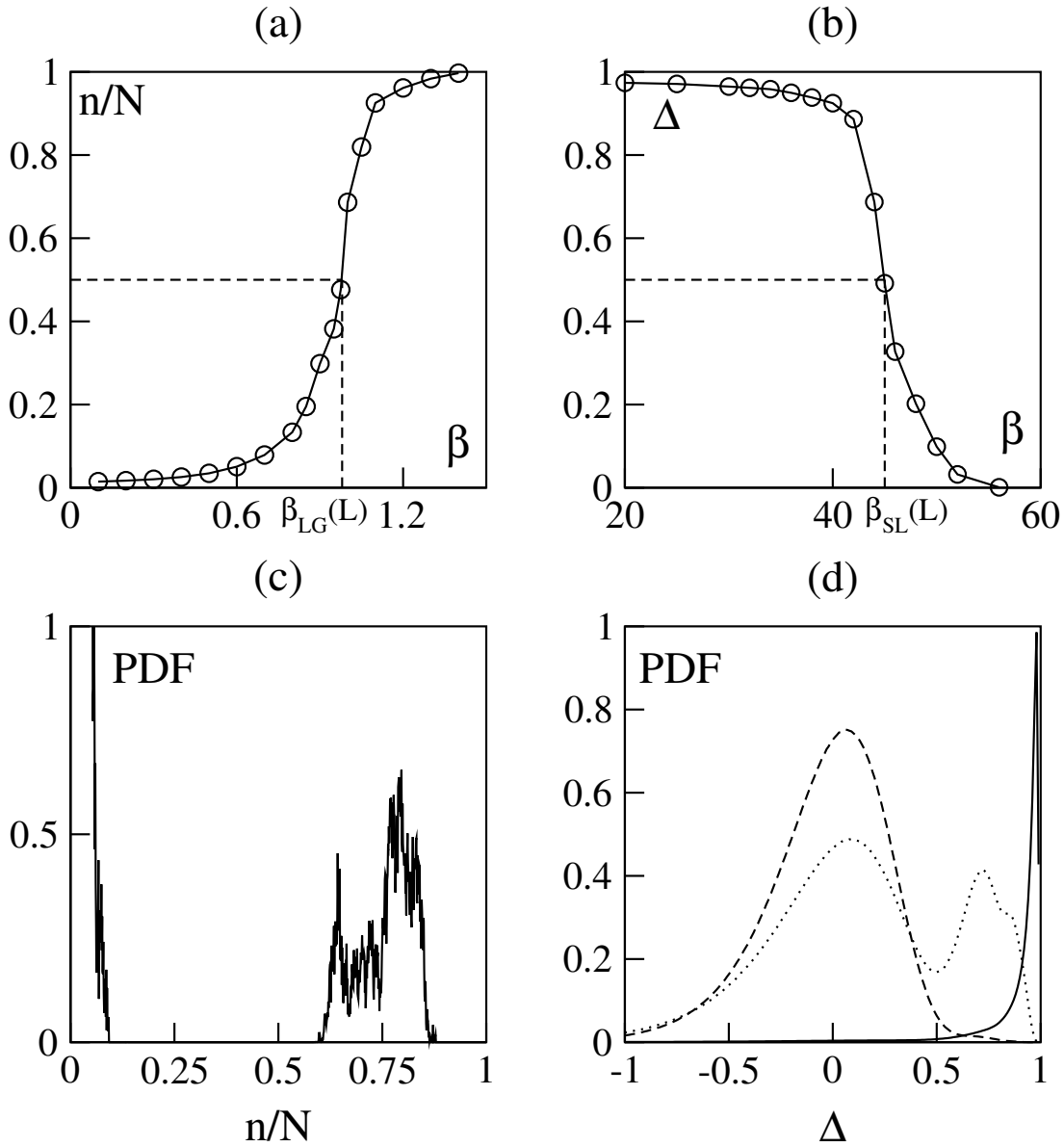
FIG. 6.5 – Nature des transitions de cohésion. Nous nous sommes placés à \rho = 1/16 , L = 128 , \alpha = 1,0 , c'est-à-dire en phase fixe, \eta = 1,0 et avec le modèle Br2-Fh. (a) paramètre d'ordre de la transition gaz-liquide. (b) paramètre d'ordre de la transition liquide-solide. Nous avons fait figurer les seuils des transitions \beta_{GL}(L) et \beta_{LS}(L) . (c) distribution des masses des différents agrégats au point de coexistence gaz-liquide, \beta = 1,0 . (d) distribution du paramètre d'ordre \Delta le long de la transition du liquide vers le solide, \beta = 36,0 (trait continu), \beta = 48,0 (trait pointillé) et \beta = 60,0 (trait discontinu).
