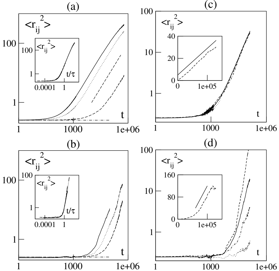
FIG. 6.3 – Variations de l'écart relatif moyen. 10000 animoïdes ont été suivis au cours du temps sur un espace L = 400 , \rho = 1/16 le long des transitions ((a) et (b)) ou en fonction de leur localisation dans le troupeau ((c) et (d)), en échelle logarithmique. Pour chacune des courbes, le modèle Br2-Fh a été utilisé avec un bruit constant \eta = 1,0 . (a) gouttelette fixe ( \alpha = 1,0 ) du liquide vers le solide (du haut vers le bas : \beta = 25,0, 35,0, 45,0 et 150,0 ). La ligne discontinue a une pente unité. (b) gouttelette en mouvement ( \alpha = 3,0 ) du liquide vers le solide (du haut vers le bas : \beta = 40,0, 55,0, 75,0 et 150,0 ). En encart : renormalisation des courbes par le temps de piégeage. (c) gouttelette liquide fixe, \alpha = 1,0 et \beta = 40,0 . (d) gouttelette liquide volante, \alpha = 3,0 et \beta = 40,0 . Dans ces deux dernières figures, les lignes continues concernent la globalité du troupeau, les lignes pointillées la région centrale, les lignes discontinues la tête, les traits mixtes l'arrière du troupeau. En encart, les mêmes courbes en échelle linéaire pour la région de tête, la droite continue sert de comparaison.
