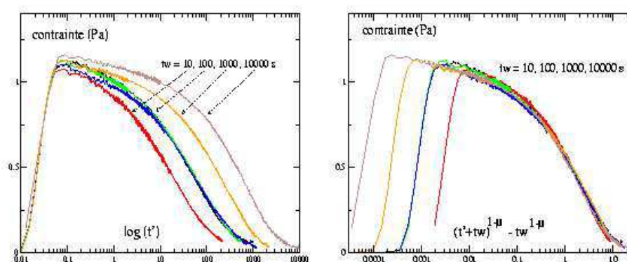
Fig. 1.4: Module de relaxation élastique d'une suspension concentrée de sphères de silice pour différents âges du système. L'âge est défini comme le temps écoulé depuis la cessation du fort précisaillement. La décroissance du module est d'autant plus lente que le système est vieux. L'ensemble des courbes peut se remettre à l'échelle ( figure (b)) [34].
