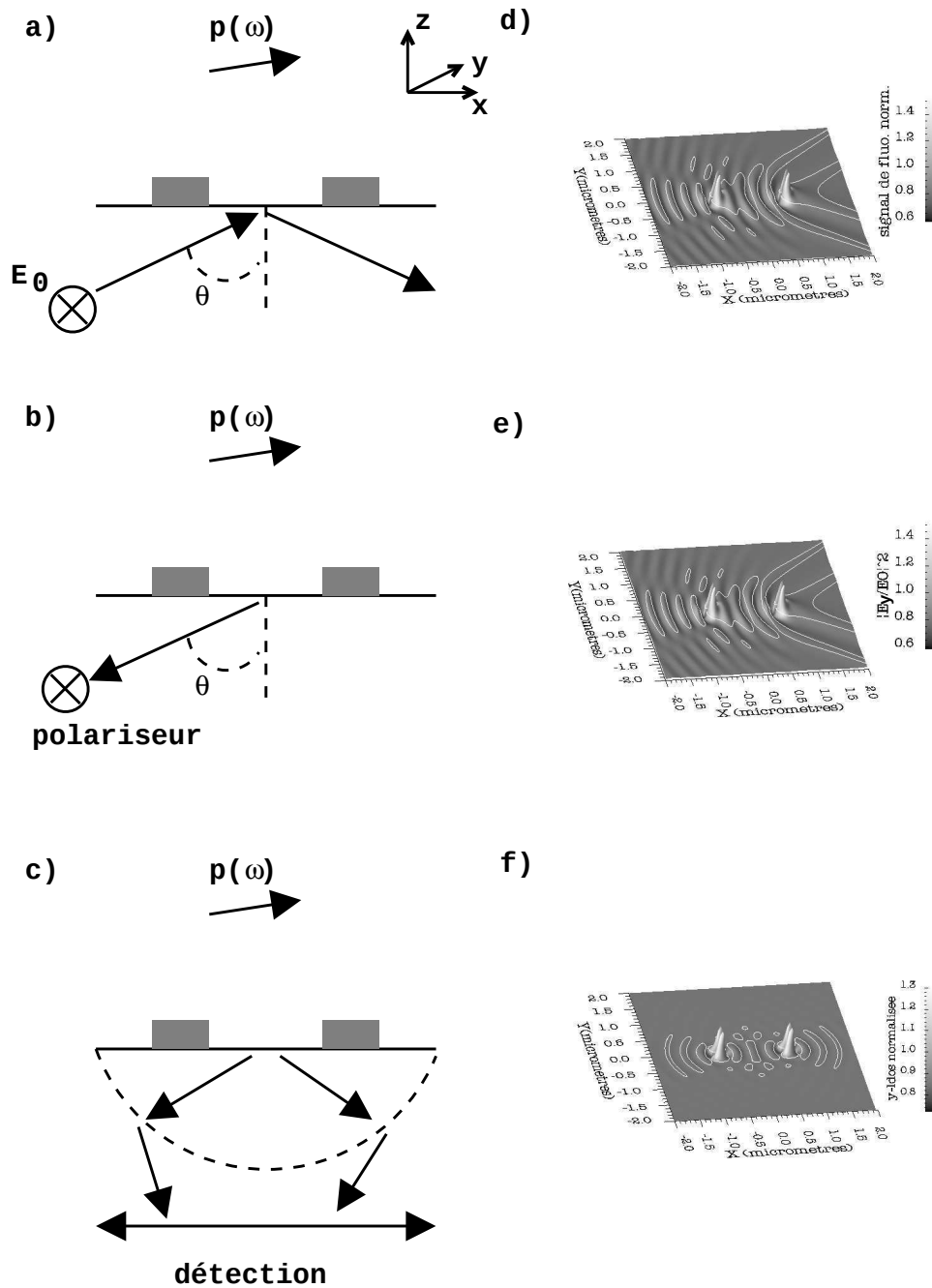
FIG. 2 – Différentes configurations de microscopes optiques en champ proche. Le dipôle \mathbf{p}(\omega) est orienté selon l'axe Y . a) PSTM, le champ incident est polarisé TE, b) SNOM en lumière interdite équivalente et c) SNOM à grand angle de détection. Les images calculées pour chacune de ces configurations sont représentées figures d), e) et f) respectivement ( \theta = 55^\circ et \lambda_0 = 630 nm).
