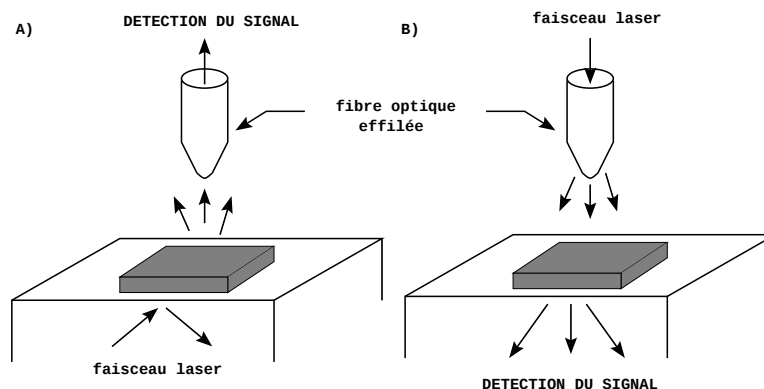
FIG. 2 – Montages de microscope en champ proche optique. a) Mode détection ; l'onde de surface est détectée localement à l'aide d'une fibre optique effilée au-dessus de la surface (PSTM). b) Mode illumination ; l'objet est illuminé avec l'onde non radiative formée à l'extrémité de la pointe. Le signal est détecté par transmission sous la surface (SNOM).
