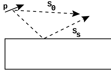
FIG. 5 – Représentation diagrammatique des deux contributions S_0 et S_s qui composent la susceptibilité du champ S_{surf} associée à la surface.
