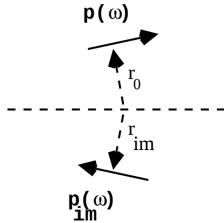
FIG. 6 – a) Rayonnement dipolaire en présence d’une surface. b) Système équivalent. La surface est remplacée par un dipôle image (voir le texte pour les détails).
