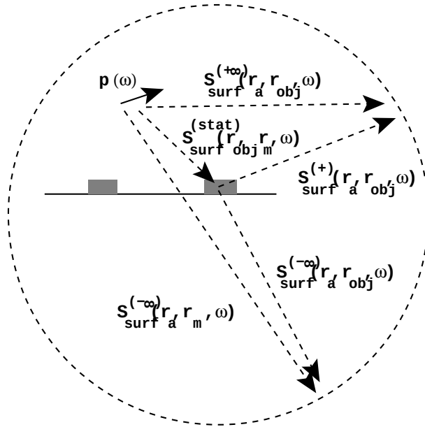
FIG. 18 – Différentes formes approchées de la susceptibilité du champ de la surface. La forme asymptotique S_{surf}^{(+\infty)}(\mathbf{r}, \mathbf{r}', \omega) de la susceptibilité du champ dans la zone d'onde au-dessus du système complète les formes déjà présentées sur la figure (14).
