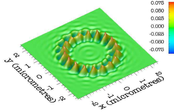
FIG. 24 – Cartes des termes corrélés. a) \omega_0^2 \Delta n_{xy}(\mathbf{r}_m, \omega_0) , b) \omega_0^2 \Delta n_{xz}(\mathbf{r}_m, \omega_0) , c) \omega_0^2 \Delta n_{yz}(\mathbf{r}_m, \omega_0) . Les cartes sont calculées 75 nm au-dessus du corral de la figure (24) à la longueur d'onde \lambda_0 = 2\pi c/\omega_0 = 594 nm. Ces termes ne sont pas des observables mais contribuent au signal détecté en accord avec la relation (III.46).
