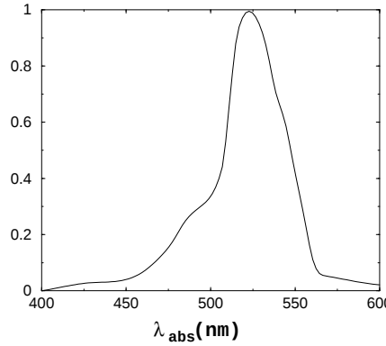
FIG. 5 – Profil spectral expérimental d'absorption de la rhodamine 6G. L'absorption est maximale à la longueur d'onde d'excitation \lambda_1 = 520 nm.
