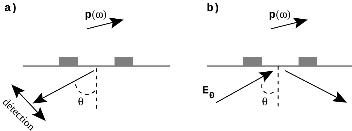
FIG. 1 – a) SNOM en lumière interdite. b) PSTM équivalent ; le faisceau incident E_0 est non polarisé.
