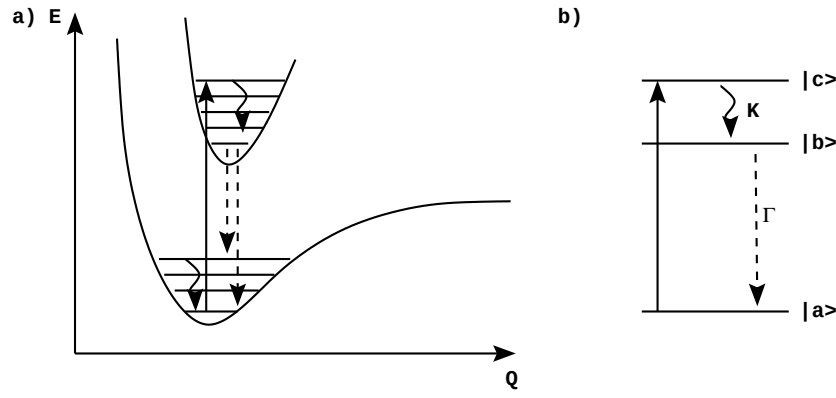
FIG. 4 – a) Représentation schématisée des niveaux d'une molécule fluorescente. La flèche en trait continu indique l'excitation par le champ proche, celles en pointillés la fluorescence et les flèches ondulées représentent la relaxation vibrationnelle. b) Simplification à trois niveaux.
