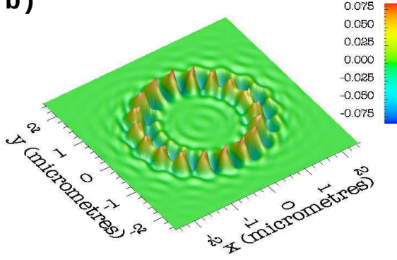
FIG. 24 – Cartes des termes corrélés. a) \omega_0^2 \Delta n_{xy}(\mathbf{r}_m, \omega_0) , b) \omega_0^2 \Delta n_{xz}(\mathbf{r}_m, \omega_0) , c) \omega_0^2 \Delta n_{yz}(\mathbf{r}_m, \omega_0) . Les cartes sont calculées 75 nm au-dessus du corral de la figure (24) à la longueur d'onde \lambda_0 = 2\pi c/\omega_0 = 594 nm. Ces termes ne sont pas des observables mais contribuent au signal détecté en accord avec la relation (III.46).
