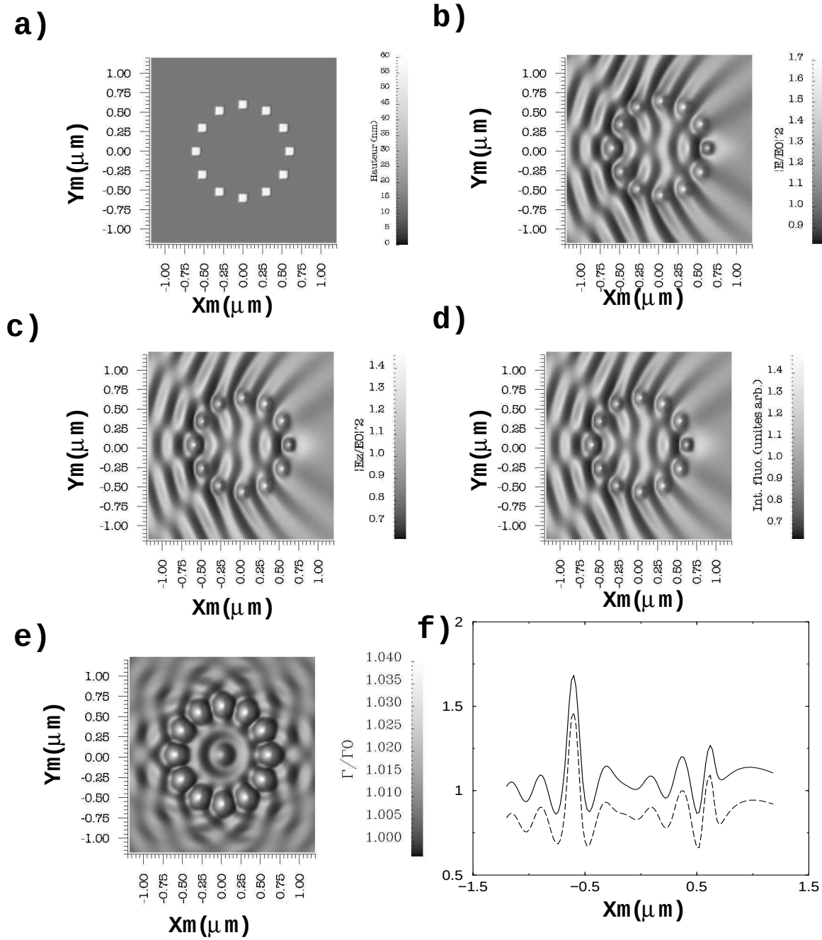
FIG. 8 – Simulation du signal détecté avec un PSTM à sonde moléculaire. Le champ incident est polarisé TM. a) Géométrie de l'échantillon. b) Intensité normalisée au-dessus de l'échantillon (le facteur de normalisation est donné par l'intensité électrique |E_0|^2 en absence d'échantillon sur la surface). c) Produit quadratique normalisé |E_z/E_0|^2 de la composante selon Z du champ proche électrique. d) Intensité de fluorescence (unités arbitraires). e) Elargissement du niveau excité de la molécule en fonction de sa position. f) Coupes le long de l'axe X de |E_z/E_0|^2 (courbe continue) et du signal de fluorescence (courbe en pointillés, décalée pour plus de lisibilité). Le dipôle de fluorescence est orienté selon l'axe Z et balaye la surface 40 nm au-dessus des plots.
