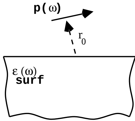
FIG. 6 – a) Rayonnement dipolaire en présence d’une surface. b) Système équivalent. La surface est remplacée par un dipôle image (voir le texte pour les détails).
