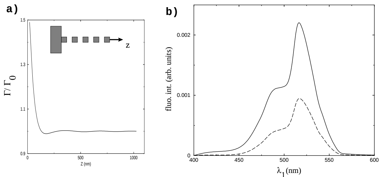
FIG. 17 – a) Elargissement du niveau excité de la molécule en fonction de sa distance au guide. b) Spectre d'excitation pour deux positions de la molécule : Z_m = 20 nm (courbe continue) et Z_m = 200 nm (courbe en pointillés).
