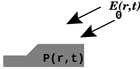
FIG. 1 – Un objet de forme quelconque est illuminé par le champ électrique E_0(\mathbf{r}, t) . On cherche à déterminer le champ électrique E(\mathbf{r}, t) qui en résulte. La matière est décrite par le vecteur polarisation P(\mathbf{r}, t) .
