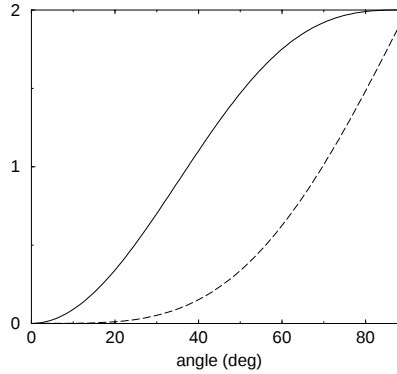
FIG. 7 – Variation angulaire des deux contributions du signal détecté présentes dans \mathcal{D}_0(\theta_{obs}) (voir la relation (III.20)). courbe continue : (2 - 2 \cos^3 \theta_{obs}) et (courbe en pointillée : (2 - 3 \cos \theta_{obs} + \cos^3 \theta_{obs}) ).
