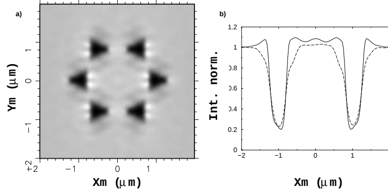
FIG. 21 – Carte (a) et coupe selon l'axe X (courbe en continu de la figure (b)) de l'intensité transmise dans l'angle solide \Omega = 2\pi str. La courbe en pointillés de la figure (b) représente la coupe de l'intensité transmise dans l'angle solide \Omega = 0.38 str ( \Delta\theta = \pi/5 ).
