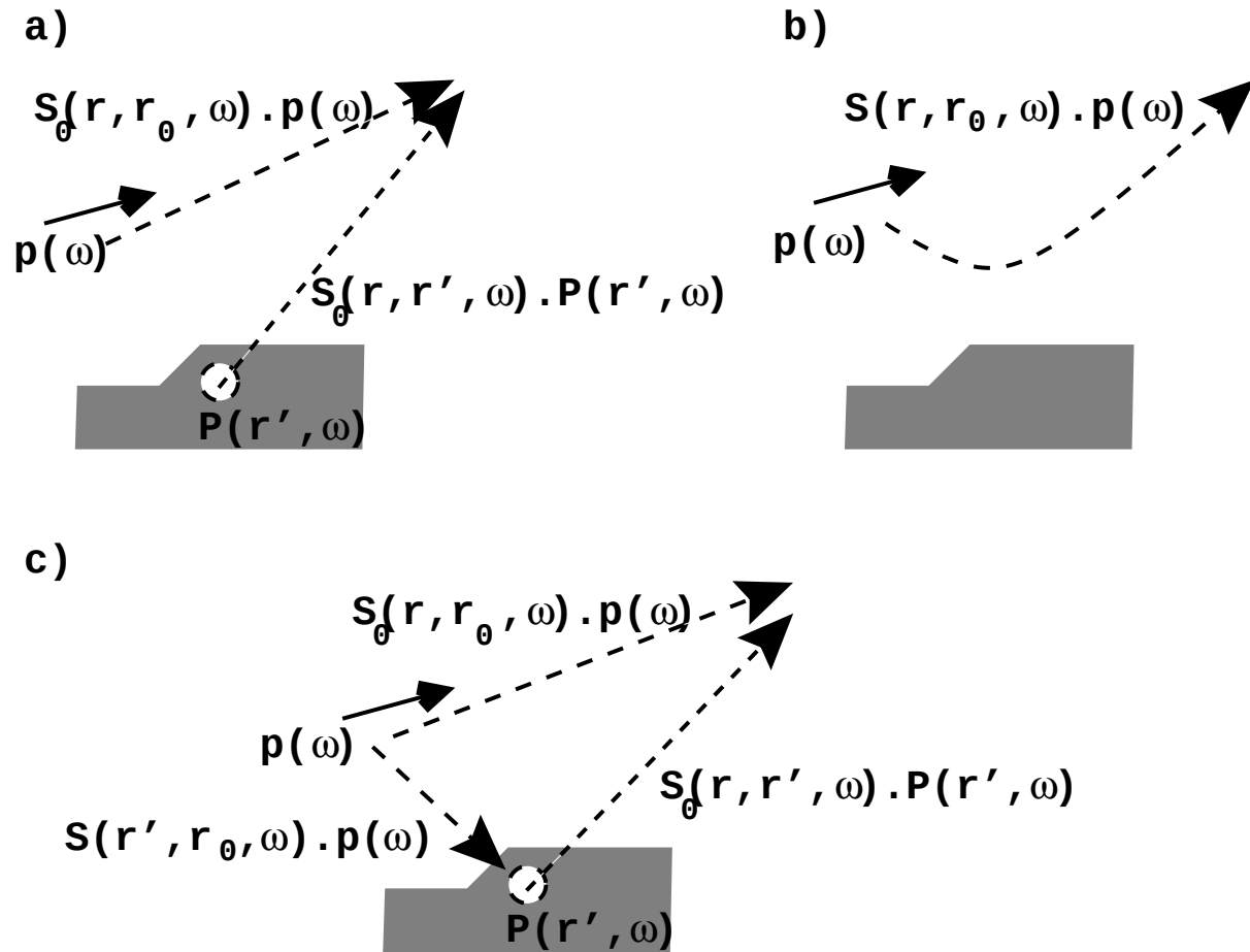
FIG. 3 – Champ électrique rayonné par un dipôle \mathbf{p}(\omega) en présence de matière. Différents points de vue. a) Rayonnement dipolaire et rayonnement dipolaire induit. b) Rayonnement dipolaire perturbé par la matière. c) Combinaison de a) et b).
