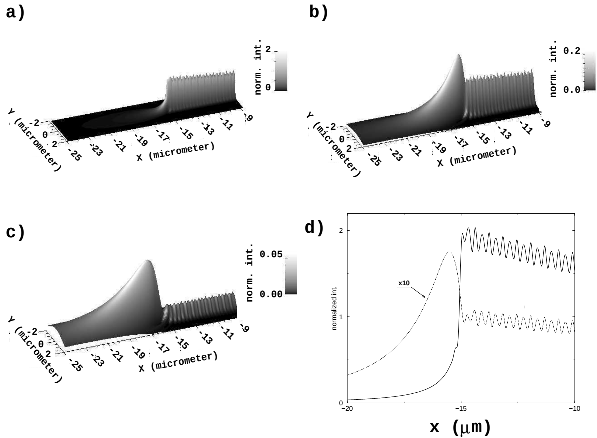
FIG. 7 – Intensité calculée à différentes hauteurs. a) Z_{obs} = 200 nm, b) Z_{obs} = 500 nm et c) Z_{obs} = 800 nm. d) Coupe selon l'axe X de l'intensité calculée 200 nm au-dessus de la surface (courbe continue) et 500 nm au-dessus de la surface (courbe en pointillés).
