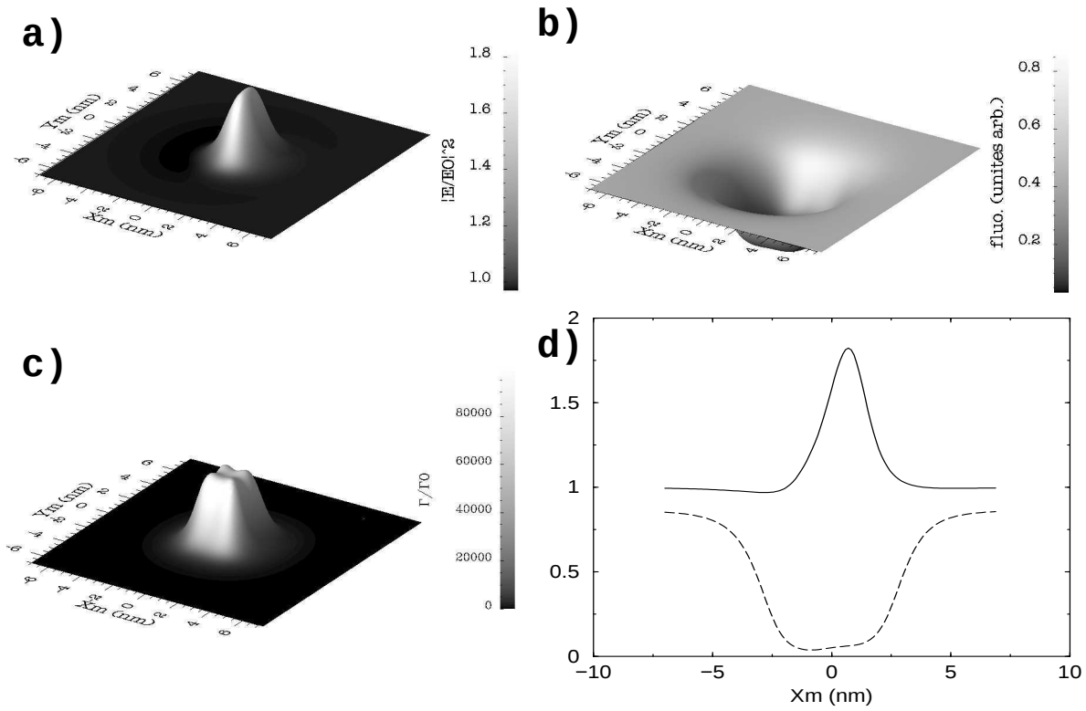
FIG. 11 – a) Intensité normalisée au-dessus du plot d'or. b) Intensité de fluorescence (unités arbitraires). c) Elargissement du niveau excité de la molécule en fonction de sa position. d) Coupes de l'intensité (courbe continue) et du signal de fluorescence (courbe en pointillée). Le champ incident est polarisé TM. Le dipôle de fluorescence est orienté selon l'axe Z et balaye la surface 1 nm au-dessus du plot.
