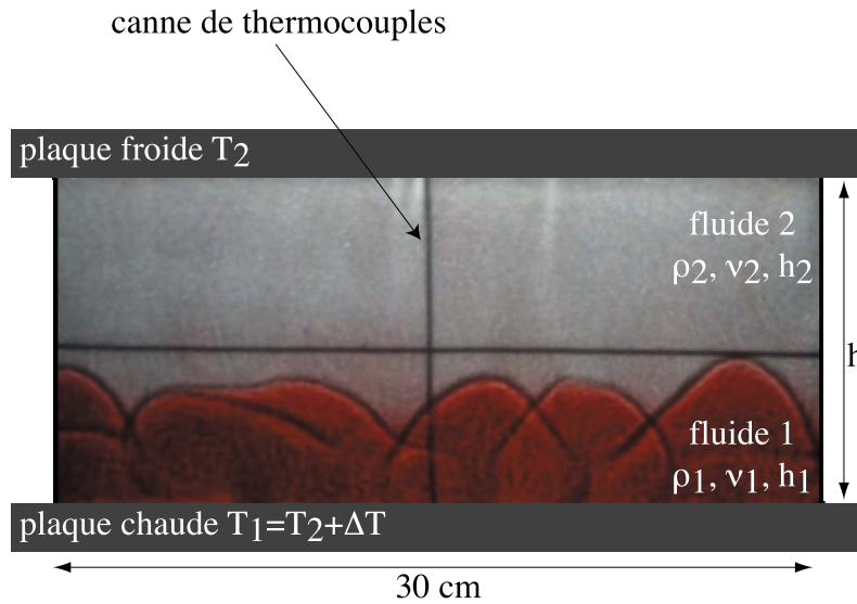
FIG. 3.1 – Dispositif expérimental.
