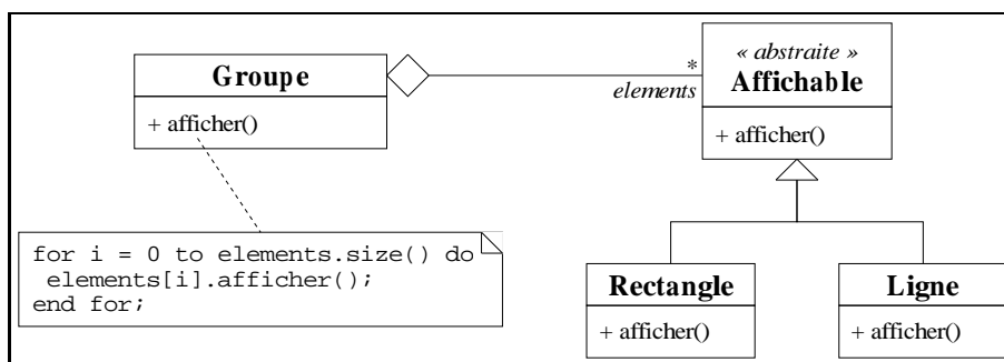
Figure 7.20: Un autre exemple d'héritage.
