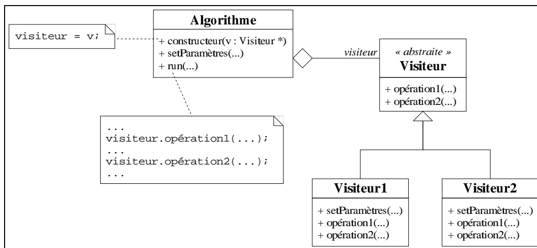
Figure 8.9: Un exemple d'extension d'un algorithme par visiteur abstrait.
