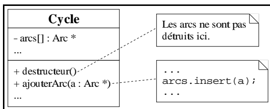
Figure 7.12: Un exemple d'implémentation d'une agrégation.
