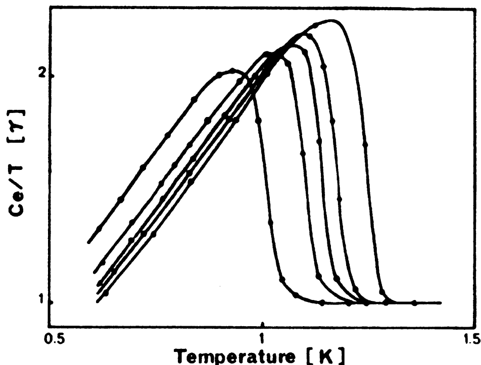
Figure 1-2 : Influence du désordre des anions sur l'état supraconducteur du (TMTSF)_2ClO_4 . La transition métal-supraconducteur à B=0 est présentée dans un diagramme C_e/T vs T , pour cinq vitesses de refroidissement : dT/dt = 3, 12, 35, 85 et 325 K/h. (La température critique ainsi que le saut de la chaleur spécifique décroissent de façon monotone de 3 à 325 K/h) [Réf. P7].
