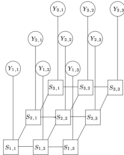
FIG. 1.9 – La structure des modèles de champ de Markov cachés.
