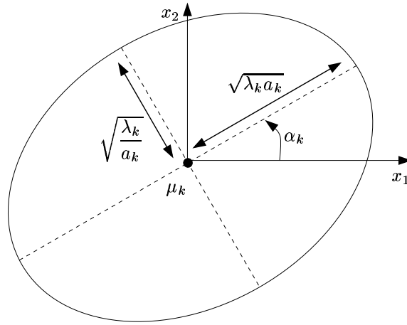
FIG. 3.1 – Interprétation géométrique de la décomposition spectrale. La quantité \lambda_k représente le volume de l'ellipse de concentration, a_k = A_k(1,1) détermine sa forme et l'angle \alpha_k de la matrice de rotation D_k détermine son orientation.
