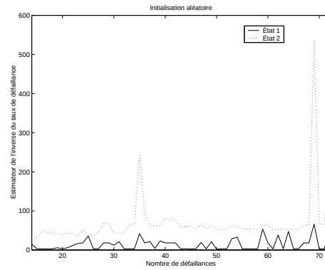
FIG. 3.14b). Initialisation aléatoire
