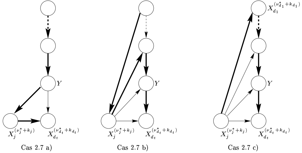
FIG. 2.7 – Insertion d'un sommet dans un chemin passant par les sommets X_{d_1}^{(\nu_{d_1}^*+k_{d_1})}, \dots, X_{d_t}^{(\nu_{d_t}^*+k_{d_t})} adjacents à la source S_0 . Dans le cas 2.7. a), le t+1 ème sommet est inséré entre Y et le dernier sommet du chemin. Dans le cas 2.7. b), le t+1 ème sommet est inséré après le premier ancêtre de X_j^{(\nu_j^*+k_j)} (dans le chemin représenté) parent de X_{d_t}^{(\nu_{d_t}^*+k_{d_t})} . Dans le cas 2.7. c), le t+1 ème sommet est inséré avant le premier sommet X_{d_1}^{(\nu_{d_1}^*+k_{d_1})} du chemin. Le chemin obtenu est tracé en gras. Sa longueur est augmentée de 1.
