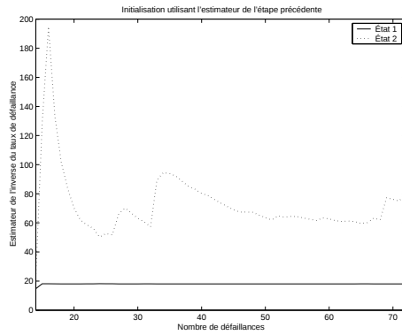
FIG. 3.14a). Initialisation non aléatoire
