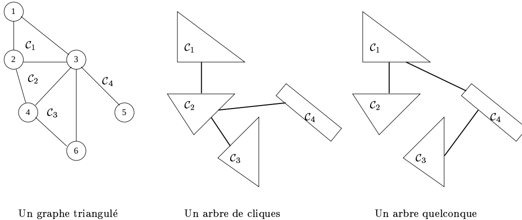
FIG. 1.13 – La notion d'arbre de jonction
