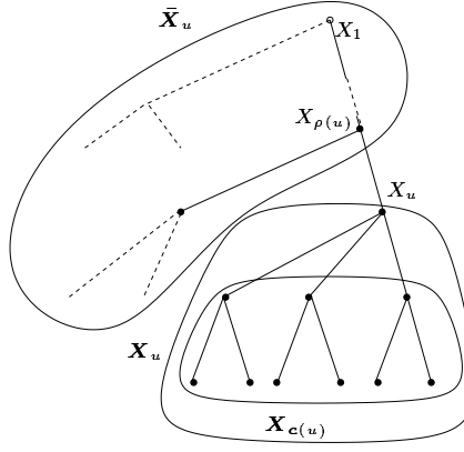
FIG. 2.13 – Notations utilisées pour désigner des sous-arbres.
