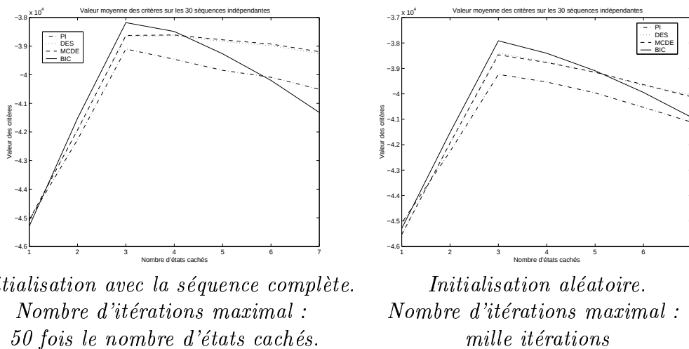
FIG. 3.7 – Moyenne, sur les 30 séquences simulées, des quatre critères considérés ci-dessus, en fonction du nombre d'états cachés (en abscisse). Les séquences sont générées suivant le modèle de séparation la plus forte des composants.
