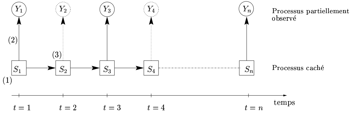
FIG. 3.3 – Suppression des observations d'indice pair dans une chaîne de Markov cachée. Le processus correspondant aux indices impairs est encore une chaîne de Markov cachée : (1) de même loi initiale \pi ; (2) de même paramètres d'émission (\theta_i)_{i \in \{1, \dots, K\}} ; (3) de matrice de transition A^2 . Ceci provient du fait que le processus caché (S_t)_{t \in \{1, \dots, n-1\}} est une chaîne de Markov de matrice de transition A^2 .
