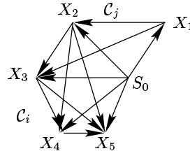
FIG. 2.6 – Suppression d'une clique contenant S_0 . Le graphe ci-dessus admet pour cliques les graphes engendrés par \{S_0, X_1, X_2\} (clique \mathcal{C}_j ) et par \{S_0, X_2, X_3, X_4, X_5\} (clique \mathcal{C}_i ). Supprimer les sommets X_4 et X_5 revient à conserver la clique \mathcal{C}_j , qui contient les parents de ses sommets.
