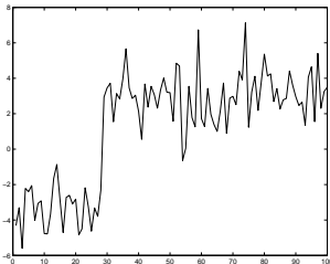
FIG. 1.6 – Réalisation d'un modèle de chaîne de Markov cachée.
