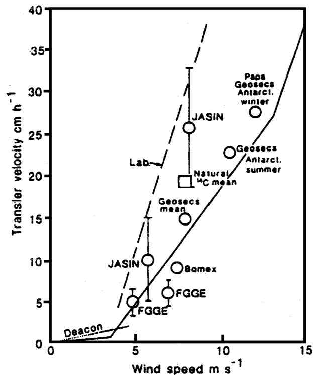
Figure VI.1: Relation du coefficient de transfert du CO 2 à l'interface air-mer pour un nombre de Schmidt de 600, en fonction de la vitesse du vent mesuré à une hauteur de 10 m au-dessus de la mer. Comparaison des courbes de prédictions des équations (VI.1a), (VI.1b) et (VI.1c) (lignes en trait plein), des résultats de mesures de radon (cercles), des mesures du 14 C naturel (carré), des résultats d'étude en soufflerie (larges pointillés) et des prédictions du modèle de Deacon (1977) (pointillés fins) (d'après Liss et Merlivat (1986)).
