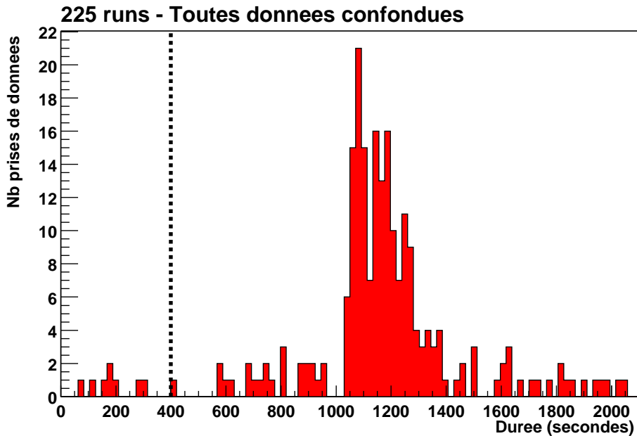
FIG. 13.1: Distribution des durées de l'ensemble des prises de données Crabe.
