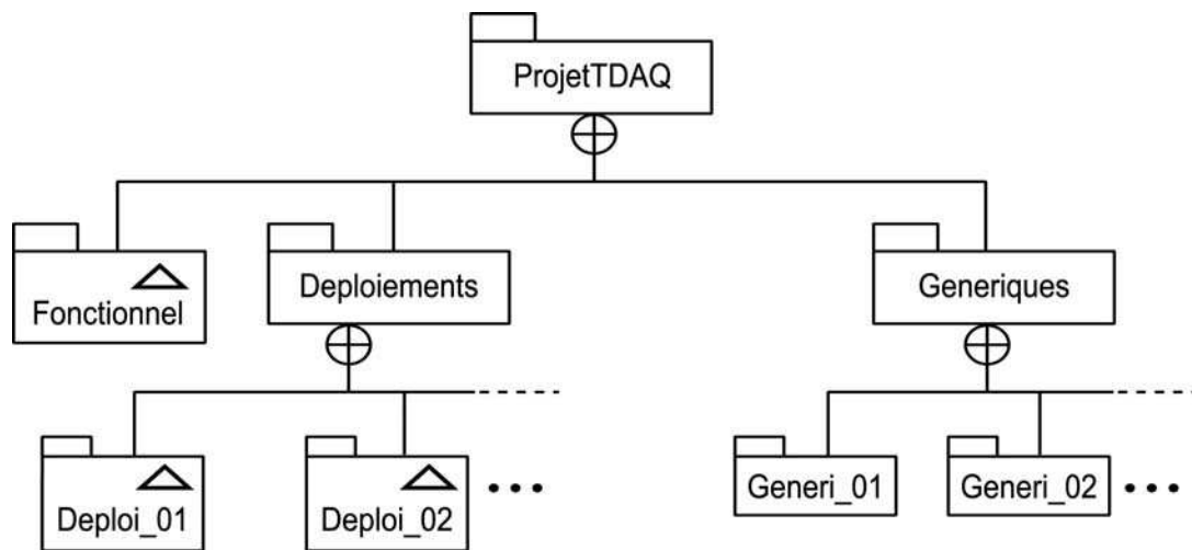
Fig. IV-27 : Arborescence des paquetages d'un projet de développement TDAQ
