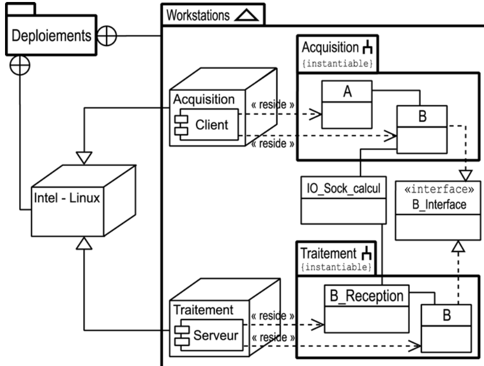
Fig. IV-36 : Organisation des paquetages effectifs de déploiement du projet AB
