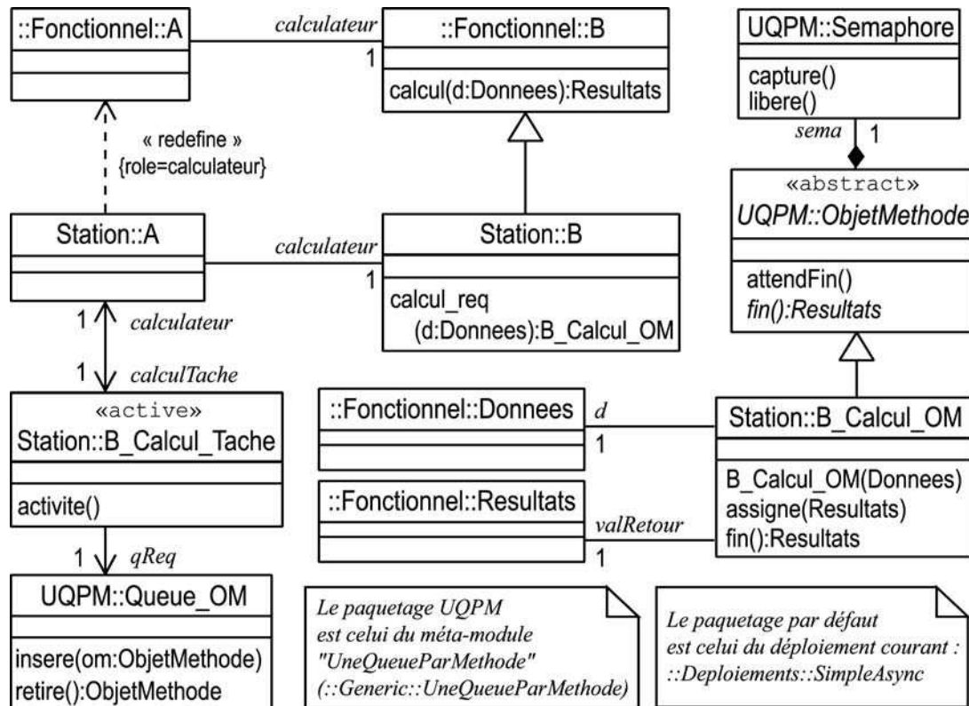
Fig. IV-40 : Diagramme de classe du projet ABbis résultant de la transformation du diagramme fonctionnel par le méta-module UneQueueParMéthode.
