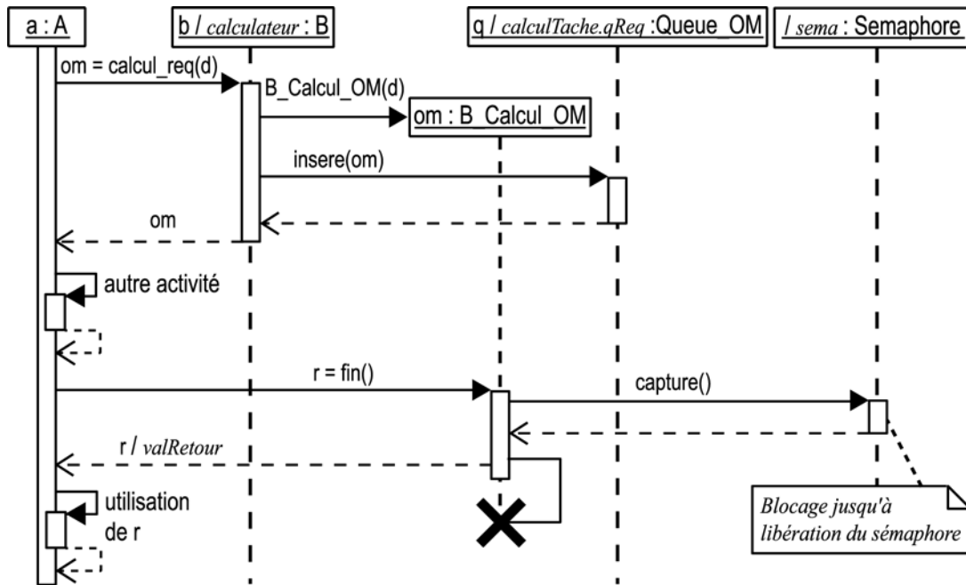
UneQueueParMethode.Transform(ABbis_Sequence) - 1 (séquence requête)
