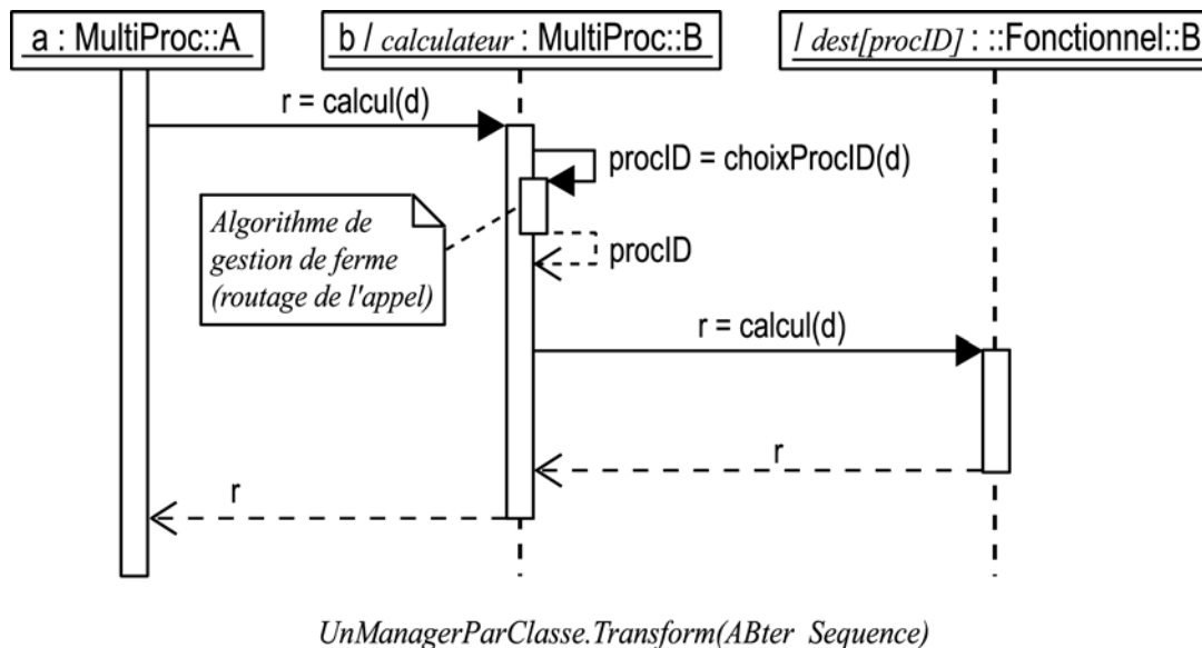
Fig. IV-46 : Séquences du projet ABter résultant de la transformation par le méta-module UnManagerParClasse . Ces séquences sont directement assimilables à du code C++ ou Java.
