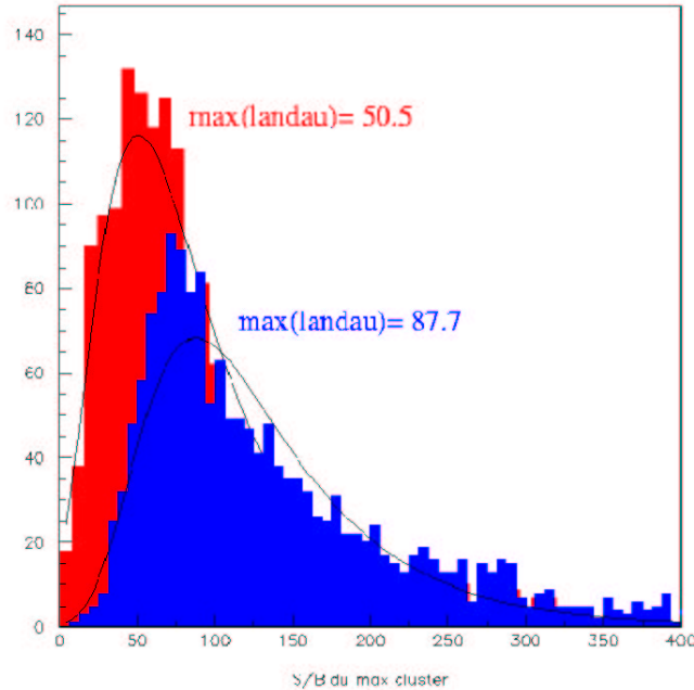
Figure 3.25 – Comparaison du rapport S/N évalué par la méthode "détecteur" (rapport S/N de 50,5) et par la méthode "substrat" (rapport S/N de 87,7).
