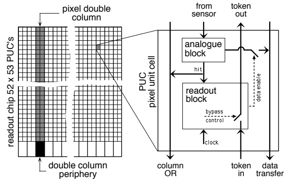
Figure 2.19 – Système de lecture des détecteurs silicium à pixels.
