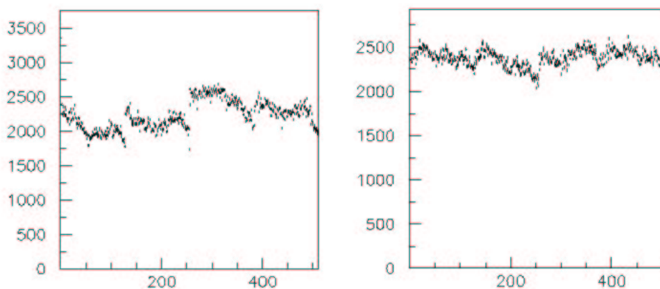
Figure 3.21 – Exemple de piédestal en nombre de coups ADC (en ordonnées) des 512 pistes (en abscisse) de deux modules MSGC.
