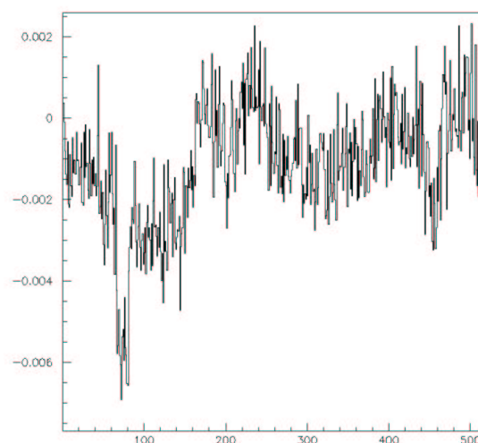
Figure 3.23 – Différence en nombre de coups ADC (en ordonnées) sur le piédestal des 512 pistes (en abscisse) d'une MSGC entre la première prise de donnée basse intensité de la troisième phase et la dernière 22 jours plus tard.
