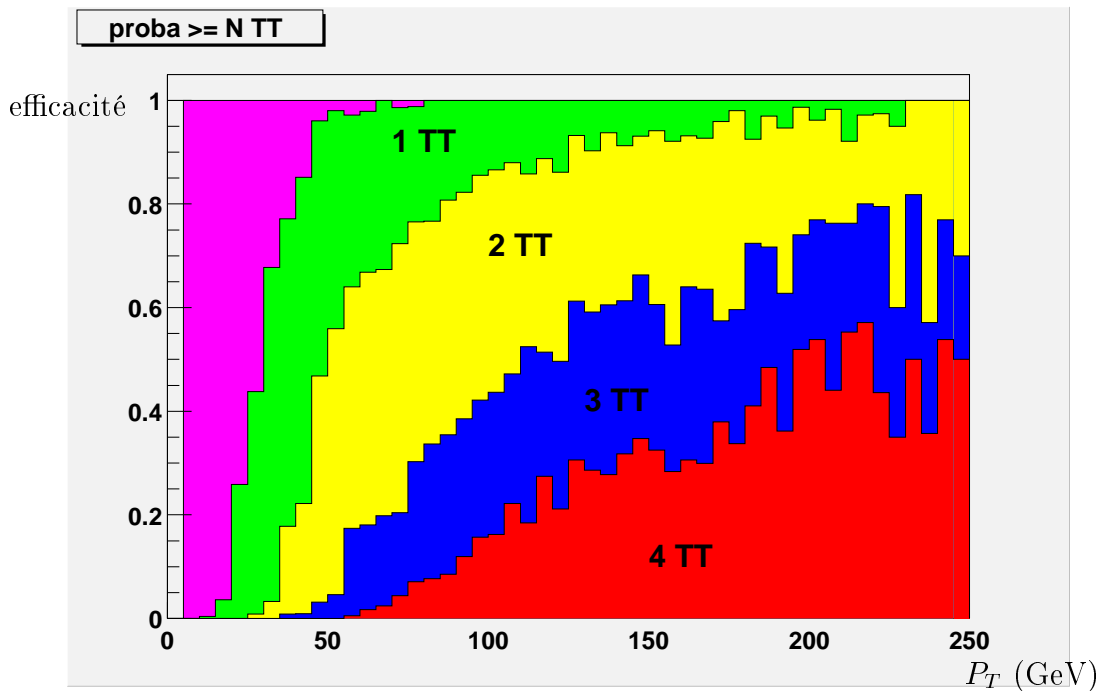
FIG. 7.8 – Probabilité qu’un jet allume respectivement une, deux, trois et au moins quatre tour(s) de déclenchement (TT) de 7 GeV ( \eta \times \phi = 0.2 \times 0.2 ) en fonction de l’impulsion transverse du jet pour des événements QCD.
