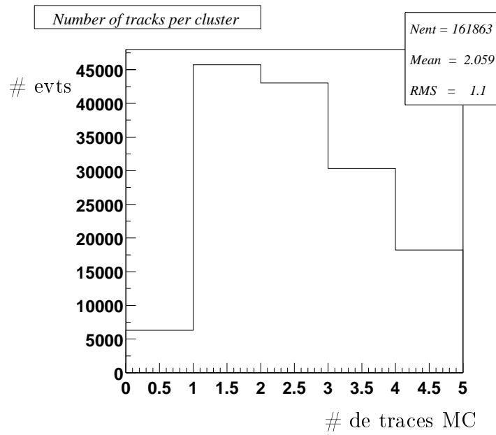
FIG. 4.12 – Nombre de particules Monte Carlo contribuant au moins à 5% de l'énergie du cluster.
