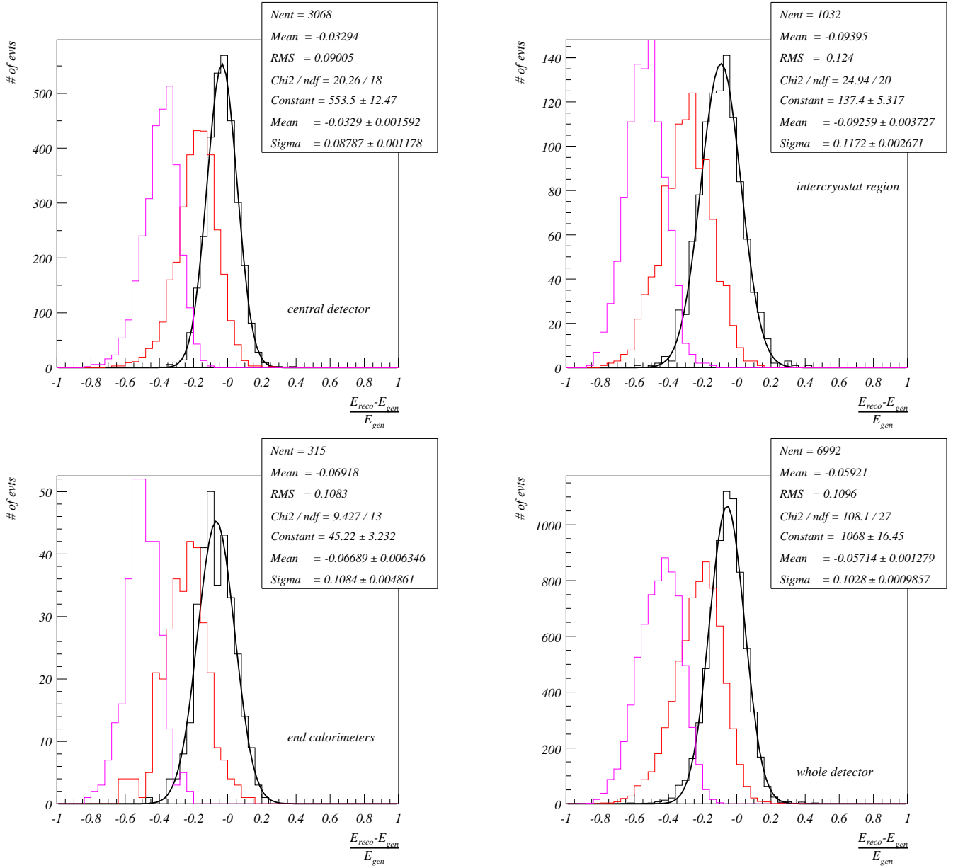
FIG. 5.3 – Distributions de \Delta E_{rel} , dans le détecteur central (en haut à gauche), dans la région intermédiaire (en haut à droite), à l'avant du détecteur (en bas à gauche) et pour l'ensemble du détecteur (en bas à droite). Les trois distributions superposées sont, de gauche à droite, \Delta E_{rel} pour les clusters cellNN, pour les clusters cellNN calibrés et pour les particules energy flow
