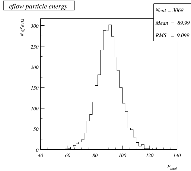
FIG. 5.14 – Distributions de l'énergie totale de toutes les particules energy flow. L'energy flow utilise ici les traces reconstruites à partir des impacts Monte Carlo.
