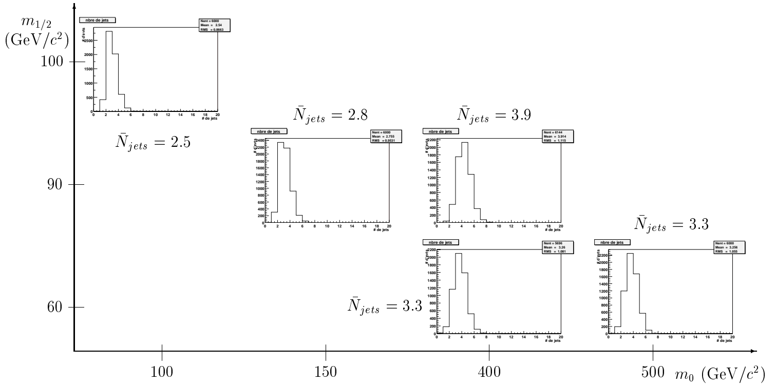
FIG. 1.9 – Nombre de jets de plus de 25 GeV pour cinq points du plan (m_0, m_{1/2}) ((100, 100), (150, 90), (400, 90), (400, 60), (500, 60), \mu < 0, \tan \beta = 2 et A_0 = 0 ).
