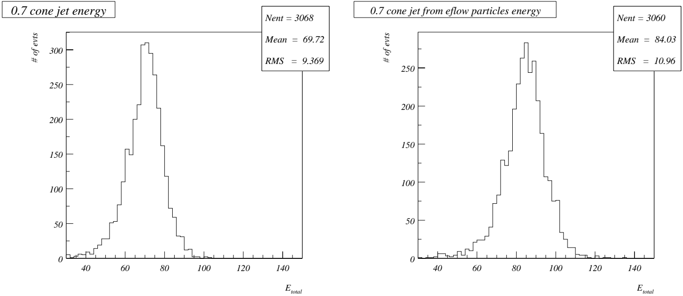
FIG. 5.9 – Distributions d'énergie totale reconstruite par les jets de cône (à gauche) et par les jets de cône basés sur les particules energy flow (à droite)
