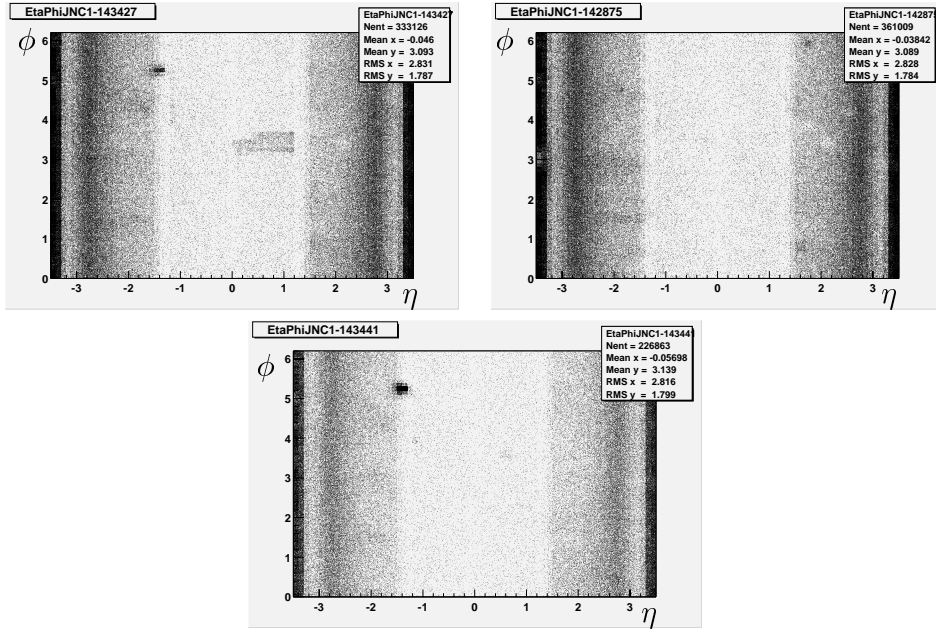
FIG. 7.16 – Positions des clusters cellNN dans le plan (\eta, \phi) pour les runs 143427, 142875 et 143441 (de haut en bas et de gauche à droite).
