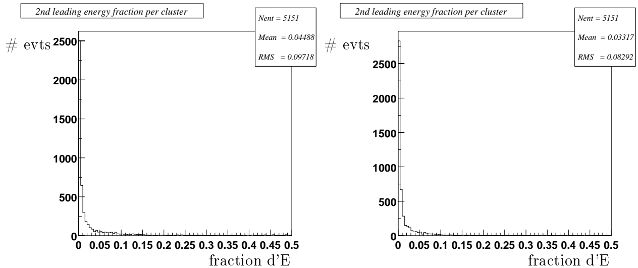
FIG. 4.11 – Fraction d'énergie que le cluster emporte de la trace Monte Carlo qui a la deuxième plus importante contribution à ce cluster. A gauche, les impacts ambigus sont oubliés et à droite tous les impacts sont pris en compte.
