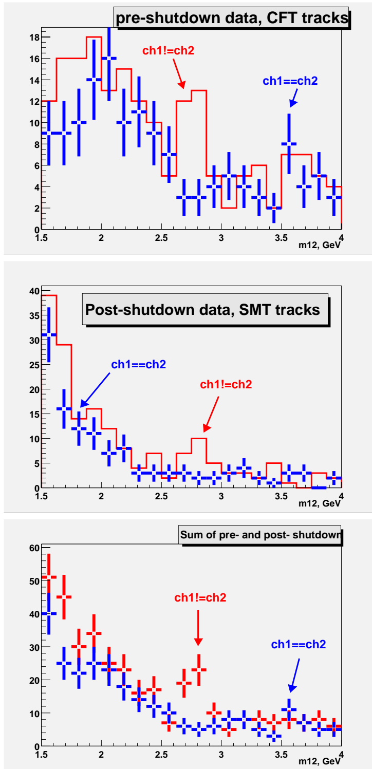
FIG. 4.30 – De haut en bas : résonance du J/\psi sur les données enregistrées avant l'arrêt prolongé du TeVatron fin octobre et début décembre 2001, après cet arrêt et la combinaison des lots de données. Avant l'arrêt, on demande une trace CFT pour identifier les électrons, ce qui limite fortement l'acceptance. Après l'arrêt, on demande une trace SMT pour identifier les électrons.
