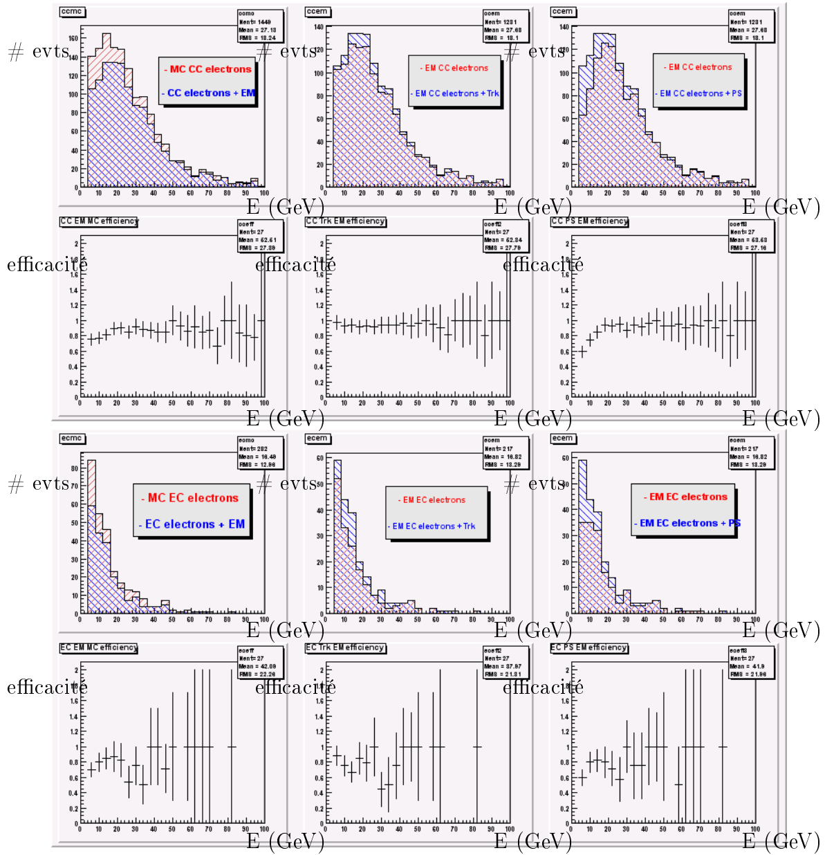
FIG. 4.28 – Les 6 premières distributions correspondent à des événements centraux et les 6 dernières à des événements à l'avant. Les distributions de gauche représentent la superposition des énergies des électrons générés et reconstruits avec l'algorithme de cône dont on déduit, directement en dessous, l'efficacité de reconstruction en fonction de l'énergie. Les distributions du milieu représentent la superposition des énergies des électrons reconstruits avec l'algorithme de cône et associés à une trace. L'efficacité d'association entre le candidat et la trace en fonction de l'énergie est représentée en dessous. Les distributions de droite représentent la superposition des énergies des électrons reconstruits avec l'algorithme de cône et associés à un dépôt d'énergie dans le détecteur de pieds de gerbe. L'efficacité d'association d'un candidat électron avec un dépôt d'énergie dans le détecteur de pied de gerbe en fonction de l'énergie se trouve directement en dessous.
