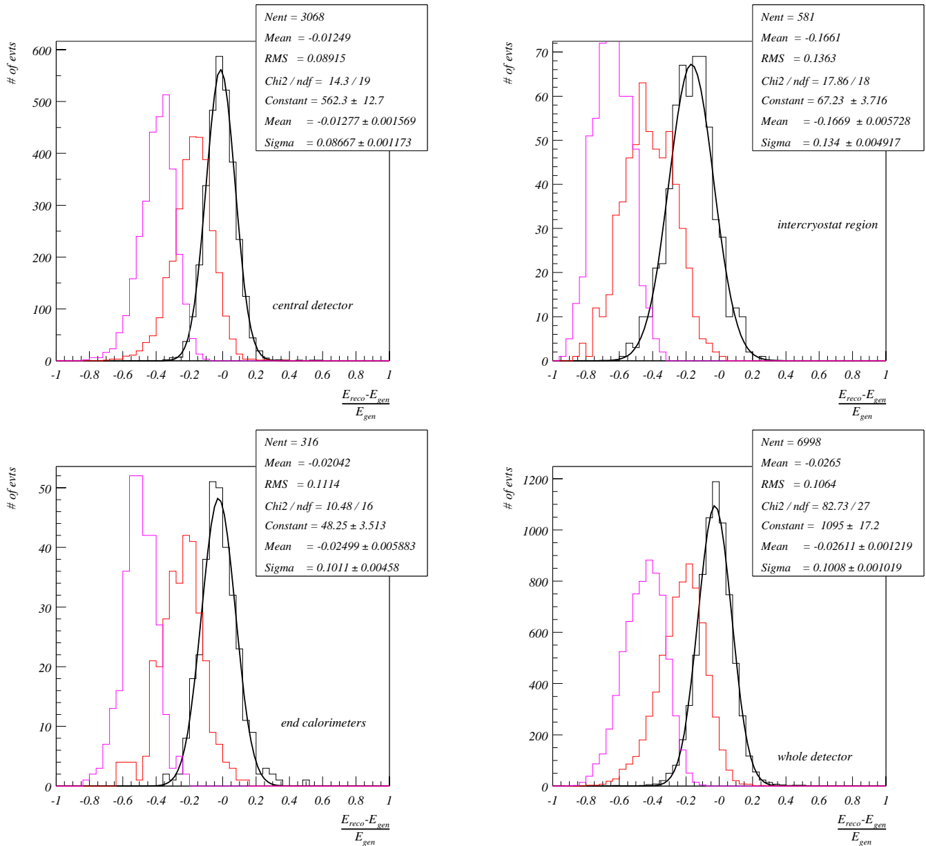
FIG. 5.13 – Distributions de \Delta E_{rel} , dans le détecteur central (en haut à gauche), dans la région intermédiaire (en haut à droite), à l’avant du détecteur (en bas à gauche) et pour l’ensemble du détecteur (en bas à droite). Les trois distributions superposées sont, de gauche à droite, \Delta E_{rel} pour les clusters cellNN, pour les clusters cellNN calibrés et pour les particules energy flow. L’energy flow utilise ici les traces reconstruites à partir des impacts Monte Carlo.
