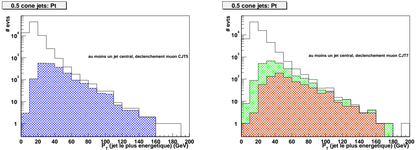
FIG. 7.2 – Le nombre d'événements passant les déclenchements muon plus une tour calorimétrique (de plus de 5 GeV à gauche et de plus de 7 GeV à droite) et pour lesquels un jet a été reconstruit dans le centre du détecteur ( |\eta| < 0.8 ) en fonction du P_T du jet (histogramme vierge). Les autres histogrammes représentent ceux qui parmi ces événements ont, en plus, passé respectivement le déclenchement 3CJT7 (hachures vertes), 4CJT5 (hachures bleues) et 4CJT7 (hachures rouges).
