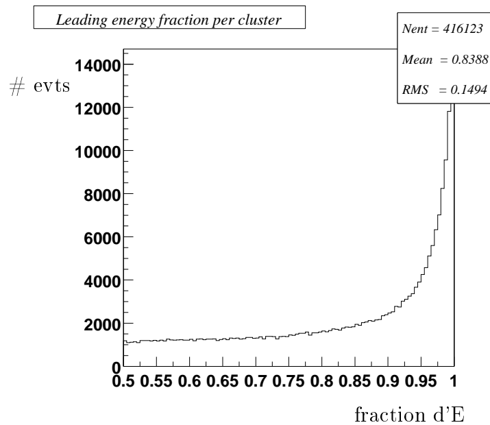
FIG. 4.13 – Fraction d'énergie que le cluster emporte de la trace Monte Carlo qui a le plus contribué à ce cluster.
