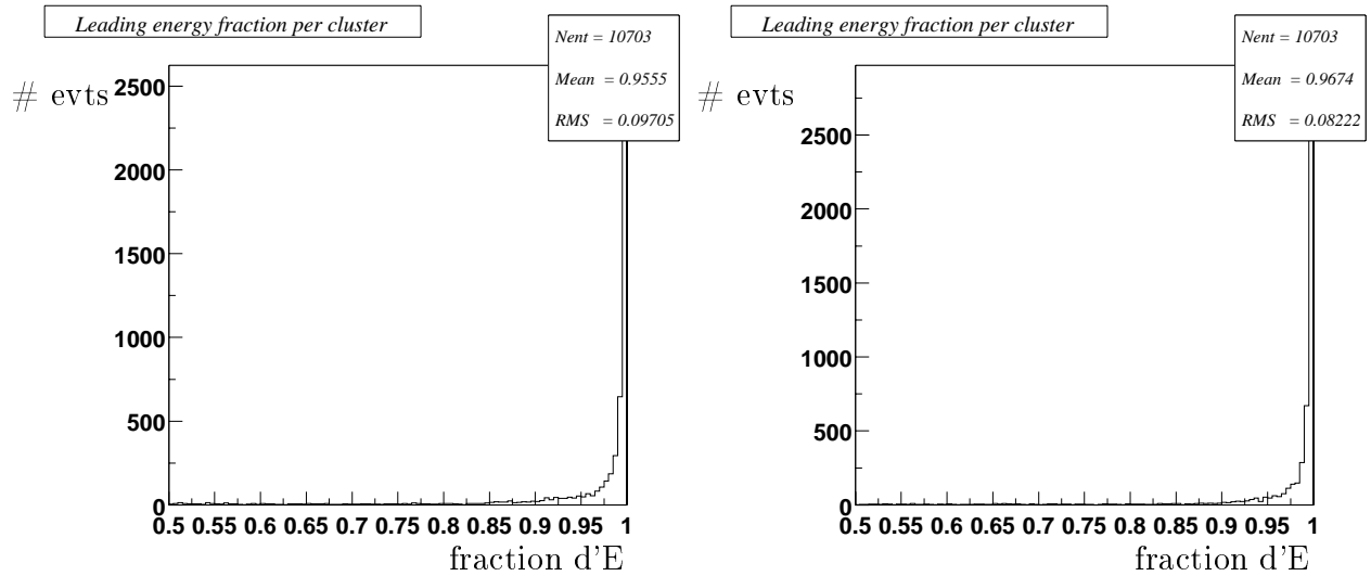
FIG. 4.10 – Fraction d'énergie que le cluster emporte de la trace Monte Carlo qui a le plus contribué à ce cluster. A gauche, les impacts ambigus sont oubliés et à droite tous les impacts sont pris en compte.
