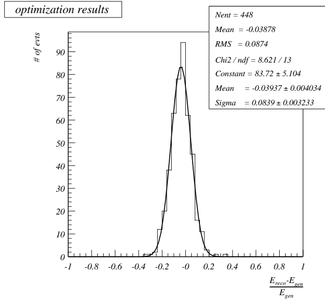
FIG. 5.2 – Distribution de \Delta E_{rel} . obtenue avec l’algorithme energy flow lors de la procédure d’optimisation
