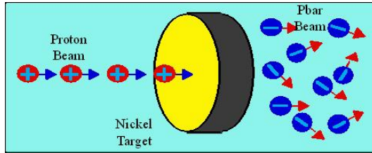
FIG. 2.4 – Schéma de la source d’antiprotons
