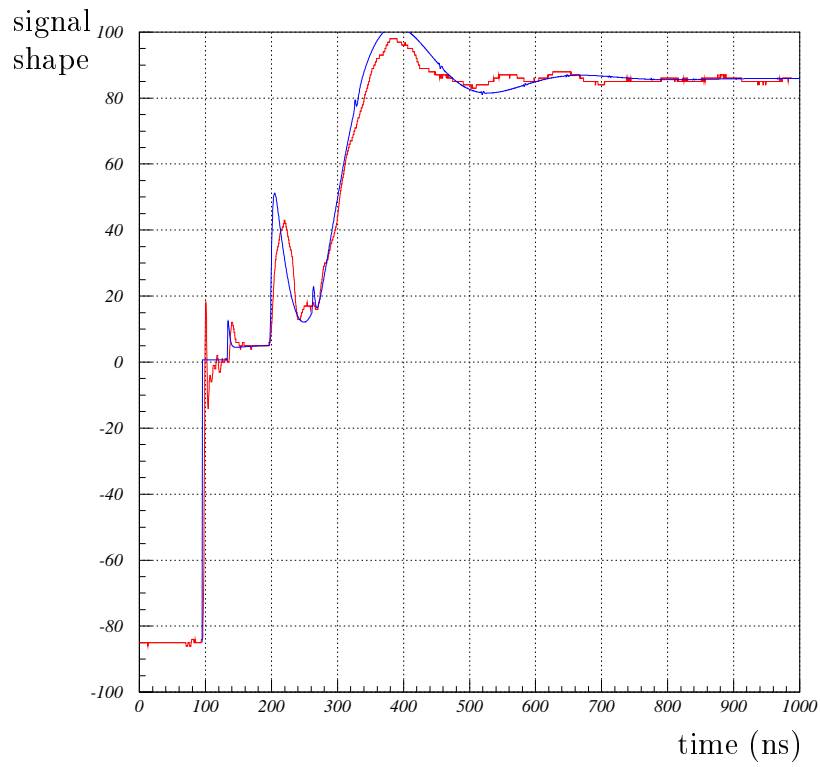
FIG. 3.12 – Superposition d’une mesure de réflectométrie et de sa simulation à partir des paramètres qui en ont été extraits
