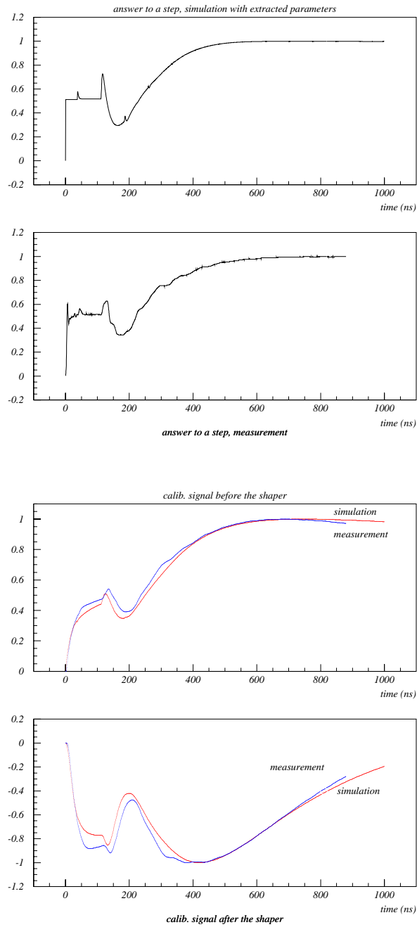
FIG. 3.20 – De haut en bas : simulation de la mesure de réflectométrie d'une voie connectée à un préamplificateur de type D basée sur les paramètres extraits, mesure de réflectométrie, superposition de la simulation du signal de calibration jusqu'à la sortie du préamplificateur à partir de deux signaux précédents, superposition de la simulation du signal de calibration jusqu'à la sortie du shaper à partir de deux signaux précédents
