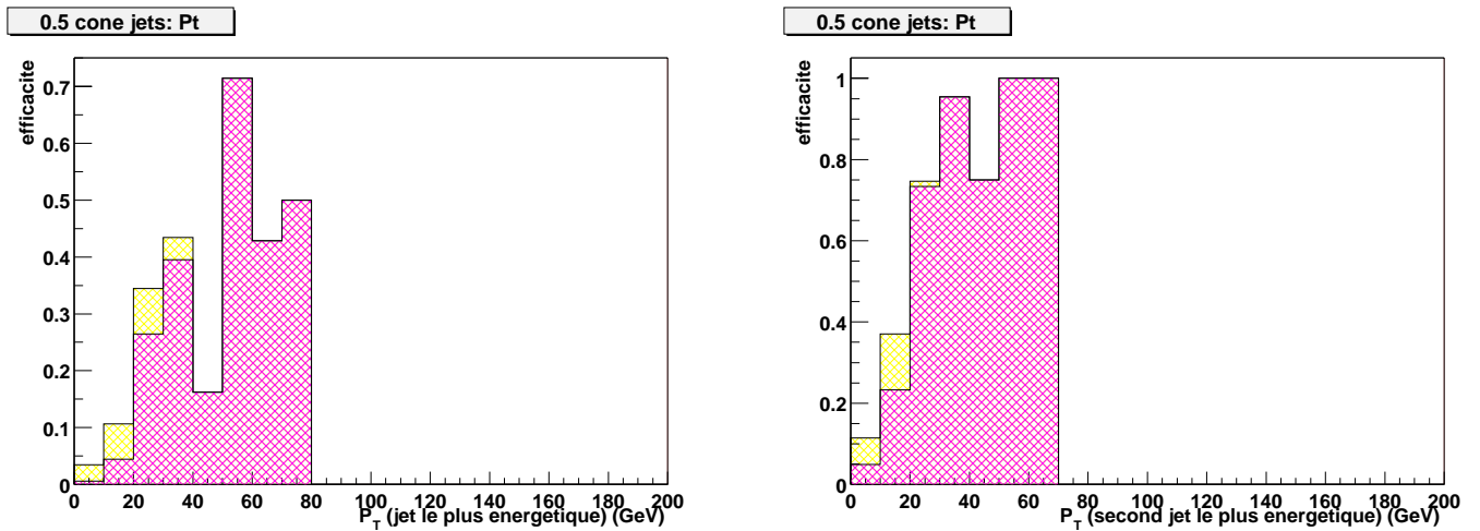
FIG. 7.4 – A gauche, efficacité de déclenchement d'une tour de plus de 5 GeV (hachures jaunes) et d'une tour de plus de 7 GeV (hachures violettes) en fonction du P_T du jet. On demande que le jet appartienne à l'acceptance |\eta| < 0.8 et qu'il n'y ait pas d'autres bons jets dans l'acceptance |\eta| < 1.1 . A droite, on demande deux bons jets dans l'acceptance |\eta| < 0.8 et pas d'autres bons jets dans l'acceptance |\eta| < 1.1 . Les efficacités de droite sont représentées en fonction du P_T du second jet.
