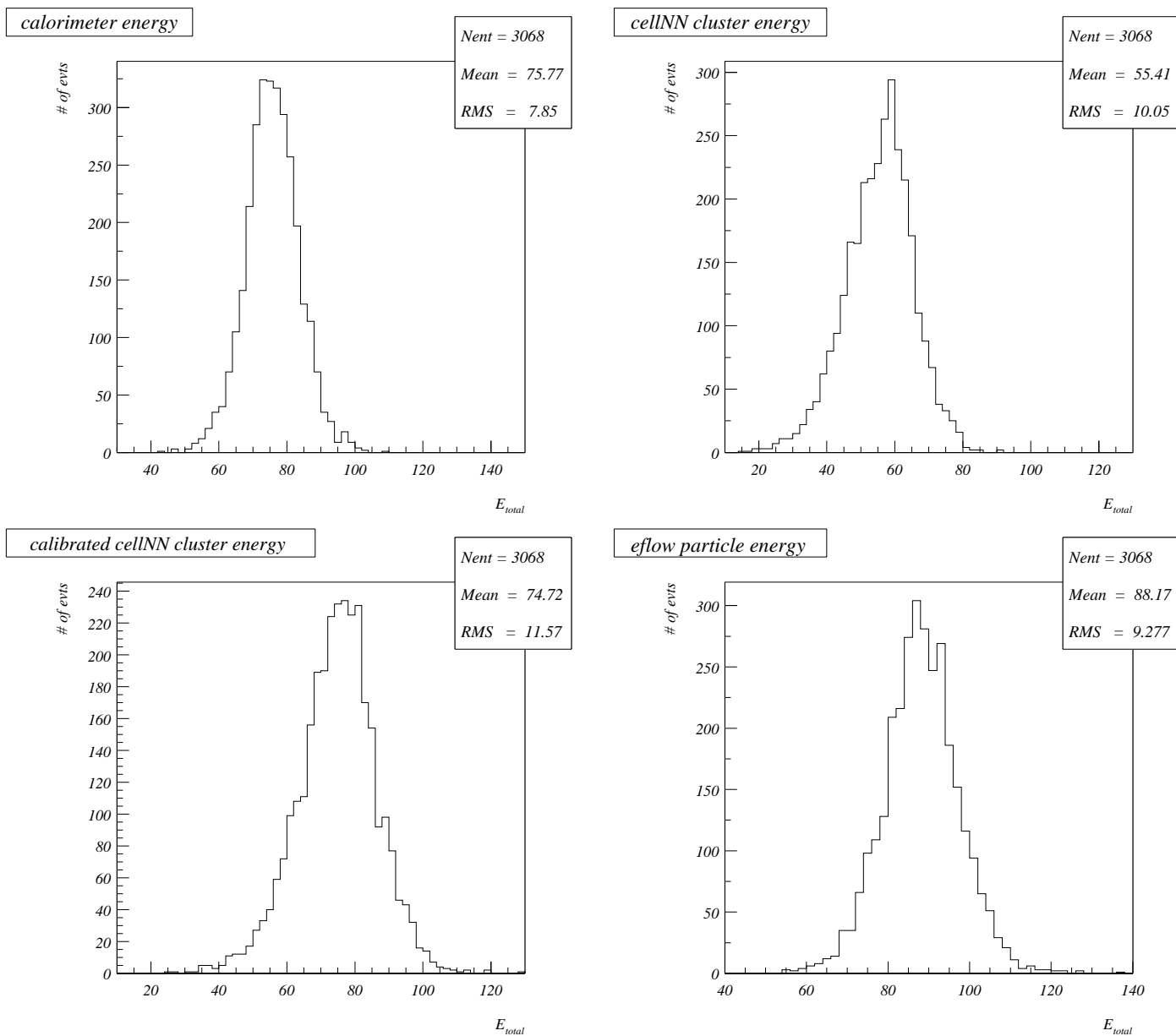
FIG. 5.7 – Distributions d'énergie totale déposée dans le calorimètre (en haut à gauche), reconstruite par les clusters cellNN (en haut à droite), reconstruite par les clusters cellNN calibrés (en bas à gauche) et reconstruite par les particules energy flow (en bas à droite)
