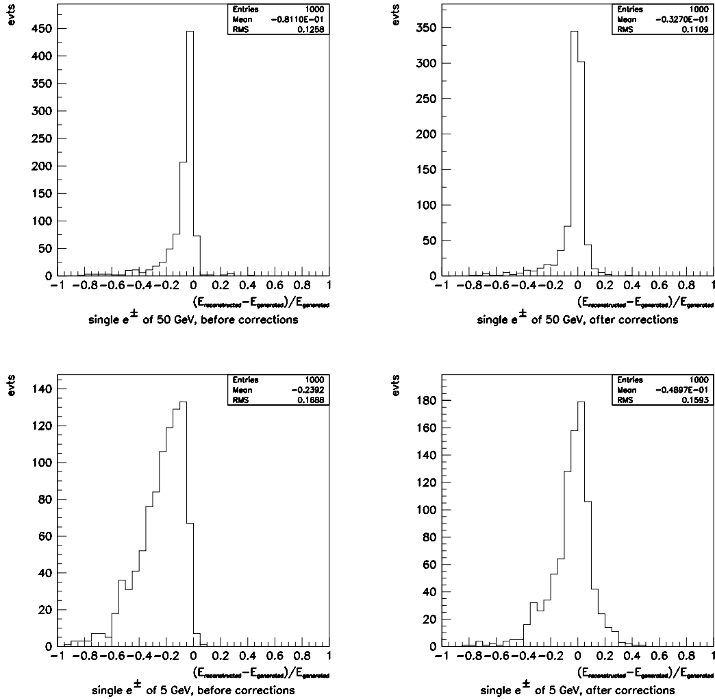
FIG. 4.22 – De haut en bas, distributions de \Delta E_{rel} . pour des électrons de hautes et basses énergies. Les distributions de gauche représentent \Delta E_{rel} . des clusters cellNN avant corrections et celles de droite, \Delta E_{rel} . des clusters cellNN après corrections (les critères d'identification sont appliqués avant les corrections).
