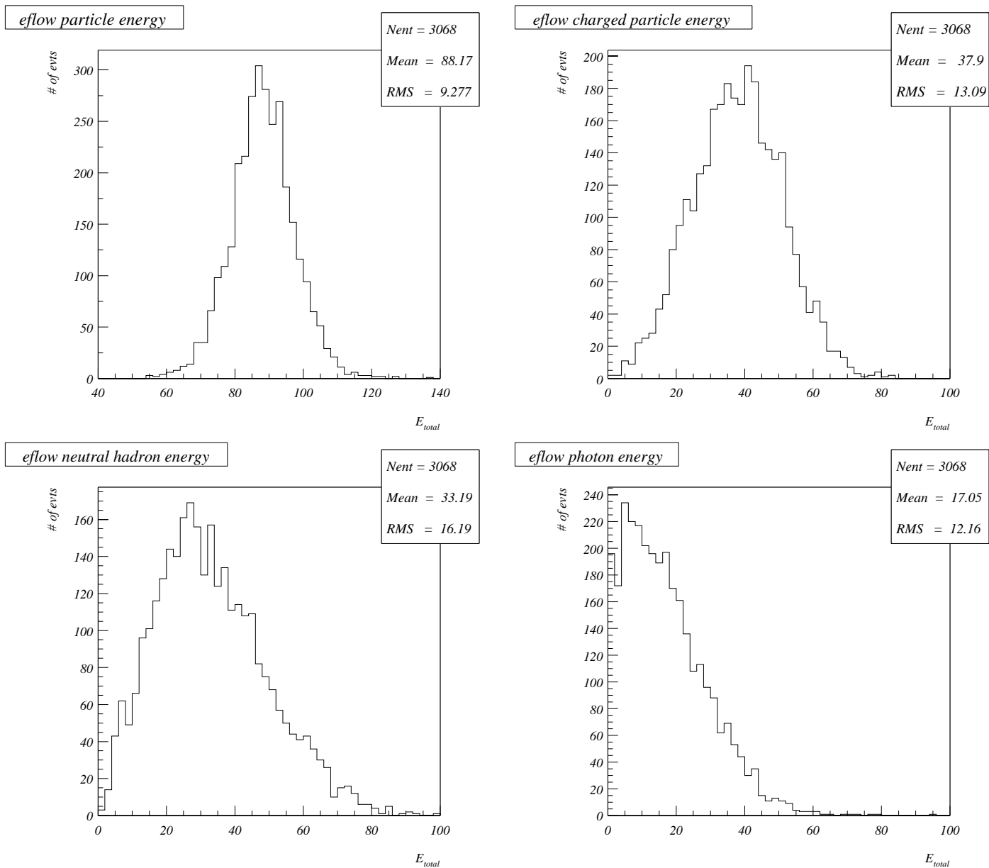
FIG. 5.5 – Distributions de l'énergie totale de toutes les particules energy flow (en haut à gauche), des particules chargées (en haut à droite), des hadrons neutres (en bas à gauche) et des photons (en bas à droite)
