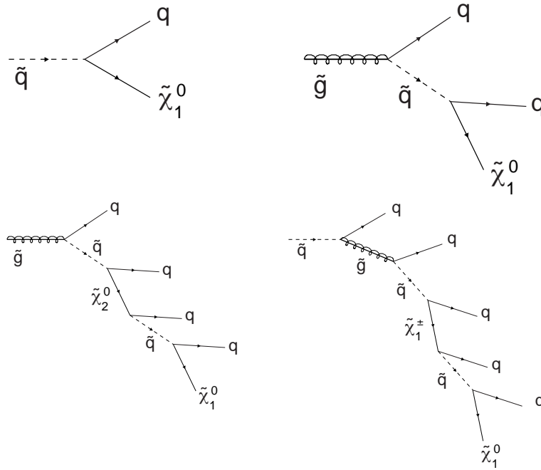
FIG. 1.8 – Exemples de désintégration directe (en haut) de squarks et gluinos. Le squark se désintègre ici directement en jet et LSP et le gluino se désintègre via un squark en deux jets et LSP. Exemples de désintégration en cascade (en bas) de squarks et gluinos.
