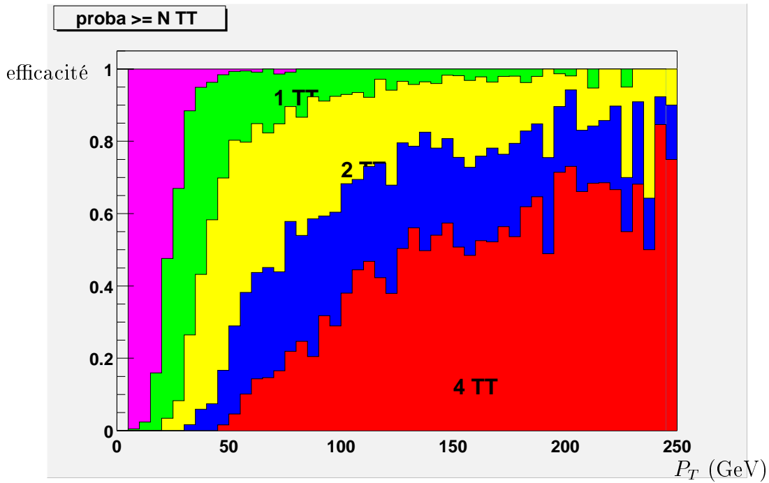
FIG. 7.7 – Probabilité qu’un jet allume respectivement une, deux, trois et au moins quatre tour(s) de déclenchement (TT) de 5 GeV ( \eta \times \phi = 0.2 \times 0.2 ) en fonction de l’impulsion transverse du jet pour des événements QCD.
