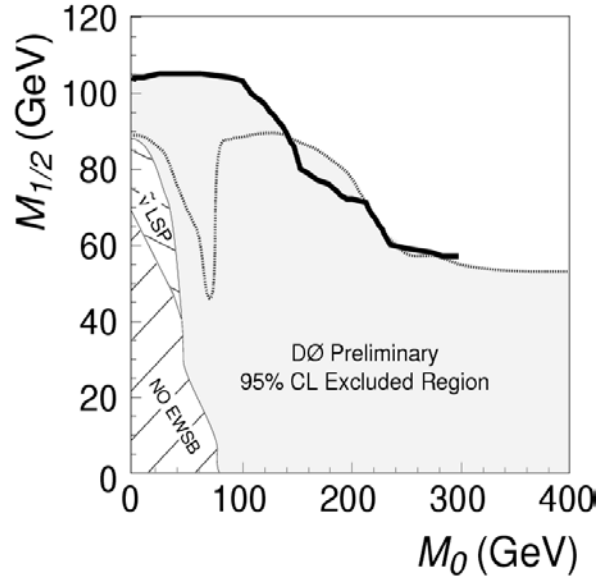
FIG. 1.15 – Contours d'exclusion les plus récents sur la masse des squarks et des gluinos dans le plan (m_0, m_{1/2}) à 95% de degré de confiance et en utilisant la signature jets, énergie transverse manquante et di-leptons en pointillé et la signature jets et énergie transverse manquante en trait plein ( \mu < 0 , A_0 = 0 et \tan \beta = 2 ).
