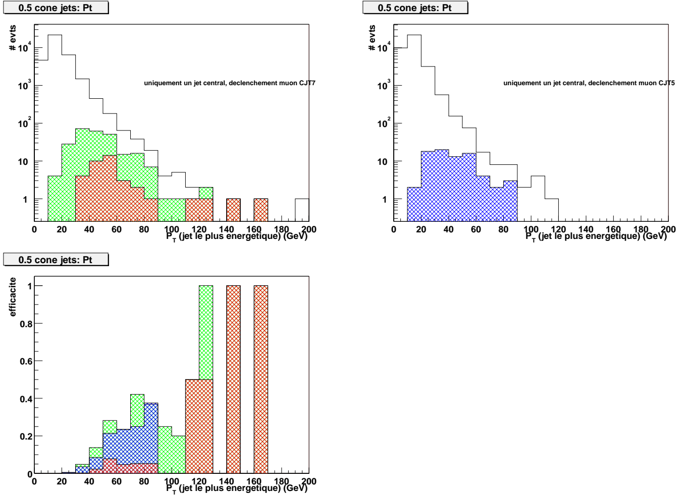
FIG. 7.5 – En haut, les événements du lot de contrôle à un seul jet ainsi que la proportion des événements qui satisfont en plus les déclenchements 3CJT7 et 4CJT7 à gauche et 4CJT5 à droite en fonction du P_T du jet ; la figure du bas donne les efficacités correspondantes.
