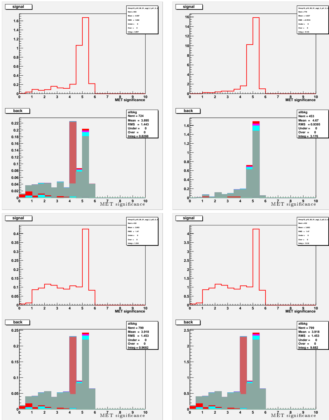
FIG. 7.13 – Les histogrammes du haut sont faits à partir d'événements de signal et ceux du bas à partir d'événements de bruit de fond normalisés à 10 pb -1 (à gauche) ou 100 pb -1 (à droite). En haut, le signal est le point ( m_0 = 100, m_{1/2} = 100 ) et en bas le point ( m_0 = 500, m_{1/2} = 70 ). Pour chacune des optimisations, la valeur de la signification en énergie transverse manquante est représentée.
