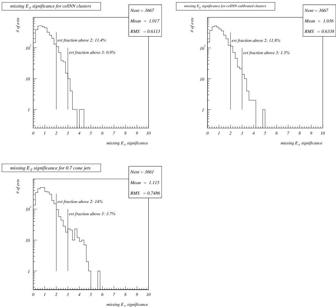
FIG. 4.27 – De gauche à droite et de haut en bas : distributions de signification d'énergie transverse manquante pour les clusters cellNN, les clusters cellNN calibrés et les jets de cône de 0.7 dans l'acceptance |\eta_{det}| < 3.5 . La fraction des événements au-dessus de 2 et 3 en signification d'énergie transverse manquante est donnée dans chacun des cas.
