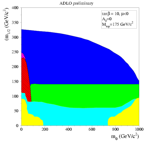
FIG. 1.17 – Domaines du plan (m_0, m_{1/2}) exclus à LEP ( \mu < 0 , A_0 = 0 et \tan\beta = 10 ). La zone jaune est exclue théoriquement, la zone bleu clair est en désaccord avec les mesures des paramètres électrofaibles à LEP1, la zone verte est exclue par les recherches de charginos, la zone rouge est exclue par les recherches de sleptons ou de staus, la zone bleu foncé est exclue par la recherche de hZ et la zone magenta est exclue par la recherche de particules chargées lourdes stables appliquée aux staus.
