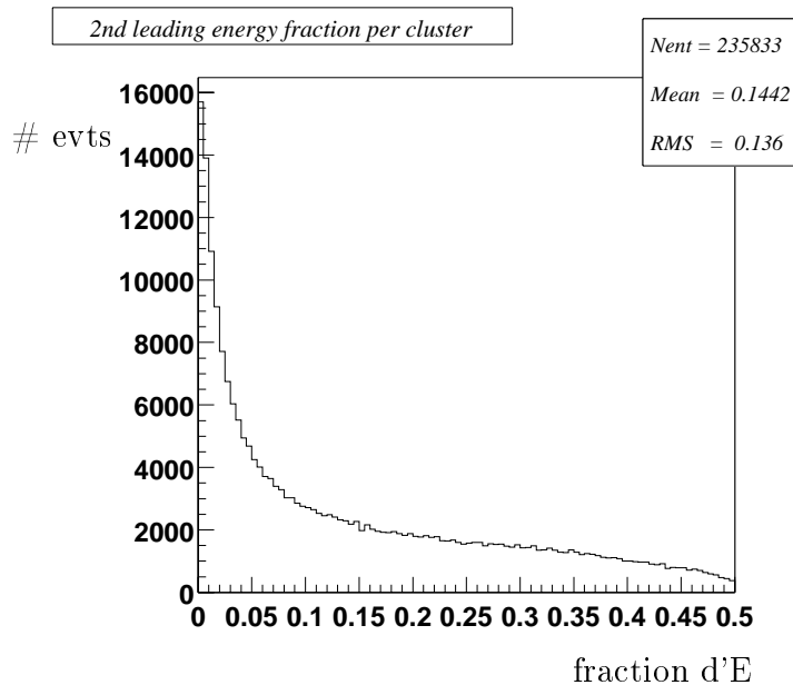
FIG. 4.14 – Fraction d'énergie que le cluster emporte de la trace Monte Carlo qui a la deuxième plus importante contribution à ce cluster.
