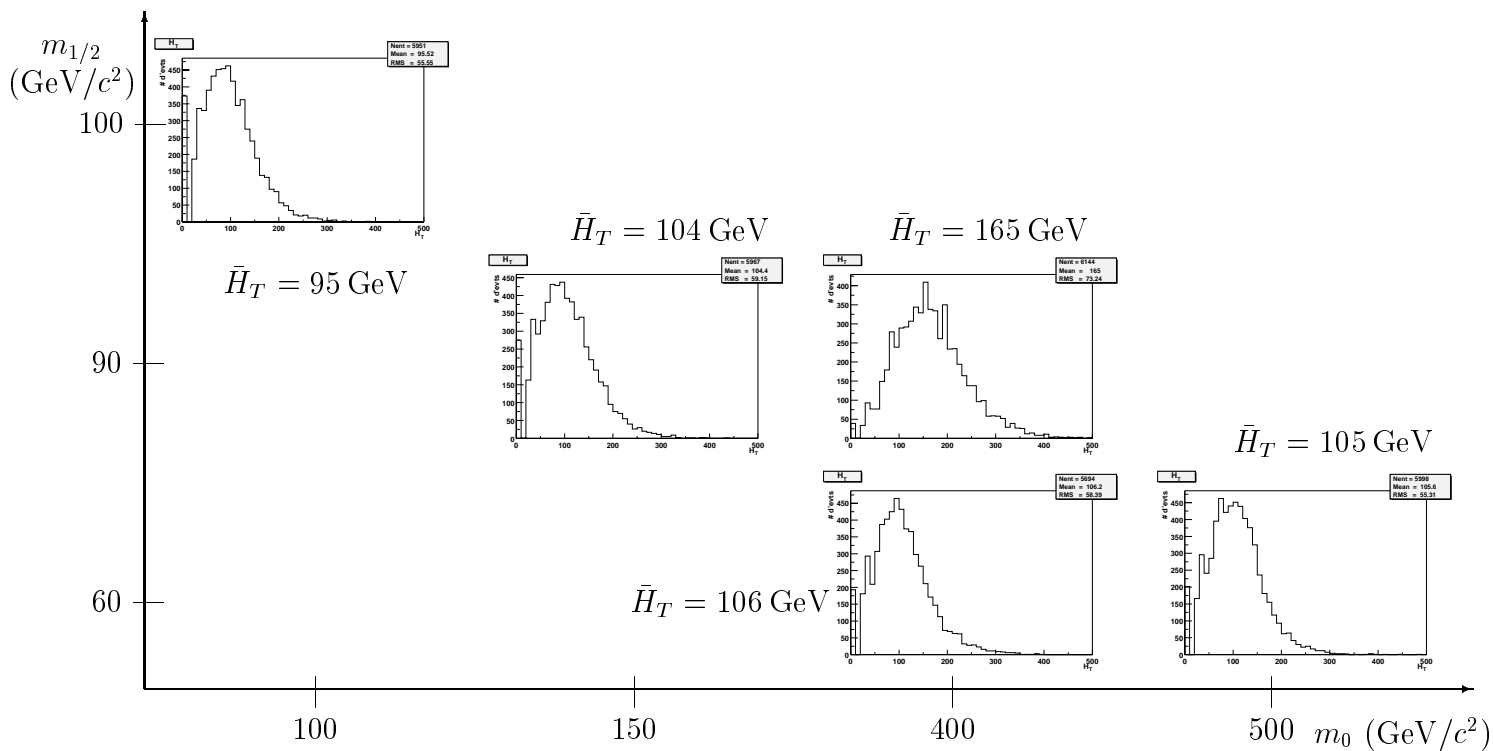
FIG. 1.12 – H_T pour cinq points du plan (m_0, m_{1/2}) , ((100, 100), (150, 90), (400, 90), (400, 60), (500, 60)) , \mu < 0 , \tan \beta = 2 et A_0 = 0 . H_T est la somme des énergies transverses des jets de plus de 25 GeV de l'événement à l'exclusion du jet le plus énergétique. H_T est une variable discriminante pour différencier le signal du bruit de fond et sera utilisée dans le chapitre 7 mais varie relativement peu dans l'espace des paramètres.
