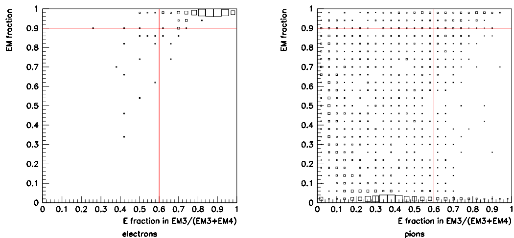
FIG. 4.21 – Résultats des critères d’identifications des clusters comme électromagnétiques ou hadroniques pour des électrons à gauche et pour des pions à droite.
