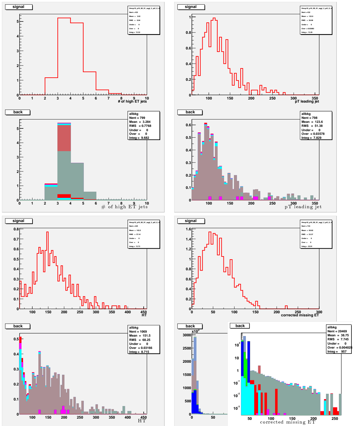
FIG. 7.12 – Les histogrammes du haut sont faits à partir d'événements de signal ( m_0 = 500, m_{1/2} = 70 ) et ceux du bas à partir d'événements de bruit de fond normalisés à 100 \text{ pb}^{-1} . De gauche à droite et de haut en bas sont représentés le nombre de bons jets de plus de 25 GeV, l'énergie transverse du jet le plus énergétique, H_T et E_T . Toutes les coupures ont été appliquées sauf celle sur la variable représentée. Un agrandissement en échelle logarithmique de la distribution de E_T a été ajouté.
