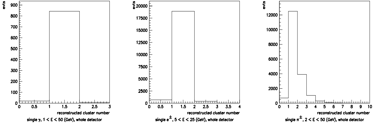
FIG. 4.6 – Distributions du nombre de clusters reconstruits à partir d'événements faits de particules uniques (des photons à gauche, des électrons au milieu et des pions à droite)
