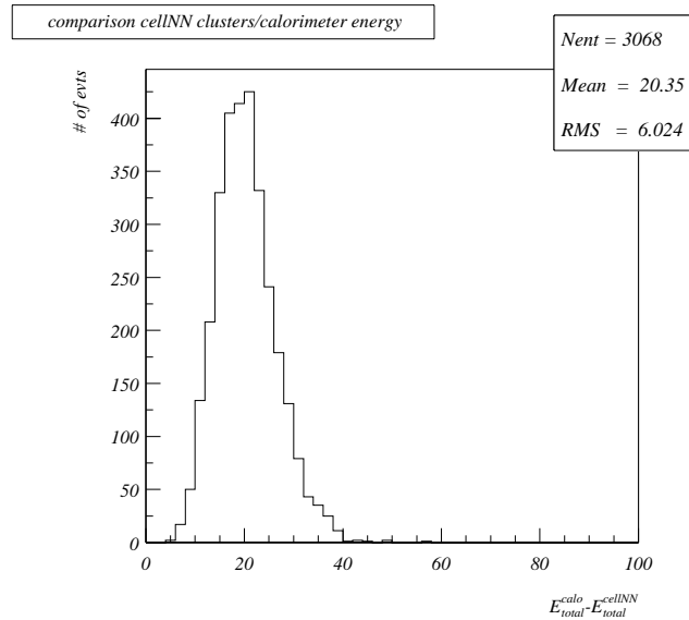
FIG. 5.8 – Différence d'énergie déposée dans le calorimètre et reconstruite par les clusters cellNN
