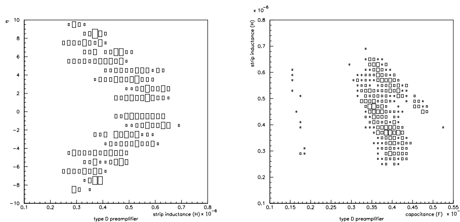
FIG. 3.31 – De gauche à droite : corrélation entre la valeur extraite de l'inductance de la piste et \eta et entre la valeur extraite de l'inductance de la piste et de la capacité détecteur pour des voies connectées à un préamplificateur de type D
