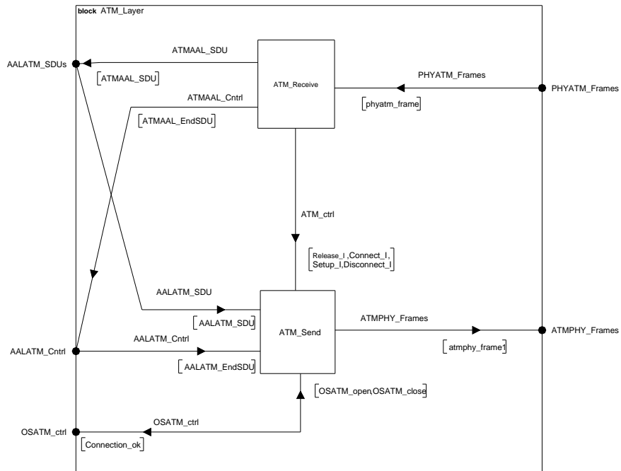
FIG. A.19: Structure de la couche ATM
