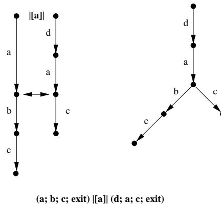
FIG. 3.7: Synchronisation de processus LOTOS
