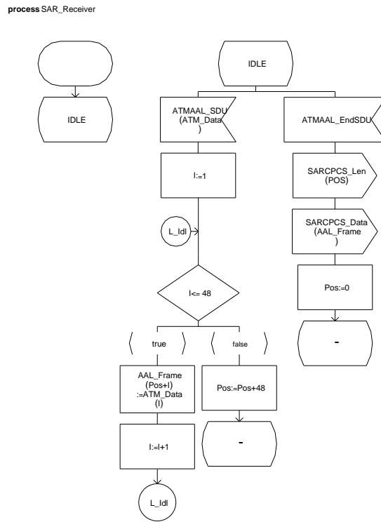
FIG. A.18: Automate de réception la couche SAR
