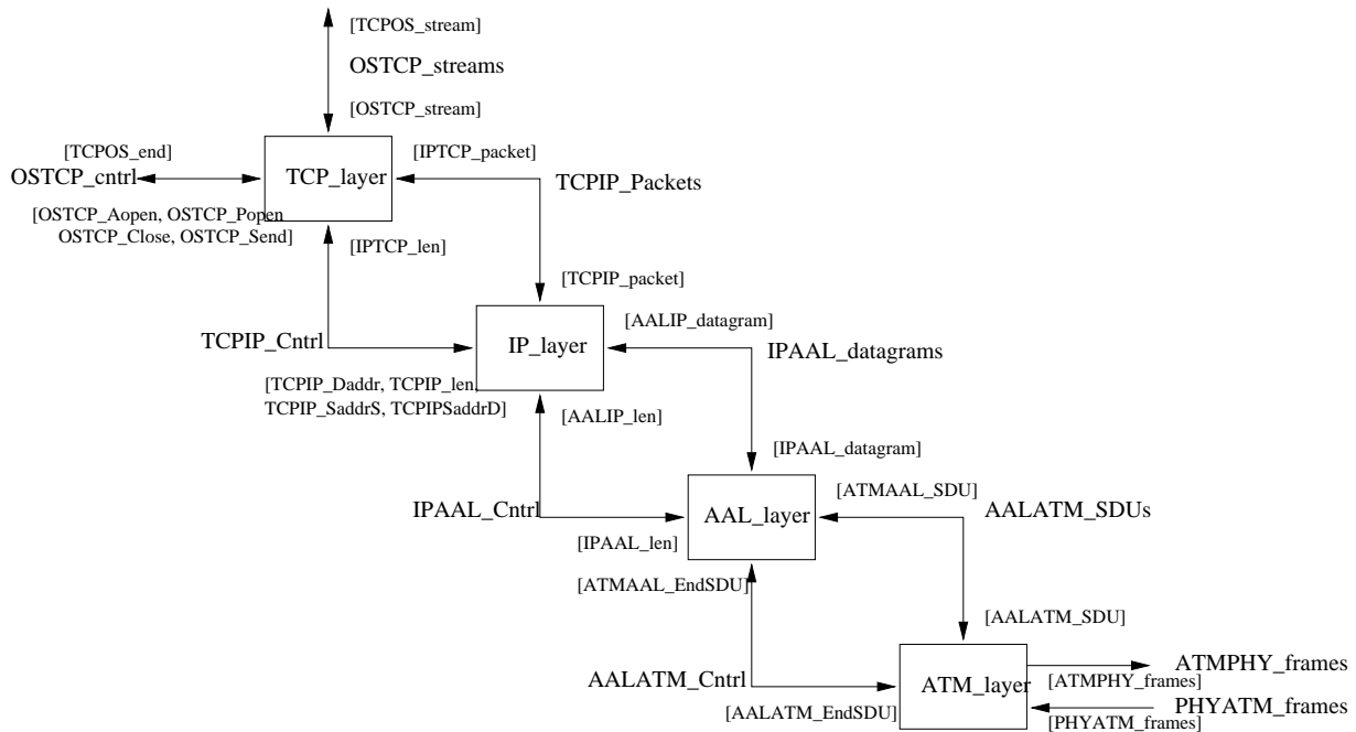
FIG. 6.15: Structure de la description SDL de l'ATM
