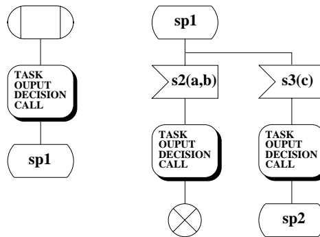
FIG. 3.14: Procédure en SDL
