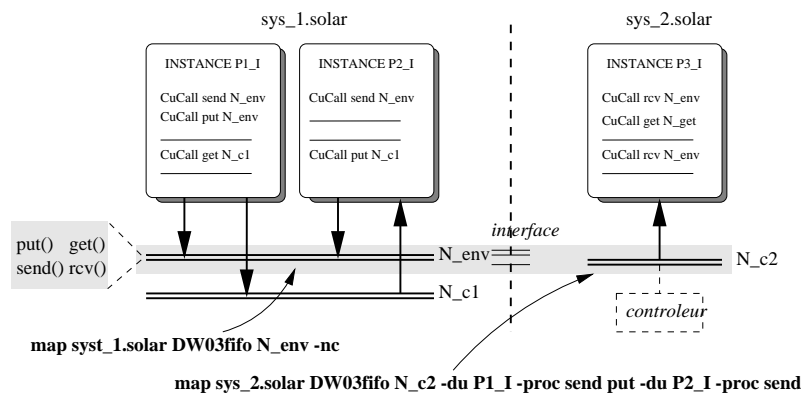
FIG. C.1: Map avec contrôleur externe
