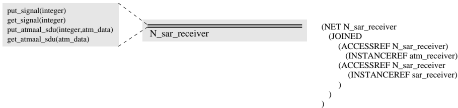
FIG. 4.3: Concept de canal abstrait et sa représentation SOLAR
