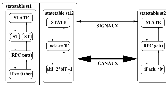
FIG. 2.2: Machines d'états finis hiérarchiques communicantes
