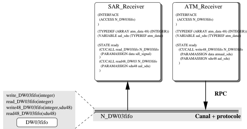
FIG. 4.21: Système communicant à travers des protocoles
