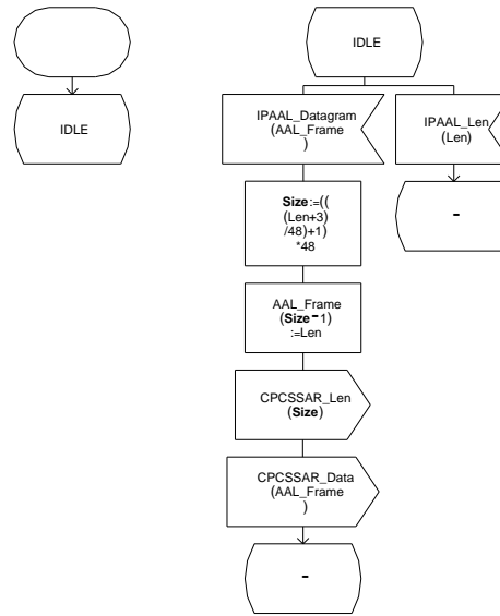
FIG. A.14: Automate d'émission la couche CPCS
