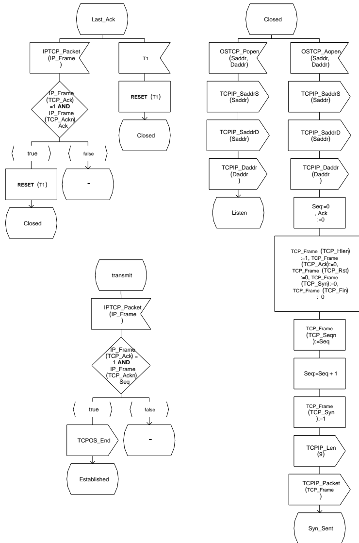
FIG. A.8: Automate de la couche TCP
