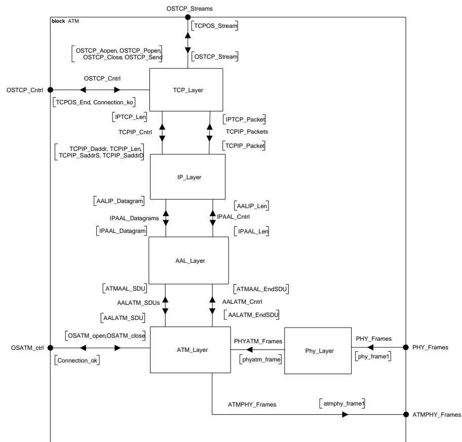
FIG. A.1: Modèle général de l'ATM
