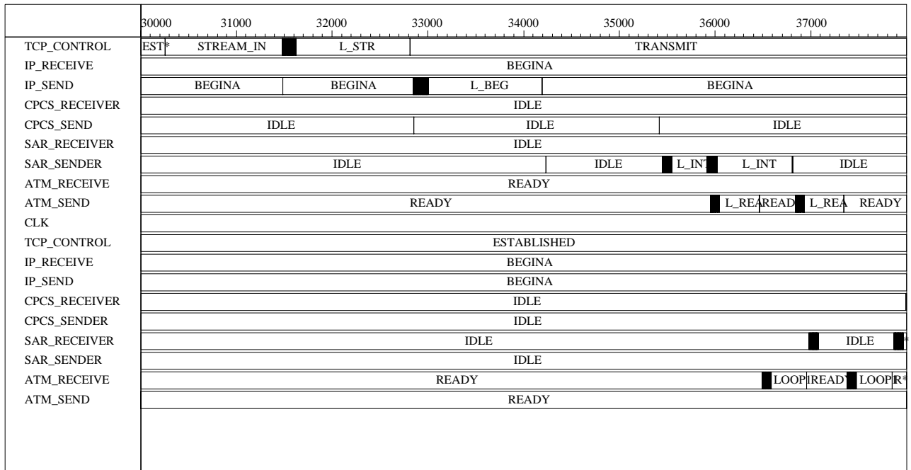
FIG. 6.21: Détail de la simulation VHDL de l'ATM
