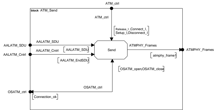
FIG. A.20: Structure du bloc d'émission de la couche ATM
