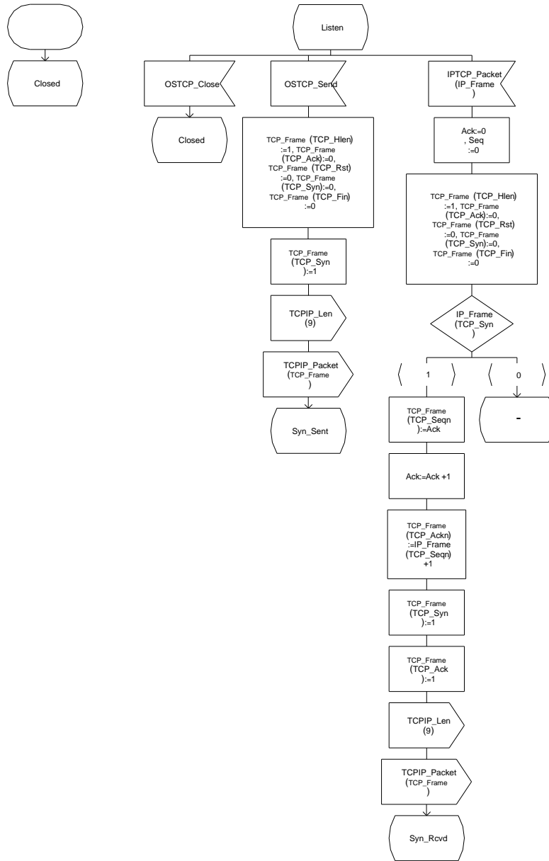
FIG. A.3: Automate de la couche TCP
