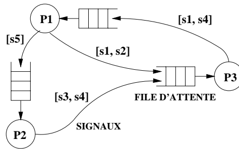
FIG. 3.11: Modèle de spécification SDL
