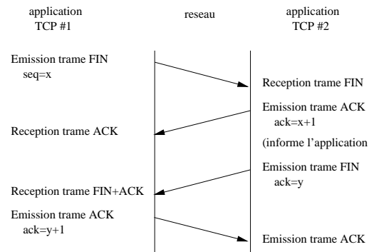
6.4.2: Fermeture d'une connexion TCP
