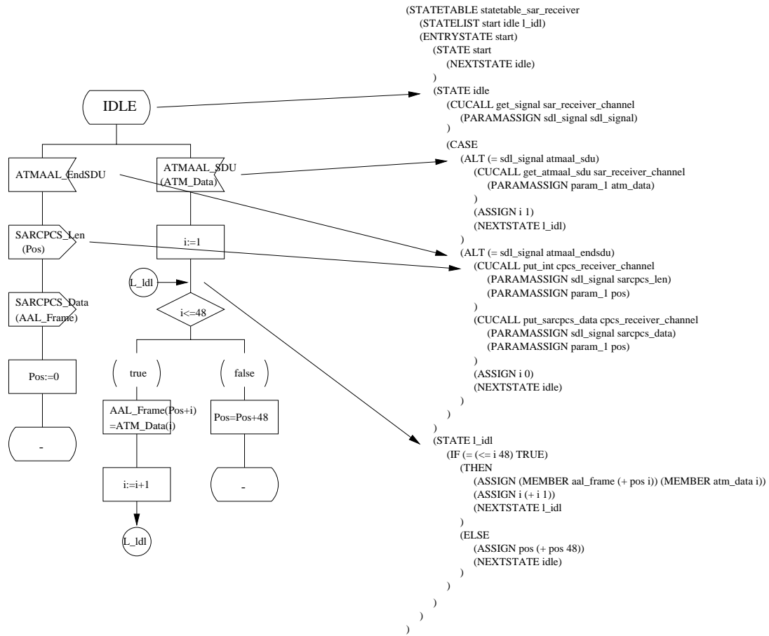
FIG. 5.3: Traduction SDL à SOLAR
