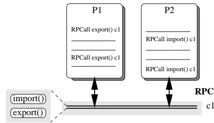
FIG. 5.5: Canal abstrait pour les variables importées et exportées
