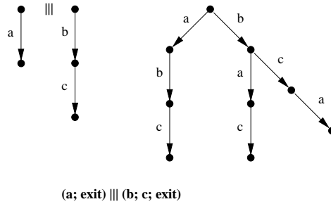
FIG. 3.6: Entrelacement de processus LOTOS
