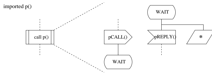
FIG. 3.16: Appel de procédure à distance en SDL : processus appelant
