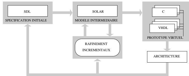
FIG. 2.1: Flôt de conception du système COSMOS
