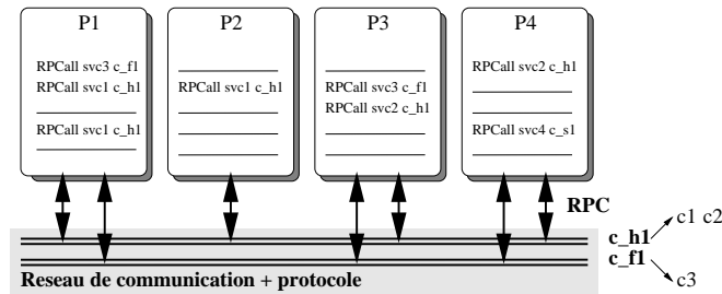
FIG. 4.11: Système après allocation des unités de communication
