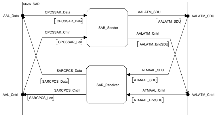
FIG. A.16: Structure de la couche SAR
