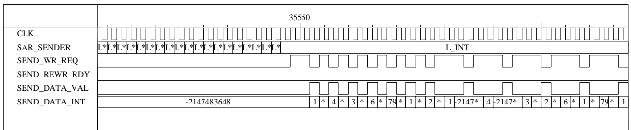
FIG. 6.23: Protocole de communication entre les processus sar_sender et atm_sender
