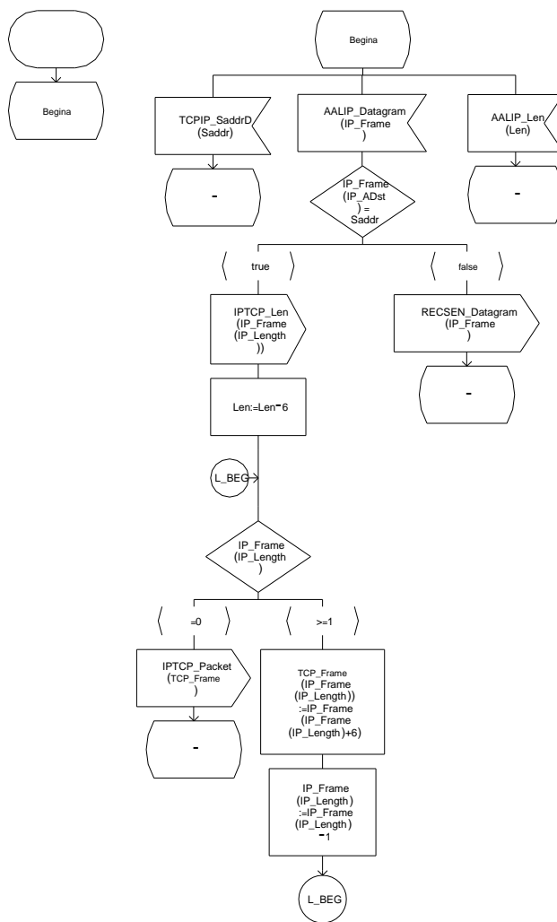
FIG. A.11: Automate de réception la couche IP
