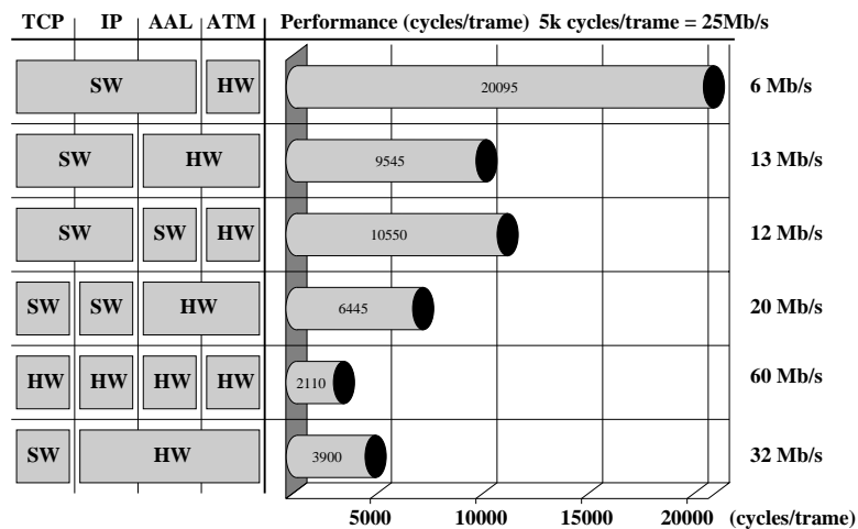
FIG. 6.18: Alternatives de partitionnement logiciel/matériel de l'ATM
