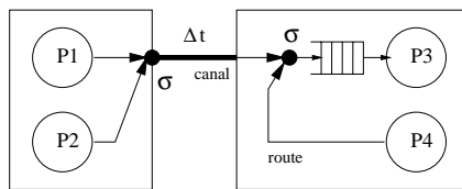
4.26.1: Non déterminisme dans le modèle de communication SDL
