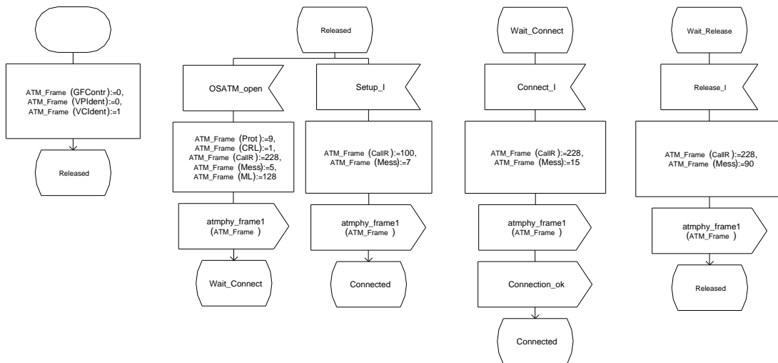
FIG. A.21: Automate d'émission la couche ATM
