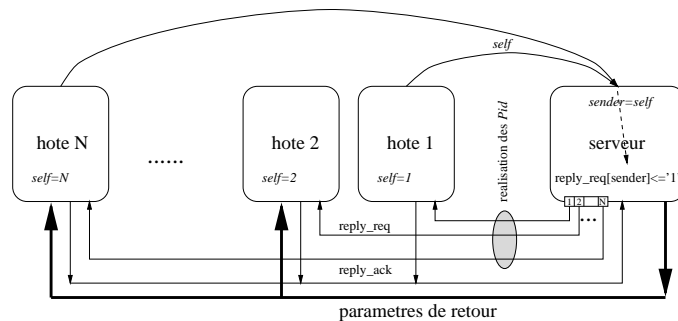
FIG. 4.25: Réalisation du canal RPC
