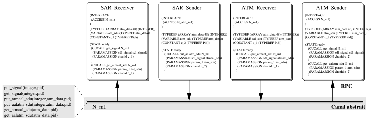
FIG. 4.19: Fusion de canaux abstraits
