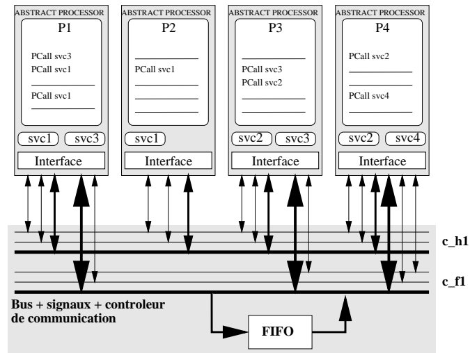
FIG. 4.14: Système après la synthèse d'interface
