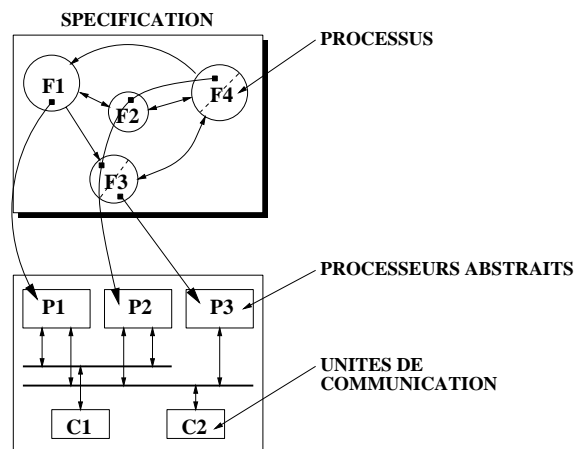
FIG. 2.9: Partitionnement pour les architectures multiprocesseurs
