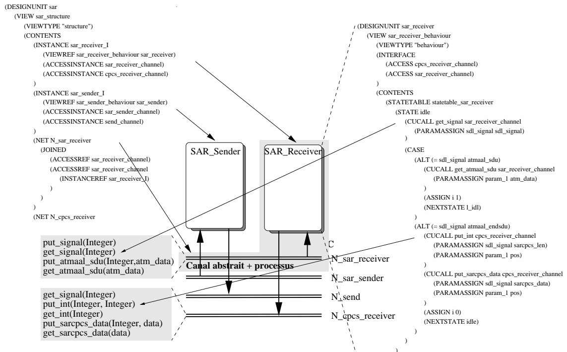
FIG. 5.2: Modélisation de la communication SDL à l'aide de canaux abstraits
