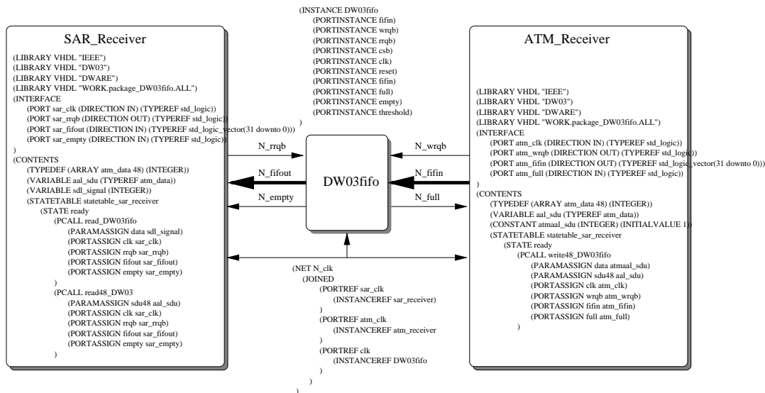
FIG. 4.22: Système interconnecté communiquant à travers des bus et des signaux
