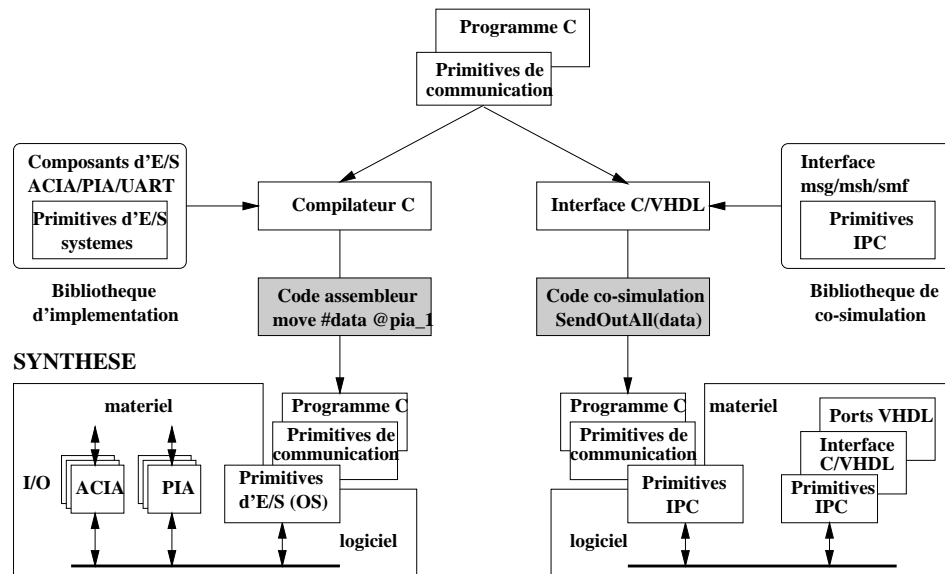
FIG. 2.10: Co-simulation logiciel/matériel
