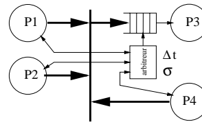
4.26.2: Réalisation VHDL
