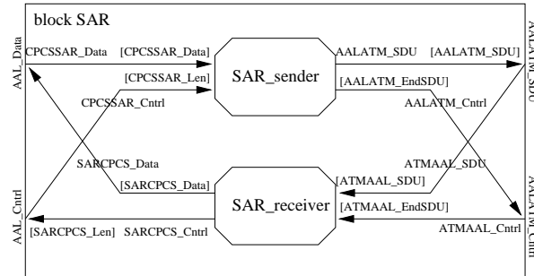
3.8.2: Bloc SDL
