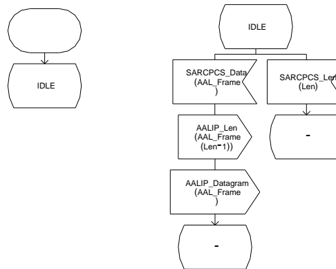
FIG. A.15: Automate de réception la couche CPCS
