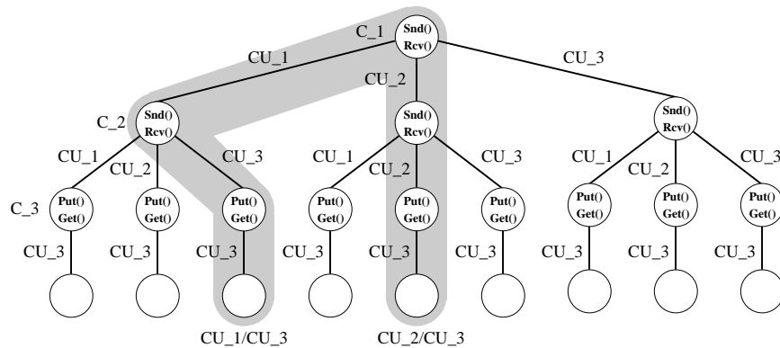
FIG. 4.17: Arbre de décision pour l'allocation
