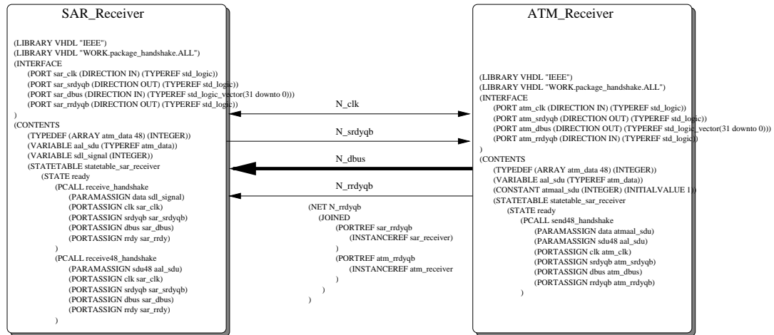
FIG. 4.23: Alternative de sélection de protocole/génération d'interface
