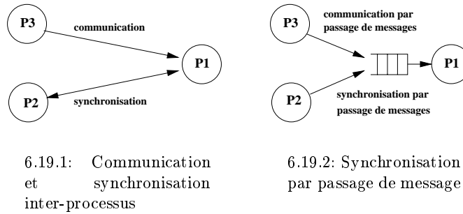
FIG. 6.19: Limitation de la communication en SDL
