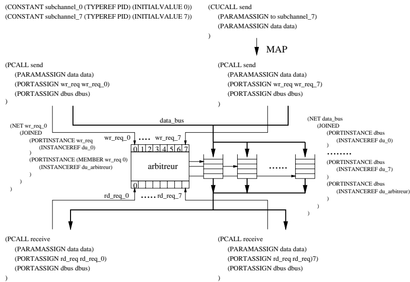
FIG. 4.24: Réalisation câblée du paramètre to Pid
