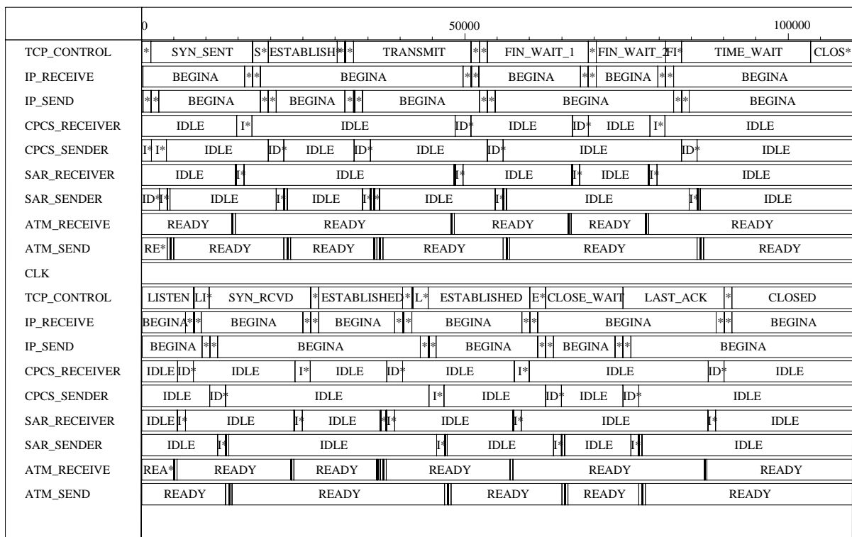
FIG. 6.20: Simulation VHDL de l'ATM
