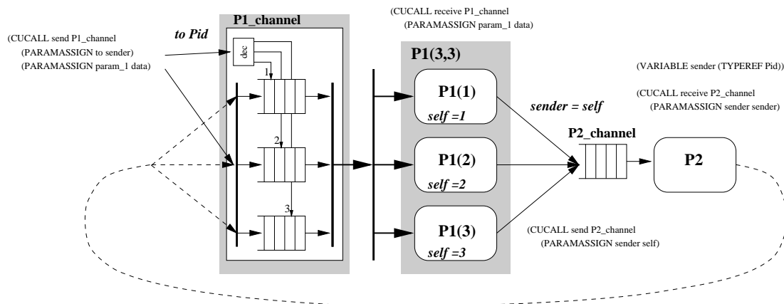
FIG. 5.4: Paramètre to et sender des primitives de communication
