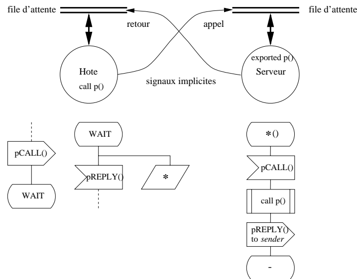
FIG. 5.6: Modèle d'exécution SDL des appels de procédure à distance
