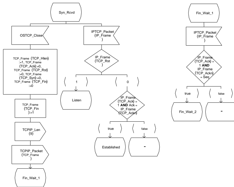
FIG. A.4: Automate de la couche TCP
