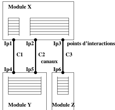
FIG. 3.3: Modules et canaux ESTELLE
