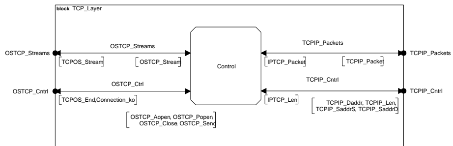
FIG. A.2: Structure de la couche TCP
