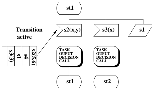
3.12.1: Automate d'états finis SDL
