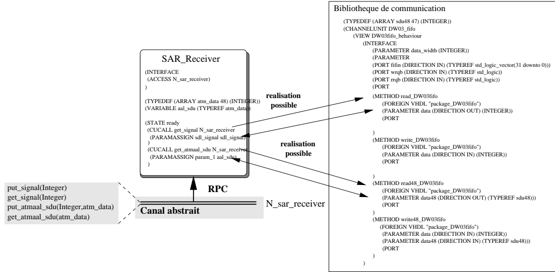
FIG. 4.20: Allocation d'une unité de communication pour un canal abstrait
