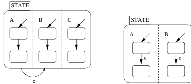
3.1.1: Synchronisation par initialisation
