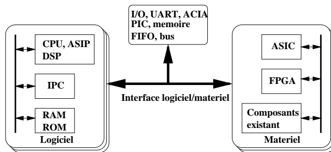
FIG. 2.11: Modèle d'architecture logicielle/matérielle
