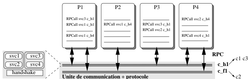
FIG. 4.10: Fusion de canaux abstraits sur une unité de communication
