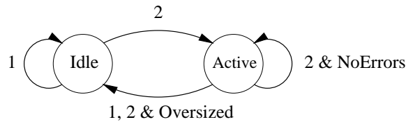
FIG. 6.11: Automate de réception de la couche AAL
