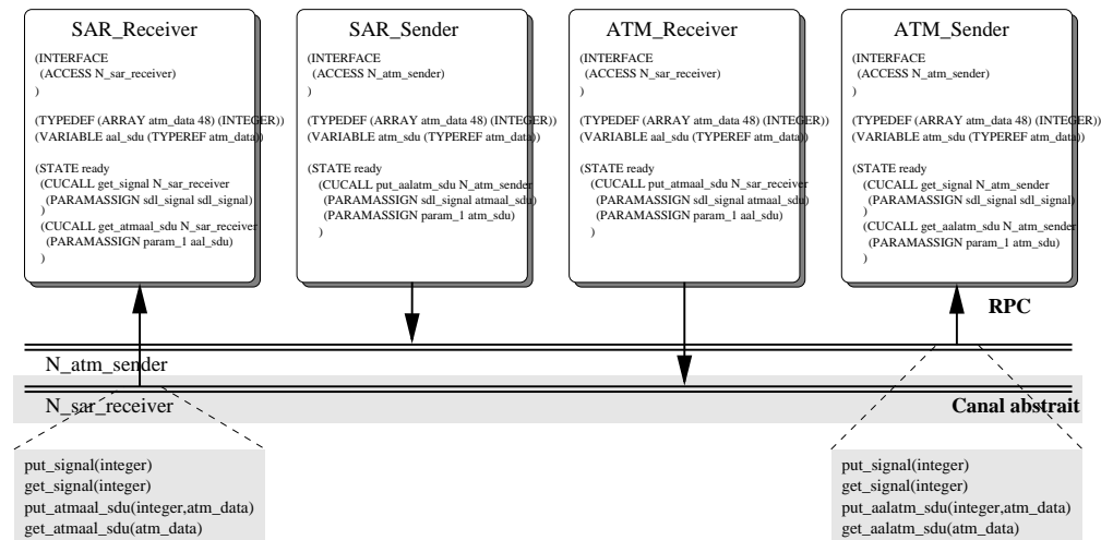
FIG. 4.2: Spécification de la communication à l'aide de canaux abstraits
