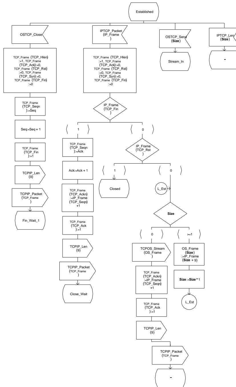
FIG. A.6: Automate de la couche TCP
