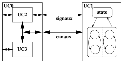
FIG. 2.6: Unité de conception structurelle et comportementale
