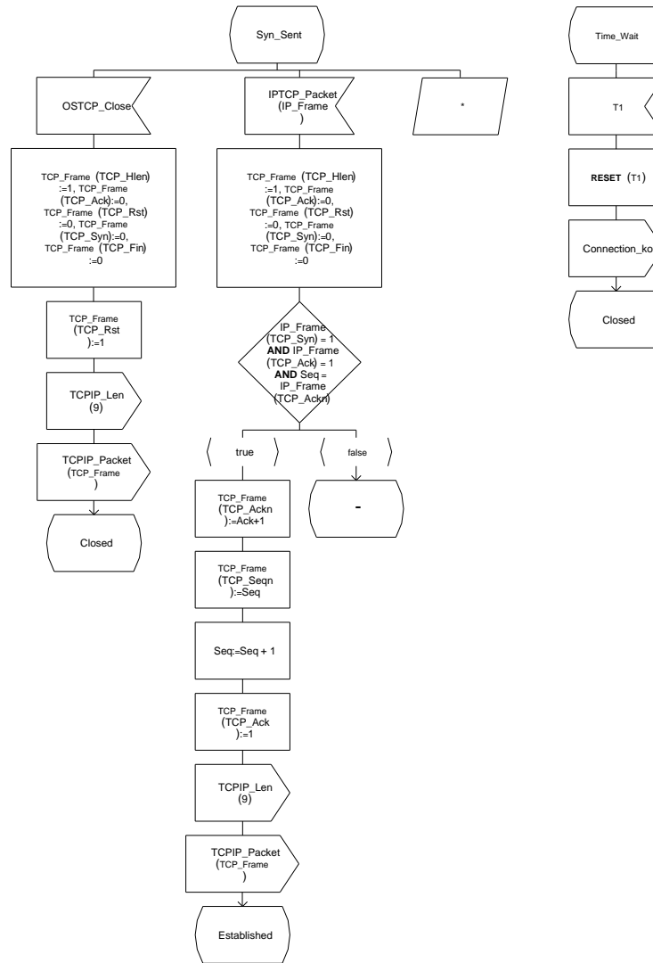
FIG. A.5: Automate de la couche TCP
