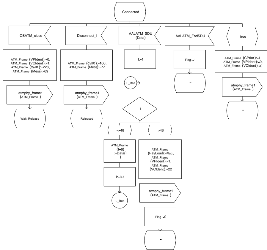
FIG. A.22: Automate d'émission la couche ATM
