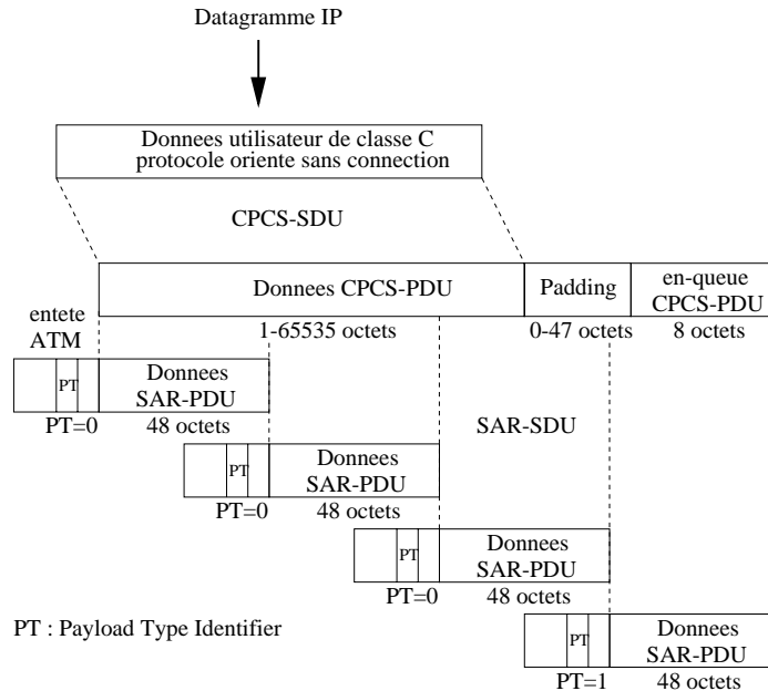
FIG. 6.10: Flût de données de la couche AAL 5
