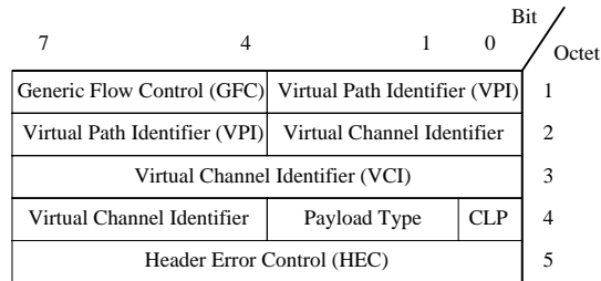
FIG. 6.13: Format de l'entête ATM
