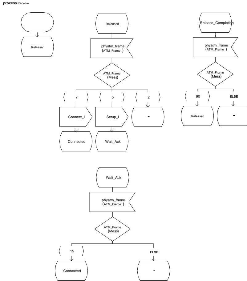
FIG. A.24: Automate de réception la couche ATM
