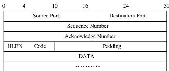
6.2.2: Structure de l'entête utilisée
