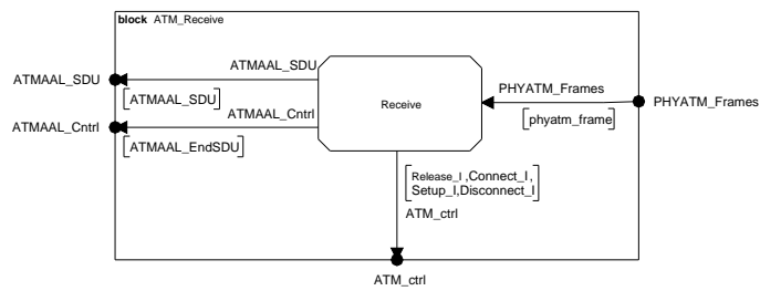
FIG. A.23: Structure du bloc de réception de la couche ATM
