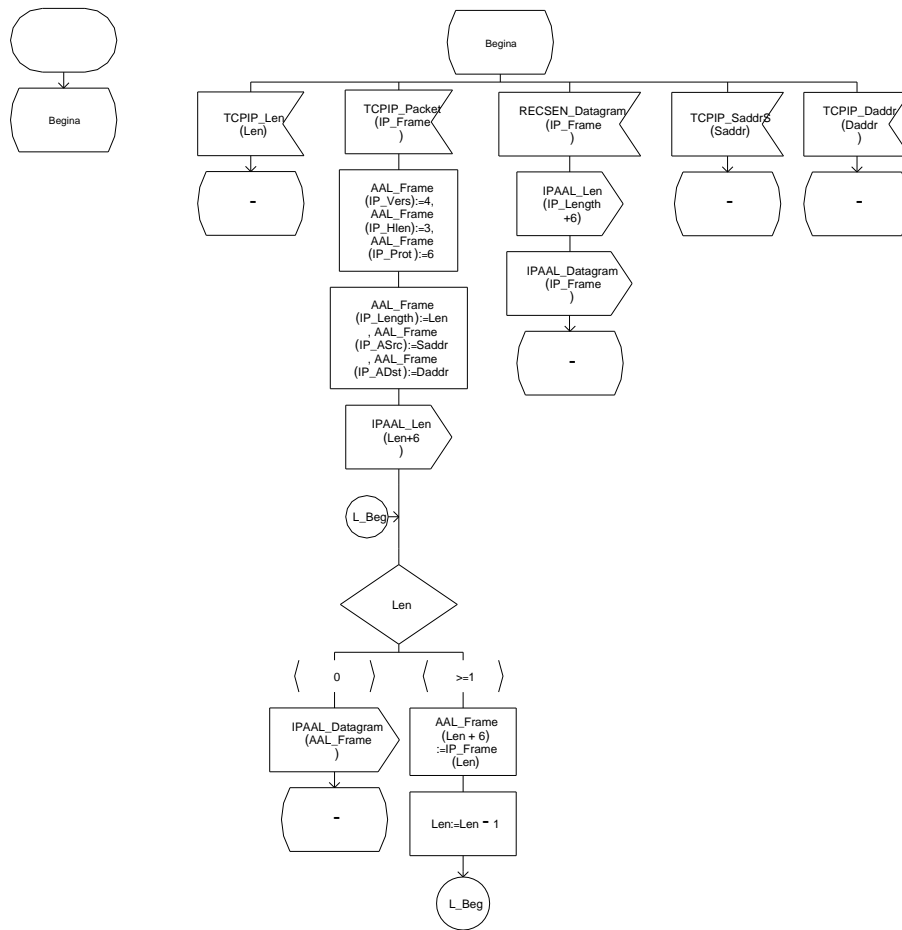
FIG. A.10: Automate d'émission la couche IP
