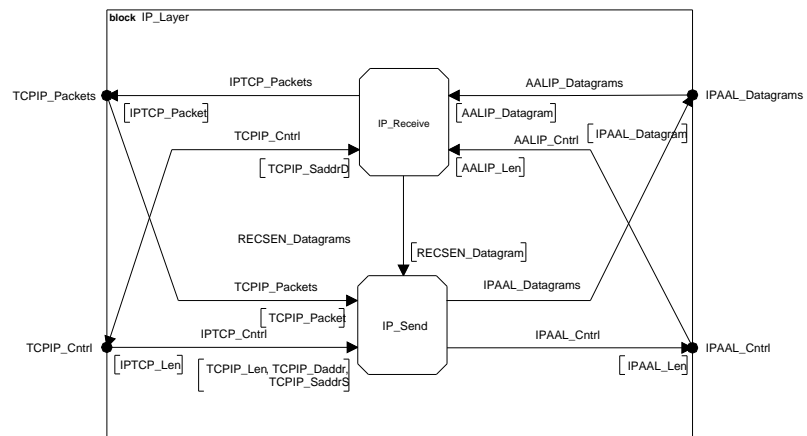
FIG. A.9: Structure de la couche IP
