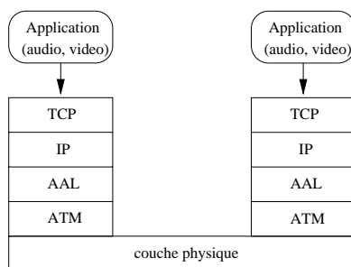
FIG. 6.1: Modèle général de l'application
