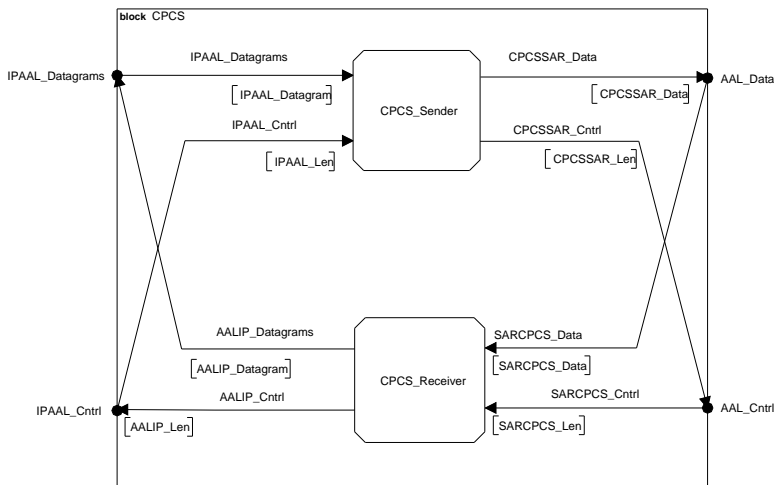
FIG. A.13: Structure de la couche CPCS
