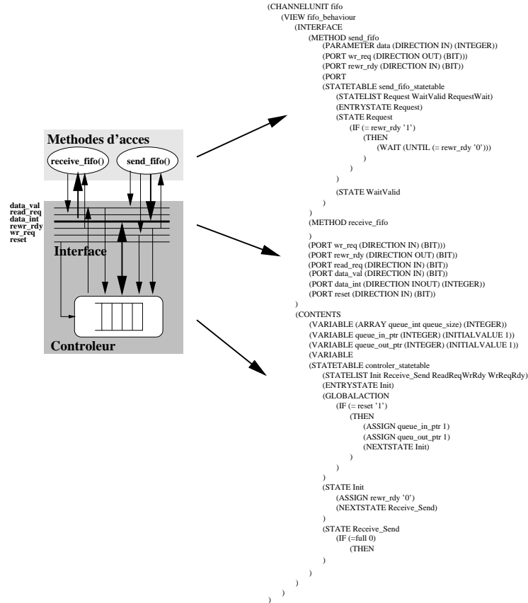
FIG. 2.3: Le canal SOLAR
