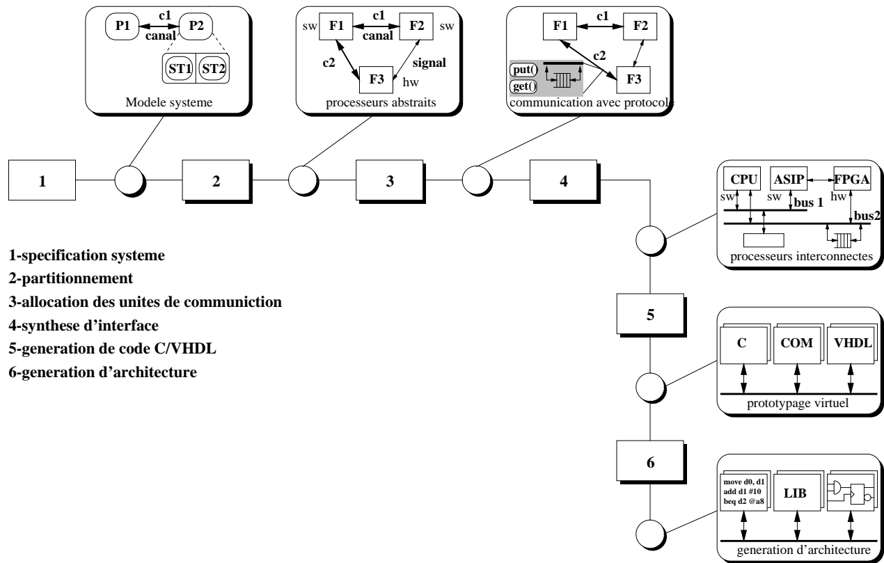
FIG. 2.8: Méthodologie de conception COSMOS
