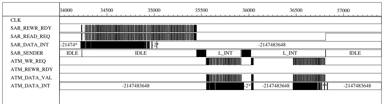
FIG. 6.22: Réalisation de la communication SDL en VHDL
