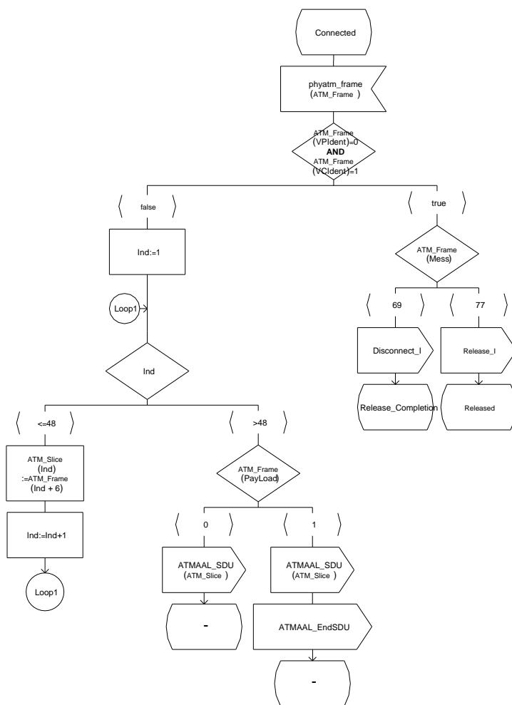
FIG. A.25: Automate de réception la couche ATM
