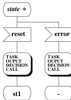
FIG. 3.15: Exception en SDL
