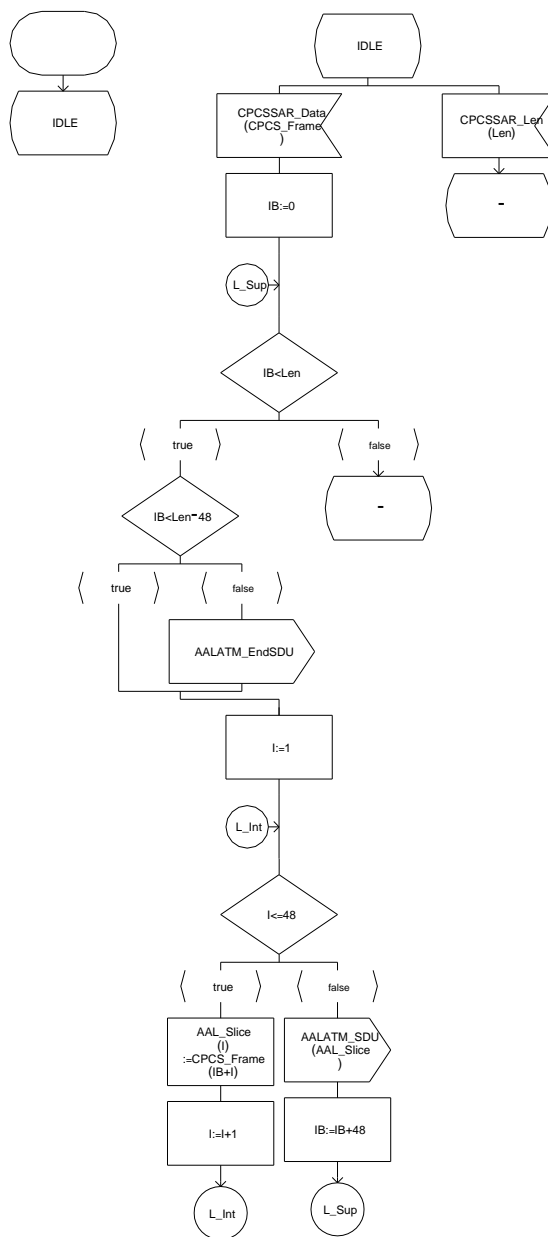
FIG. A.17: Automate d'émission la couche SAR
