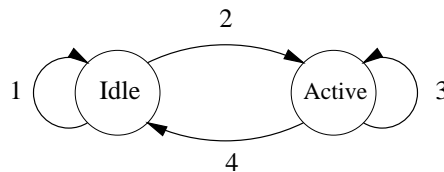
FIG. 6.12: Automate d'émission de la couche AAL
