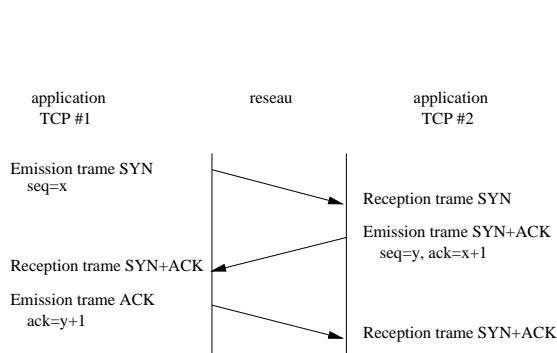
6.4.1: Ouverture d'une connexion TCP par protocole handshake
