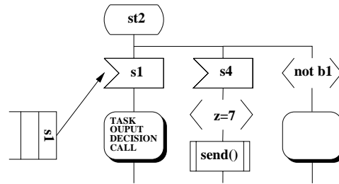
3.12.4: Signaux continus et condition d'autorisation
