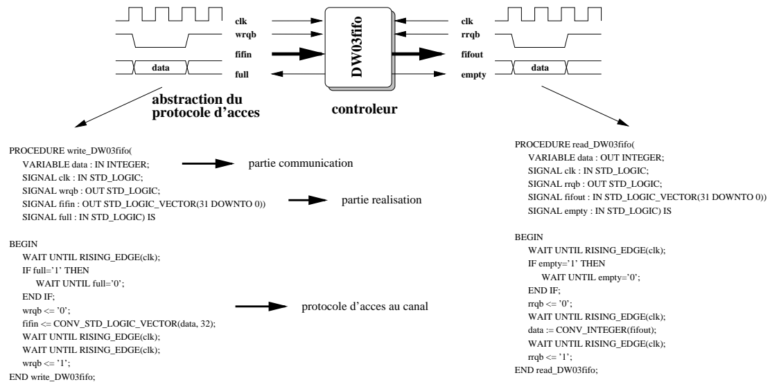
FIG. 4.4: Primitives de communication et abstraction d'un canal de communication
