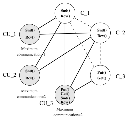
FIG. 4.15: Graphe de compatibilité pour l'allocation
