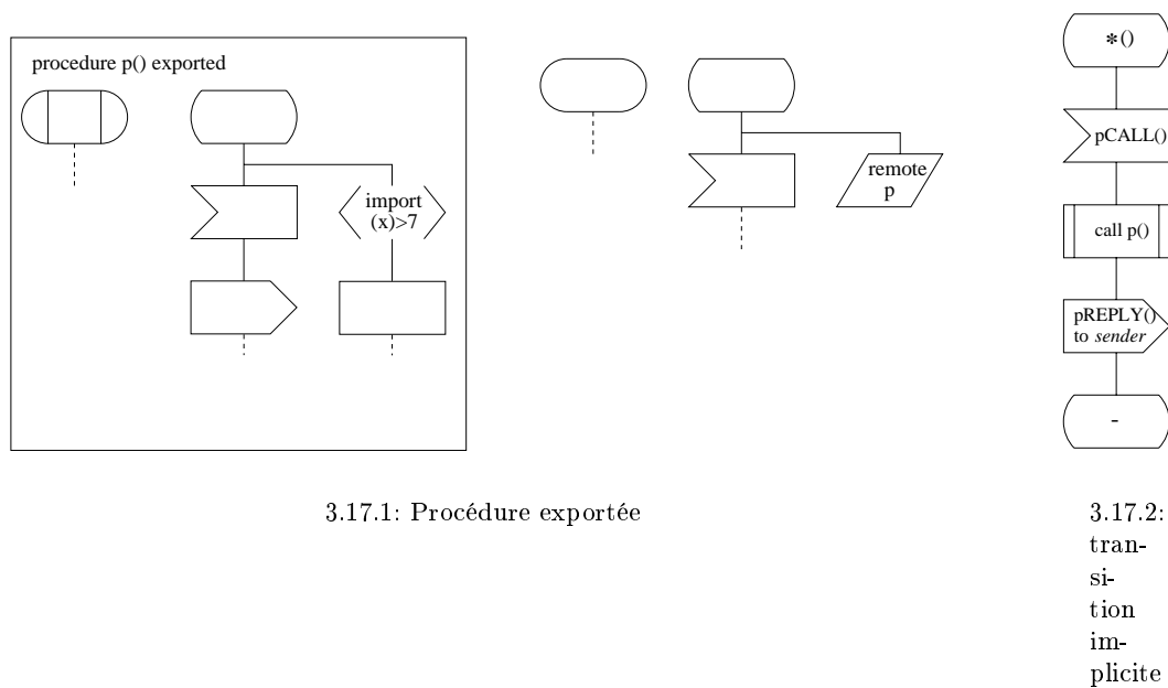
FIG. 3.17: Modèle d'exécution SDL des appels de procédure à distance : processus serveur
