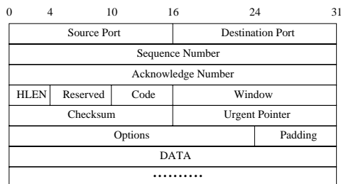
6.2.1: Structure d'une entête TCP
