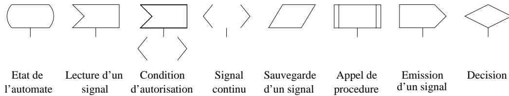
FIG. 3.12: Modèle d'exécution SDL
