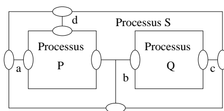
FIG. 3.5: Processus LOTOS
