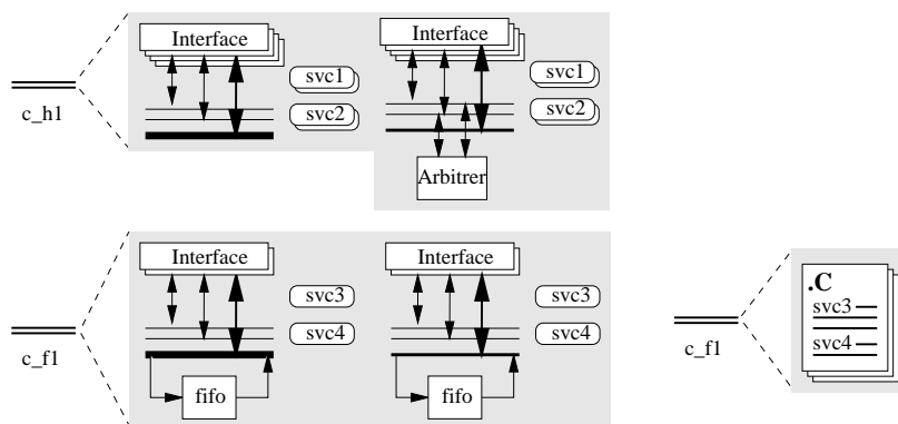
FIG. 4.13: Bibliothèque d'implémentation
