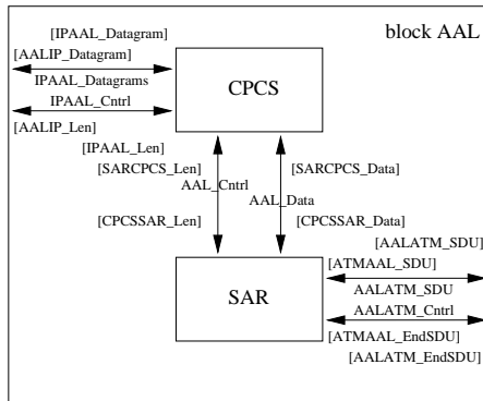
3.8.1: Système SDL
