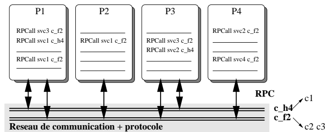
FIG. 4.12: Alternative d'allocation
