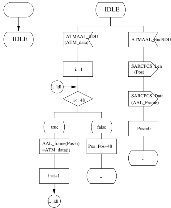
3.13.1: Description graphique de processus SDL
