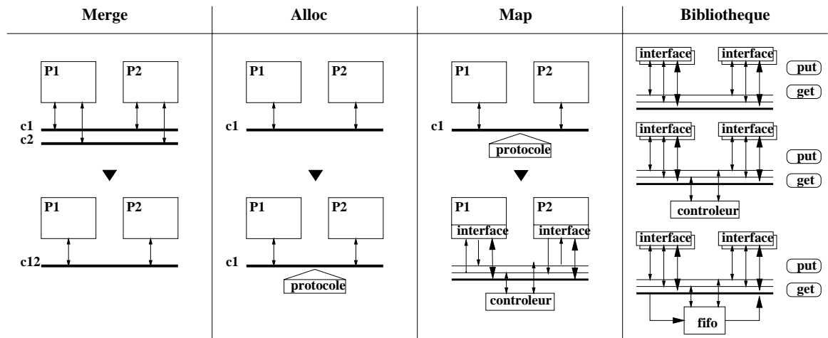
FIG. 4.18: Primitives pour la synthèse de la communication
