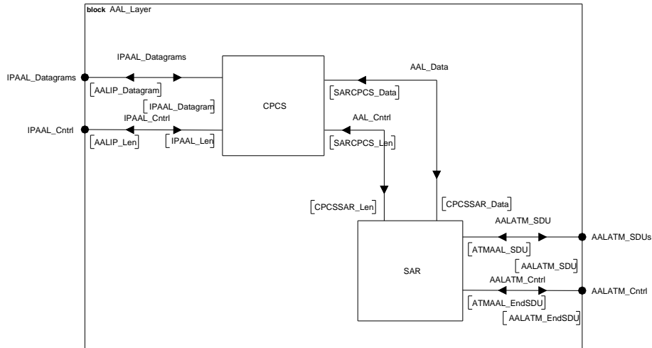
FIG. A.12: Structure de la couche AAL
