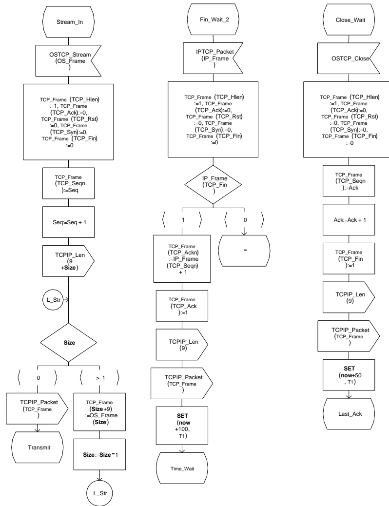
FIG. A.7: Automate de la couche TCP
