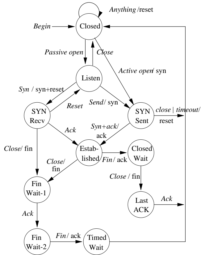
FIG. 6.3: Automate du protocole TCP
