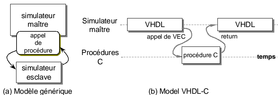
figure 3.1 : Cosimulation maître-esclave
