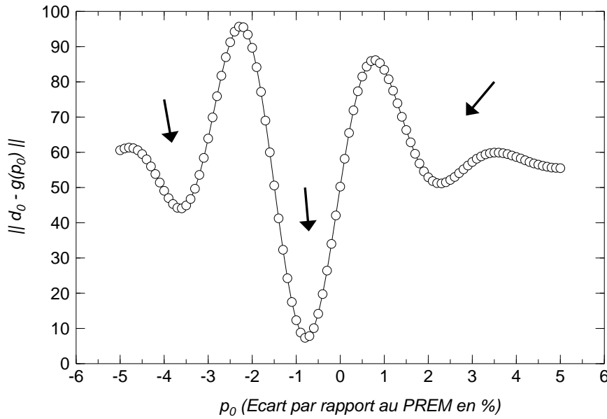
FIG. 2.10: Exploration de l'espace des modèles de départ possibles à très grande échelle fréquentielle entre -5% et 5% avec un pas de 0.1%. L'écart (ou distance) entre la donnée ( \mathbf{d} ) et son image obtenue par la fonction g est calculé pour chaque \mathbf{p}_{k=0} . Chaque minimum que l'on désigne ici par une flèche est susceptible d'être un modèle de départ.
