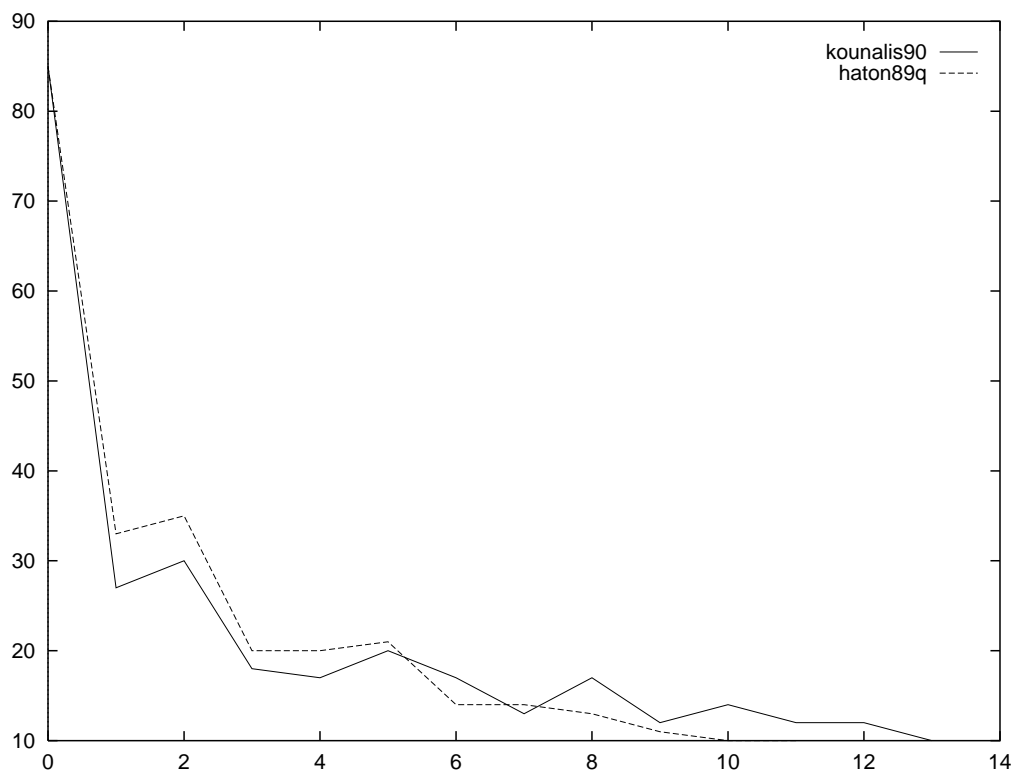
FIG. 4.29 – Évolution des températures lors des traitements des références kounalis90a et haton89q .
