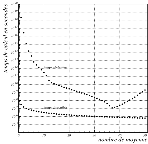
Figure 7.24: Temps de calcul en fonction du nombre de transformées
