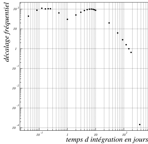
Figure 7.16: Décalage fréquentiel moyen en fonction du temps d'intégration
