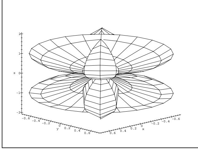
Figure 5.10: Diagramme d'antenne pour une onde polarisée h_x . Les bras du détecteur coïncident avec l'axe des x et l'axe des y
