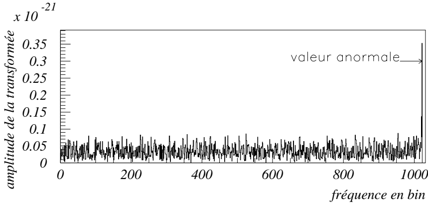
Figure 7.13: Visualisation du lot de données 31
