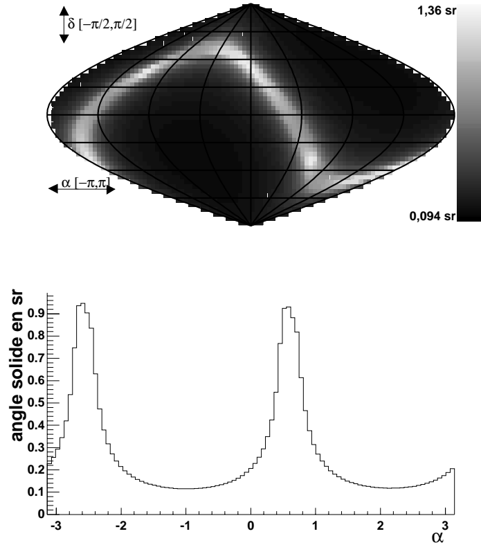
Figure 5.5: Taille de l'erreur tolérable sur la position d'une étoile à neutrons pour un jour d'intégration à une fréquence de 20 Hz, suivant la direction de la source en coordonnées galactiques
