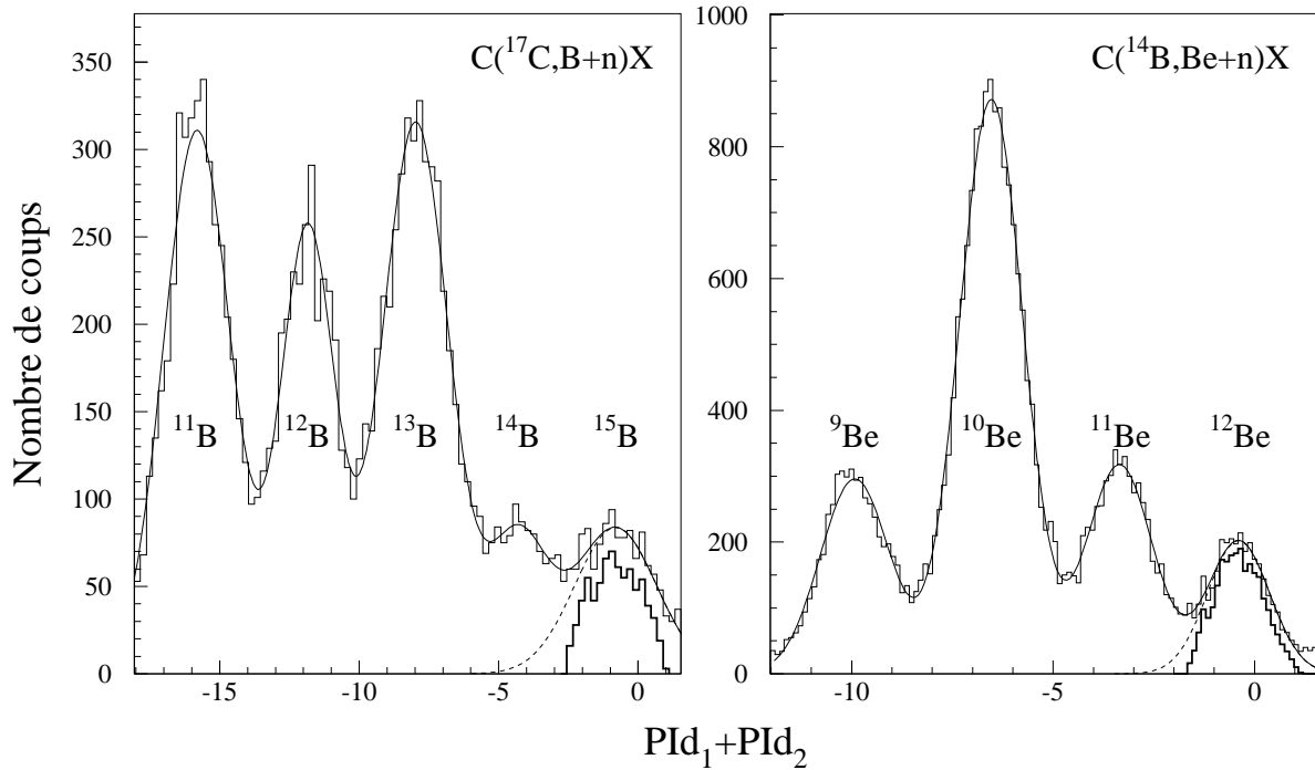
FIG. 4.1 – Sélection des isotopes de B (première expérience) et de Be (seconde expérience). Les courbes en trait plein sont des ajustements gaussiens aux spectres PID_1+PID_2 . Les courbes en trait pointillé correspondent aux composantes gaussiennes associées au ^{15}\text{B} et au ^{12}\text{Be} . Les spectres en trait épais résultent de la sélection bidimensionnelle du ^{15}\text{B} et du ^{12}\text{Be} .
