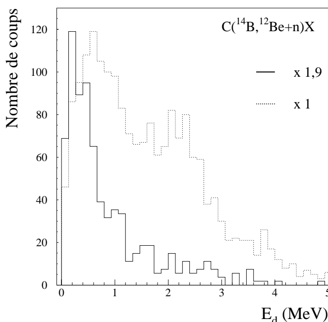
FIG. 5.20 – Spectre en énergie de décroissance du ^{13}\text{Be} obtenu avec une acceptation angulaire neutron limitée à 5^\circ (trait continu). L'histogramme en pointillé est le spectre obtenu en utilisant tous les modules DéMoN.
