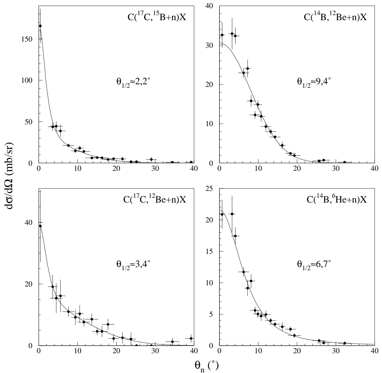
FIG. 4.3 – Sections efficaces angulaires des neutrons en coïncidence avec le ^{15}\text{B} et le ^{12}\text{Be} de la première expérience (à gauche) et le ^{12}\text{Be} et l' ^6\text{He} de la seconde (à droite). Les barres d'erreur ne prennent pas en compte l'incertitude sur \mathcal{K} . L'angle noté \theta_{1/2} correspond à la largeur à mi-hauteur des courbes ajustées aux données.
