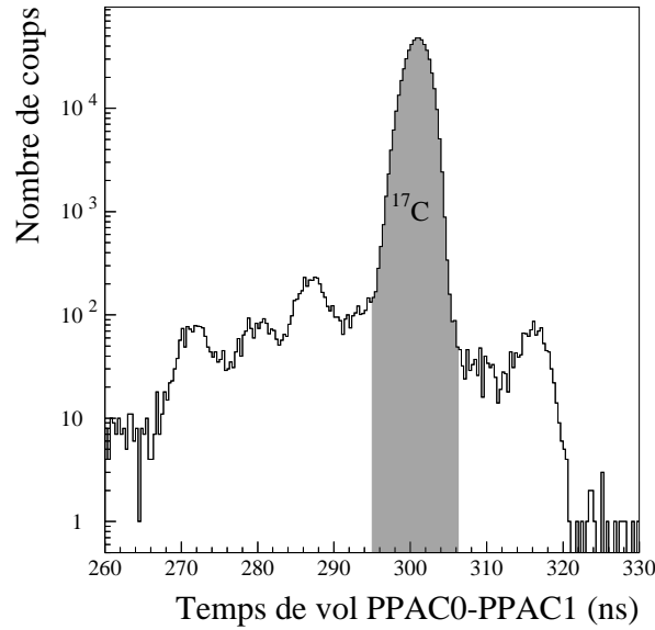
FIG. 3.5 – Spectre en temps de vol des ions incidents (98% de 17 C).
