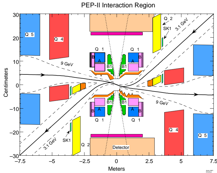
FIG. 2.2 – Système optique de PEP-II au voisinage du point d’interaction
