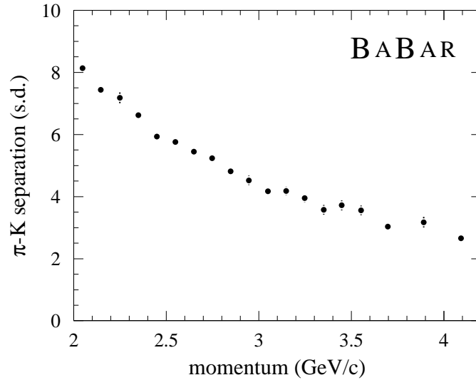
FIG. 3.16 – Pouvoir séparateur du DIRC entre les hypothèses pion et kaon, déterminé avec un échantillon de contrôle de D^* , en fonction de l'impulsion des traces rentrant dans le DIRC.
