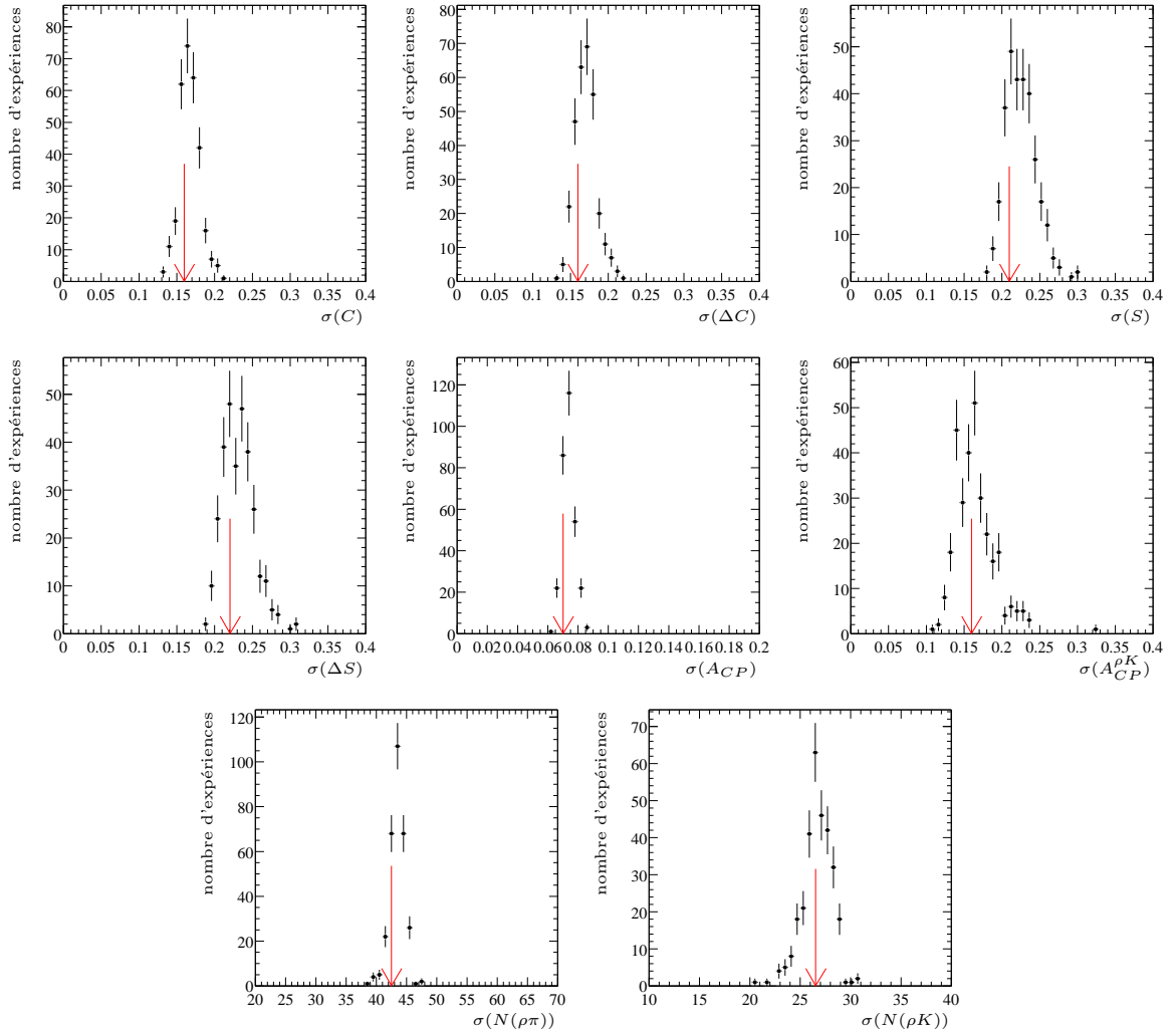
FIG. 4.27 – Distribution de l'erreur obtenue dans les échantillons de Monte-Carlo rapide, pour les 8 paramètres mesurés. La flèche indique l'erreur de l'ajustement des vraies données.
