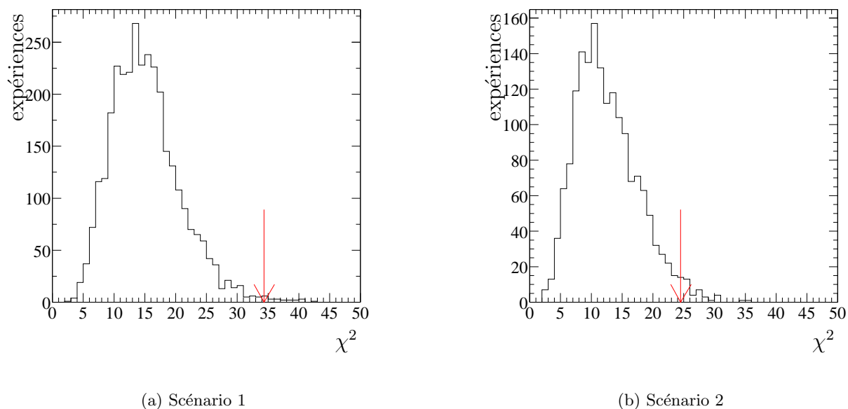
FIG. 5.5 – Distribution de \chi^2 trouvée dans les échantillons de Monte-Carlo rapides (histogramme), comparée à la valeur obtenue dans les données (flèche). Le scénario 1 se réfère à la “factorisation QCD” pure, et le “scénario 2” à la correction additionnelle des “pingouins charmants”.
