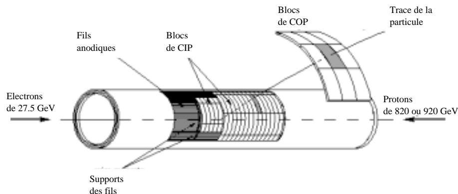
FIG. 2.6 – Schéma d'une chambre proportionnelle multifil intérieure CIP, et des premiers blocs d'une chambre extérieure COP.
