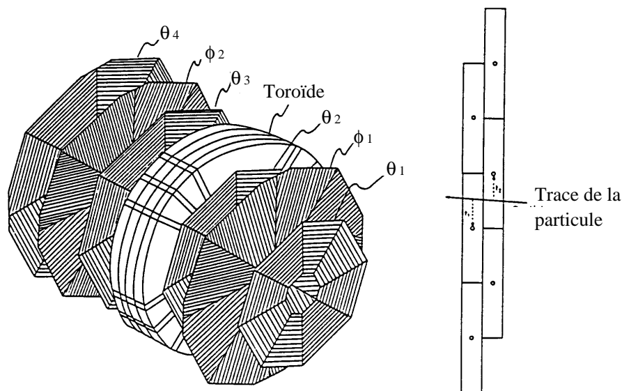
FIG. 2.19 – Vue schématique du spectromètre à muons avant. Le schéma de droite illustre la levée de l’ambiguïté de reconstruction des traces grâce au décalage des plans de fils.
