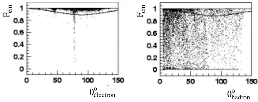
FIG. 2.11 – Spectre de la fraction électromagnétique F_{EM} en fonction de l'angle polaire de l'amas, pour des amas d'électrons (figure de gauche) et des amas de hadrons (figure de droite). La courbe continue représente la coupure F_{EM}^{min} au-dessus de laquelle les amas sont sélectionnés.
