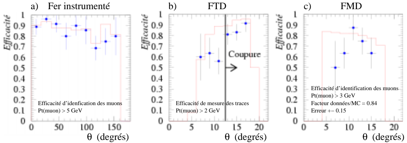
FIG. 4.2 – Efficacité d'identification des muons dans le fer instrumenté (figure a), efficacité de mesure des traces dans le FTD (figure b) et efficacité d'identification des muons dans le FMD (figure c). Les données sont représentées par des points et le Monte-Carlo LPAIR de production de paires de muons est représenté sous forme d'histogramme.
