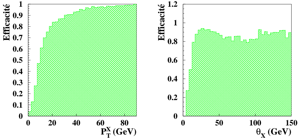
FIG. 2.22 – Efficacité de déclenchement en fonction de l'impulsion transverse P_T^X , et de l'angle polaire \theta_X du système hadronique pour P_T^X > 12 GeV, dans le cas de production de W suivie de sa désintégration W \rightarrow \mu\nu avec le Monte-Carlo EPVEC.
