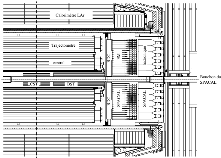
FIG. 2.16 – Vue longitudinale du calorimètre arrière de H1 (SPACAL).
