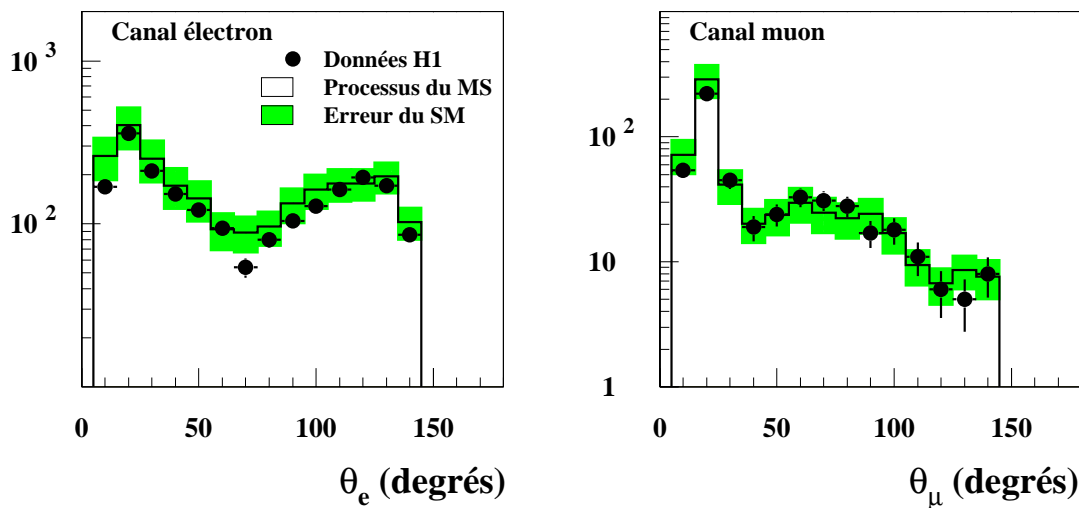
FIG. 4.21 – Distribution de l'angle polaire du second électron reconstruit (figure de gauche) et du muon reconstruit (figure de droite), dans une sélection de courants neutres avec la contrainte d'un deuxième lepton identifié, sur l'ensemble des données e^+p de HERA-1 correspondant à une luminosité intégrée de 104.7 \text{ pb}^{-1} . Des erreurs de 30% sur la prédiction du Modèle Standard ont été considérées.
