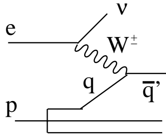
FIG. 3.14 – Interaction profondément inélastique à courant chargé.
