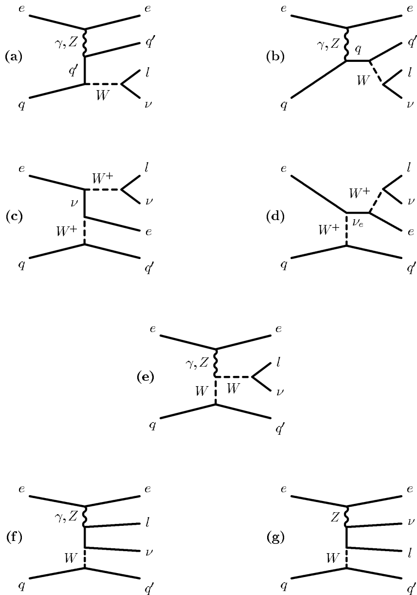
FIG. 3.2 – Diagrammes de premier ordre de production du boson W par les interactions ep \rightarrow eWX : rayonnement du W à partir de la diffusion d'un quark du proton (a et b) ; production impliquant l'échange d'un deuxième boson W (c et d) ; W produit depuis un vertex WW\gamma (e) ; diagrammes de production non résonante de W (f et g).
