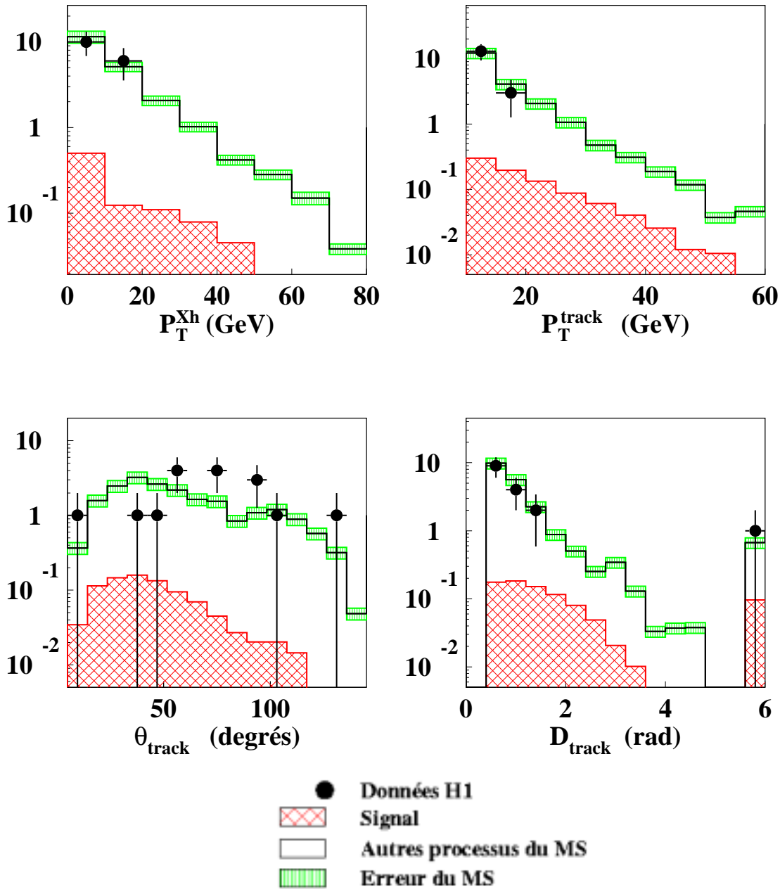
FIG. 4.23 – Distributions de l'impulsion transverse hadronique P_T^{Xh} , l'impulsion transverse de la trace candidate P_T^{track} , de son angle polaire \theta_{track} et de son isolation D_{track} par rapport aux autres traces, pour l'échantillon hadron isolé (données e^+p , 104.7 \text{ pb}^{-1} ). Le dernier intervalle de la distribution en P_T^{Xh} ( D_{track} ) contient tous les événements dont la valeur de P_T^{Xh} ( D_{track} ) est au-dessus de la limite supérieure de l'histogramme.
