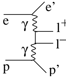
FIG. 3.16 – Production de paires de leptons.
