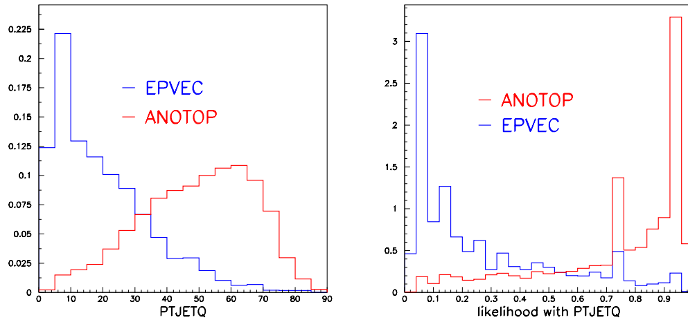
FIG. B.7 – Distribution de la variable d'entrée P_T^{jet} avec discrétisation grossière et distribution de la vraisemblance résultante.
