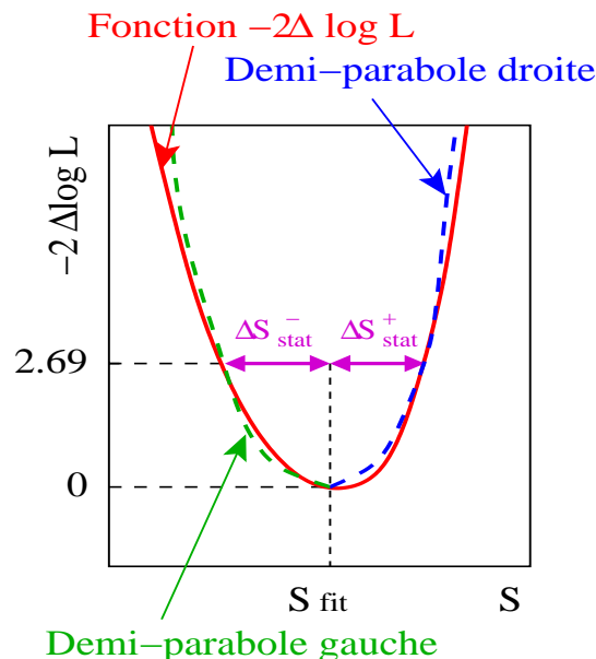
FIG. 5.16 – Schéma représentant le choix des largeurs des demi-paraboles utilisées pour approximer la fonction -2\Delta \log \mathcal{L} . Ces largeurs sont déterminées pour la valeur -2\Delta \log \mathcal{L} = 2.69 .
