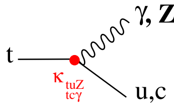
FIG. 5.20 – Diagramme de production de top par couplage anormal \kappa_{tuZ} ou \kappa_{tc\gamma} au Tevatron.
