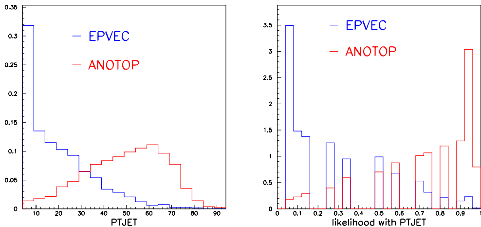
FIG. B.5 – Distribution de l'impulsion transverse du jet pour le signal ANOTOP et le bruit EPVEC (figure de gauche) et fonction de vraisemblance uni-dimensionnelle résultante avec P_T^{jet} comme variable d'entrée.
