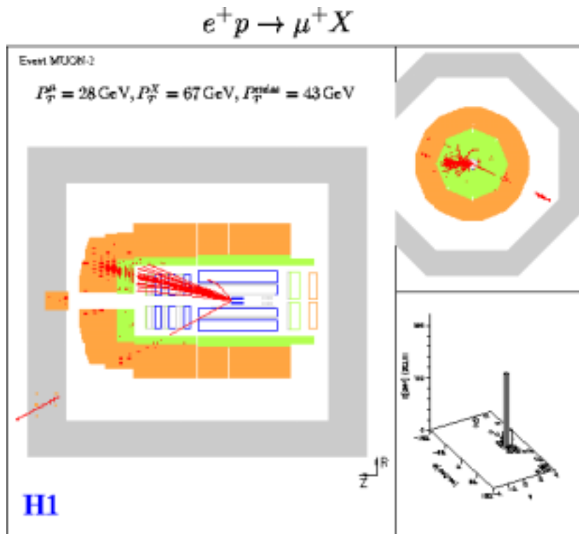
FIG. 3.1 – Exemple de candidat à muon isolé et impulsion transverse manquante (extrait des données 1997 e^+p ).
