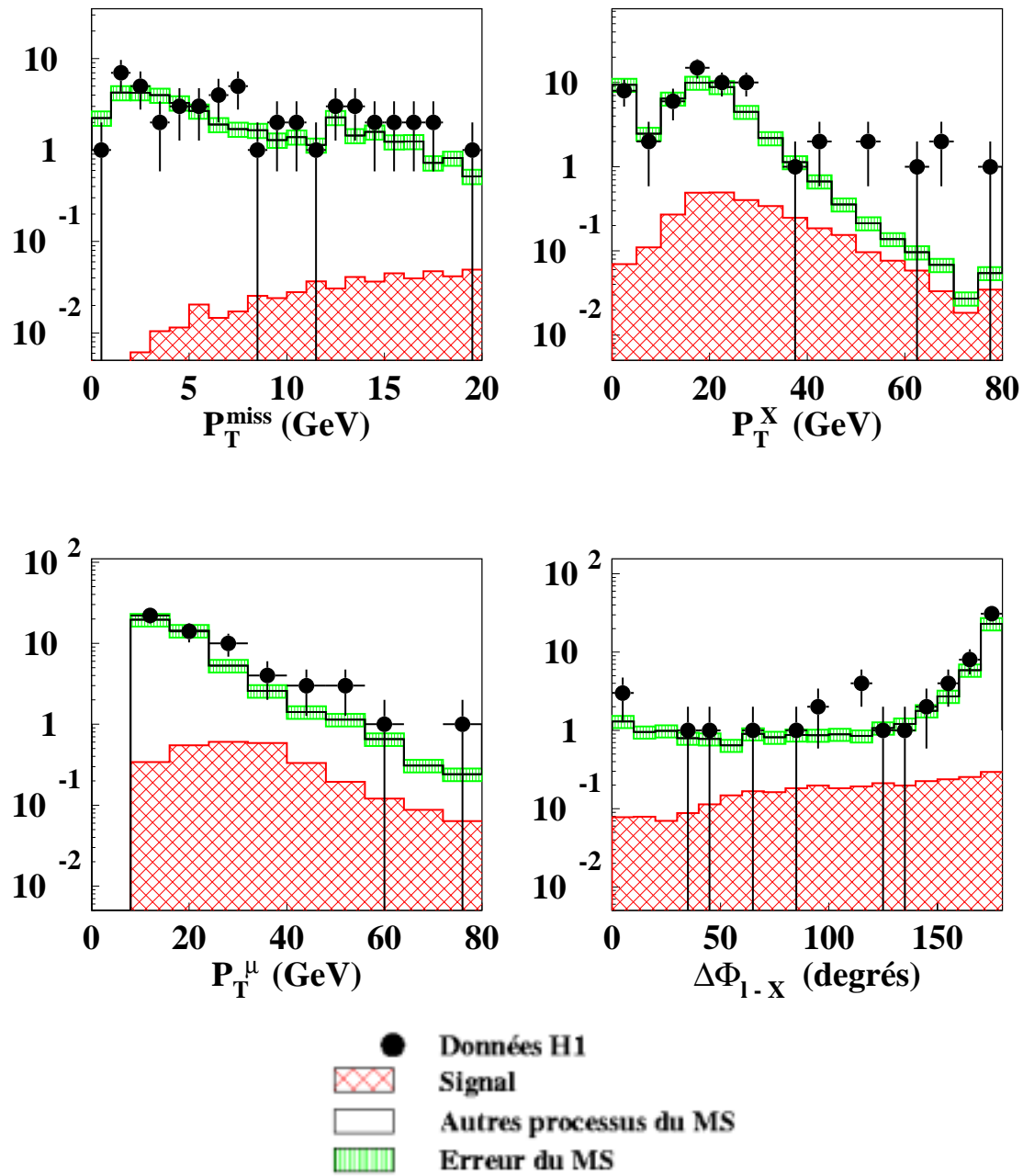
FIG. 4.19 – Distributions de contrôle dans le canal muon pour l'échantillon enrichi en production de paires de muons et en photoproduction (données e^+p , 104.7 \text{ pb}^{-1} ). Le dernier intervalle de la distribution en P_T^X contient tous les événements dont la valeur de P_T^X est au-dessus de la limite supérieure de l'histogramme.
