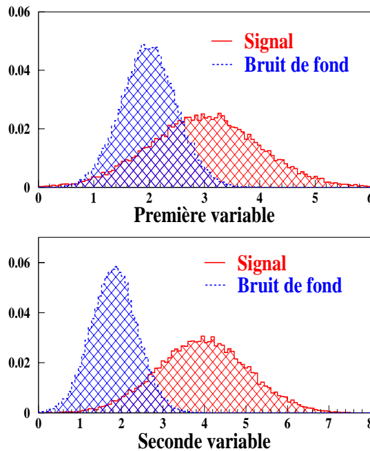
FIG. B.1 – Distribution des variables simulées par des fonctions tests. Un coefficient de corrélation de 0.9 a été choisi. Les distributions en trait continu (pointillés) représentent le signal (bruit).
