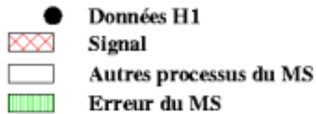
FIG. A.3 – Distributions de D_{jet} et P_T^X pour le canal électron (figures du haut) et de D_{track} et P_T^X pour le canal muon (figures du bas) après la sélection de 1998 étendue à l'ensemble des données e^+p ( 104.7 \text{ pb}^{-1} ). Le dernier intervalle de la distribution en P_T^X contient tous les événements dont P_T^X est au-dessus de la limite supérieure de l'histogramme.
