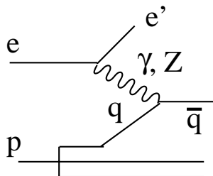
FIG. 3.12 – Diffusion profondément inélastique à courant neutre.
