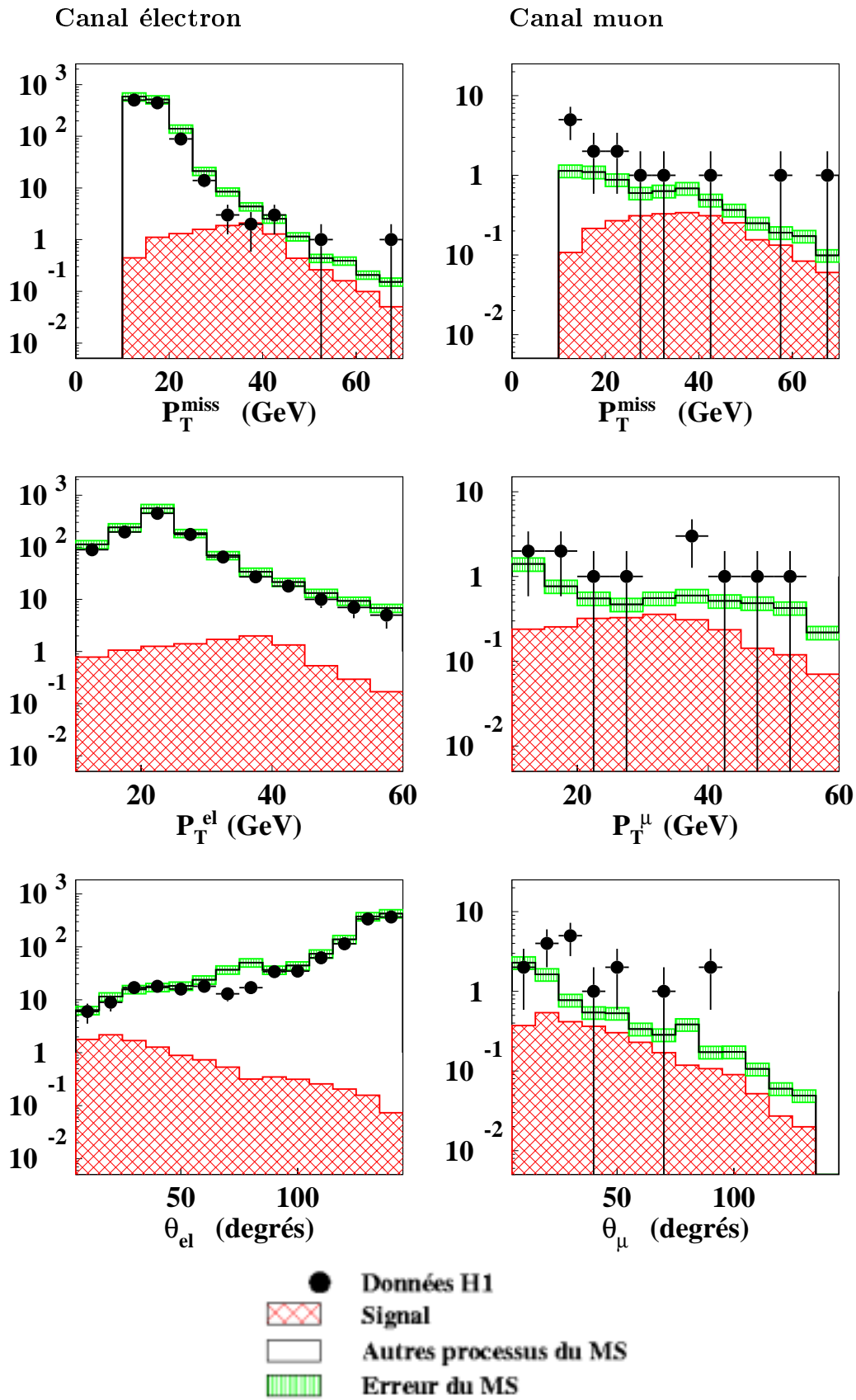
FIG. 4.9 – Impulsion transverse calorimétrique de l'événement, impulsion transverse et angle polaire du lepton final pour le canal électron (figures de gauche) et le canal muon (figure de droite), pour l'ensemble des données e^+p ( 104.7 \text{ pb}^{-1} ) dans l'espace de phase P_T^{cal} > 12 \text{ GeV} , P_T^{miss} > 12 \text{ GeV} , P_T^{lep} > 10 \text{ GeV} et 5^\circ < \theta_{lep} < 140^\circ .
