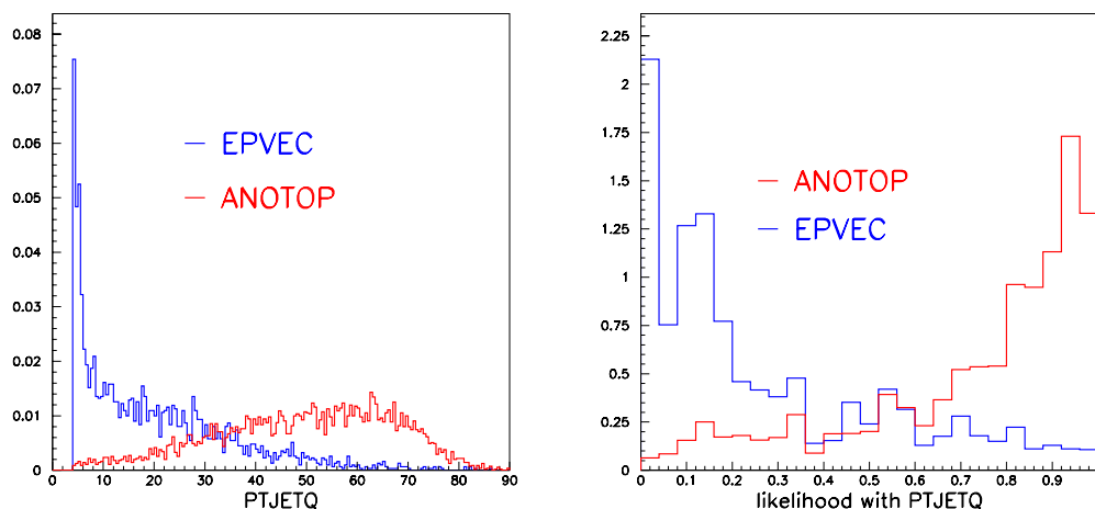
FIG. B.6 – Distribution de la variable d'entrée P_T^{jet} avec une discrétisation fine et distribution de la vraisemblance résultante.
