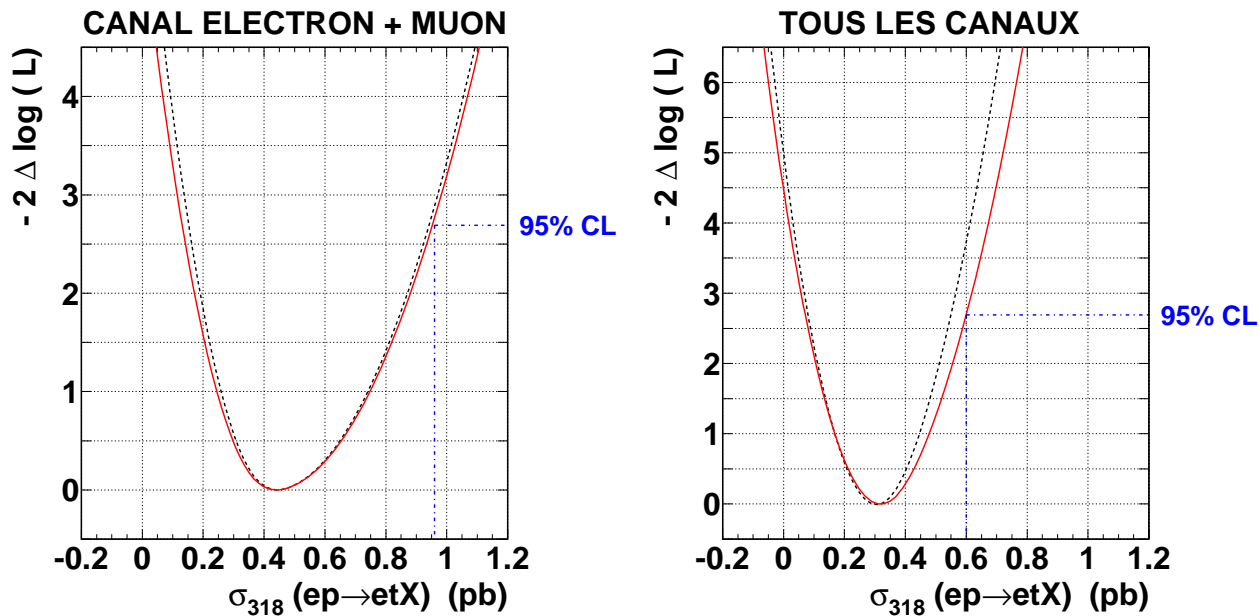
FIG. 5.18 – Ajustement -2\Delta \log \mathcal{L} en fonction de la section efficace de production du top, pour la combinaison des canaux leptoniques (figure de gauche) et de l'ensemble des canaux (figure de droite). La courbe continue représente la fonction exacte -2\Delta \log \mathcal{L} et la courbe en pointillés représente son approximation à deux paraboles, tenant compte des erreurs systématiques.
