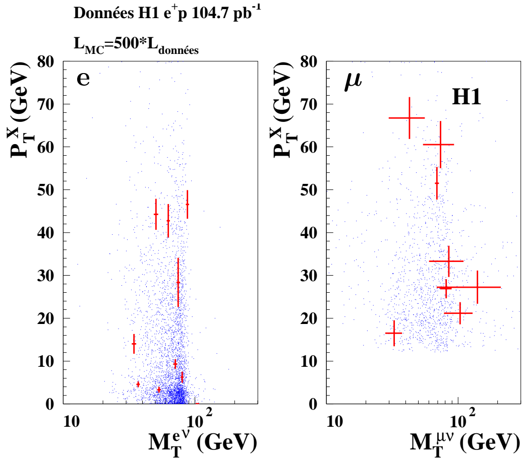
FIG. 4.16 – Distribution de l'impulsion transverse du système hadronique des événements en fonction de la masse transverse M_T^{l\nu} , pour le canal électron (figure de gauche) et le canal muon (figure de droite). Les croix représentent les candidats sélectionnés avec leurs erreurs et les points correspondent à la prédiction du signal simulée pour une luminosité de 500 fois la luminosité des données.
