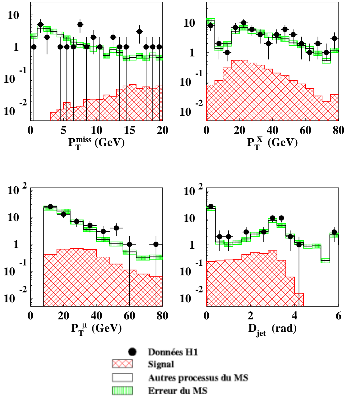
FIG. 4.20 – Distributions de contrôle dans le canal muon pour l'échantillon enrichi en production de paires de muon et en courants chargés (données e^+p , 104.7 \text{ pb}^{-1} ). Le dernier intervalle de la distribution en P_T^X ( D_{jet} ) contient tous les événements dont la valeur de P_T^X ( D_{jet} ) est au-dessus de la limite supérieure de l'histogramme.
