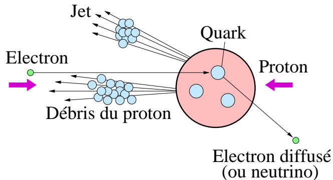
FIG. 1.2 – Schéma d'une interaction électron-proton.
