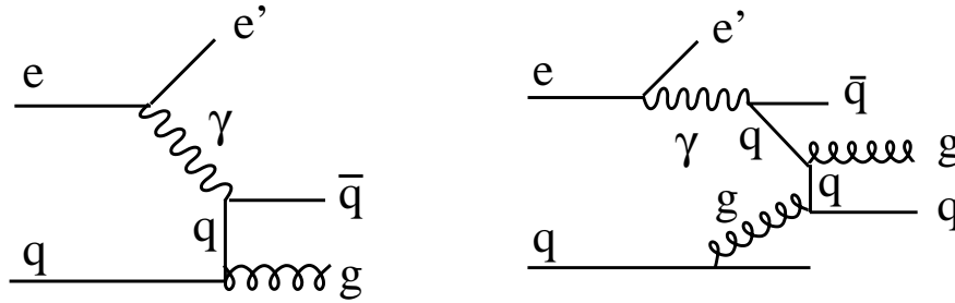
FIG. 3.18 – Processus de photoproduction : photoproduction directe (figure de gauche) et résolue (figure de droite)
