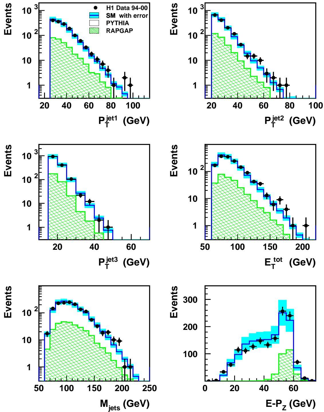
FIG. 5.11 – Distribution de l'impulsion transverse de chacun des trois jets, de l'énergie transverse totale, de la masse de tous les jets et enfin de E - P_z après la présélection du canal hadronique de recherche du top, pour l'ensemble des données e^{\pm}p de HERA-1 ( 118.3 \text{ pb}^{-1} )
