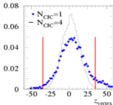
FIG. 4.8 – Coordonnée longitudinale du vertex reconstruit pour un échantillon de pseudo CC, pour un nombre de traces CJC égale à 1 (faible multiplicité) et à 4 (grande multiplicité).
