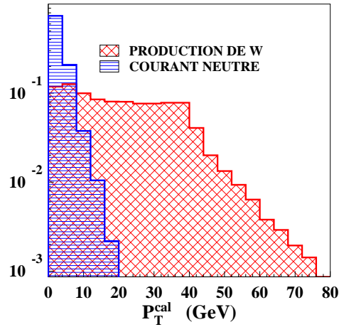
FIG. 4.3 – Distribution de l'impulsion transverse calorimétrique P_T^{cal} pour la production de W \rightarrow e\nu et le bruit de fond à courant neutre (échelle verticale arbitraire).
