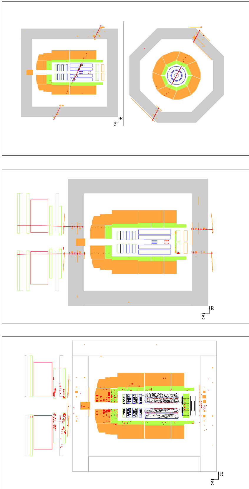
FIG. 3.20 – Exemples de rayonnement cosmique (figure du haut), de halo de muons (figure du milieu) et d'interaction faisceau-gaz (figure du bas).
