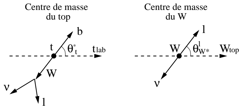
FIG. 5.4 – Désintégration du top dans son centre de masse (figure de gauche) et désintégration du W dans son centre de masse (figure de droite).
