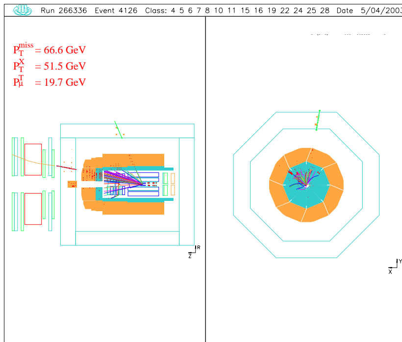
FIG. 4.14 – Candidat muon à P_T^X = 51.5 \text{ GeV} .
