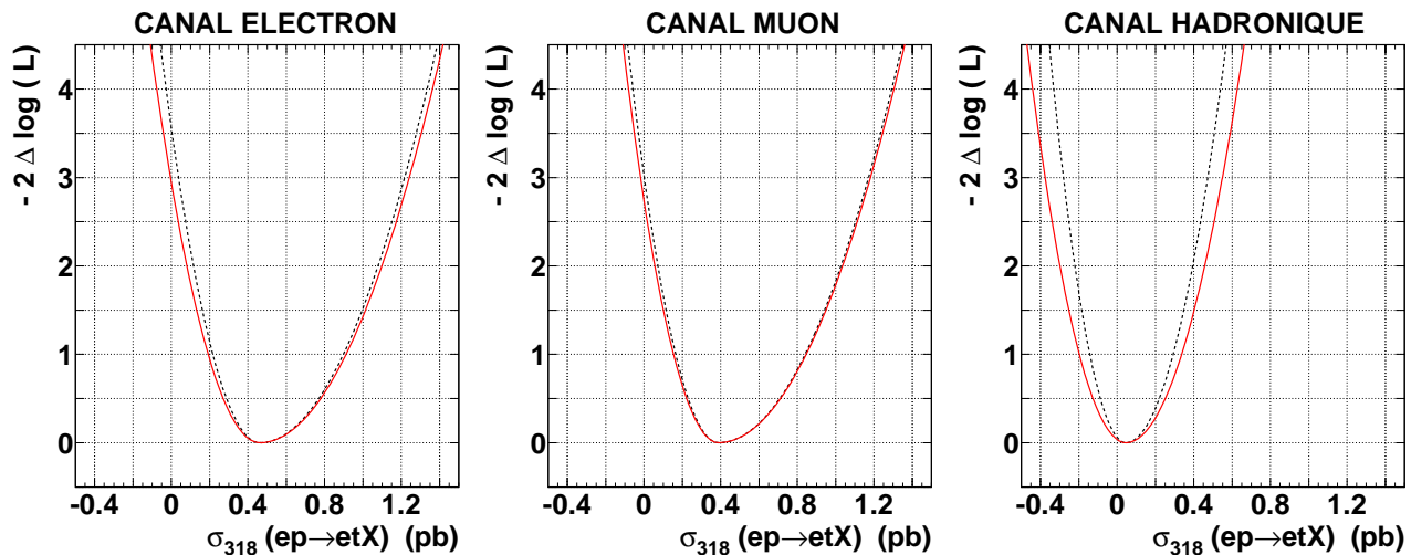
FIG. 5.17 – Ajustement -2\Delta \log \mathcal{L} en fonction de la section efficace de production du top, pour les canaux électron, muon et hadron. La courbe continue représente la fonction exacte -2\Delta \log \mathcal{L} sans erreurs systématiques, et la courbe en pointillés représente son approximation à deux paraboles, tenant compte des erreurs systématiques.
