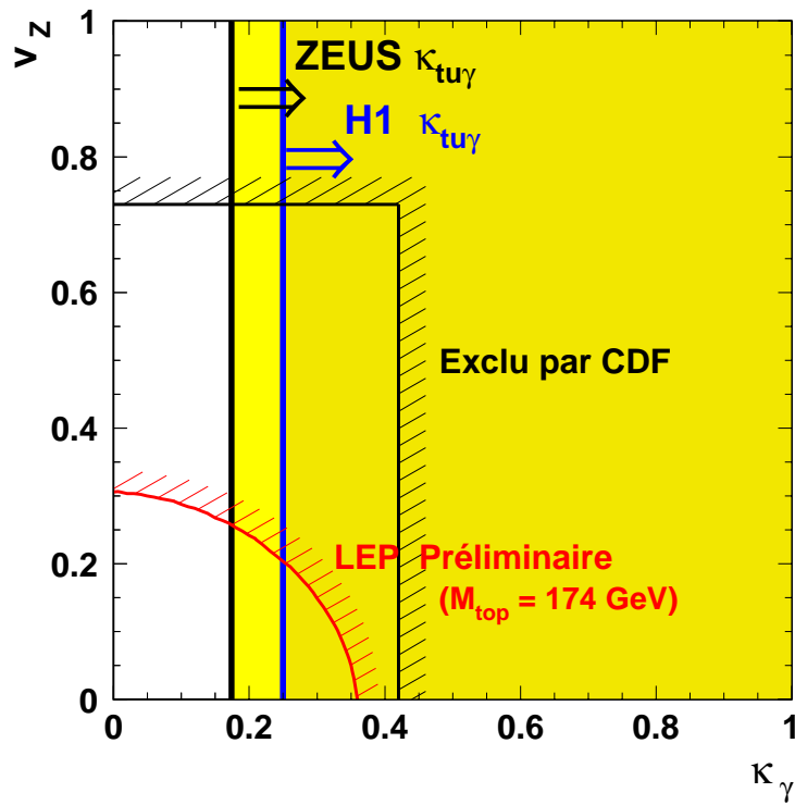
FIG. 5.21 – Limites d'exclusion sur les couplages \kappa_\gamma et v_Z auprès des accélérateurs HERA (expériences H1 et ZEUS), Tevatron (expérience CDF) et LEP. La constante v_Z est le couplage vecteur entre le quark top, un boson Z et un quark léger. La constante \kappa_\gamma est le couplage magnétique entre le quark top, un photon \gamma et un quark léger.
