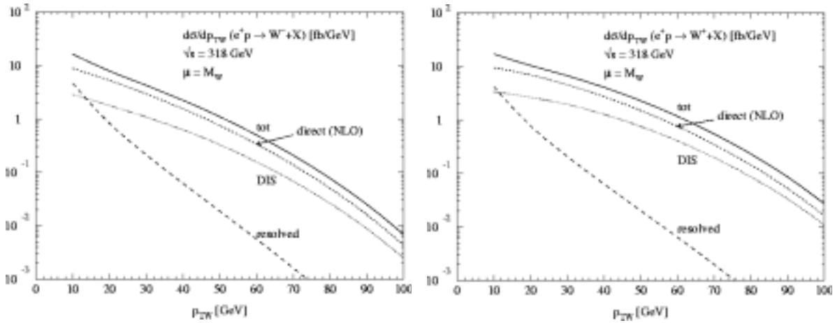
FIG. 3.9 – Sections efficaces différentielles d\sigma/dP_{TW} pour les processus direct, DIS et résolu dans le cas d'une production de W^- (à gauche) et de W^+ (à droite) pour une énergie dans le centre de masse de 318 GeV.
