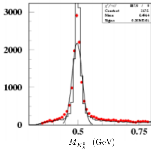
FIG. 4.24 – Distribution en masse de l'échantillon de mésons K_S^0 déterminée sur l'ensemble des données de HERA-1 (points) et comparée à la prédiction du Monte-Carlo courant neutre RAPGAP (histogramme) (échelle verticale arbitraire).
