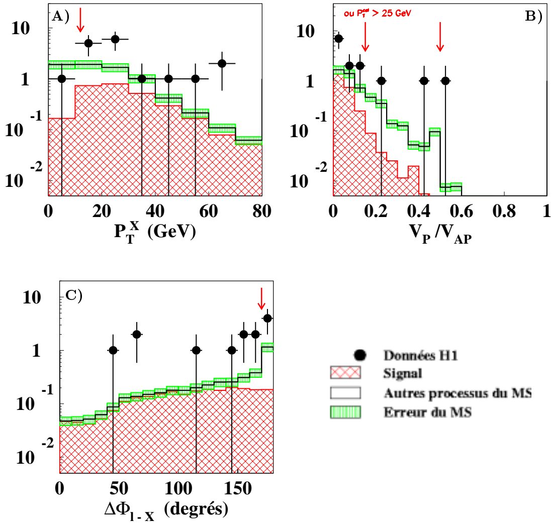
FIG. 4.11 – Distributions dans le canal muon à différentes étapes de sélection : impulsion transverse P_T^X du système hadronique avant l'étape A, balance azimutale V_p/V_{ap} après l'étape B, acoplanarité \Delta\Phi_{\ell-X} après l'étape C. Les flèches verticales indiquent les valeurs des coupures de sélection sur chaque variable (données e^+p , 104.7 \text{ pb}^{-1} ).
