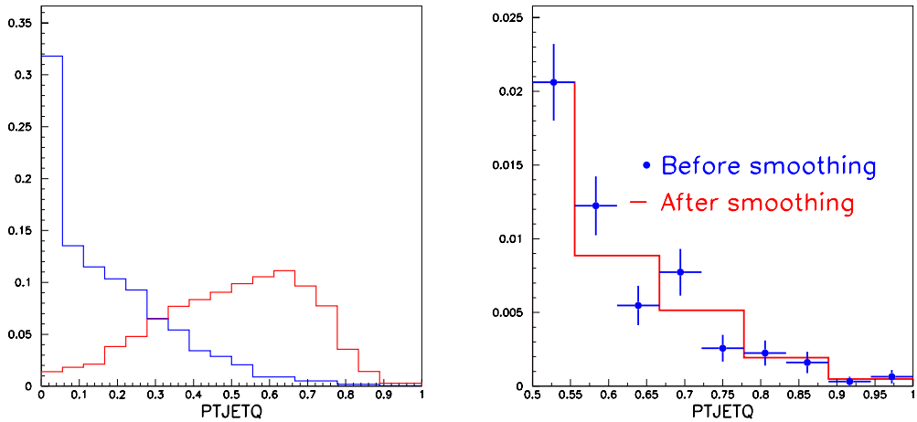
FIG. B.10 – Effet de l'association de deux intervalles de plus de 15% d'erreur sur les distributions de la variable d'entrée et de la vraisemblance résultante.
