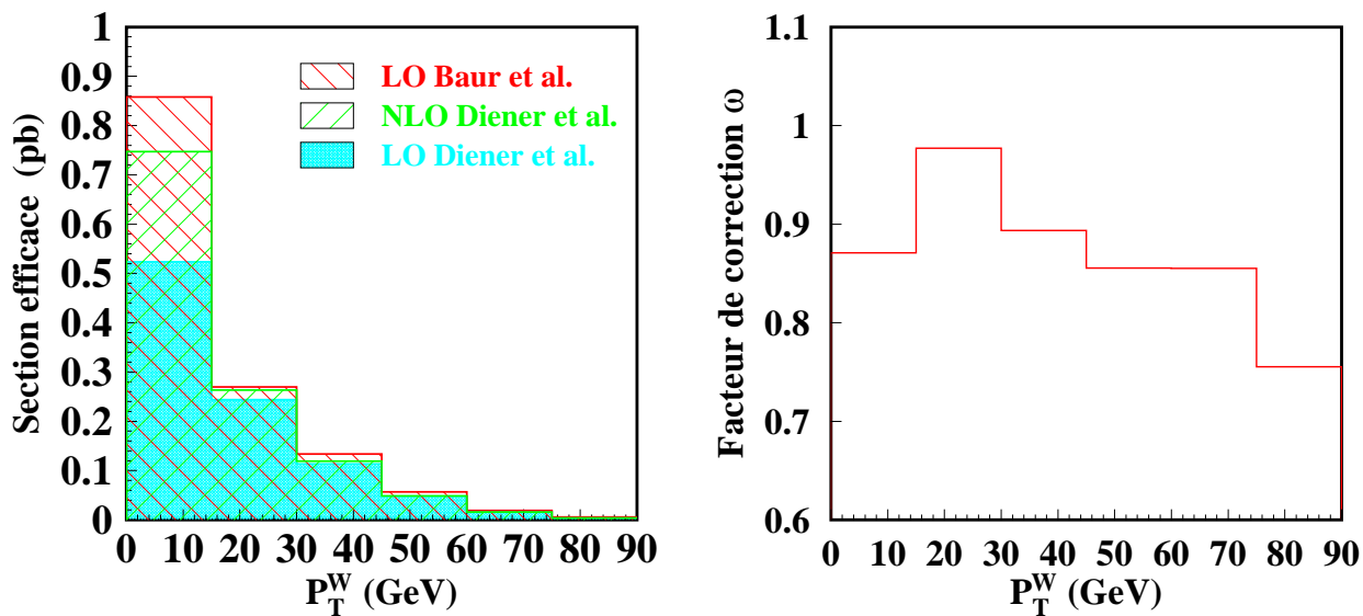
FIG. 3.10 – Figure de gauche : sections efficaces en fonction de l'impulsion transverse P_T^W du boson W pour les calculs LO selon Baur et al. et selon Diener et al. , et le calcul NLO de Diener et al. Figure de droite : facteur \omega de correction NLO appliqué sur le générateur EPVEC en fonction de l'impulsion transverse P_T^W du boson W. Ces résultats sont obtenus pour une énergie dans le centre de masse de 318 GeV.
