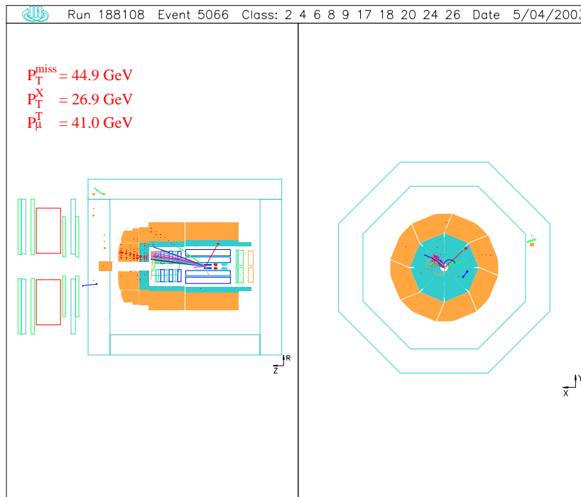
FIG. 4.15 – Candidat muon avec détection de l'électron diffusé.
