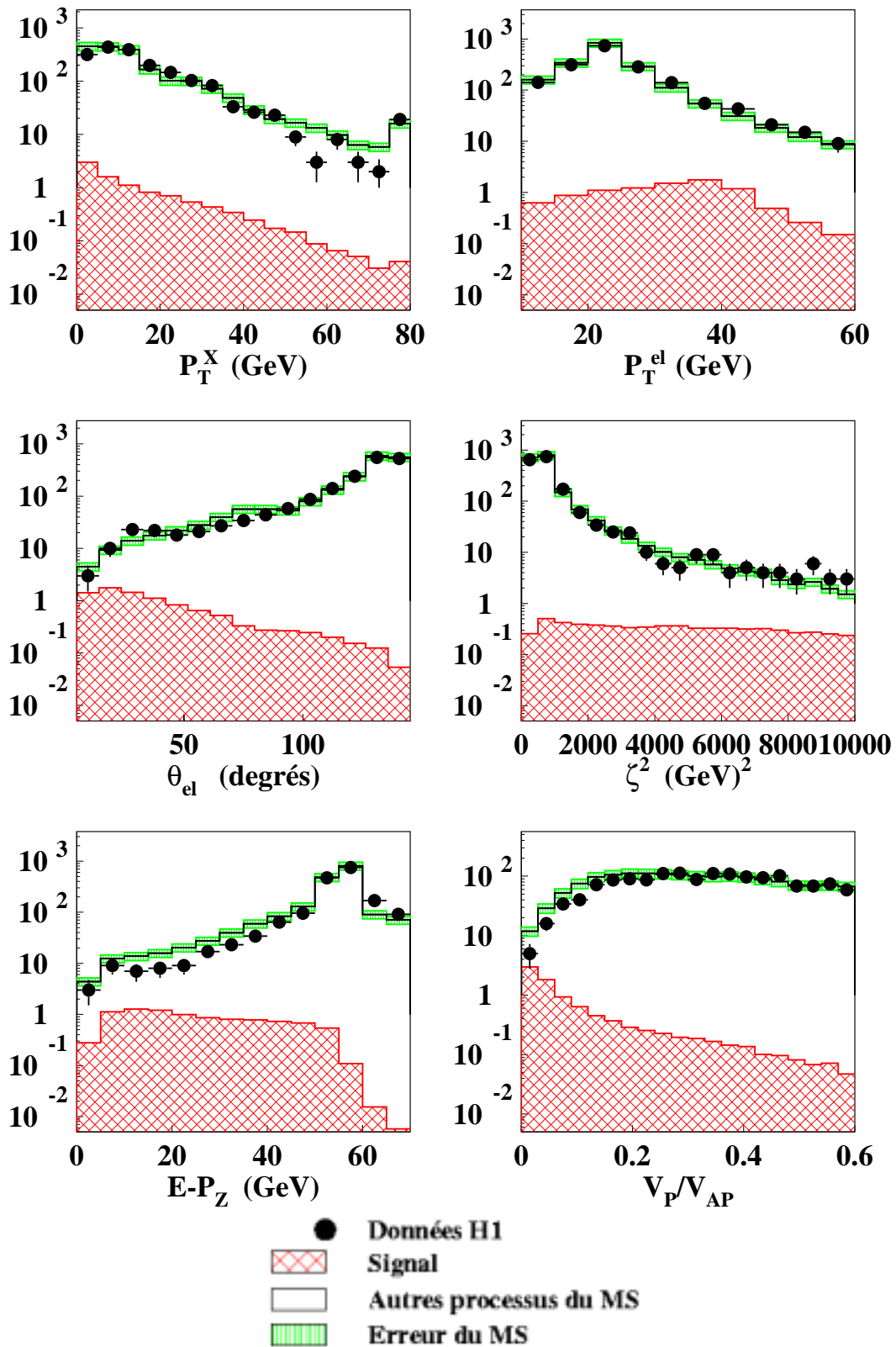
FIG. 4.17 – Distributions de contrôle dans le canal électron pour l'échantillon enrichi en courants neutres (données e^+p , 104.7 \text{ pb}^{-1} ). Le dernier intervalle de la distribution en P_T^X contient tous les événements dont la valeur de P_T^X est au-dessus de la limite supérieure de l'histogramme.
