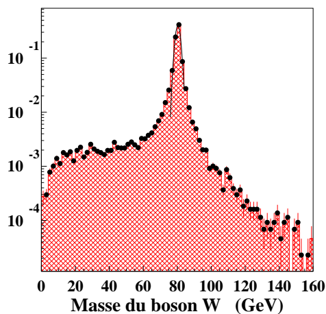
FIG. 3.3 – Masse du boson W, simulée par le générateur EPVEC pour le processus e^\pm p \rightarrow eW^\pm + X (échelle verticale arbitraire).
