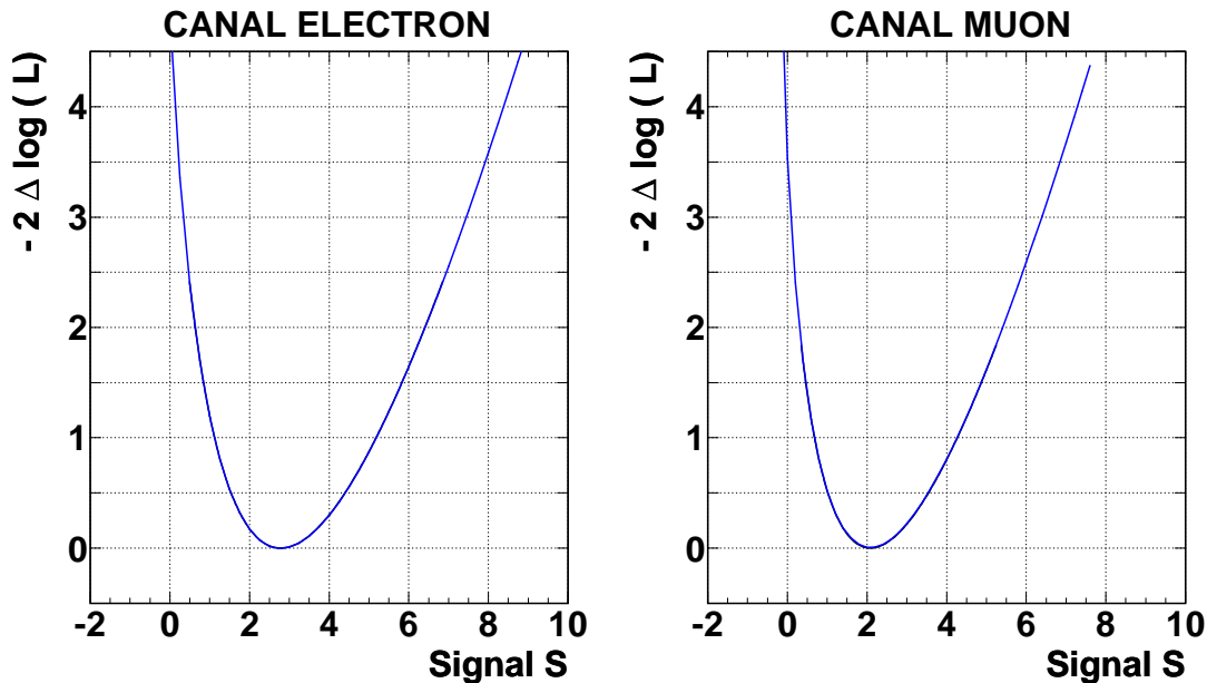
FIG. 5.14 – Ajustement -2\Delta \log \mathcal{L} en fonction de la normalisation du signal S , pour les canaux électron (figure de gauche) et muon (figure de droite).
