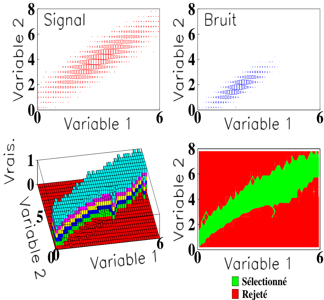
FIG. B.11 – Distribution bi-dimensionnelle des variables d'entrée de la fonction de vraisemblance pour le signal et pour le bruit (figures du haut) ; vraisemblance en fonction des variables d'entrée (figure du bas à gauche) ; vraisemblance coupée à 0.8 sur la vraisemblance en fonction des variables d'entrée (figure du bas à droite).
