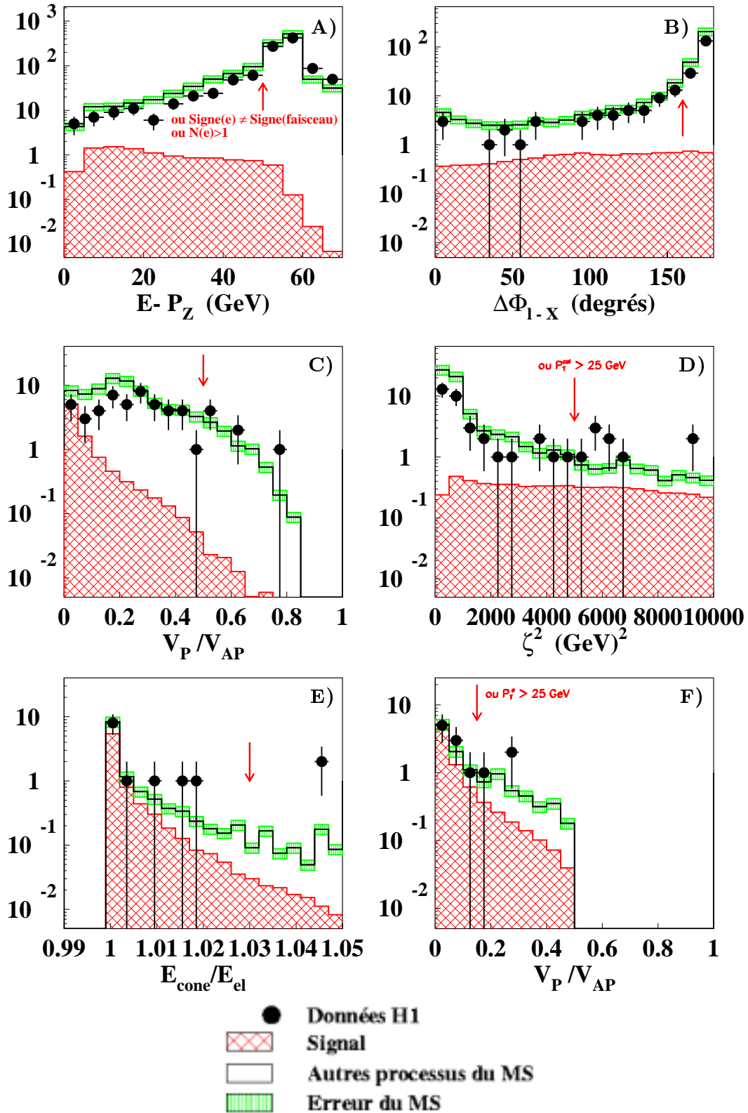
FIG. 4.10 – Distributions dans le canal électron à différentes étapes de sélection : E - P_z avant l'étape A, acoplanarité \Delta\Phi_{\ell-X} avant l'étape B, balance azimutale V_p/V_{ap} avant l'étape C, \zeta^2 avant l'étape D, E_{\text{cône}}/E_e avant l'étape E et balance azimutale V_p/V_{ap} avant l'étape F. Les flèches verticales indiquent les valeurs des coupures de sélection sur chaque variable (données e^+p , 104.7 \text{ pb}^{-1} ).
