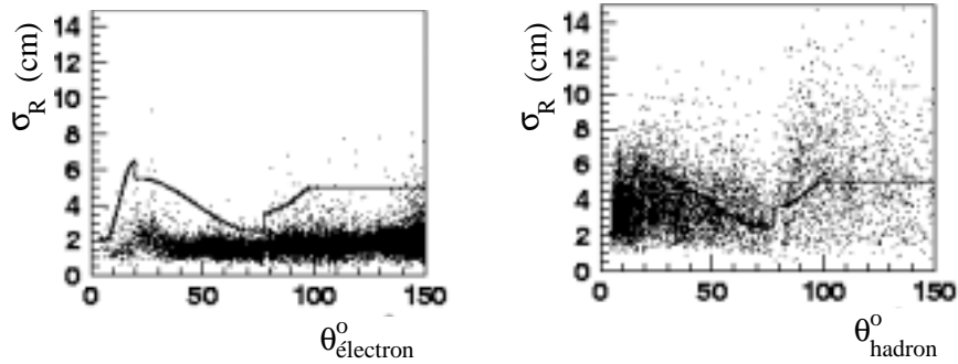
FIG. 2.12 – Spectre du rayon transverse \sigma_R en fonction de l'angle polaire de l'amas, pour des amas d'électrons (figure de gauche) et des amas de hadrons (figure de droite). La courbe continue représente la coupure \sigma_R^{max} en-dessous de laquelle les amas sont sélectionnés.
