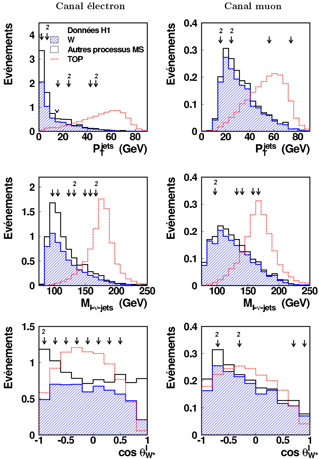
FIG. 5.6 – Pour chacun des deux canaux, distributions de la somme de l'impulsion transverse des jets P_T^{\text{jets}} , de la masse du système lepton-neutrino-jet M_{l-\nu\text{-jets}} et du cosinus de l'angle de désintégration du W dans son centre de masse \cos \theta_{W^*}^l pour la production de top (histogrammes pointillés), le Modèle Standard (histogrammes pleins) et les données expérimentales (flèches; les chiffres au-dessus des flèches indiquent le nombre d'événements de données dans l'intervalle concerné). Ces distributions sont effectuées après la présélection top, pour l'ensemble des données de HERA-1 ( 118.3 \text{ pb}^{-1} ).
