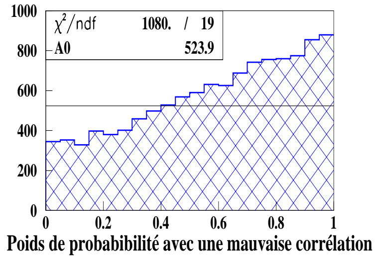
FIG. B.4 – Distribution du poids de probabilité des fonctions tests simulant le signal avec une bonne reconstruction de la corrélation (0.9) entre les variables d'entrée (figure du haut) et une mauvaise reconstruction de cette corrélation artificiellement posée à 0.7 (figure du bas).
