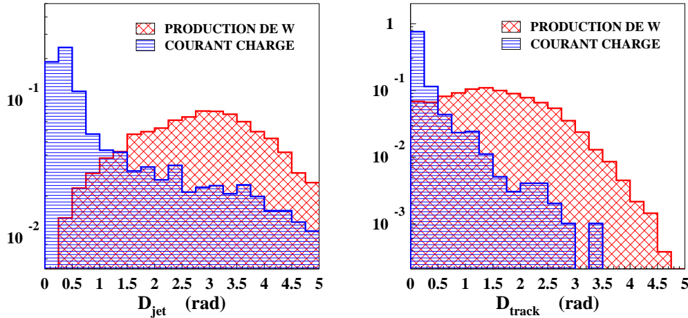
FIG. 4.1 – Distribution de la distance D_{jet} entre l'électron et le jet (figure de gauche) et de la distance D_{track} entre l'électron et la trace la plus proche (figure de droite) pour la production de W et les processus à courant chargé (échelle verticale arbitraire).
