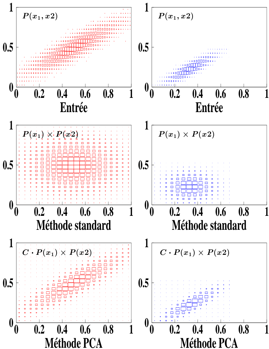
FIG. B.2 – Corrélation entre les deux variables d'entrée pour le signal (figures de gauche) et le bruit (figures de droite). Les deux figures du haut représentent la corrélation réelle entre les deux variables, celles du milieu la corrélation avec la méthode standard, et enfin celles du bas la corrélation reconstruite avec la méthode PCA.
