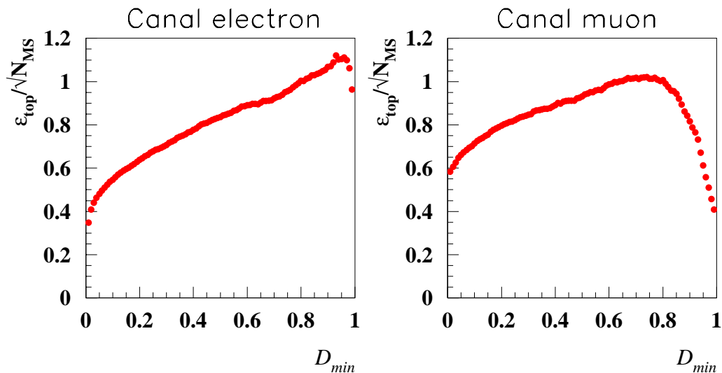
FIG. 5.9 – Rapport entre l’efficacité du signal top et la racine carrée du nombre de bruit de fond attendu \varepsilon_{top}/\sqrt{N_{MS}} en fonction de la coupure \mathcal{D}_{min} sur la fonction de vraisemblance, pour le canal électron et le canal muon.
