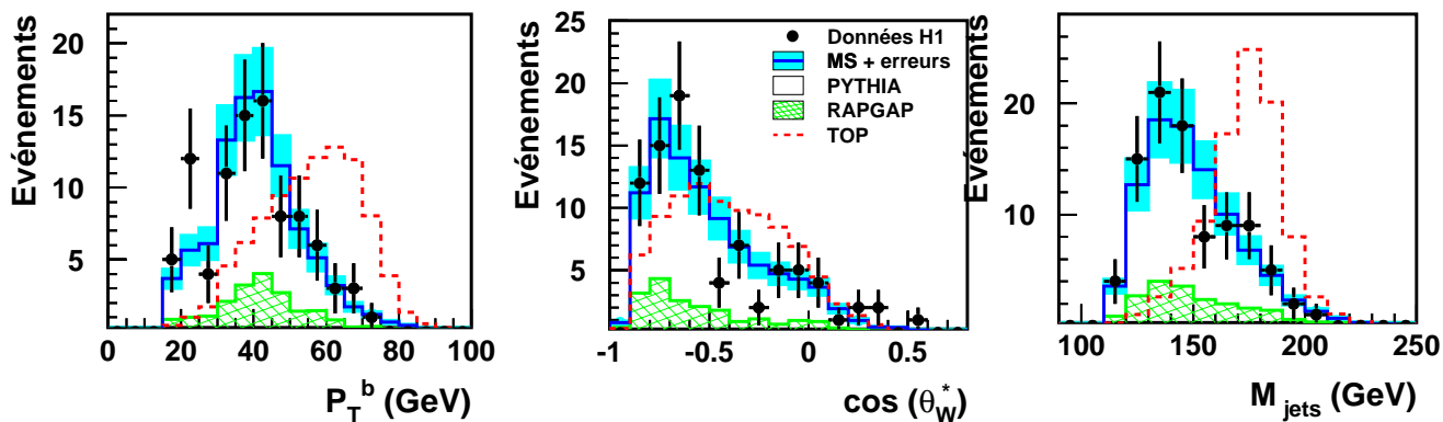
FIG. 5.12 – Distributions de l'impulsion transverse du candidat b , du cosinus de l'angle \theta_W^* de désintégration du W et de la masse invariante après la sélection 3-jets pour l'ensemble des données e^\pm p de HERA-1 ( 118.3 \text{ pb}^{-1} ). La normalisation du Monte-Carlo de production de top en pointillés est arbitraire.
