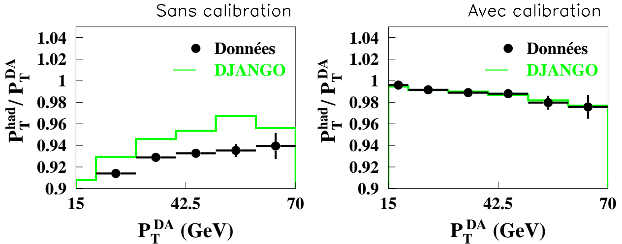
FIG. 2.15 – Valeur centrale de la distribution de P_T^{had}/P_T^{DA} en fonction de l'impulsion transverse calculée par la méthode double angle P_T^{DA} pour les données 1996-1997 et le Monte-Carlo courant neutre DJANGO sur un lot de courants neutres. Figure de gauche : calorimètre non calibré ; figure de droite : calorimètre calibré.
