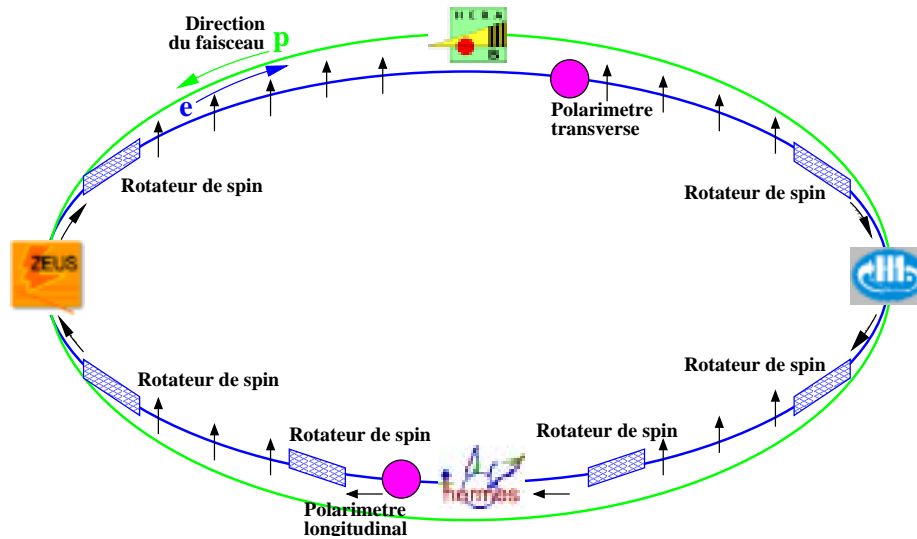
FIG. 2.3 – Polarisation du faisceau d'électrons de HERA à l'aide de rotateurs de spin.
