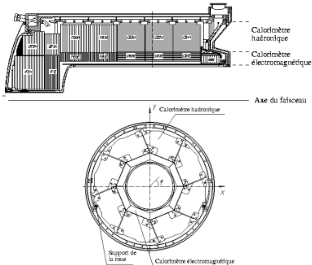
FIG. 2.10 – Coupes longitudinale (figure du haut) et transverse (figure du bas) du calorimètre à argon liquide de H1.
