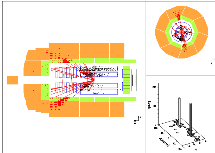
FIG. 3.19 – Exemple d'événement de photoproduction (extrait des données 1994 e^+p ).
