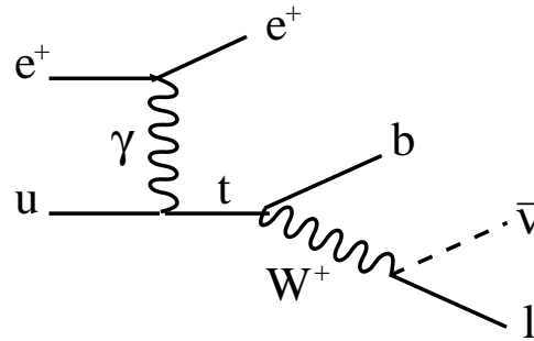
FIG. 5.2 – Production du quark top par FCNC suivie de sa désintégration en quark b et boson W (le W se désintégrant ensuite dans son canal leptonique).
