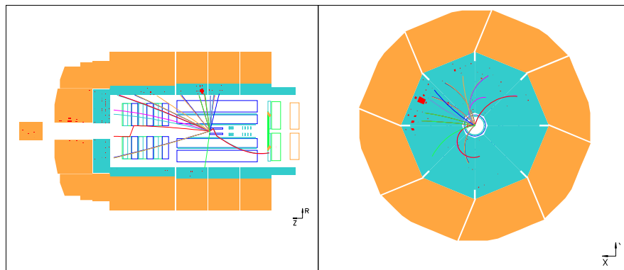
FIG. 3.15 – Exemple d'événement à courant chargé (Monte-Carlo DJANGO) extrait d'une sélection de jets étroits ( <0.1 rad) de grande fraction électromagnétique d'énergie ( >0.9 ) dans le calorimètre. Un dépôt compact et électromagnétique est présent dans l'événement, il est néanmoins entouré d'autres dépôts calorimétriques et donc non-isolé.
