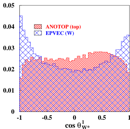
FIG. 5.5 – Angle de désintégration du W dans son centre de masse au niveau générateur pour les Monte-Carlo ANOTOP et EPVEC (échelle verticale arbitraire).
