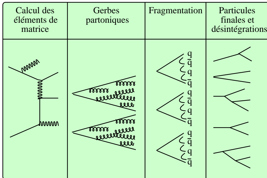
FIG. 2.23 – Les différentes étapes de génération d'un événement Monte-Carlo.
