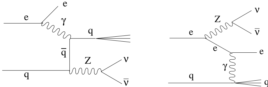
FIG. 3.11 – Diagrammes de production du boson Z dans les collisions ep avec désintégration en deux neutrinos.
