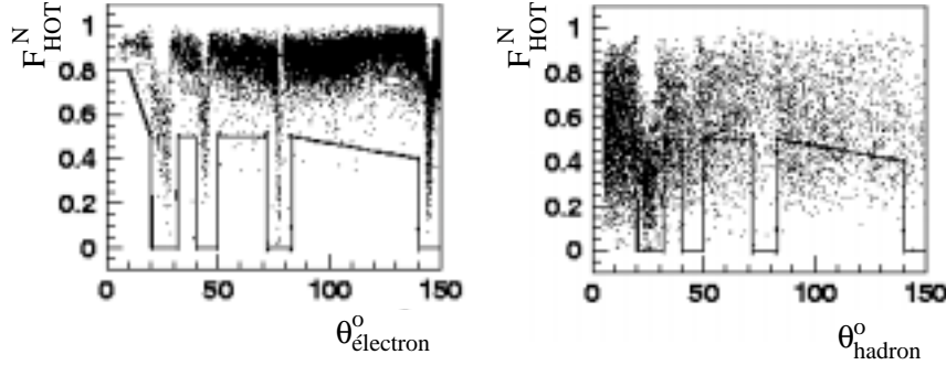
FIG. 2.13 – Spectre de la fraction d'énergie F_{HOT}^N contenue dans le cœur chaud en fonction de l'angle polaire de l'amas, pour des amas d'électrons (figure de gauche) et des amas de hadrons (figure de droite). La courbe continue représente la coupure F_{HOT}^{N,min} au-dessus de laquelle les amas sont sélectionnés.
