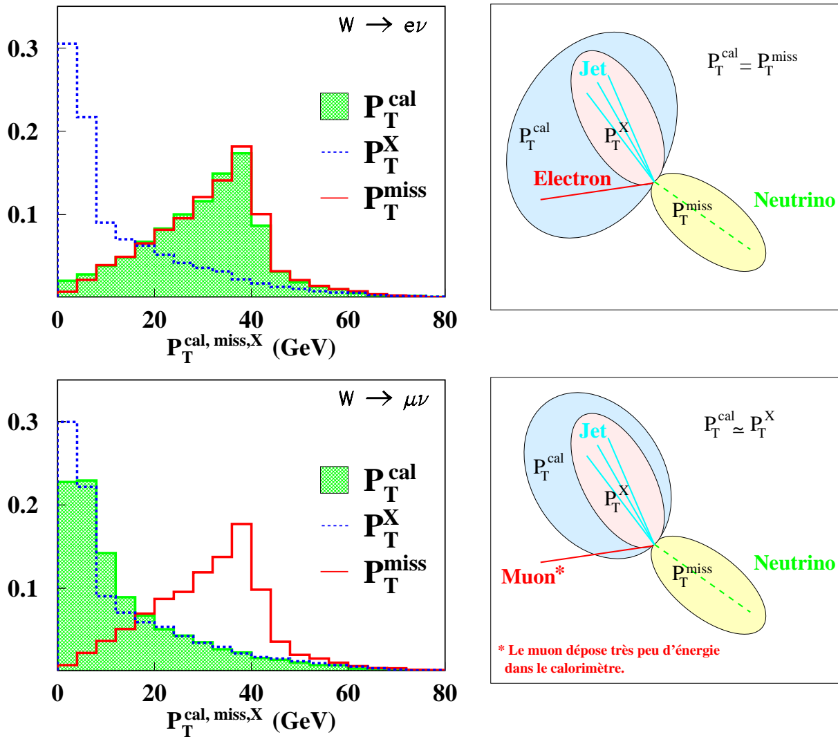
FIG. 4.4 – Figures de gauche : distributions des impulsions transverses P_T^{\text{cal}} , P_T^X et P_T^{\text{miss}} pour la prédiction de production de W pour les canaux électron ( W \rightarrow e\nu ) et muon ( W \rightarrow \mu\nu ) (échelle verticale arbitraire). Figure de droite : Vue transverse des objets considérés dans le calcul de chacune de ces variables, pour chacun des deux canaux (ces figures supposent que l'électron diffusé n'est pas détecté).
