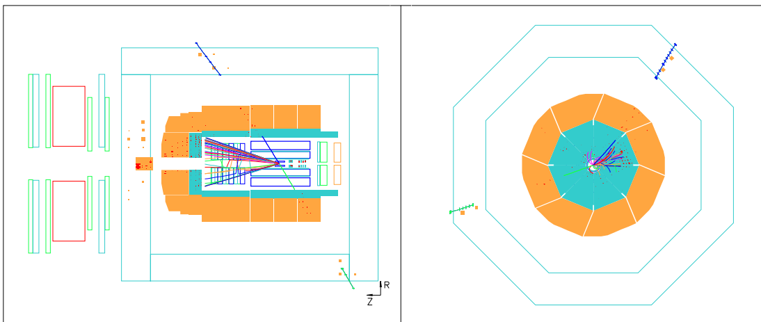
FIG. 3.17 – Exemple de production de paire de muons (extrait des données 2000 e^+p ).
