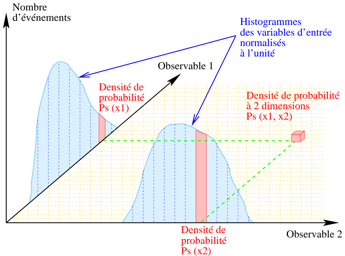
FIG. 5.7 – Schéma des densités de probabilités propres à chaque variable, P_S(x_1) = \int_{x_2} P_S(x_1, x_2) et P_S(x_2) = \int_{x_1} P_S(x_1, x_2) dans le cas où l'estimateur est construit à partir de deux variables discriminantes, et densité de probabilité à 2 dimensions correspondante P_S(x_1, x_2) .
