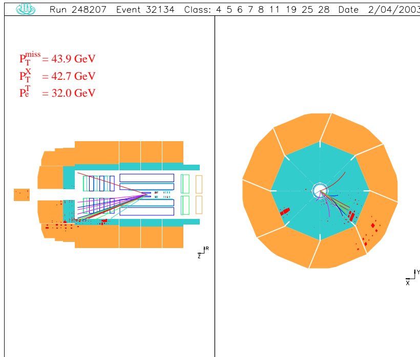
FIG. 4.13 – Candidat électron à P_T^X = 42.7 \text{ GeV} .
