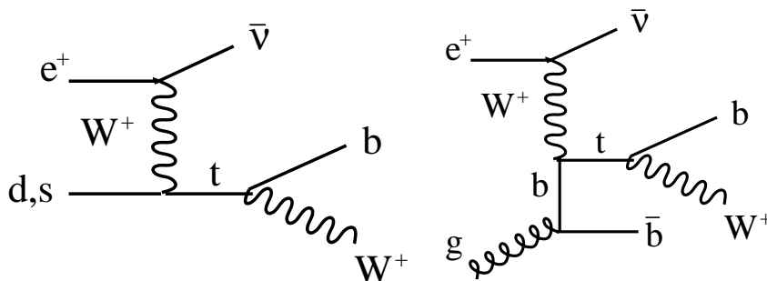
FIG. 5.1 – Production du quark top par courant chargé dans le cadre du Modèle Standard, à travers l'interaction d'un quark d ou s (figure de gauche) ou d'un quark b (figure de droite), suivie de sa désintégration en quark b et boson W .
