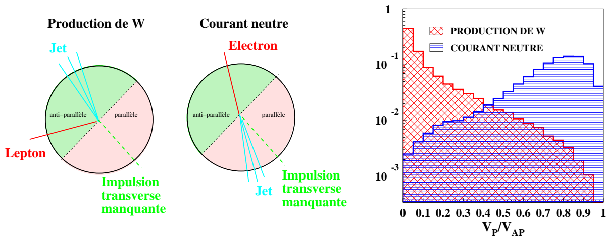
FIG. 4.6 – Figure de gauche: dans le plan transverse, topologie d'un événement de production de W (cercle de gauche), et topologie d'un événement à courant neutre (cercle de droite). Figure de droite: distribution de la balance azimutale V_p/V_{ap} pour la production de W \rightarrow e\nu et le bruit de fond à courant neutre (échelle verticale arbitraire).
