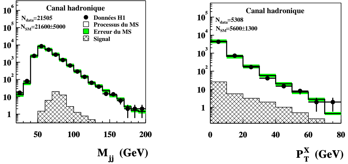
FIG. 4.26 – Distribution de la masse invariante des deux jets formant le candidat W (après toutes les coupures exceptée celle sur M_{jj} ). et distribution de l'impulsion transverse du système hadronique de recul, après toutes les coupures (données e^\pm p , 118.3 \text{ pb}^{-1} ).
