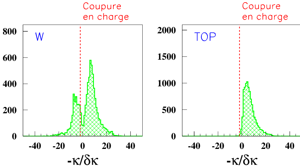
FIG. 5.3 – Distribution de -\kappa/\delta\kappa pour les Monte-Carlo de production de W (à gauche) et de top (à droite). La ligne en pointillés désigne la valeur de -\kappa/\delta\kappa à laquelle la coupure est effectuée ( -\kappa/\delta\kappa=-2 ).
