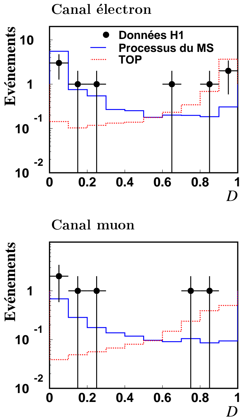
FIG. 5.8 – Distributions de la vraisemblance D du signal, du bruit de fond et des données dans le canal électron (figure du haut) et le canal muon (figure du bas), déterminées sur l'ensemble des données e^\pm p de HERA-1 ( 118.3 \text{ pb}^{-1} ).
