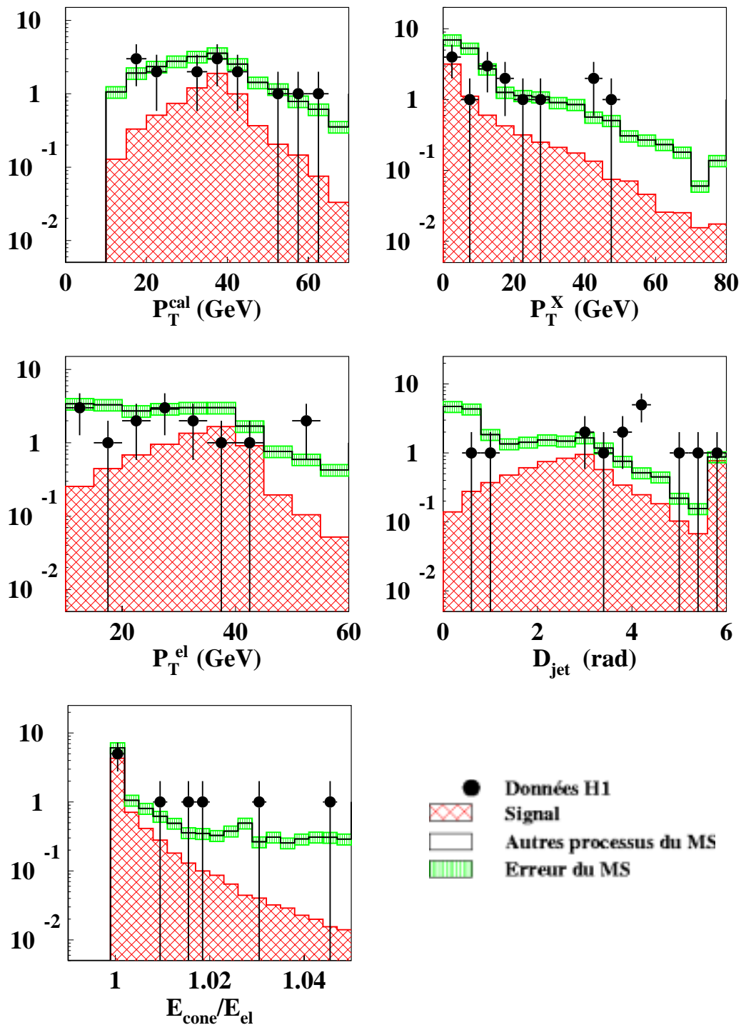
FIG. 4.18 – Distributions de contrôle dans le canal électron pour l'échantillon enrichi en courants chargés (données e^+p , 104.7 \text{ pb}^{-1} ). Le dernier intervalle de la distribution en P_T^X ( D_{jet} ) contient tous les événements dont la valeur de P_T^X ( D_{jet} ) est au-dessus de la limite supérieure de l'histogramme.
