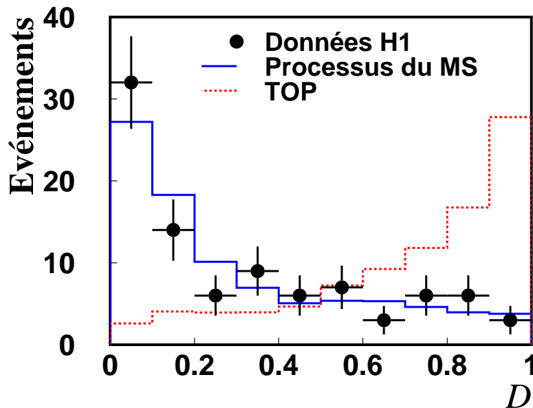
FIG. 5.13 – Distribution de la vraisemblance obtenue dans le canal hadronique, obtenue à partir des variables d'entrée P_T^{jets} , \cos\theta_W^* et M_{jets} , sur l'ensemble des données e^\pm p de HERA-1 ( 118.3 \text{ pb}^{-1} ).
