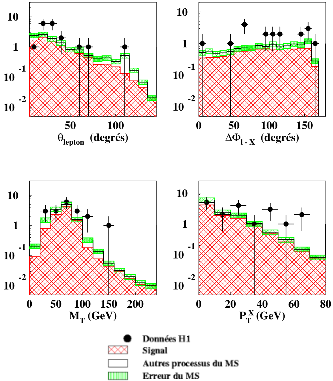
FIG. 4.12 – Distribution de l'angle polaire du lepton \theta_{\ell ep} , de l'acoplanarité \Delta\Phi_{\ell-X} , de la masse transverse M_T^{\ell\nu} du système lepton-neutrino et de l'impulsion transverse hadronique P_T^X pour les canaux électron et muon combinés (données e^+p , 104.7 \text{ pb}^{-1} ).
