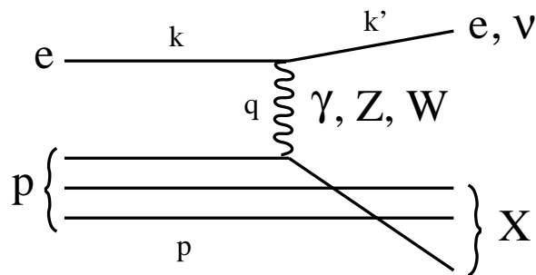
FIG. 1.3 – Diffusion profondément inélastique (DIS) à HERA. k, k', q et p sont respectivement les quadrivecteurs de l'électron incident, de l'électron diffusé, du boson échangé et du proton incident. X représente le système hadronique de l'état final de la réaction. Le processus ep \rightarrow eX est une interaction profondément inélastique à courant neutre, tandis que le processus ep \rightarrow \nu X est une interaction profondément inélastique à courant chargé.
