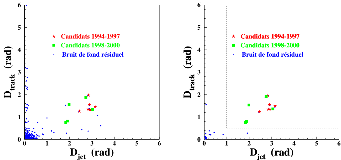
FIG. A.2 – Isolation D_{track} de la trace par rapport aux jets en fonction de son isolation D_{jet} par rapport aux autres traces de l'événement, pour les coupures générales avant l'identification des leptons (figure de gauche) et après identification des leptons (figure de droite). Du bruit résiduel persiste à faible isolation du lepton dans le canal électron.
