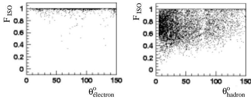
FIG. 2.14 – Spectre de l'isolation F_{ISO} en fonction de l'angle polaire de l'amas, pour des amas d'électrons (figure de gauche) et des amas de hadrons (figure de droite).
