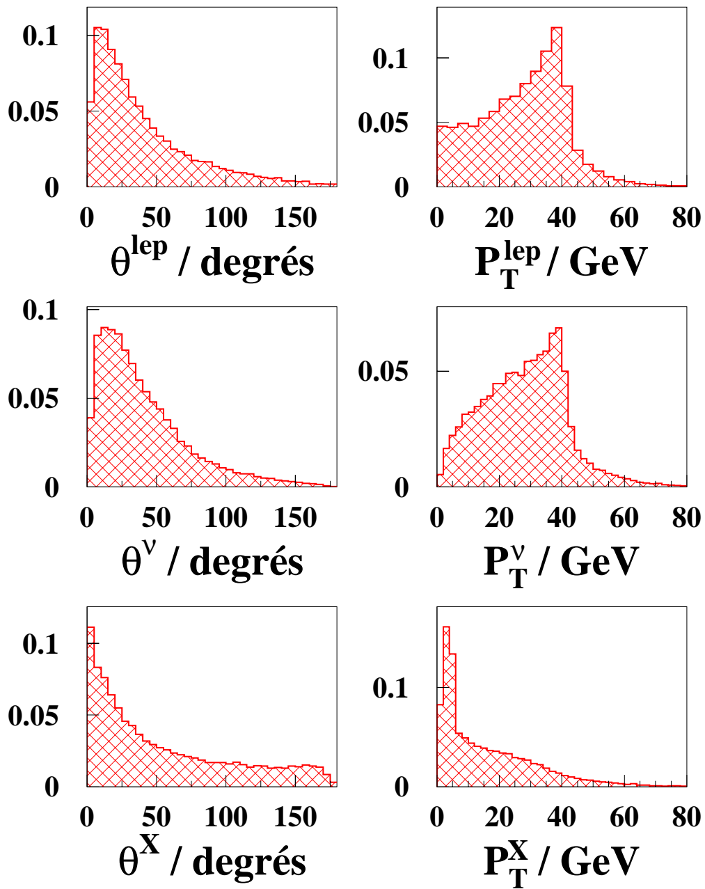
FIG. 3.4 – Distributions de l'angle polaire (colonne de gauche) et de l'impulsion transverse (colonne de droite) du lepton, du neutrino et du jet issu du boson W, simulés par le générateur EPVEC pour le processus e^{\pm}p \rightarrow eW^{\pm} + X (échelle verticale arbitraire).
