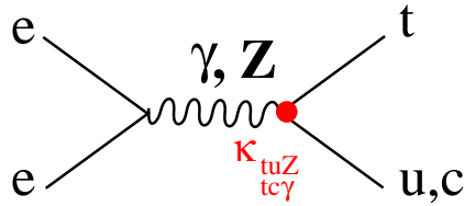
FIG. 5.19 – Diagramme de production de top par couplage anormal \kappa_{tuZ} ou \kappa_{tc\gamma} au LEP.
