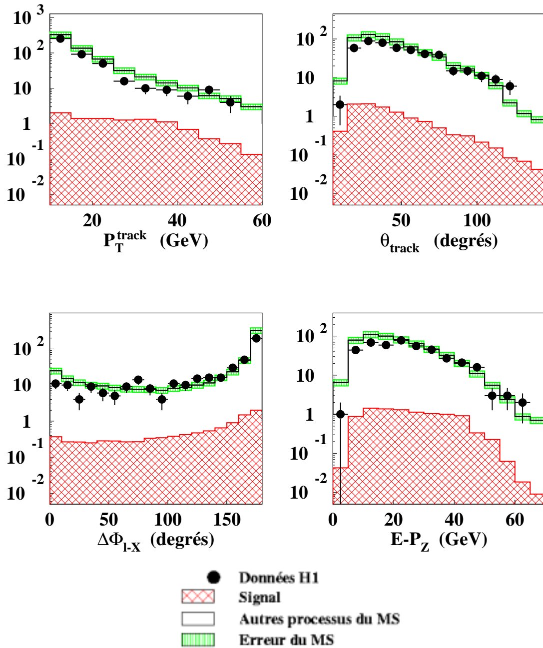
FIG. A.1 – Distributions de P_T^{\text{track}} , \theta_{\text{track}} , \Delta\Phi_{l-X} et E - P_z après la sélection générale de l'analyse publiée en 1998 (données e^+p 104.7 \text{ pb}^{-1} ).
