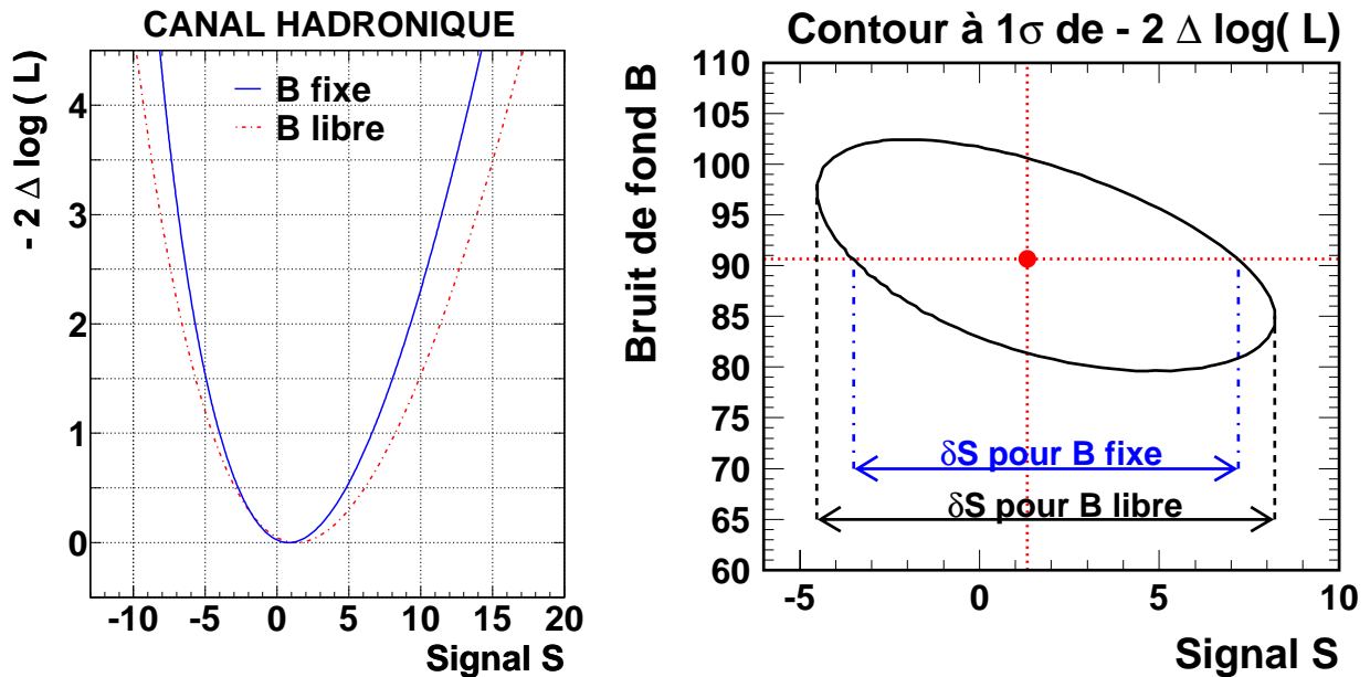
FIG. 5.15 – Ajustement -2\Delta\log\mathcal{L} en fonction de la normalisation du signal S , pour le canal hadronique, en conservant la normalisation au bruit B fixe et en variant B (figure de gauche). Contour bi-dimensionnel de la fonction -2\Delta\log\mathcal{L} à 1\sigma en fonction des normalisations au signal et au bruit S et B (figure de droite).
