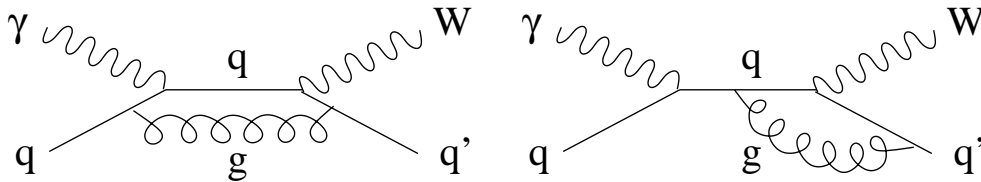
FIG. 3.7 – Diagrammes typiques de corrections virtuelles sur la production de W .
