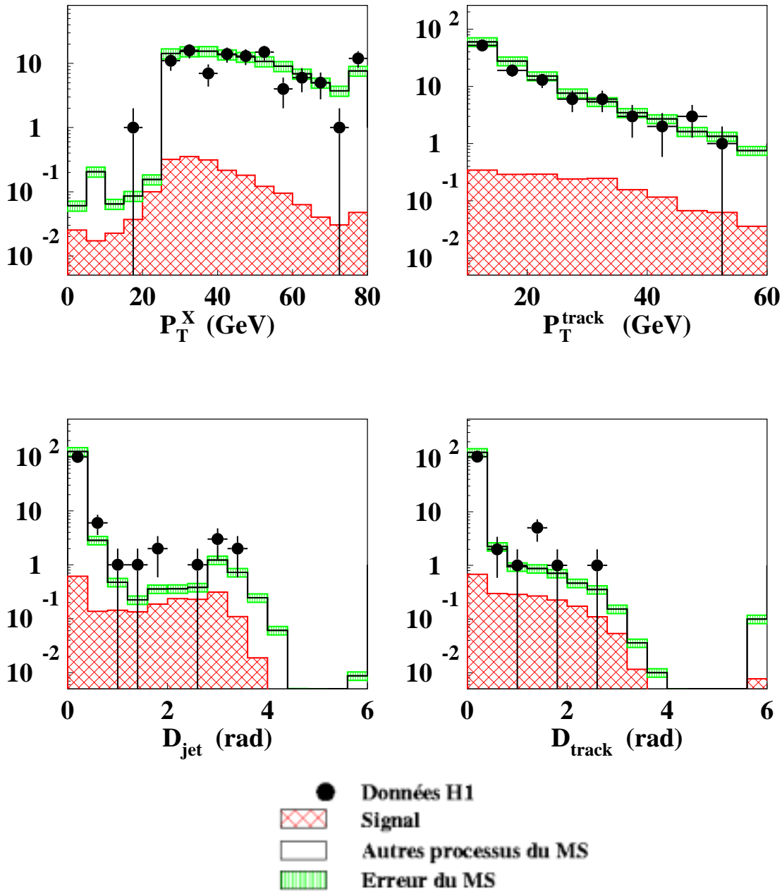
FIG. 4.22 – Distributions de l'impulsion transverse hadronique P_T^X , de l'impulsion transverse de la trace candidate P_T^{\text{track}} et de son isolation par rapport aux jets et aux traces, D_{\text{jet}} et D_{\text{track}} , pour l'échantillon de fuite de jets (données e^+p , 104.7 \text{ pb}^{-1} ). Le dernier intervalle des distributions en P_T^X , D_{\text{jet}} et D_{\text{track}} contient tous les événements dont les valeurs de P_T^X , D_{\text{jet}} et D_{\text{track}} est au-dessus de la limite supérieure de l'histogramme.
