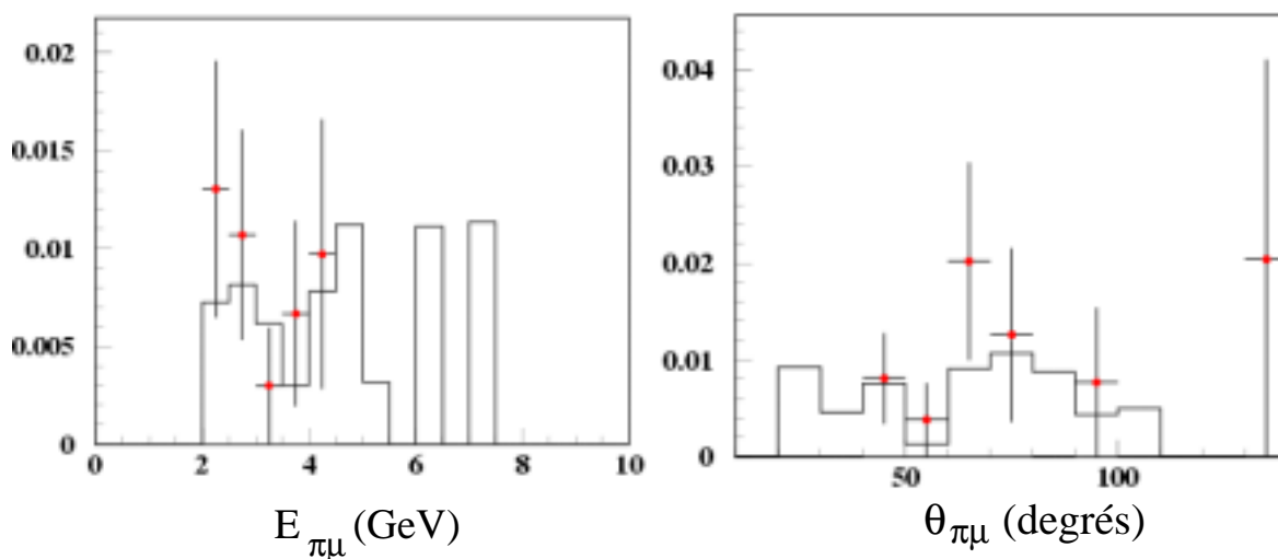
FIG. 4.25 – Taux de pions provenant de K_S^0 et ayant une signature muonique, en fonction de l'énergie et de l'angle polaire du candidat pion, déterminés sur l'ensemble des données de HERA-1 (points) et comparés à la prédiction du Monte-Carlo de courants neutres RAPGAP (histogramme).
