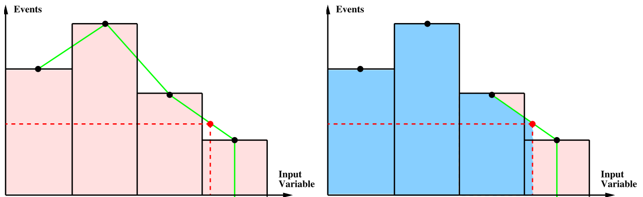
FIG. B.8 – Lissage de la hauteur des intervalles de la variable d'entrée (figure de gauche) et transformation des deux derniers intervalles de la variable d'entrée (figure de droite).
