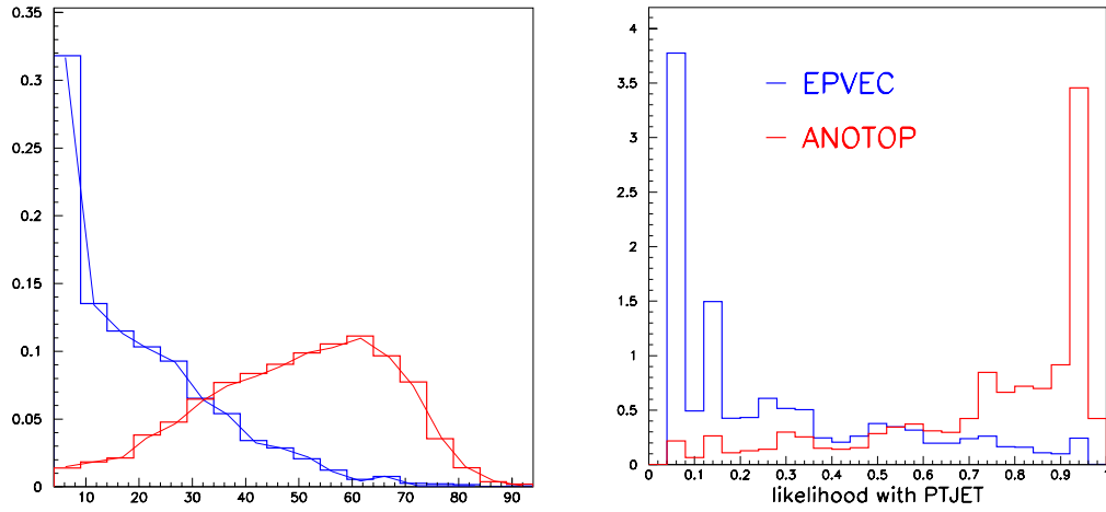
FIG. B.9 – Effet du lissage de la hauteur des intervalles sur les distributions de la variable d'entrée et de la vraisemblance résultante.
