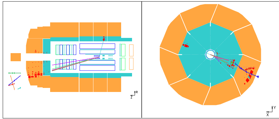
FIG. 3.13 – Exemple d'événement à courant neutre (Monte-Carlo RAPGAP) extrait d'une sélection d'événements de grande impulsion transverse manquante ( >25 GeV). Dans cet événement, une fluctuation dans la mesure du jet hadronique engendre de l'impulsion transverse manquante alors que l'électron et le jet sont dos-à-dos dans le plan transverse.
