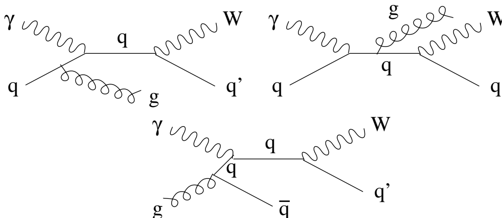
FIG. 3.8 – Diagrammes typiques de corrections réelles sur la production de W .
