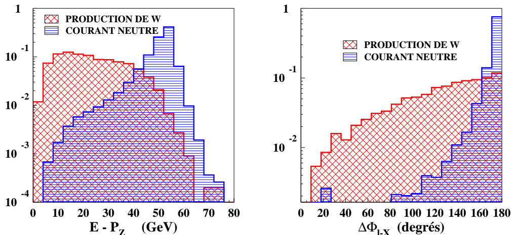
FIG. 4.5 – Distribution de E - P_z (figure de gauche) et de l'acoplanarité \Delta\Phi_{\ell-X} (figure de droite) pour la production de W \rightarrow e\nu et le bruit de fond à courant neutre (échelle verticale arbitraire).
