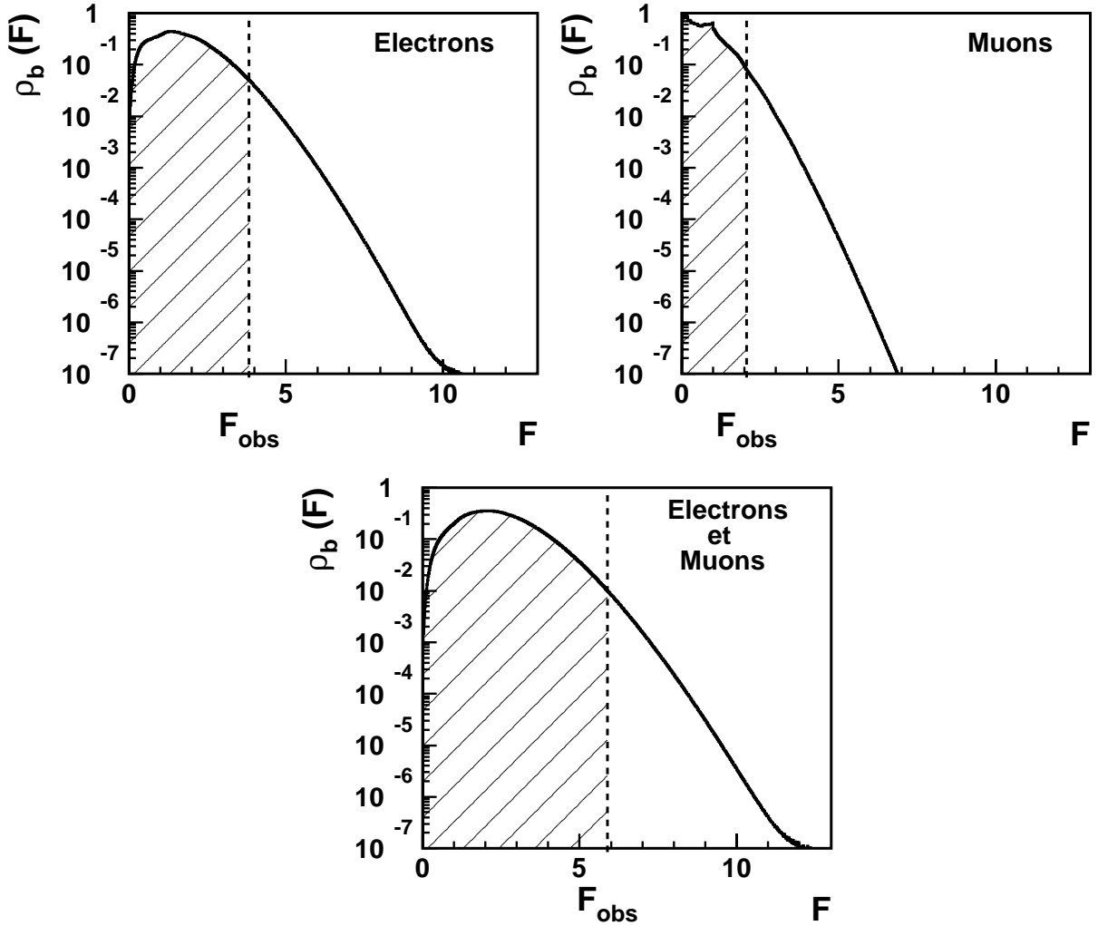
FIG. 5.10 – Densité de probabilité \rho_b(F) en fonction de l'estimateur F , calculé à partir de la distribution de l'estimateur \mathcal{D} , pour les canaux électron, muon et la combinaison des deux. F_{obs} est la valeur observée dans les données. La région hachurée à gauche de F_{obs} représente le niveau de confiance CL_b de l'hypothèse "bruit seulement".
