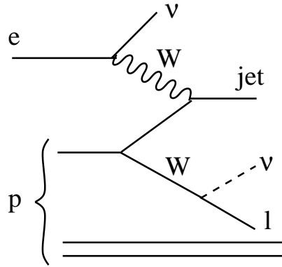
FIG. 3.5 – Production et désintégration du boson W dans les collisions ep pour le processus e^\pm p \rightarrow \nu W^\pm + X suivi de la désintégration W \rightarrow \ell\nu .
