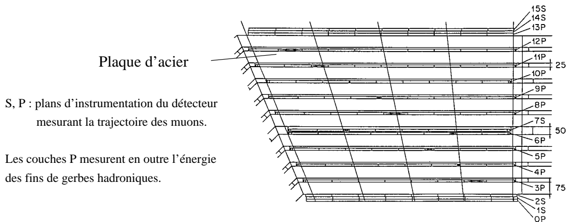
FIG. 2.18 – Vue schématique d'un octant du fer instrumenté de H1.
