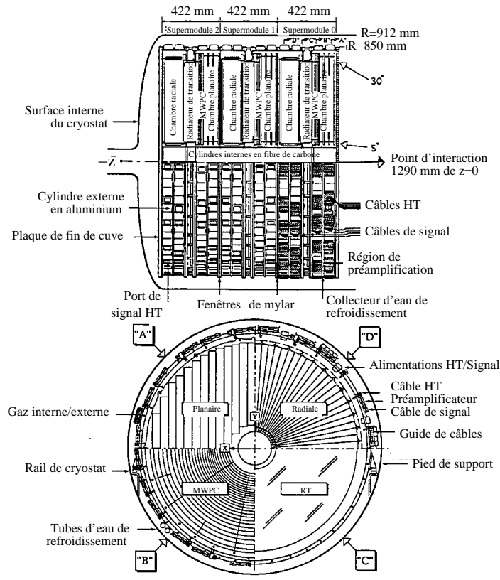
FIG. 2.8 – Schéma d'un détecteur de traces avant (FTD).
