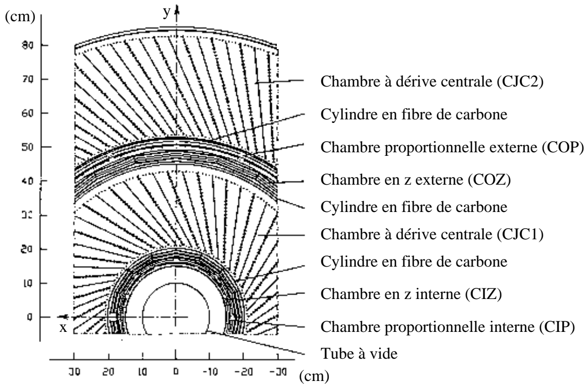
FIG. 2.5 – Vues longitudinale (figure du haut) et transverse (figure du bas) du système de trajectographie de H1. Il est constitué de plans successifs de chambres proportionnelles (CIP et COP), chambres en z (CIZ et COZ) et chambres à dérive (CJC1 et CJC2).
