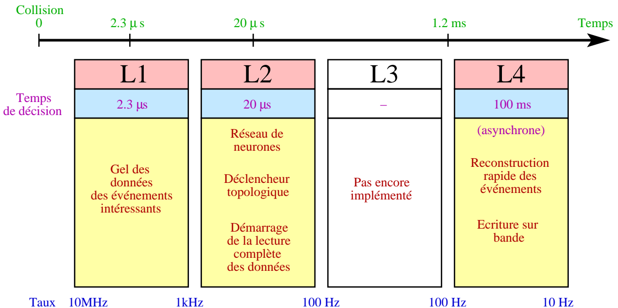
FIG. 2.21 – Schéma des quatre niveaux du système de déclenchement de H1. Le niveau L3 n'était pas encore implémenté lors de l'acquisition des données analysées dans cette thèse.
