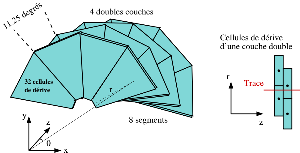
FIG. 2.9 – Schéma d'une chambre à dérive arrière (BDC). Le schéma de droite illustre la levée de l'ambiguïté de reconstruction des traces grâce au décalage des plans de fils.
