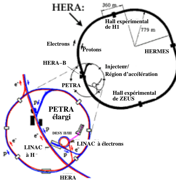
FIG. 2.1 – Schéma de l'accélérateur HERA. Les électrons sont progressivement accélérés depuis le LINAC à électrons, en passant par DESY II, PETRA, jusqu'à HERA. Les protons sont progressivement accélérés depuis le LINAC à protons, en passant par DESY III, PETRA, jusqu'à HERA.
