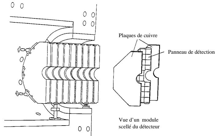
FIG. 2.17 – Bouchon calorimétrique de H1 (PLUG).
