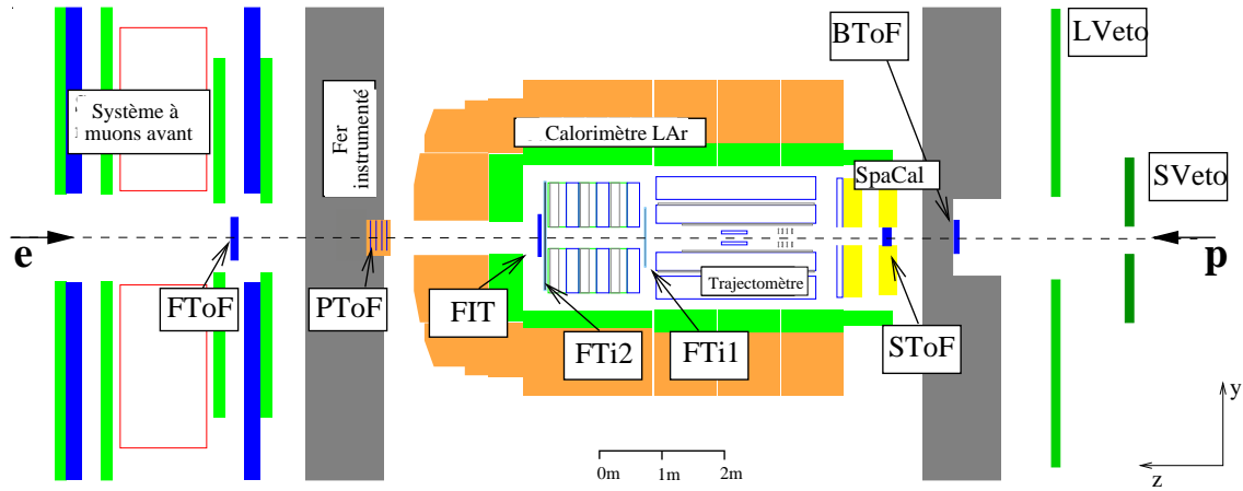
FIG. 2.20 – Position des détecteurs à temps de vol sur le détecteur H1.
