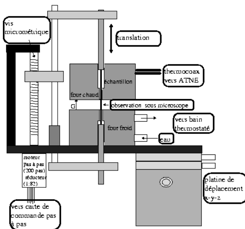
FIG. 2.6 – Four de croissance directionnelle.
