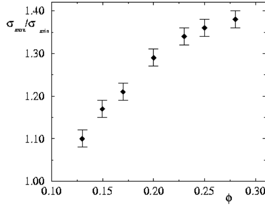
FIG. 5.9 – L'anisotropie de l'énergie interfaciale, définie par le rapport \sigma(0)/\sigma(\theta_0) , croît dans les régions concentrées .
