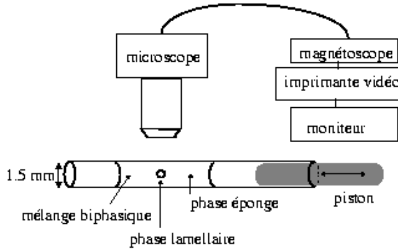
FIG. 9.3 – La déformation initiale est obtenue par un cisaillement initial causé par le déplacement d'un piston dans le capillaire.
