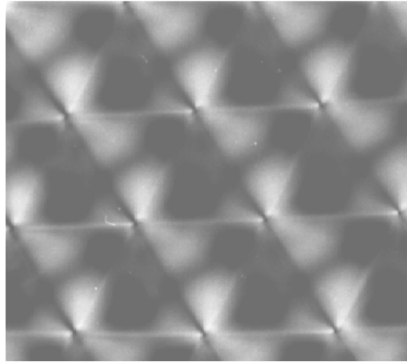
FIG. 7.26 – Aux grandes épaisseurs ( > 100\mu ), l'interface Sm-A-Air présente un treillis dont les sommets sont les hyperboles des défauts. On ne peut donc considérer que la géométrie des défauts en contact est celle des défauts isolés.
