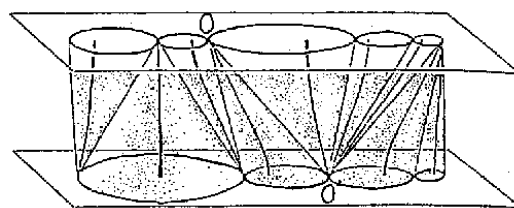
FIG. 1.11 – Assemblages de coniques focales, les cônes sont tangents le long des génératrices OO' (d'après BOULIGAND [26]).
