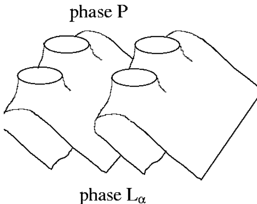
FIG. 11.1 – L'ajustement des distances caractéristiques d_\alpha et d_3 implique une déformation des membranes au voisinage de l'interface se traduisant par une énergie interfaciale dont l'ordre de grandeur est \sigma \approx \kappa/d_3^2 .
