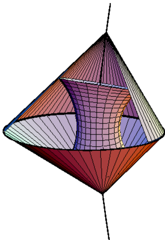
FIG. 1.10 – Les coniques focales complètes ne sont que rarement observées dans les Sm-A. Les coniques focales sont limitées, en effet à des domaines dont les frontières sont deux cônes reposant sur l'ellipse.
