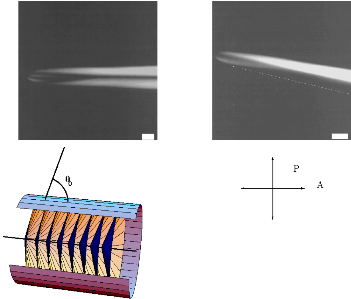
FIG. 4.4 – Bâtonnet dont les couches sont en forme de cône et dont la surface quasi-cylindrique est lisse. Barre 20 \mu m.
