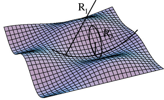
FIG. 1.3 – Les courbures principales c_1 et c_2 sont les inverses des rayons de courbures principaux R_1 et R_2 .
