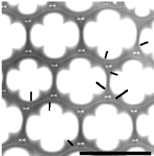
FIG. 7.21 – Ici, l'épaisseur est voisine de x_{c,2} et quelques disques interstitiels de 2 e génération sont présents (indiqués par les traits sombres). Épaisseur 905 \mu\text{m} (ce qui donne \omega_{1,exp} \approx 0,043 pour \omega_{1,theo} \approx 0,068 ). Barre 100 \mu\text{m} .
