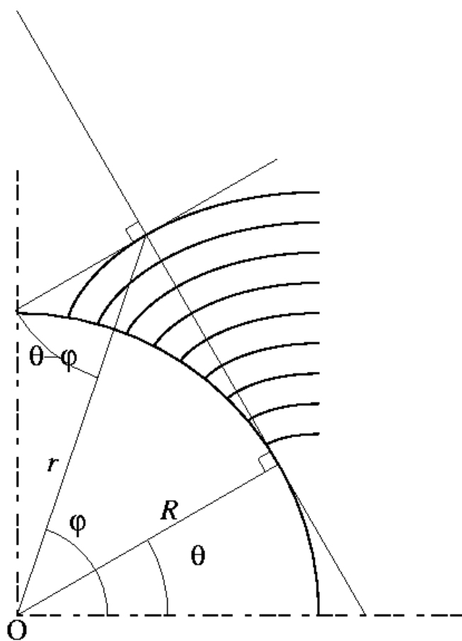
FIG. 6.21 – Dans l'approximation géométrique et dans la limite de l'ancrage planaire fort les sections des couches sont les développantes du cercle de rayon R .
