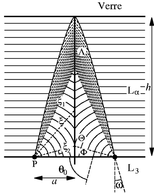
FIG. 6.16 – Texture satisfaisant les conditions aux limites et d'énergie la plus faible. Les couches de la région \Lambda ne sont pas représentées, les droites en pointillés représentant leurs normales communes.
