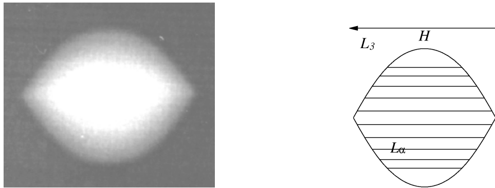
FIG. 11.20 – Sous faible champ magnétique ( H \approx 100 \sim 1000 \text{A.m}^{-1} ), les couches smectiques des gouttes de ferrosmectique de petites tailles (ici \sim 15 \mu\text{m} ) sont orientées parallèlement au champ. La forme des gouttes est très proche de ce qui a été observé dans le système CPCl (voir photo 5.2); G=6 , \varphi \approx 1\% .
