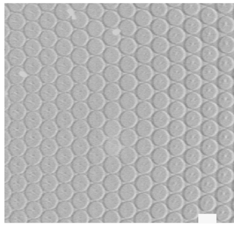
FIG. 6.8 – Réseau hexagonal de domaines focaux en lumière parallèle blanche. Barre= 20\mu\text{m} .
