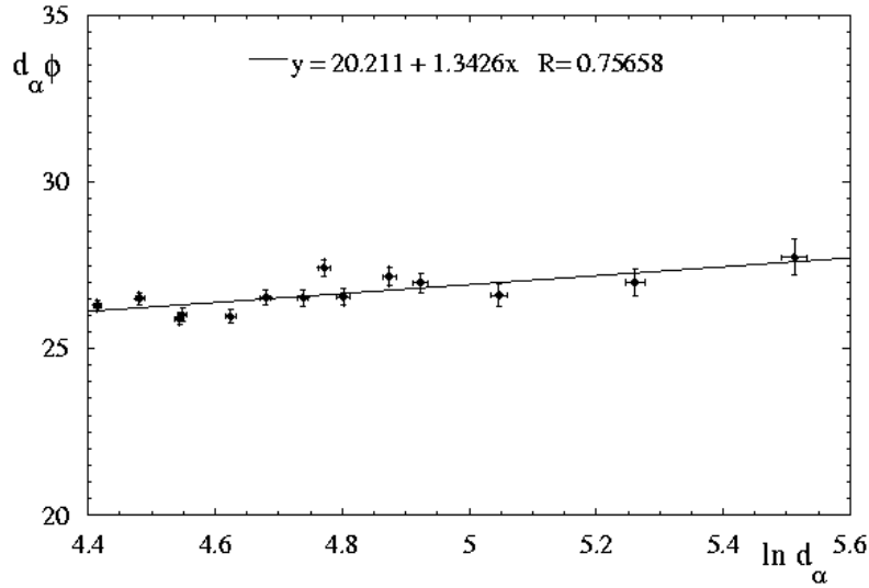
FIG. 10.11 – Représentation des points expérimentaux de la phase lamellaire dans le système de coordonnées (\ln d_\alpha, d_\alpha \phi) et droite d'ajustement obtenue par régression linéaire.
