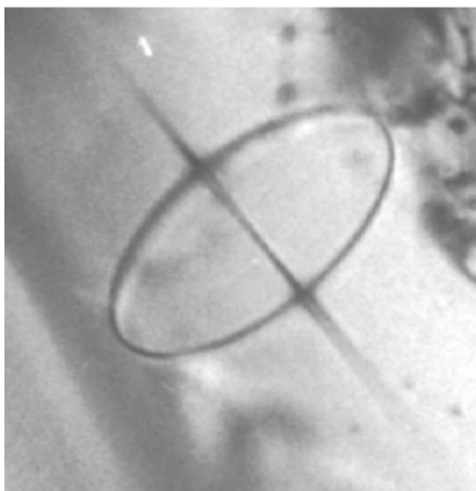
FIG. 1.8 – Les lignes singulières observées dans les Sm-A, sont des ellipses et hyperboles conjuguées (Observations réalisées dans le 4,4'-diéthyl azoxydibenzoate utilisé par G.FRIEDEL).
