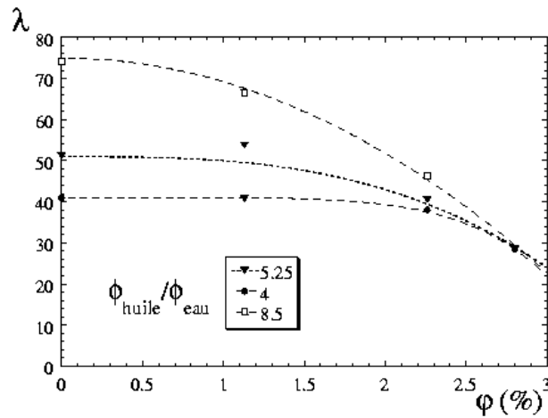
FIG. 11.17 – Allure de l'évolution de la longueur de pénétration smectique \lambda en fonction de la fraction volumique \varphi en particules dopantes pour différents rapports \phi_{\text{huile}}/\phi_{\text{eau}} , d'après [157]. Le gonflement G = 4 est proche de \phi_{\text{huile}}/\phi_{\text{eau}} = 5,25 et G = 6 correspond approximativement à \phi_{\text{huile}}/\phi_{\text{eau}} = 8,5 .
