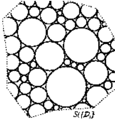
FIG. 7.8 – Assemblée quelconque de disques non-congruents, modélisant les assemblées de défauts précédents.
