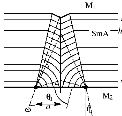
FIG. 7.5 – Modèle incluant à la fois une paroi et une déformation de la surface. La valeur de \eta est fixée par la compétition entre effets interfaciaux et effets de volume. On retrouve le cas de la FIG. 7.2 lorsque \sigma_1 \rightarrow \infty
