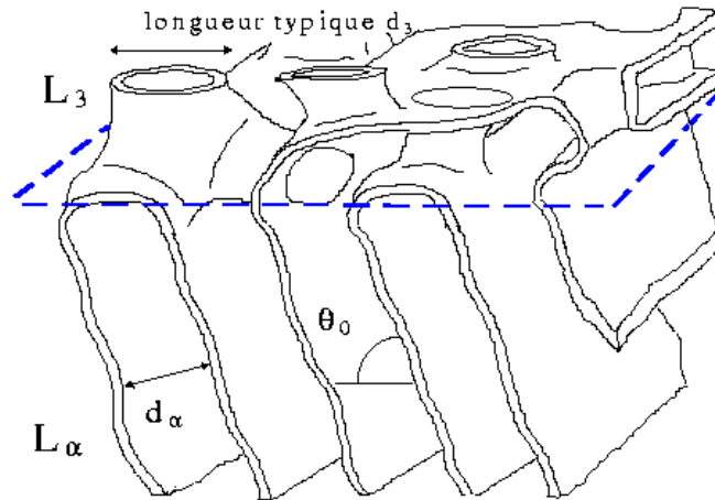
FIG. 10.1 – Vue schématique de l'interface L_\alpha - L_3 . Une faible déformation des phases en contact nécessite un ajustement des distances caractéristiques des deux phases à l'interface.
