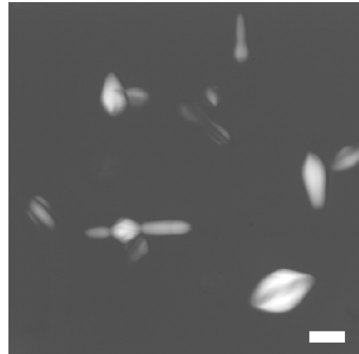
FIG. 4.10 – La forme et la texture des bâtonnets change avec leurs mode de croissance, mais ce polymorphisme peut être intrinsèque à certains régimes. Soumis à des conditions expérimentales communes, ces bâtonnets présentent des formes et textures finales variées. Barre 100\mu\text{m} .
