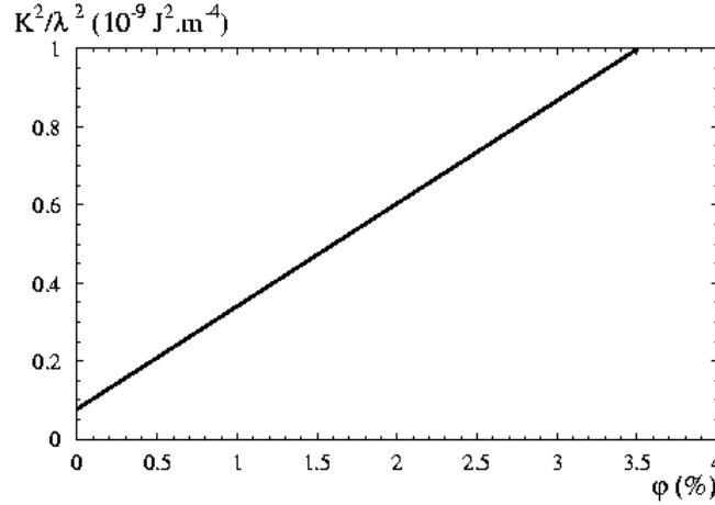
FIG. 11.18 – Allure de l'évolution du rapport K^2/\lambda^2 en fonction de la fraction volumique \varphi en particules dopantes pour un ferrosmectique de périodicité 30nm (ce qui correspond approximativement à G \approx 4 ); d'après[160].
