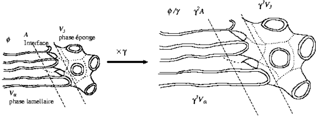
FIG. 11.3 – La dilatation du système \mathcal{S} d'un facteur \gamma laisse l'énergie libre invariante alors que les volumes sont multipliés par \gamma^3 et l'interface par \gamma^2 .
