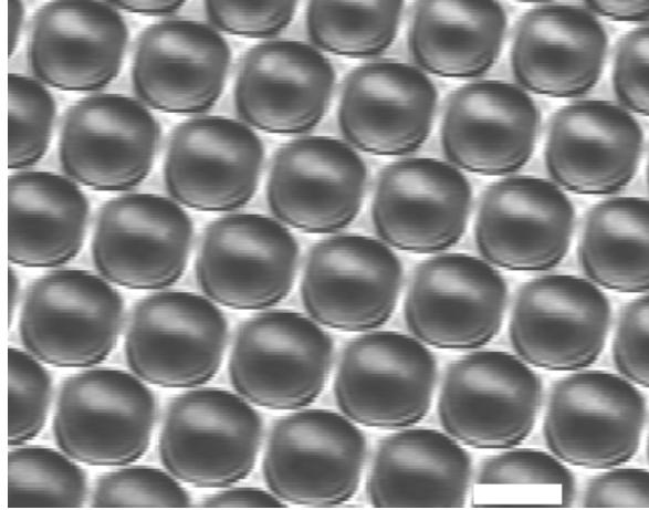
FIG. 7.1 – Les défauts apparaissant dans les couches minces de Sm-A comprises entre l'air et l'isotrope forment également des réseaux hexagonaux (4,4'-diéthyl azoxydibenzoate; polariseurs non parfaitement croisés; barre \approx 20\mu\text{m} ).
