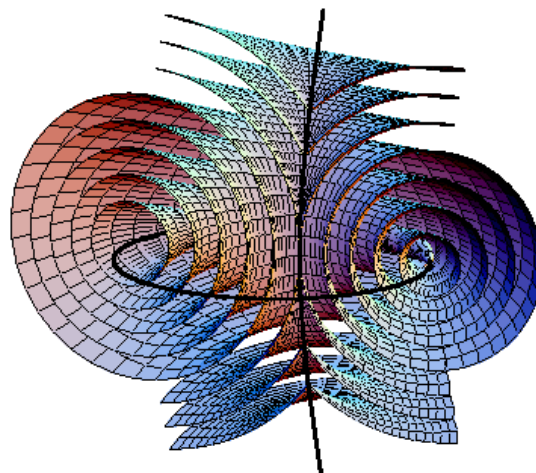
FIG. 1.9 – Conique focale de première espèce: les lieux des centres de courbures sont dégénérés en deux lignes singulières (ellipse et hyperbole). Dans les smectiques, seule la partie centrale est effectivement rencontrée (conique focale dite complète).
