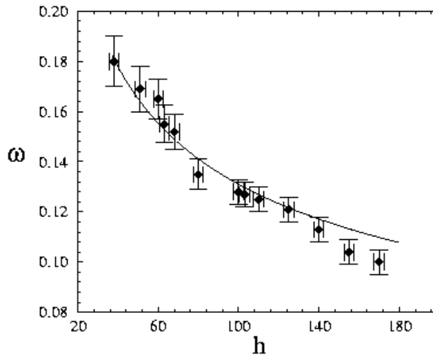
FIG. 6.13 – Évolution de \omega(\text{rad.}) vs. l'épaisseur h(\mu\text{m}) de la couche lamellaire.
