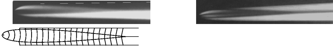
FIG. 6.5 – La construction proposée rend également compte de la forme de la paroi, lorsque la symétrie de révolution n'est plus respectée ( \phi_{w,m} = 0,6 ; taille latérale \approx 20\mu\text{m} ).
