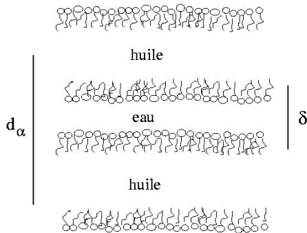
FIG. 11.12 – Phase lamellaire gonflée par le cyclohexane. La membrane est un film d'eau.
