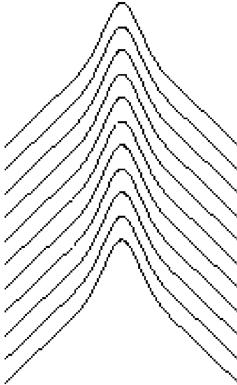
FIG. 6.17 – Aux grands angles dans les copolymères diblock, des parois en «omega» sont observées (ici une représentation schématique).
