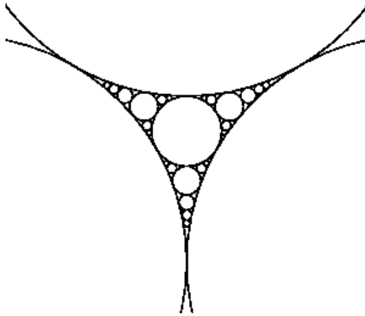
FIG. 7.24 – Le pavage apollonien consiste à remplir les interstices du réseau RH par des disques de tailles décroissantes (ici seuls les disques les plus grands sont représentés). La dimension fractale (de Hausdorff) de cet empilement est voisine de 1,31.
