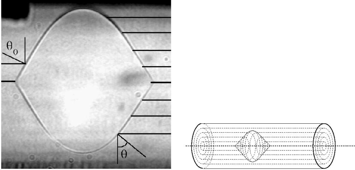
FIG. 5.4 – Goutte de phase L_3 située au centre d'un capillaire cylindrique de phase L_\alpha orientée par le substrat. Son axe de révolution est l'axe du capillaire et elle présente deux points singuliers à ses pôles. Gonflement: \phi_w = 0,85 .
