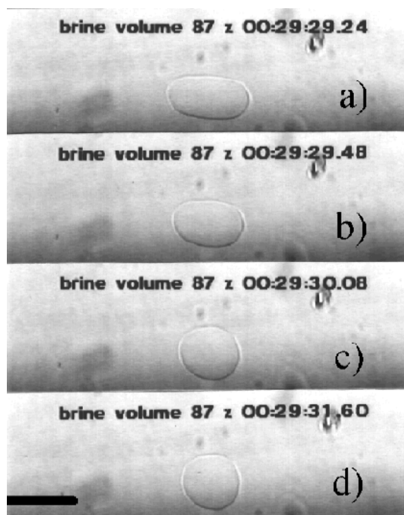
FIG. 9.4 – Exemple typique de la relaxation d’une goutte de phase lamellaire dans la phase éponge. Fraction massique de solvant \phi_{w,m} = 0,87 , fraction volumique de membrane \phi = 0,147 ; rayon de la goutte 44\mu\text{m} .
