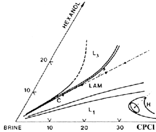
FIG. 2.2 – Diagramme de phase (d'après [51]) du système quasi-ternaire CPCI/hexanol/saumure (NaCl 0,2M).
