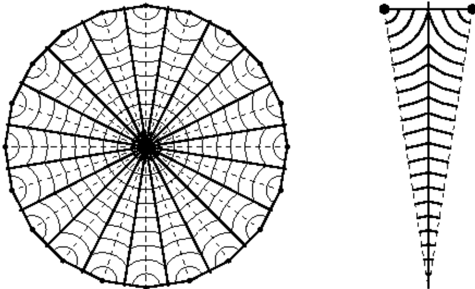
FIG. 8.5 – L'introduction de défauts permet toujours d'approcher une forme sphérique en assurant l'orientation \theta_0 des couches à l'interface. Dans ce pavage de DCFs, aucune paroi n'est géométriquement nécessaire car les interstices entre domaines peuvent toujours être comblés par des portions de sphères centrées sur le centre de la goutte.
