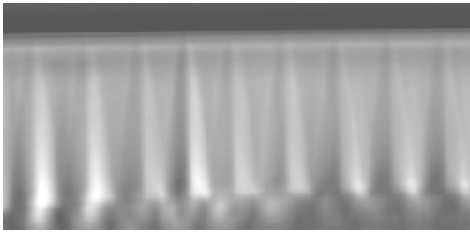
FIG. 6.15 – Vue de côté des défauts sur la paroi latérale d'un capillaire. On s'aperçoit que la surface de discontinuité n'est pas parfaitement conique. h \approx 65\mu\text{m} .
