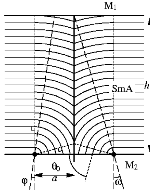
FIG. 7.3 – Lorsque l'ancrage est plus faible, les déformations volumiques relaxent et la paroi disparaît.
