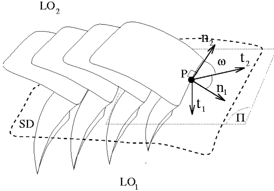
FIG. 6.4 – Paroi de courbure à l'échelle optique entre deux organisations lamellaires quelconques.
