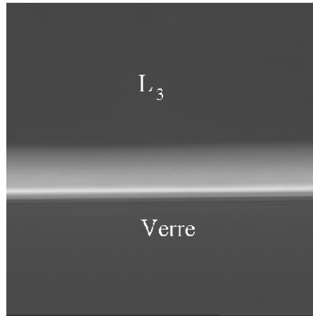
FIG. 4.6 – Une mince couche de phase L_\alpha (épaisseur 30\mu\text{m} ) est prise en « sandwich » entre la phase L_3 et le substrat de verre qui l’a orientée (région centrale de la paroi latérale d’un capillaire de 400\mu\text{m} d’épaisseur). Dans cette géométrie, les couches sont parallèles à l’interface et l’angle de contact \theta_0 n’est pas observé. Remarquons la différence de comportement avec la FIG. 4.3.
