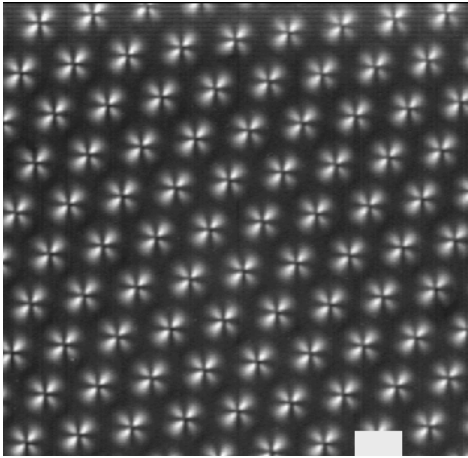
FIG. 6.7 – Réseau hexagonal de domaines focaux entre polariseurs croisés. Barre= 20\mu\text{m} .
