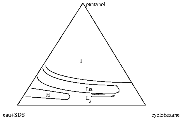
FIG. 11.13 – Allure du diagramme des phases du système lyotrope SDS/ cyclohexane /eau /pentanol à rapport E/S=2,5 . H désigne une phase hexagonale.
