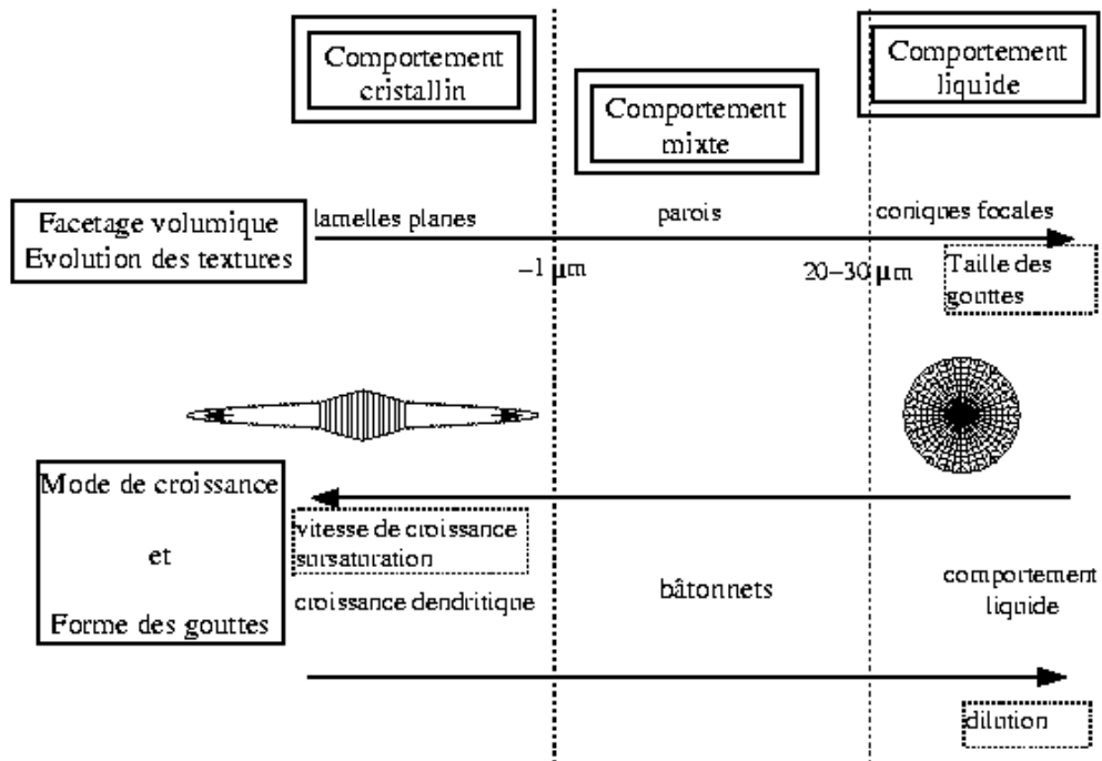
FIG. 8.12 – Evolution qualitative des caractéristiques des gouttes de phase L_\alpha dans la phase L_3 en fonction de la taille des gouttes, des vitesses de croissance et de la dilution.
