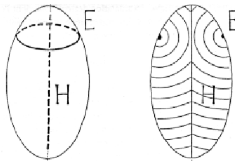
FIG. 1.18 – L'introduction de coniques focales abaisse l'énergie interfaciale de -\Delta\sigma L^2 pour un coût énergétique de KL . Les coniques focales apparaissent donc spontanément pour des tailles plus grandes que l_0 = K/\Delta\sigma (d'après FOURNIER[36]).
