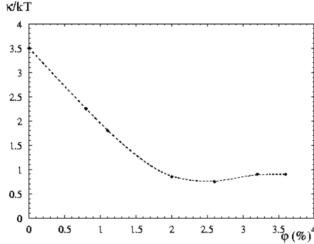
FIG. 11.16 – Allure de l'évolution de la constante de rigidité \kappa de la membrane des phases ferrosmectiques au voisinage de la phase éponge en fonction de la fraction volumique \varphi en particules dopantes; d'après [150].
