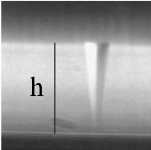
FIG. 6.9 – Vue de côté d'un défaut sur la paroi latérale d'un capillaire. Le défaut est inséré dans une couche homéotrope de phase lamellaire. h \approx 37\mu\text{m} .
