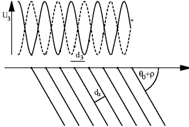
FIG. 11.7 – Dans la limite de la phase L_\alpha infiniment rigide, l'énergie d'ancrage provient uniquement du champ de déplacement \nu(x) à l'interface.
