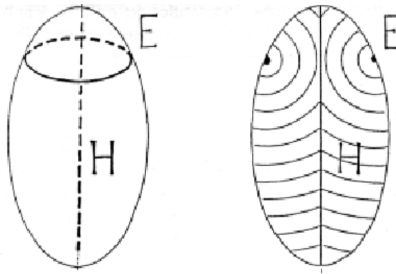
FIG. 6.18 – L'introduction de coniques focales abaisse l'énergie interfaciale de -\Delta\sigma L^2 pour un coût énergétique de KL . Les coniques focales apparaissent donc spontanément pour des tailles plus grandes que l_0 = K/\Delta\sigma (d'après FOURNIER[36]).
