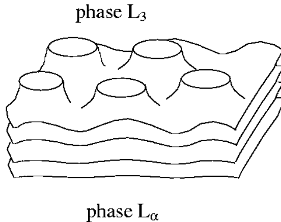
FIG. 11.10 – Le contact tangentiel des couches à l'interface est une alternative à l'épitaxie des deux phases car l'ajustement des distances d_\alpha et d_3 n'est plus nécessaire.
