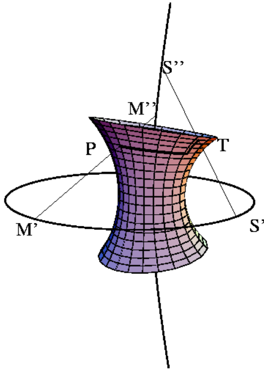
FIG. 1.12 – Paramétrisation d'une cyclide de Dupin, à partir des points de l'ellipse et de l'hyperbole.
