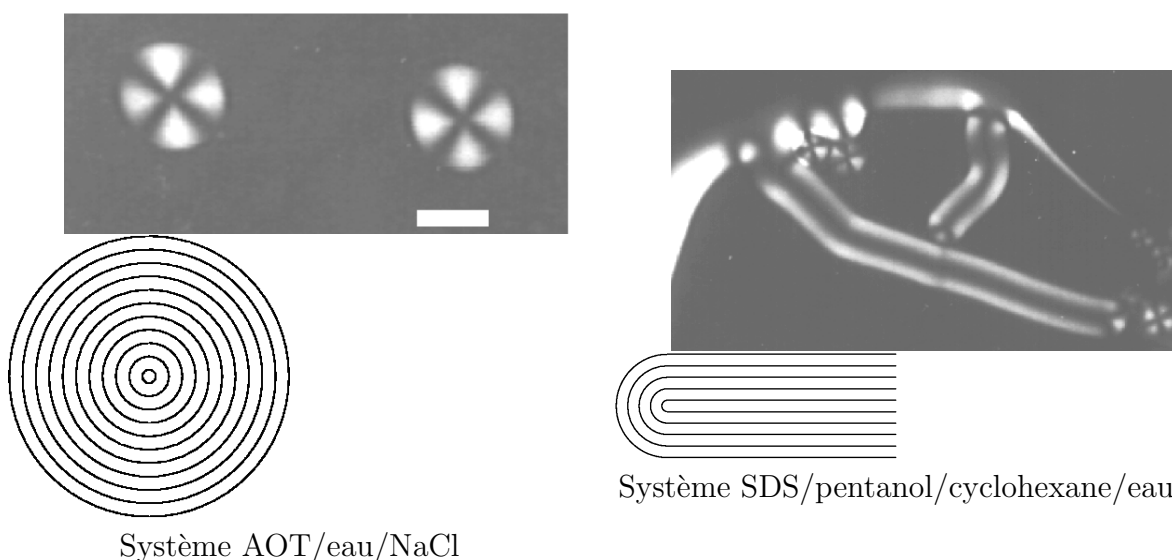
FIG. 11.11 – Dans certains systèmes lyotropes, les couches arrivent tangentiellement à l'interface L_\alpha - L_3 . Les gouttes de phase L_\alpha sont alors constituées d'un empilement de couches sphériques (photo de gauche) ou encore de formes «myélines», encore appelées «filaments», constituées d'un empilement de couches cylindriques et dont l'extrémité est un empilement de couches en demi-sphères (photo de droite).
