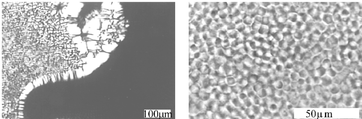
FIG. 3.6 – À gauche : l'obtention de la phase lamellaire par refroidissement de la phase micellaire en croissance directionnelle lente ( 0,1\mu.m.s^{-1} ) donne une phase homéotrope (fond noire) présentant des stries huileuses, alors que le reste de l'échantillon qui a subi une trempe est constitué d'objets de taille homogène ( vraisemblablement des sphérolites : voir agrandissement à droite). Les textures sont stables et conservent leur apparence au cours du temps. \phi = 0.25 , h/c = 0.49 , épaisseur 50\mu.m .
