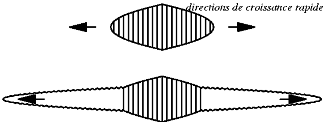
FIG. 8.7 – La symétrie particulière du cristal L_\alpha , la raideur de surface (minimale en \theta = 0 ) et la plage d'orientations interdites au voisinage de \theta = \pi/2 conduisent à des dendrites sans branches secondaires présentant une instabilité d'Herring sur sa surface latérale.
