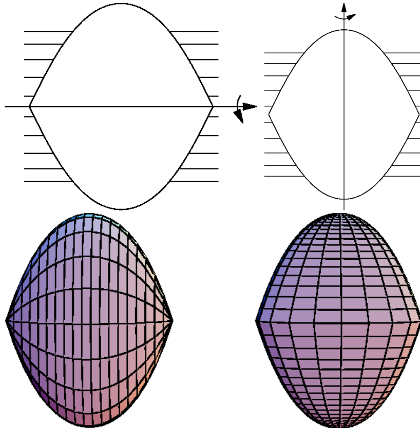
FIG. 5.12 – Si la construction de Wulff est identique en deux dimensions, la forme tridimensionnelle des gouttes diffère selon l'organisation des lamelles en plan ou en cylindres. Les gouttes 3D présentent soit deux points singuliers (lamelles empilées en cylindres : FIG. 5.4 et 5.19), soit une ligne équatoriale singulière (lamelles planes : FIG. 5.2).
