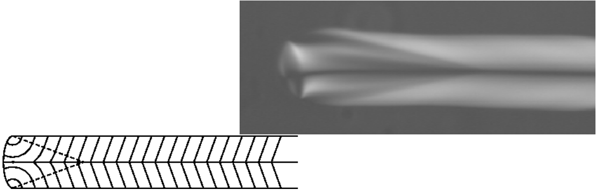
FIG. 6.6 – Un domaine focal à l'extrémité des bâtonnets «glaive I» est observé dans les gouttelettes de taille \mathcal{T} > \mathcal{T}_c . Ici le cylindre a pour rayon r_b \approx 20\mu\text{m} .
