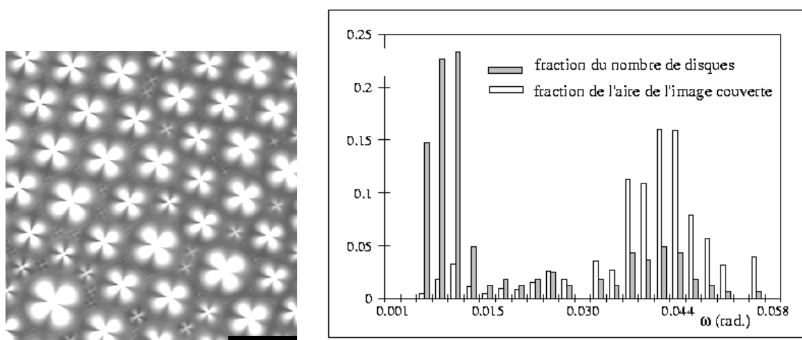
FIG. 7.23 – Aux grandes épaisseurs, il n'y a pas d'organisation à grande distance. Néanmoins les distances caractéristiques \omega_1 \approx \omega_0 et les tailles dérivées (ici \beta\omega_1 ) sont mises en évidence dans l'histogramme des tailles, sous la forme de deux bosses représentant un maximum dans la surface couverte ( \omega_1 \approx 0,44 ) et le nombre de disques (petit défauts de taille \beta\omega_1 \approx 0,008 ). Épaisseur 900\mu m . Barre= 100\mu m .
