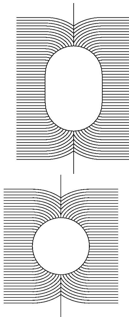
FIG. 6.22 – Texture satisfaisant les conditions aux limites et sans autre singularité que les demi-droites issues des pôles. La figure du dessous correspond à une tension interfaciale importante.
