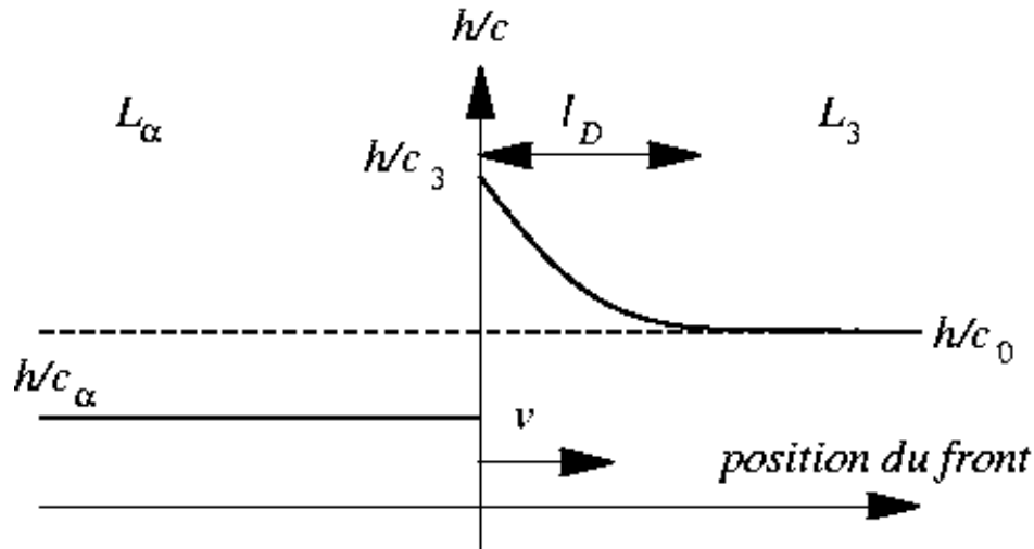
FIG. 8.4 – La croissance des germes lamellaires, dans le régime diffusif, se traduit par une croissance du rapport h/c devant le germe.
