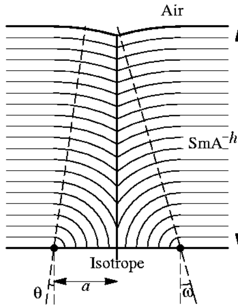
FIG. 7.4 – Déformation simple de la surface M_1/Sm sans autre défaut. Ce modèle de FOURNIER peut être amélioré en introduisant une déformation de type paroi (FIG. 7.5).
