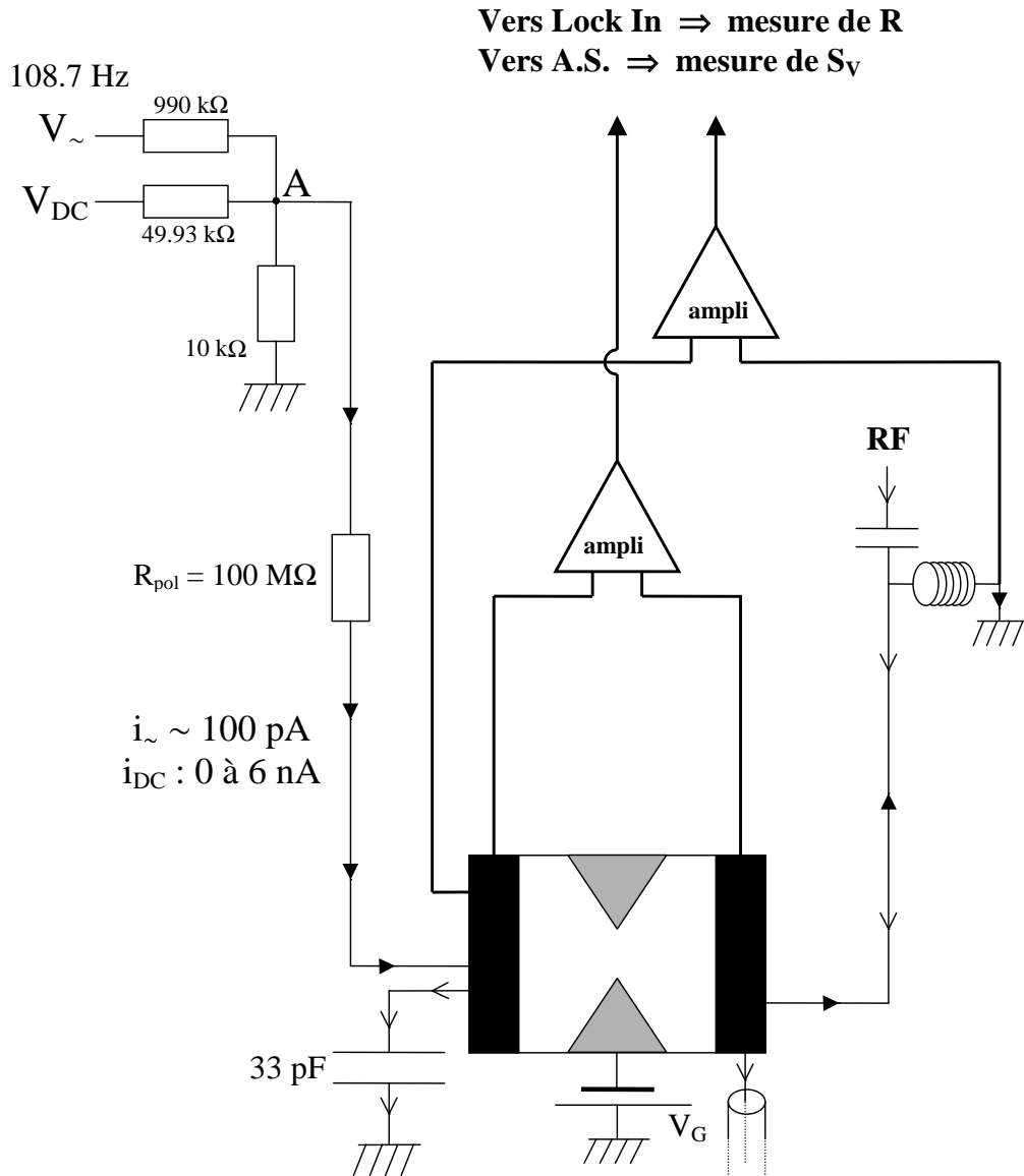
FIG. 3.6 – Schéma du montage expérimental : l'injection de courants continu et alternatif se fait par une résistance de polarisation de 100.86 \text{ M}\Omega à température ambiante. La tension aux bornes de l'échantillon est amplifiée par deux voies d'amplification bas bruit. La mesure de la résistance de l'échantillon est faite par des détections synchrones, et la mesure des corrélations de tension par un analyseur de spectre. Enfin, la modulation RF est injectée sur un contact de l'échantillon, l'autre étant maintenu à la masse par une capacité de 33 \text{ pF} .
