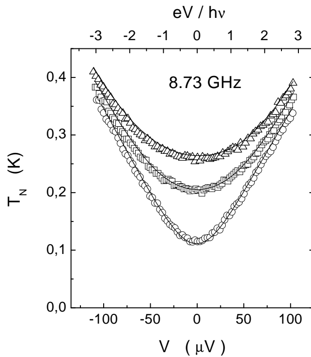
FIG. 5.14 – Température de bruit en fonction de V , pour \nu = 8.73 GHz. Les symboles correspondent aux points expérimentaux, et les courbes en trait plein sont les courbes théoriques obtenues sans paramètre ajustable pour les valeurs de \alpha et de T suivantes, déduites des mesures de la figure (5.13) : \alpha = 0.51; 1.81; 2.56 , et T = 105.5; 145; 167.7 mK.
