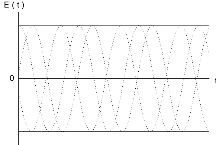
FIG. 9.3 – Représentation du champ électrique en un point donné en fonction du temps pour un état nombre. On peut l'écrire comme une somme de sinusoïdes (en pointillés) d'amplitudes parfaitement définies, mais de phases aléatoires. Le champ électrique est donc bien nul en moyenne.
