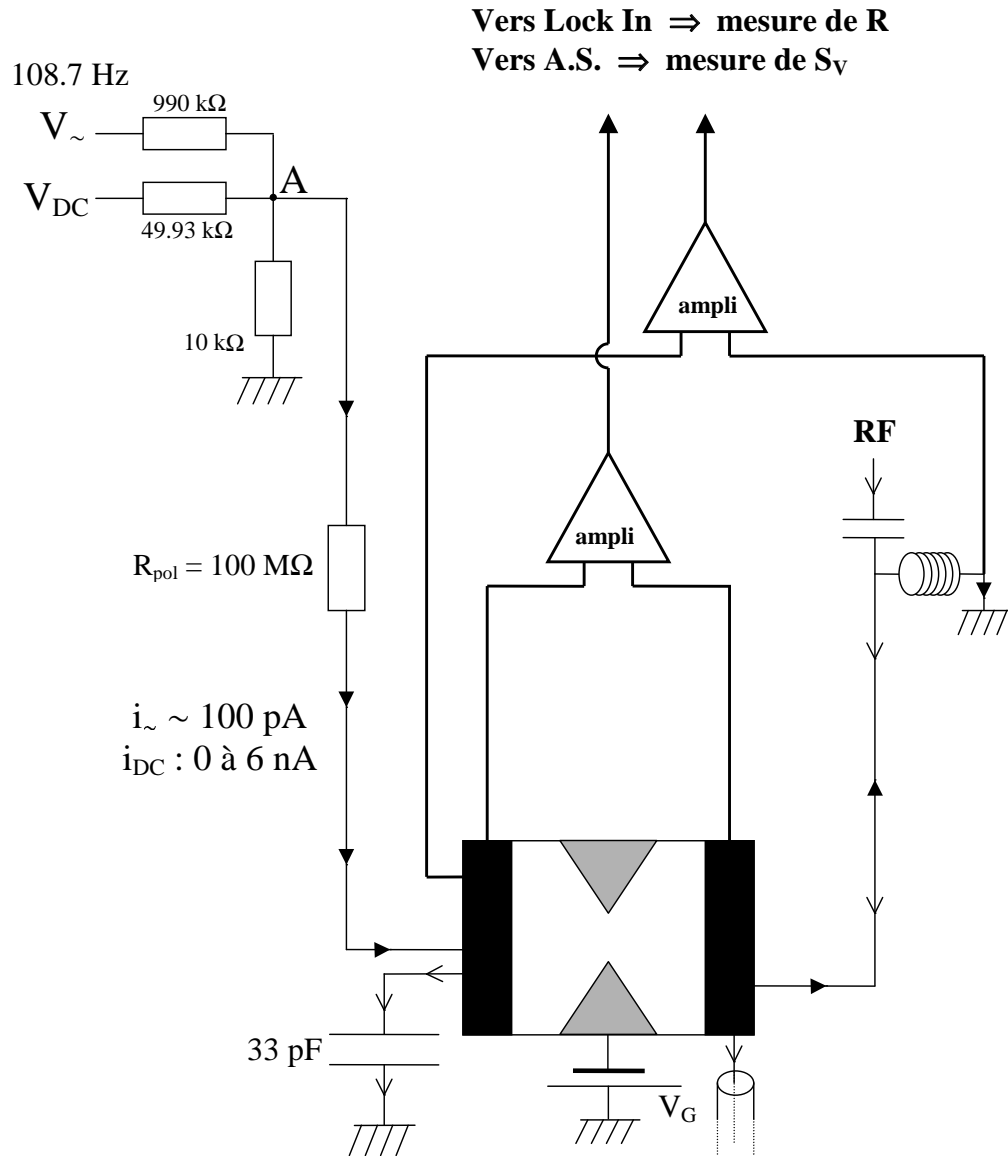
FIG. 3.6 – Schéma du montage expérimental : l'injection de courants continu et alternatif se fait par une résistance de polarisation de 100.86\text{ M}\Omega à température ambiante. La tension aux bornes de l'échantillon est amplifiée par deux voies d'amplification bas bruit. La mesure de la résistance de l'échantillon est faite par des détections synchrones, et la mesure des corrélations de tension par un analyseur de spectre. Enfin, la modulation RF est injectée sur un contact de l'échantillon, l'autre étant maintenu à la masse par une capacité de 33\text{ pF} .
