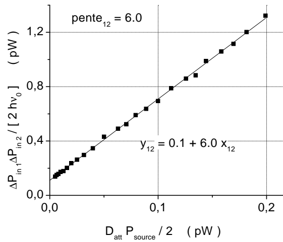
FIG. 9.18 – Courbes identiques aux courbes de la figure (9.17), mais obtenues avec les filtres B, et une fréquence d'émission de 1.72 GHz.
