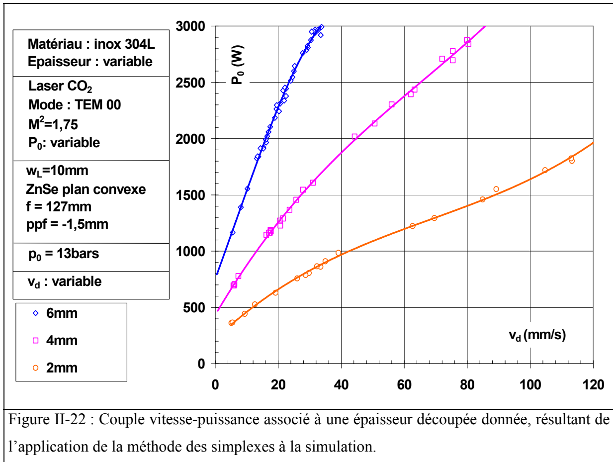
Figure II-22 : Couple vitesse-puissance associé à une épaisseur découpée donnée, résultant de l'application de la méthode des simplexes à la simulation.
