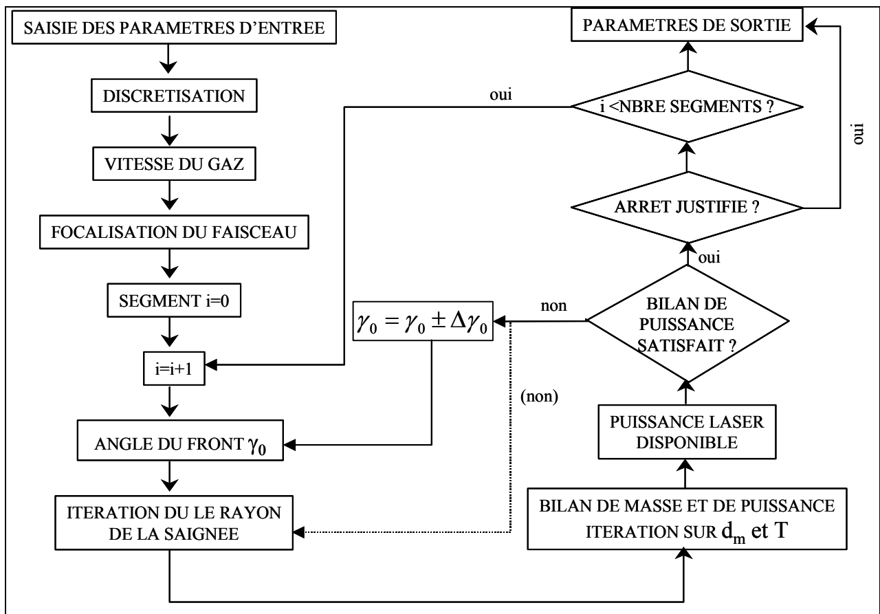
Figure I-3 : Principe de modélisation de la découpe par le Dr. D. Petring.
