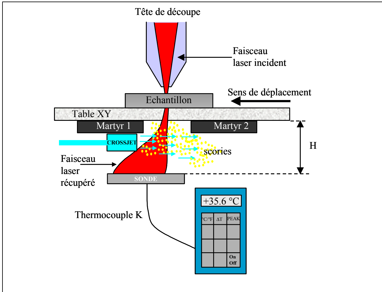
Figure II-34 : Schéma de montage de l'expérience de mesure des puissances passantes au travers de la saignée durant le procédé de découpe laser.
