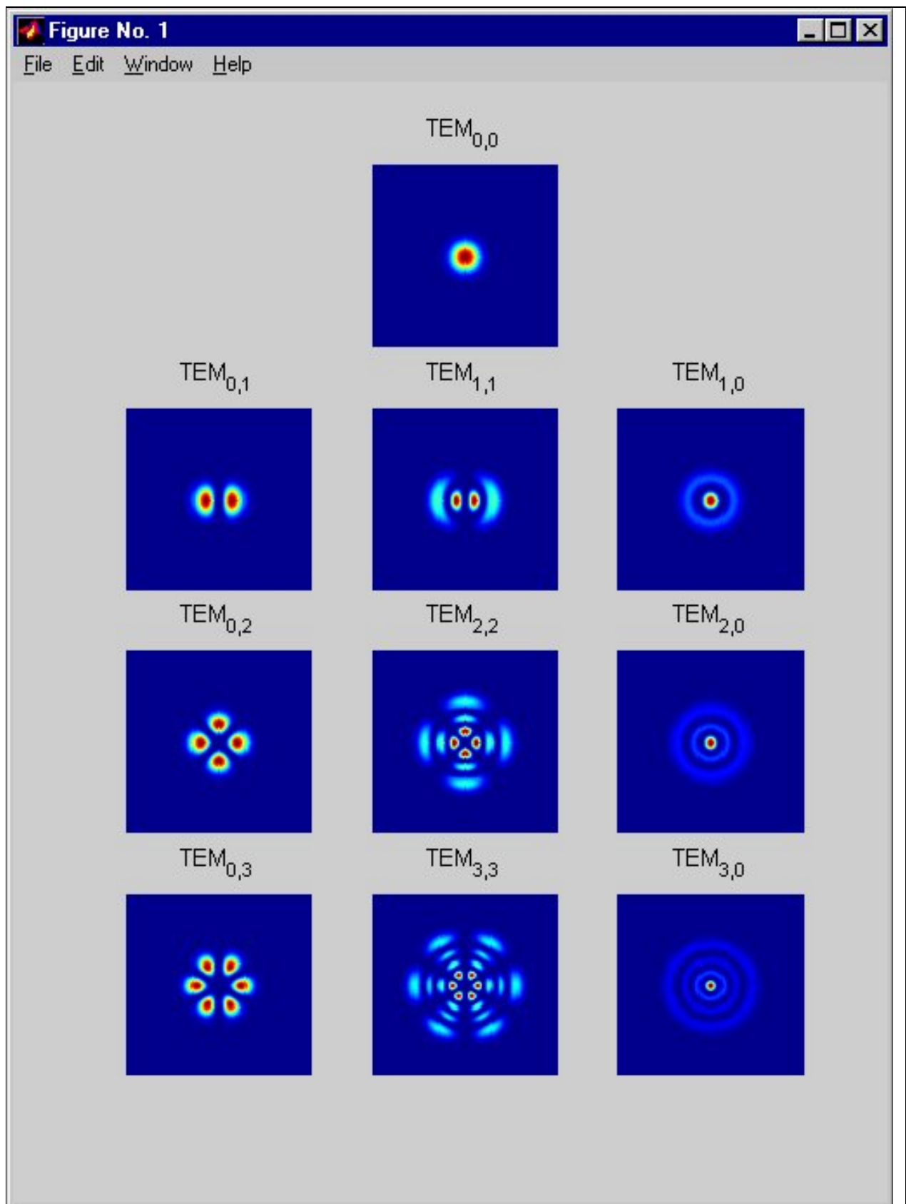
Figure III-2 : Représentation des modes LG en fonction de leur nombre d'annulation
