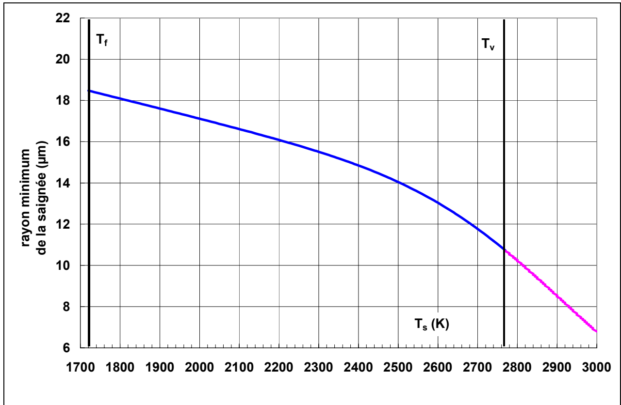
Figure II-51 : Evolution du rayon minimum de la saignée dans le cas d'un acier inoxydable, en fonction de la température de surface.
