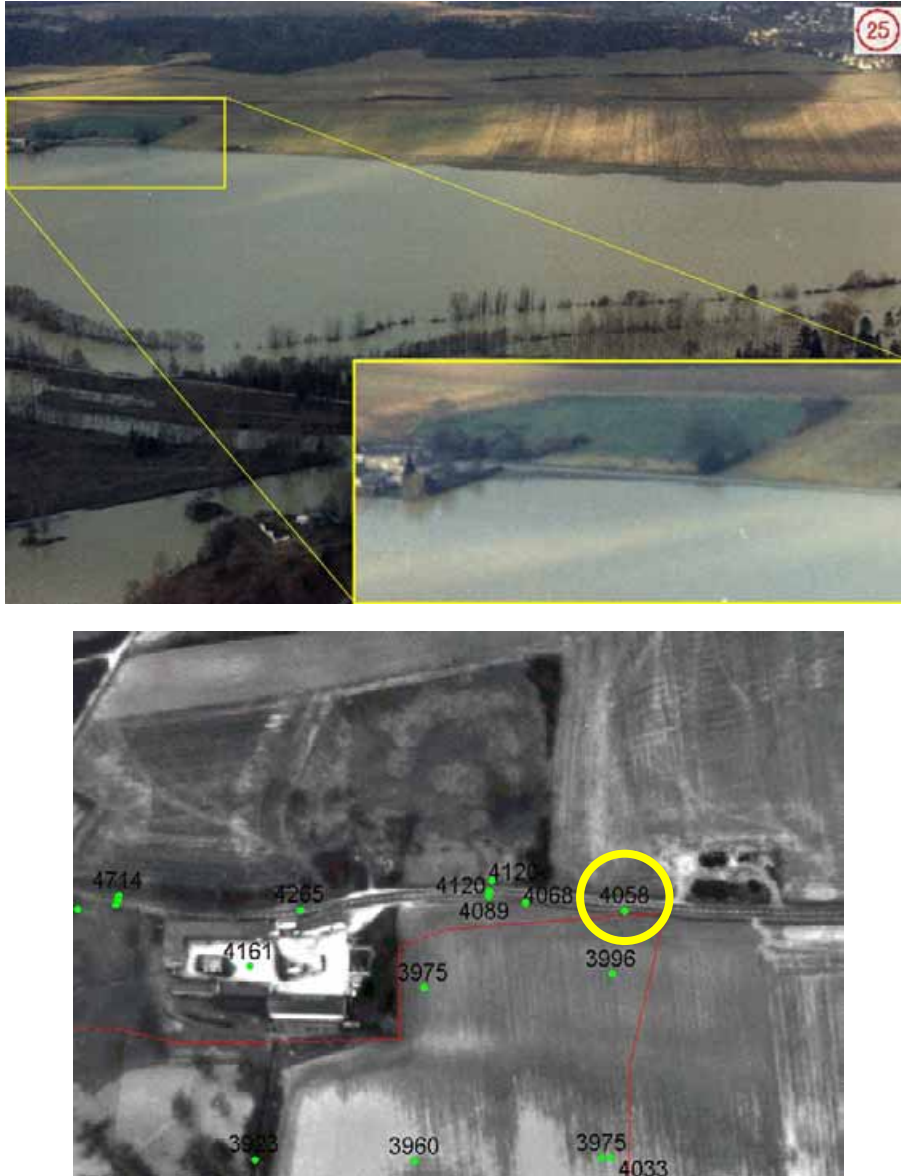
Figure 11-8 : Analyse du point coté ayant conduit à limiter les bornes Max des estimations à l'amont du pont de Pommier.
