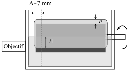
FIG. 6.12: Schéma du dispositif expérimental. La pointe liquide n'est pas collée à la paroi.
