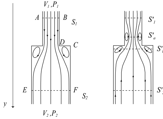
FIG. 1.9: Lignes de courant schématisées au passage de brusques élargissement et rétrécissement de sections. Les zones de recirculation sont schématisées dans les deux cas.
