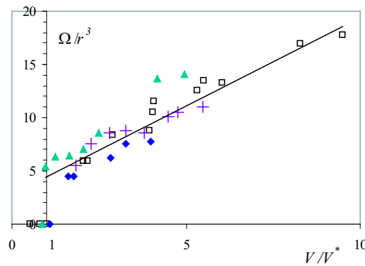
FIG. 3.20: Volume de liquide éjecté sous le trou divisé par le rayon du trou au cube, en fonction du rapport de la vitesse d'impact sur la vitesse seuil.
