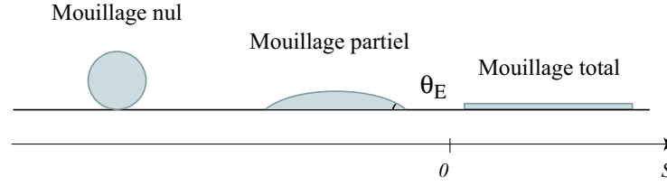
FIG. 3: Différentes situations de mouillage sur une surface plane.
