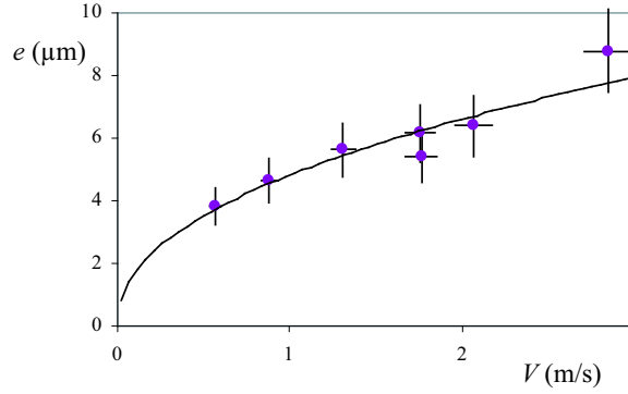
FIG. 8.14: Épaisseur du film d'air entraîné par un jet d'huile silicone ( \eta = 0.35 Pa.s) en fonction de la vitesse d'entraînement V , mesurée par la conservation du volume d'air.
