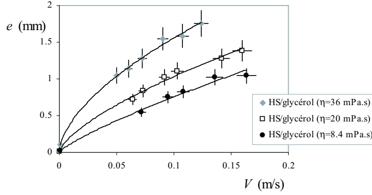
FIG. 8.16:   paisseur e d'un film d'huile silicone entra  n   par du glyc  rol en rotation solide autour d'un rouleau en fonction de la vitesse d'entra  nement V pour diff  rentes huiles. Les ajustements sont du type V^\alpha , avec 0.6 < \alpha < 0.8 .
