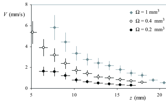
FIG. 5.13: Vitesse V de gouttes de différents volumes reportée en fonction de leur position sur la fibre z . Les gouttes sont toutes d'huile silicone de viscosité \eta = 5 \text{ mPa.s}
