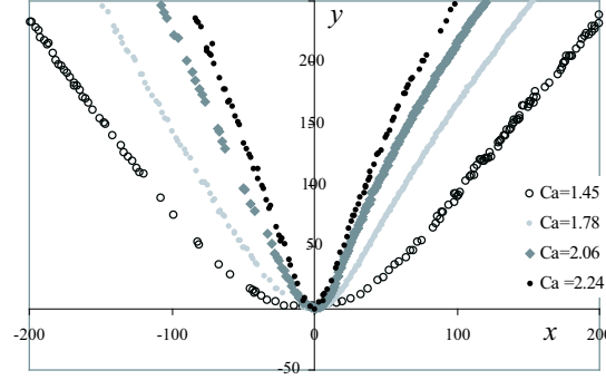
FIG. 6.20: Profil de la pointe pour différentes vitesses d'entraînement du rouleau. Les unités sont arbitraires et correspondent au grain de la photo.
