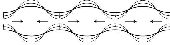
FIG. 2: Les zones de plus grandes courbures se vident dans celles de plus petites courbures, amplifiant ainsi la fluctuation initiale d'épaisseur.
