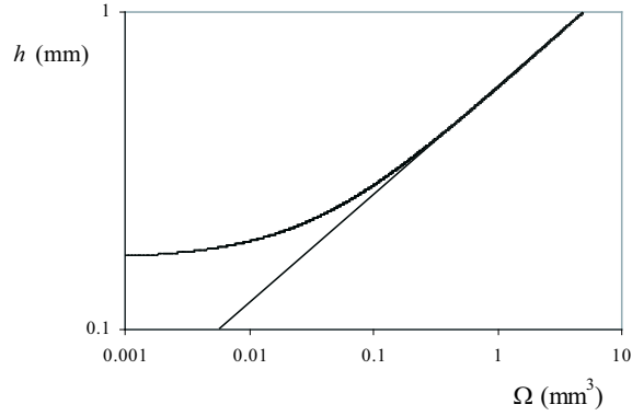
FIG. 5.9: Rayon maximal h (calculé) d'une goutte en fonction de son volume. La fibre fait 150\text{ }\mu\text{m} de rayon.
