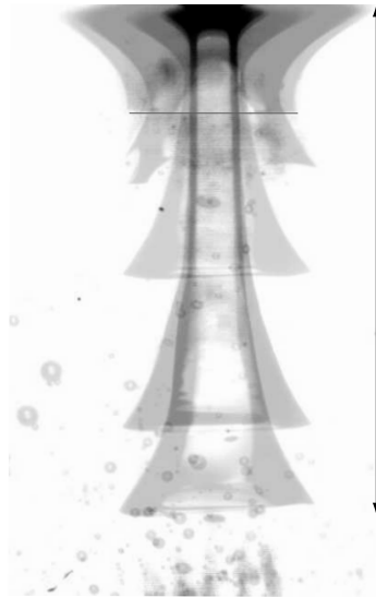
FIG. C.1: Phase de la croissance de la trompette dans de l'huile silicone visqueuse \eta = 970 mPa.s. La taille l maximale de la trompette est ici de 1.5 cm, et les images sont espacées d'environ 200 ms.
