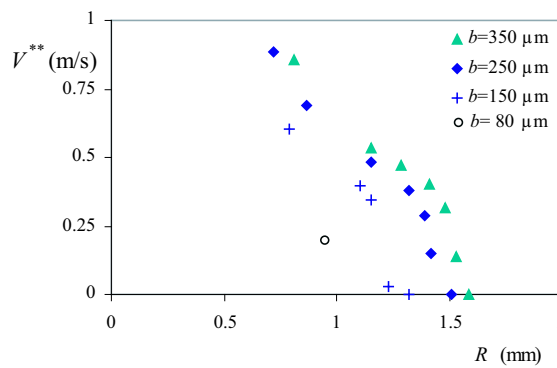
FIG. 4.17: Vitesse seuil de capture en fonction de la taille de gouttes d'eau tombant sur des fibres de rayons différents.
