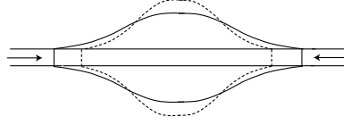
FIG. A.3: Perturbation axisymétrique de la goutte.
