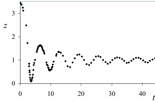
FIG. 1.7: Position de l'interface air liquide z en fonction du temps t partant d'une situation où le tube est surrempli. Le tube a un rayon de 1 cm et est immergé à 10 cm de profondeur.
