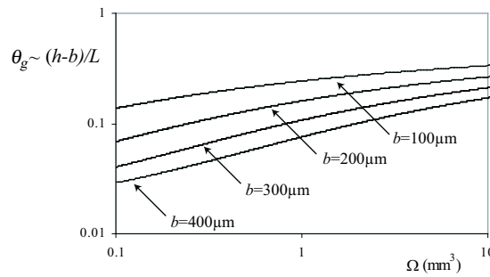
FIG. 5.16: Angle géométrique de la goutte \theta_g \sim (h-b)/L calculé à partir des formules de Carroll pour des fibres de différents rayons.
