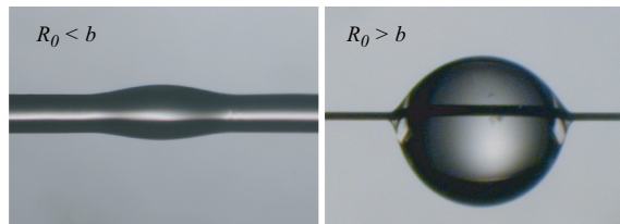
FIG. 5.10: Deux gouttes d'huile silicone dans les limites "petit" et "grand" volume. À gauche, on pose une goutte de rayon R_0 = 80\text{ }\mu\text{m} sur une fibre b = 100\text{ }\mu\text{m} : la conformation apparaît être très étalée ( h \simeq b ). À droite, on pose une goutte de rayon R_0 = 200\text{ }\mu\text{m} sur une fibre b = 12\text{ }\mu\text{m} et la goutte est quasi-sphérique.
