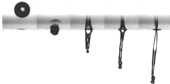
FIG. 3.18: Impact d'une goutte d'huile silicone légère très rapide ( V = 2m/s ) dans un trou de 450 μm de rayon.
