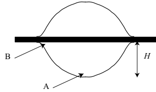
FIG. 4.11: Schéma d'une grosse goutte sur une petite fibre de rayon b .
