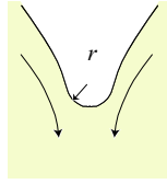
FIG. 6.18: Schéma de l'extrémité d'une pointe bidimensionnelle.
