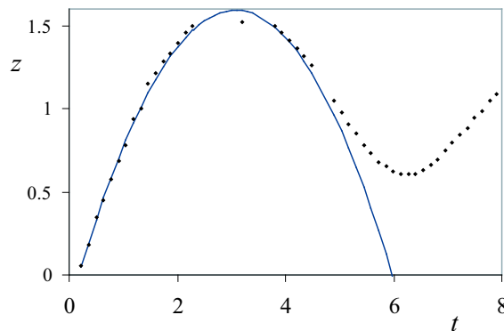
FIG. 1.5: Position de l'interface z en fonction du temps t . Les données expérimentales sont bien décrites jusqu'au maximum par une parabole d'équation z(t) = -0.2t^2 + 1.2t - 0.2 .
