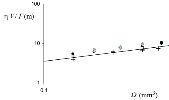
FIG. 5.18: Vitesse de gouttes de différents volumes et viscosités dévalant d'une fibre inclinée de 7^\circ .
