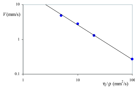
FIG. 5.14: Vitesse V de gouttes isovolumes ( \Omega = 0.6 \text{ mm}^3 ) d'huile silicone de différentes viscosités reportée en échelle logarithmique en fonction de la viscosité cinématique \eta/\rho des liquides utilisés.
