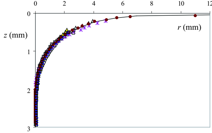
FIG. 8.21: Superposition des différents profils de l'interface air/huile silicone en amont de la trompette correspondant à différentes vitesses. La courbe en trait plein est l'équation du ménisque statique d'un liquide en mouillage nul sur un solide vertical. Chaque type de symbole indique un profil correspondant à une vitesse différente entre 0.7 et 2.2 m/s.
