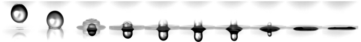
FIG. 3.3: Une goutte d'huile silicone peu visqueuse ( \eta = 0.5\ \text{mPa}\cdot\text{s} , \gamma = 16\ \text{mN/m} ) tombe dans un trou de 390\ \mu\text{m} de rayon percé dans une plaque de 250\ \mu\text{m} d'épaisseur. Les photos sont prises toutes les 2\ \text{ms} . La goutte est totalement capturée par la surface, même si un doigt de liquide apparaît transitoirement sous le trou. Noter qu'on voit sur les images le reflet de ce doigt ainsi que la figure d'impact de la goutte sur la face supérieure.
