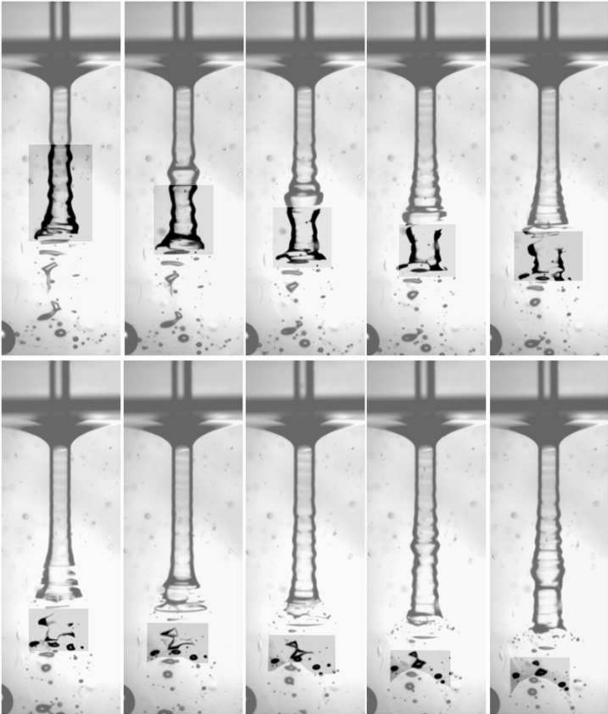
FIG. 8.13: Évolution d'une tranche d'air (en grisé) qui se déstabilise pour former des bulles. L'intervalle entre les photos est de 4 ms. La longueur de la trompette est de l'ordre de 15 mm. Le jet de 1.5 mm de diamètre d'huile silicone ( \eta = 0.35 Pa.s) tombe à 1.76 m/s dans un bain du même liquide. Nous remarquons que la trompette est ondulée, nous discutons ce point dans l'annexe C.
