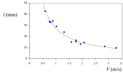
FIG. C.3: Longueur de la trompette en fonction de la vitesse d'impact dans de l'huile silicone \eta = 350 mPa.s. Les données sont ajustées par une loi de puissance d'exposant -0.92.
