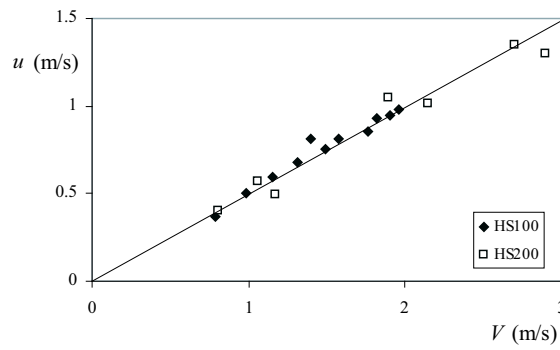
FIG. 8.15: Vitesse de déplacement d'une vague en fonction de la vitesse du jet de liquide pour deux huiles silicones de différente viscosité. La pente de la droite tracée vaut 1/2 .
