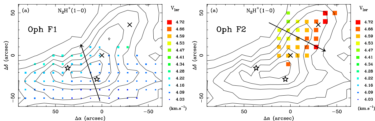
FIG. 5.14 – Cartes des vitesses centroïdes N_2H^+(1-0) des deux composantes du cœur dense Oph F. Sur chaque panneau, les vitesses centroïdes mesurées par ajustement HFS des spectres N_2H^+(1-0) de rapport signal-sur-bruit suffisant sont indiquées par des carrés pleins dont la taille augmente et dont la couleur passe du bleu au rouge lorsque la vitesse augmente. Pour les positions autour de F-MM2 dont les spectres sont doubles (cf. Fig. 5.13e), nous n’avons indiqué sur chaque panneau que la vitesse centroïde associée à la région concernée. Les contours rappellent la carte d’intensité intégrée en N_2H^+(1-0) . Les croix indiquent les positions (MAN98) des condensations préstellaires F-MM1 et F-MM2 ( 0'', 0'' ), et les étoiles symbolisent les proto-étoiles YLW15/IRS43 et CRBR85. Les directions des gradients de vitesse moyens mesurés par la méthode de GBFM93 sont indiquées par des flèches.
