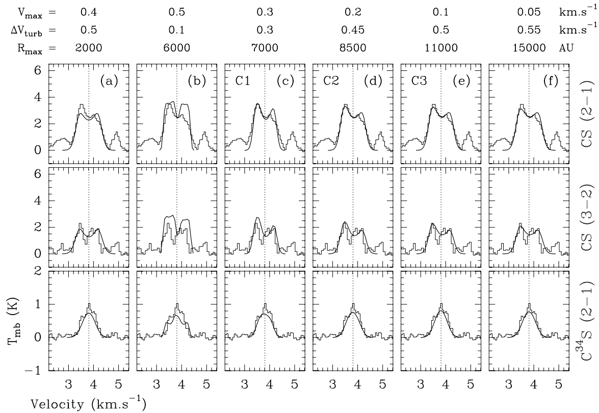
FIG. 5.12 – Effets du rayon R_{\max} et de la vitesse V_{\max} du pic de vitesse sur les spectres centraux CS(2-1) (1 ère ligne), CS(3-2) (2 ème ligne) et C^{34}S(2-1) (3 ème ligne) de OphC-MM5 . Les colonnes (c), (d) et (e) rappellent les modèles C1, C2 et C3 des Fig. 5.4, 5.5 et 5.6.
