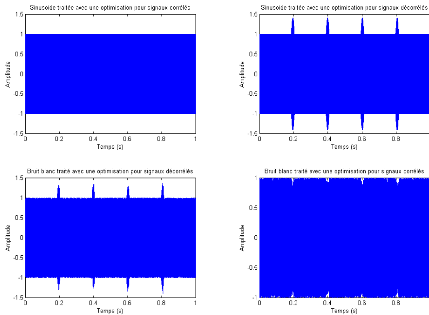
Figure 3.27 – Exemples de traitements optimisés pour des signaux corrélés et décorrésés
