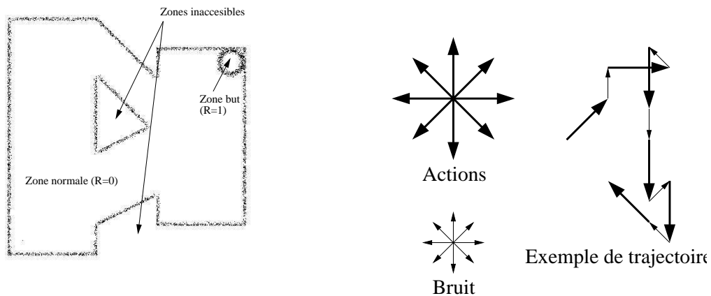
FIG. 3.1: Une tâche de navigation continue. Un agent de type robot doit se frayer un chemin dans un environnement contenant deux pièces et deux couloirs afin de rallier une zone but. Chacun de ses déplacements est bruité : à chaque mouvement se rajoute un bruit aléatoire. Par exemple, nous avons reproduit une trajectoire possible lorsque l'agent effectue successivement les actions Nord-Est, Est, Sud, Sud, Sud, Nord-Ouest.
