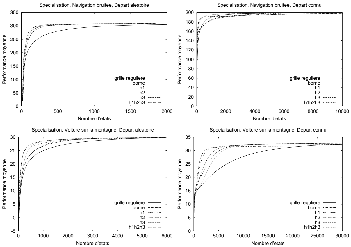
FIG. 4.8: Évaluation des heuristiques pour le processus de spécialisation. Voir les commentaires concernant ces courbes dans le texte.
