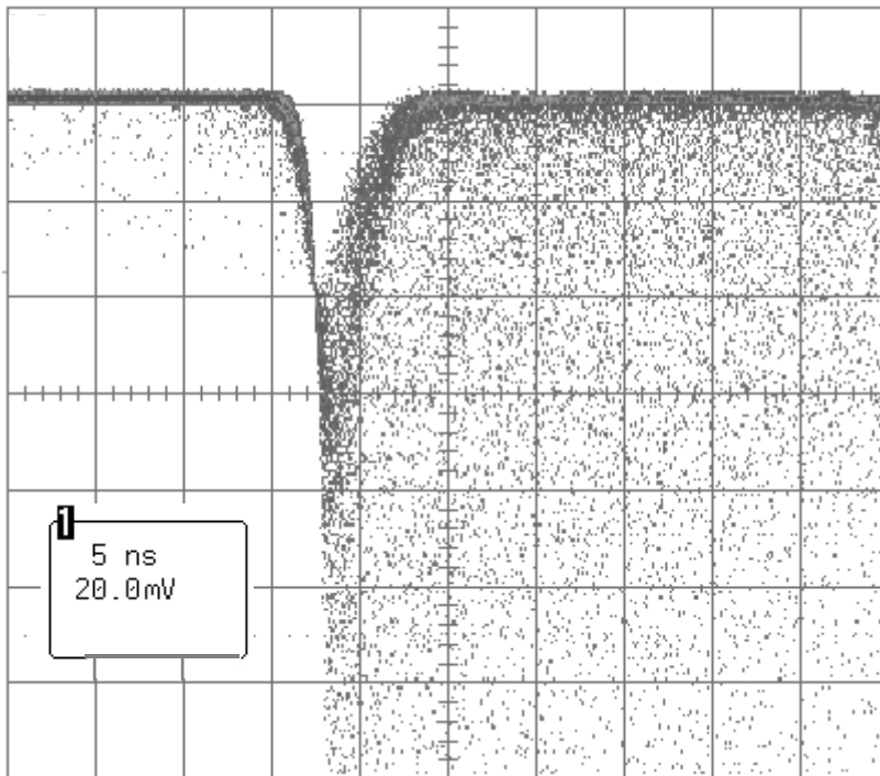
Figure III-15 : Forme des signaux de sortie à l'anode du PM avec les nouvelles embases. Il y a plus de bruit de fond que dans la figure III-9 car le PM est monté sur la latte alors que dans la figure III-9 ou il est seul.
