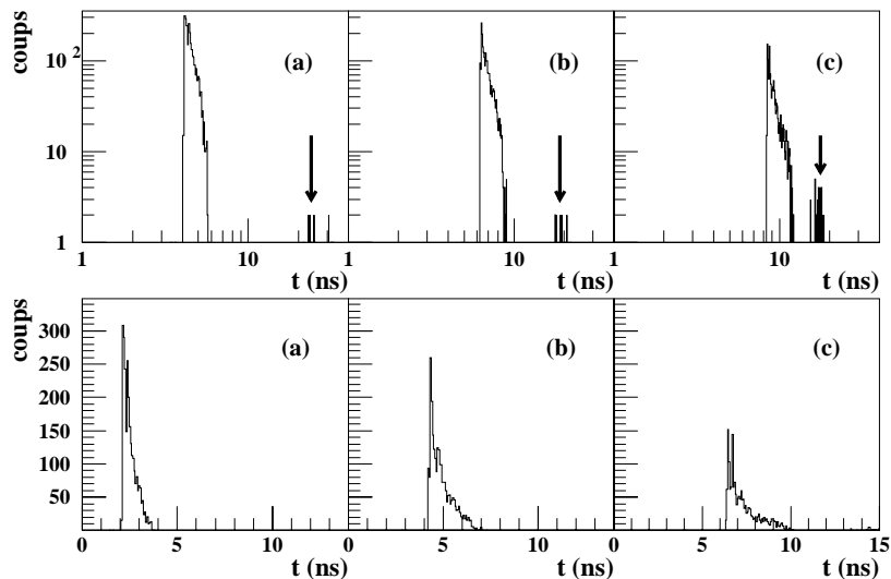
Figure IV-8 : temps de parcours de la lumière dans la latte donné par SIMOP, la "seconde bosse" est le petit pic noté par une flèche. Le seconde colonne représente les même spectres mais en échelle linéaire.
