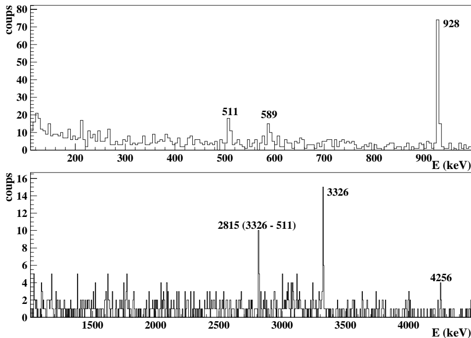
Figure VI-10 : Raies gammas présentes dans le germanium 2 (adddback) lorsque l'on sélectionne le pic à 123 keV dans le germanium 1. Le adddback explique la présence du premier pic d'échappement du gamma à 3326 keV mais pas du suivant.
