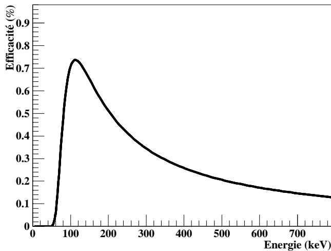
Figure A3-3a : courbe d'efficacité utilisée pour les calculs de l'influence des doubles comptages, c'est celle du pétale 1 du Germanium 1 défini au chapitre V.
