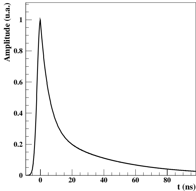
Figure III-4 : Spectre schématique du temps d'émission pour un plastique ternaire. On peut voir les deux composantes de décroissance.
