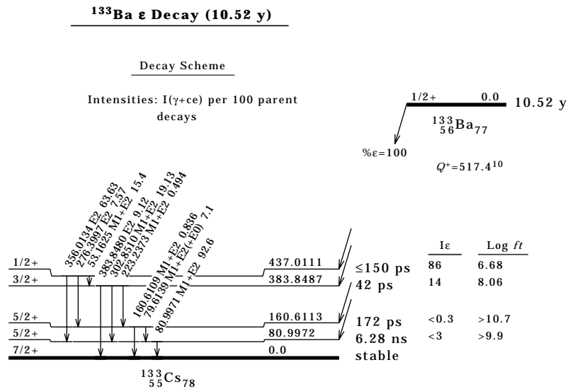
Figure A3-2 : Schéma de décroissance du ^{133}\text{Ba} d'après ENSDF. Les intensités présentées sont celles des transitions électromagnétiques, c'est à dire transition gamma et conversion interne.
