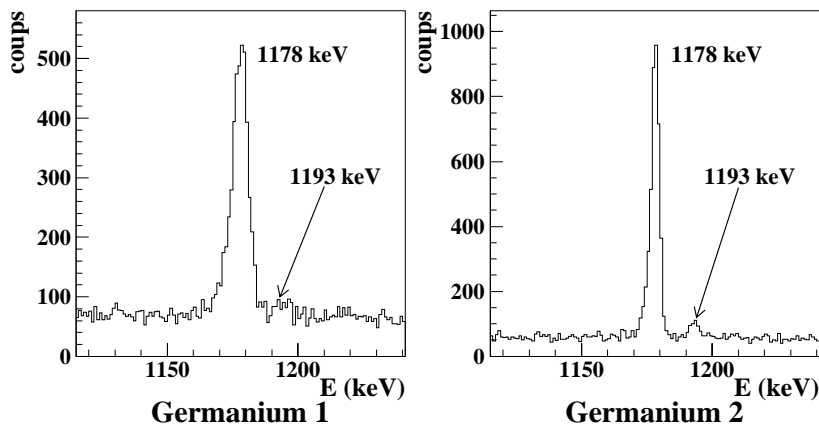
Figure VI-8 : Partie des spectres gammas provenant des deux germaniums. On peu voir que la transitions à 1193 keV est bien présente dans le germanium 2 et non dans le germanium 1 où la faible résolution du détecteur et la proximité du pic à 1178 keV provenant de la décroissance du ^{34}\text{Si} ne permettent pas de la distinguer.
