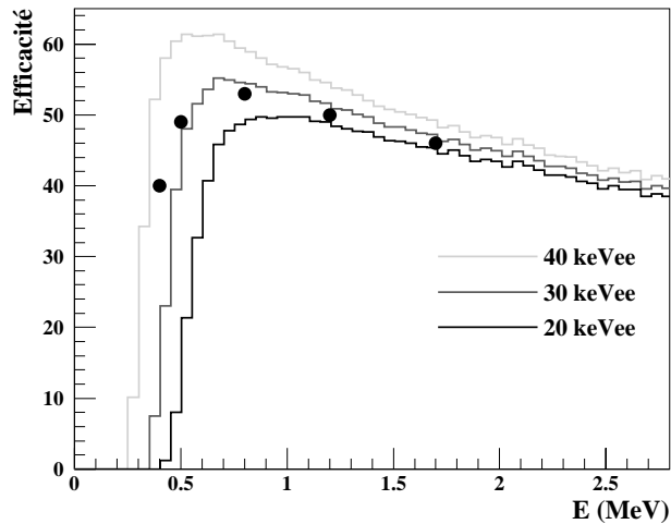
Figure IV-16 : Comparaison des efficacités simulées entre [Tim98] et notre simulation. Les courbes sont les résultats de [Tim98] pour différents seuils (voir texte), les cercles sont les résultats de nos simulations.
