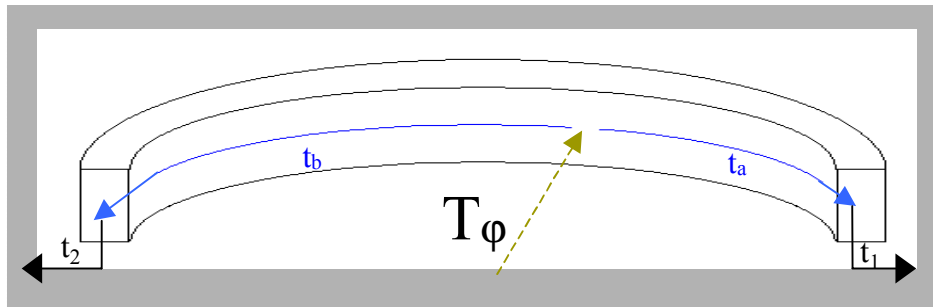
Figure III-8: présentation schématique des composantes des deux signaux temps donnés par TONNERRE. En pointillé, on voit le temps de vol physique de la particule ( T_\phi ), en trait plein le temps de transit de la lumière dans le scintillateur ( t_a et t_b ). t_1 et t_2 sont la somme du temps de vol physique ainsi que du temps de transit dépendant du point d'interaction.
