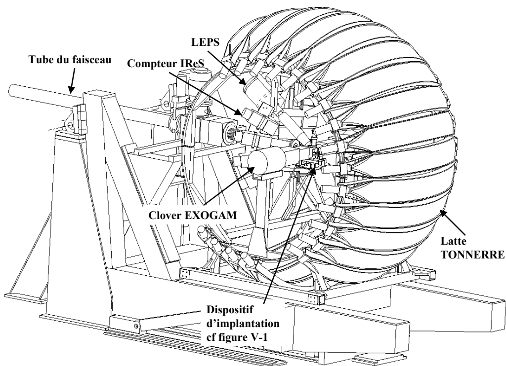
Figure V-2 : Le dispositif expérimental. On distingue les 19 lattes de TONNERRE, les 2 clovers placés perpendiculairement à l'axe du faisceau. Le LEPS étant placé au dessus du tube du faisceau aux angles arrières et les compteurs de l'Ires autour du tube.
