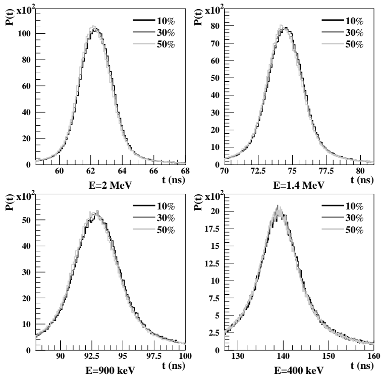
Figure IV-3a : Effet de l'efficacité sur la forme des spectres pour différentes énergies (largeur en énergie de 50 keV).
