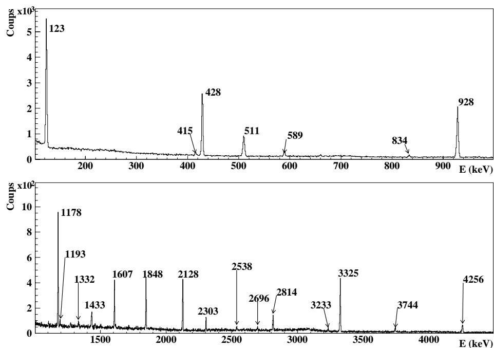
Figure VI-5 : Raies gamma présentes dans les runs du ^{34}\text{Al} . Le tableau 4 présente ces raies associées aux noyaux émetteurs.
