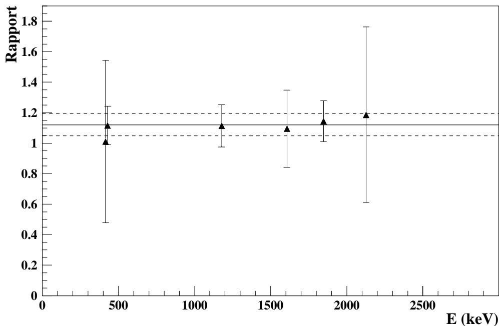
Figure V- 9 : Rapport des noyaux émetteurs estimés dans les filiations du 34 Al entre le germanium 2 et le germanium 1. La moyenne pondéré (représentée par les droites sur le dessin) est de 1.12 (7).
