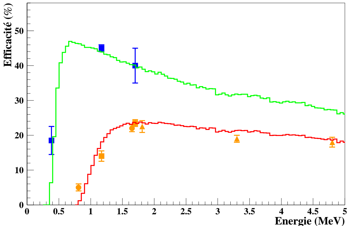
Fig III-16 Comparaison entre les nouvelles et les anciennes embases, pour des spectres en temps de vol (en haut) et pour l'efficacité (en bas). On note une nette amélioration d'efficacité et un abaissement du seuil de détection.
