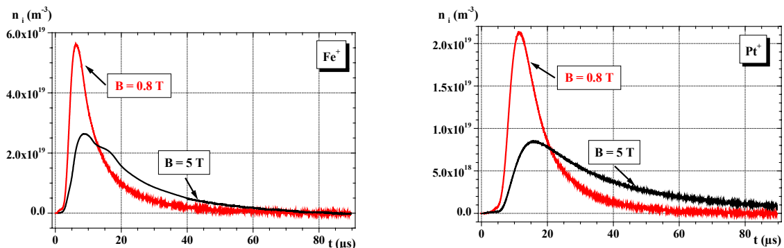
Fig. 22 : Même chose que les figures ci-dessus mais les courbes à 0.8 T sont normalisées en surface sur celles de 5 T .
