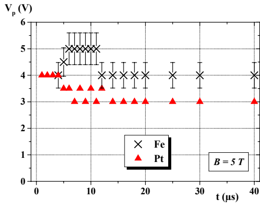
Fig. 16 : Potentiel plasma, en fonction du temps de vol, des plasmas Fe et Pt. B = 5 T , F = 0.9 J cm^{-2} et d_{cible-sonde} = 10 cm .
