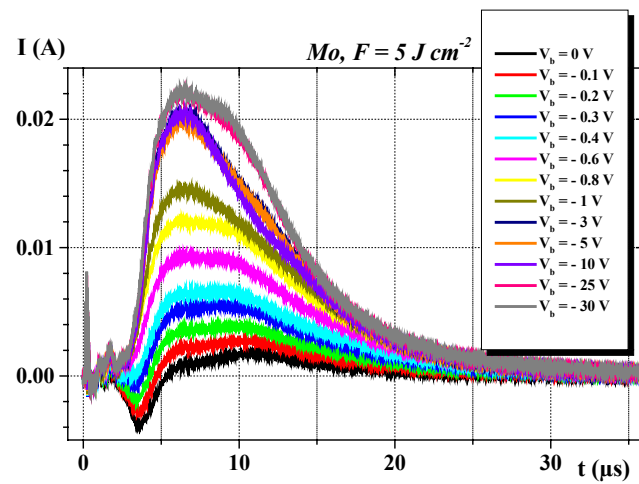
Fig. 10 : Signaux recueillis par la sonde de Langmuir immergée dans un plasma de molybdène pour V_b variant de +30 V à -30 V. F = 5 J cm^{-2} , d_{cible-sonde} = 15 cm .
