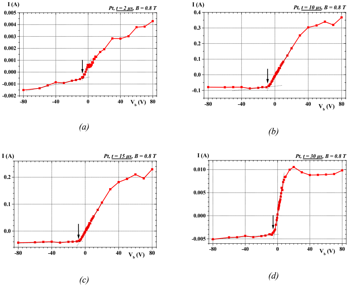
Fig. 13 : I(V_b) pour le plasma Pt, en sonde \perp , à des temps de vol de (a) 2 \mu s , (b) 10 \mu s , (c) 15 \mu s et (d) 30 \mu s . B = 0.8 T et F = 0.9 J cm^{-2} .
