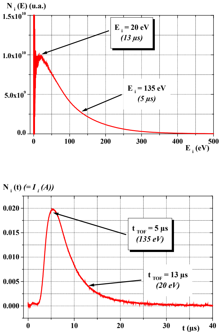
Fig. 13 : (a) Distribution énergétique et (b) distribution temporelle d'ions \text{Fe}^+ collectés par la sonde de Langmuir. V_b = -50 \text{ V} , d_{\text{cible-sonde}} = 10 \text{ cm} , F = 0.9 \text{ J cm}^{-2} et M = 100 \mu\text{s} . Précisons que nous avons toujours, dans ce manuscrit, utilisé I_i(t) et non N_i(t) , dans la relation (19), pour déterminer la fonction de distribution en énergie des ions, N_i(E) , ces 2 entités étant proportionnelles.
