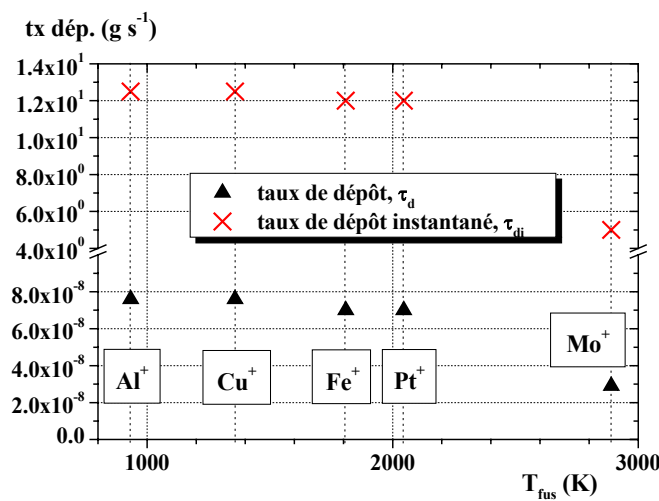
Fig. 24 : Taux de dépôt moyen et taux de dépôt instantané en fonction de la température de fusion. F \approx 1 \text{ J cm}^{-2} . d_{\text{cible-sonde}} = 10 \text{ cm} pour Fe et Pt et d_{\text{cible-substrat}} = 7 \text{ cm} pour Al , Cu et Mo .
