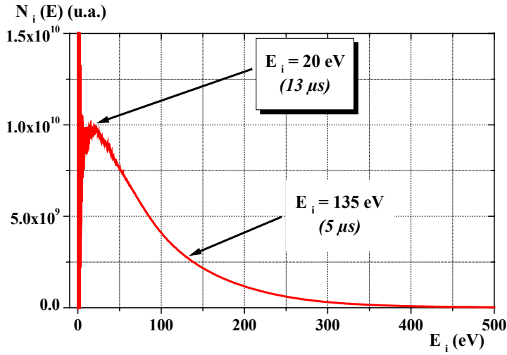
Fig. 13 : (a) Distribution énergétique et (b) distribution temporelle d'ions \text{Fe}^+ collectés par la sonde de Langmuir. V_b = -50 \text{ V} , d_{\text{cible-sonde}} = 10 \text{ cm} , F = 0.9 \text{ J cm}^{-2} et M = 100 \mu\text{s} . Précisons que nous avons toujours, dans ce manuscrit, utilisé I_i(t) et non N_i(t) , dans la relation (19), pour déterminer la fonction de distribution en énergie des ions, N_i(E) , ces 2 entités étant proportionnelles.
