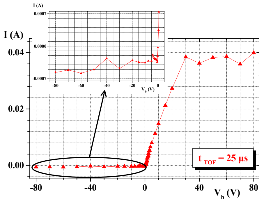
Fig. 7 : Caractéristiques I-V_b du plasma de fer pour un temps de vol de 25 \mu s . En insert, un zoom de la région de collection des ions. Notez pour V_b > +30 V, la saturation du signal collecté par la sonde.
