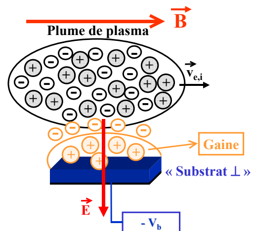
Fig. 1 : Dépôt laser pulsé sous champs magnétique et électrique.
