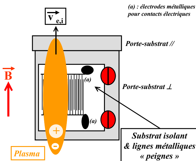
Fig. 5 : Vue de dessus schématique représentant les substrats \perp gravés et leur disposition par rapport à la plume de matière évaporée. Lors des dépôts, les lignes sont placées soit perpendiculairement au champ magnétique soit parallèlement comme sur le schéma.
