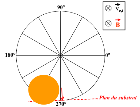
Fig. 8 : Vue de face de la position optimale du substrat. Le cercle plein correspond à l'image du spot laser sur la cible.
