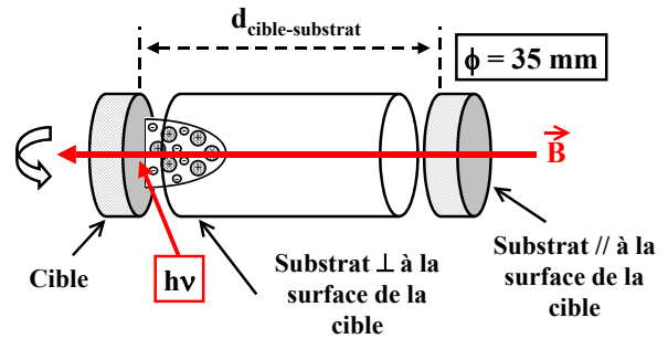
Fig. 3 : Schéma représentant la disposition de la cible et des substrats.
