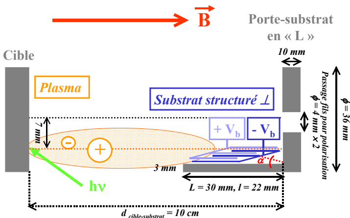
Fig. 4 : Représentation schématique du porte-substrat en L utilisé lors des dépôts perpendiculaires. La distance entre la cible et la partie du porte-substrat parallèle à la surface de la cible est de 10\text{ cm} . Le porte-substrat peut être incliné d'un angle \alpha par rapport à l'angle d'expansion.
