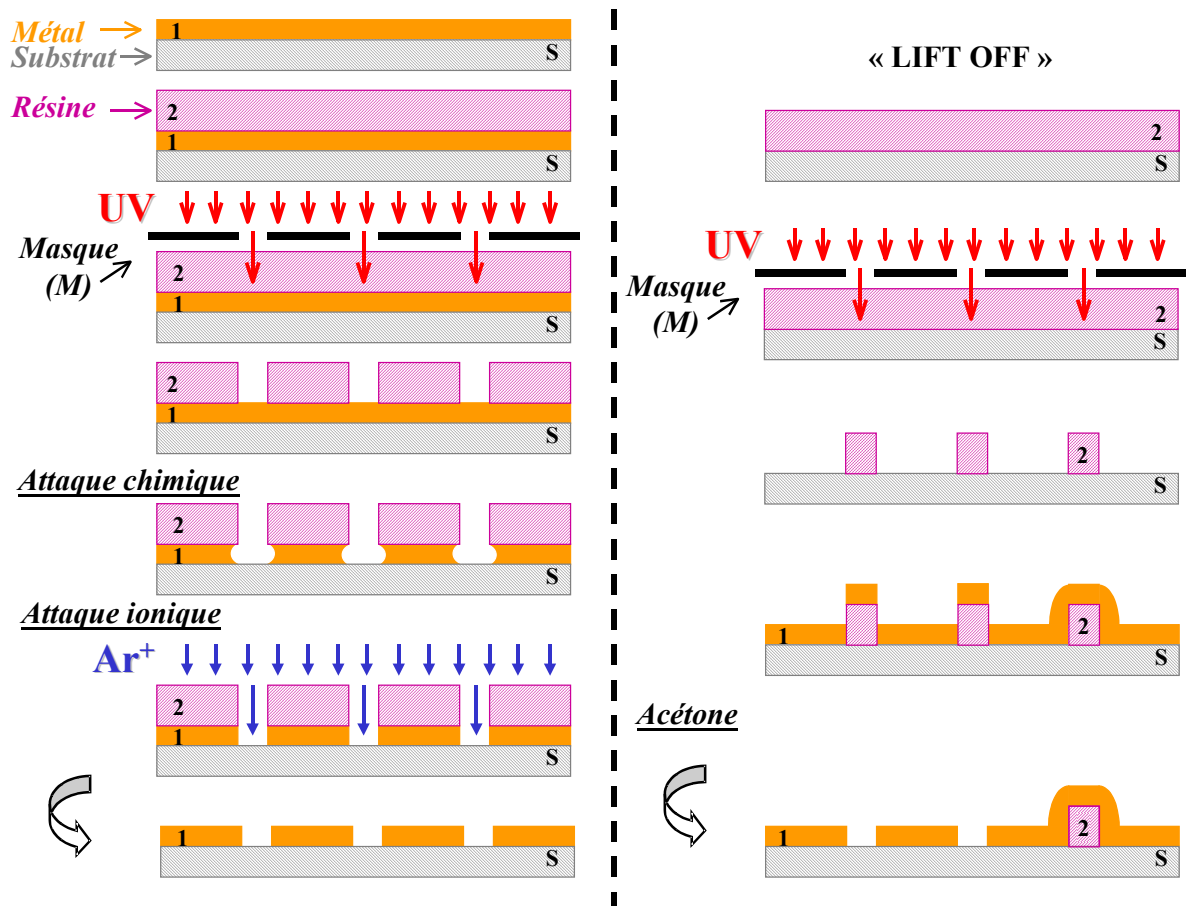
Fig. 6 : Techniques de microfabrication utilisées pour élaborer les motifs en forme de peignes imbriqués, à gauche avec une résine photosensible positive, à droite avec une résine photosensible négative (« lift off »).
