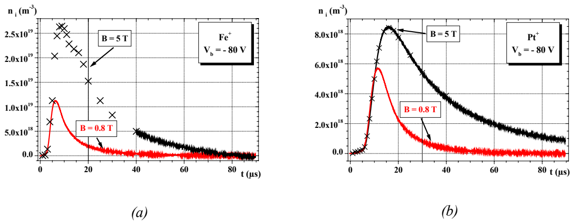
Fig. 21 : Densités ioniques ( m^{-3} ) des plasmas (a) Fe et (b) Pt , générés sous champ magnétique ( 0.8\text{ T} et 5\text{ T} ). V_b = -80\text{ V} , F = 0.9\text{ J cm}^{-2} et d_{cible-sonde} = 10\text{ cm} . Les croix représentent une densité déterminée par extrapolation des courbes I(V_b) . Notez la proportion importante d'ions sous 5\text{ T} après t = 20\text{ }\mu\text{s} pour Fe et t = 30\text{ }\mu\text{s} pour Pt . À comparer avec n_i(t) à B = 0\text{ T} (Chapitre 3 Fig. 15 p. 79).
