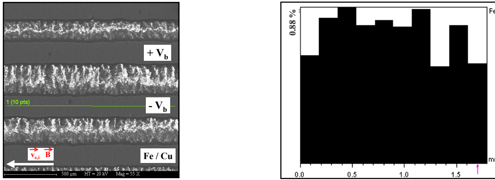
Fig. 23 : Cartographie d'une ligne d'un dépôt de Fe sur Cu, l = 200 \mu\text{m} et d \approx 200 \mu\text{m} . V_b = -80 \text{ V} / +40 \text{ V} , \alpha = 0^\circ , t_{\text{dep}} < 30 \text{ min} .
