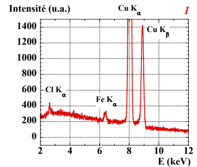
Fig. 22 : Analyse chimique (MEB) d'un dépôt alternatif de Fe et Pt sur Cu, l = 200\ \mu\text{m} et d \approx 200\ \mu\text{m} . V_b = \pm 80\text{ V} , \alpha = 5^\circ , t_{dep} = 2\text{ h} pour chacun des métaux.
