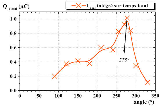
Fig. 7 : Optimisation de la position angulaire du substrat perpendiculaire. La position déterminée est telle que le plan du substrat est pratiquement parallèle au sol. Fe^+ et V_b = -50 V .
