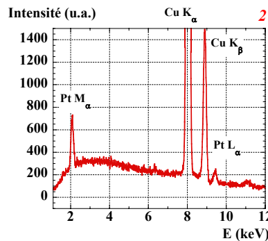
Fig. 22 : Analyse chimique (MEB) d'un dépôt alternatif de Fe et Pt sur Cu, l = 200\ \mu\text{m} et d \approx 200\ \mu\text{m} . V_b = \pm 80\text{ V} , \alpha = 5^\circ , t_{dep} = 2\text{ h} pour chacun des métaux.
