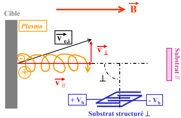
Fig. 3 : Géométrie du système dans son ensemble.
