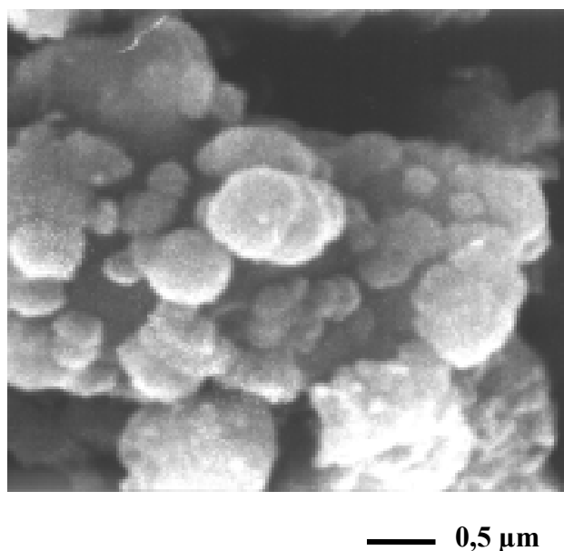
Figure 2.7 : Photographie MEB de la poudre \text{Cu}_3\text{N} obtenue par décomposition de \text{Cu}(\text{acac})_2 dans \text{NH}_3 ( T = 200^\circ\text{C} ; P = 17 \text{ MPa} ).
