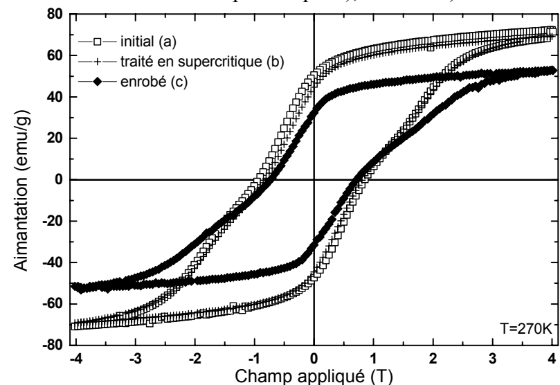
Figure 4.34 : Propriétés magnétiques du \text{SmCo}_5 broyé 2 heures à 250 tours/min : initial a), traité en milieu fluide supercritique b), enrobé c).
