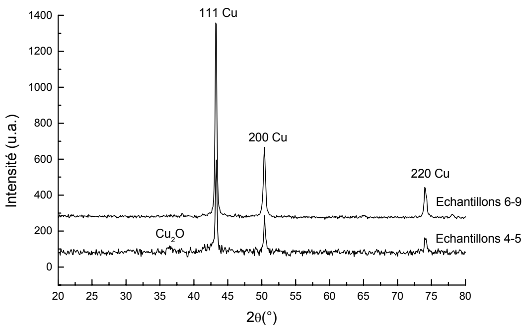
Figure 3.2 : Diffractogrammes sur poudre effectués sur les échantillons 4 à 9. Mise en évidence de la phase cuivre (fiche JCPDS n°4-0836). Nous pouvons noter la présence de la phase \text{Cu}_2\text{O} dans les échantillons 4 et 5.
