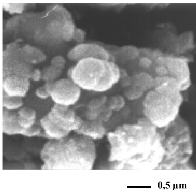
Figure 2.7 : Photographie MEB de la poudre \text{Cu}_3\text{N} obtenue par décomposition de \text{Cu}(\text{acac})_2 dans \text{NH}_3 ( T = 200^\circ\text{C} ; P = 17 MPa).
