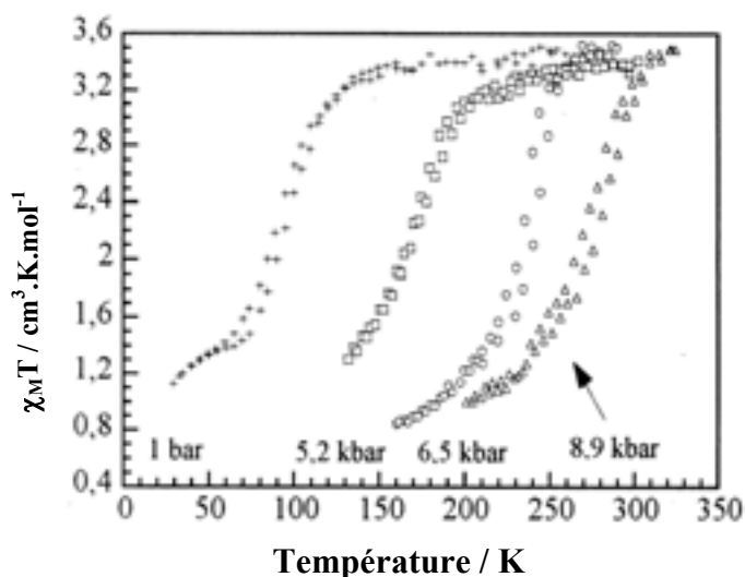
Figure I.6 : Evolution du produit \chi_M T en fonction de la température à différentes pressions, du composé [\text{Fe}(\text{hyetrz})_3](3\text{-nitrophényl sulfonate})_2 [30].
