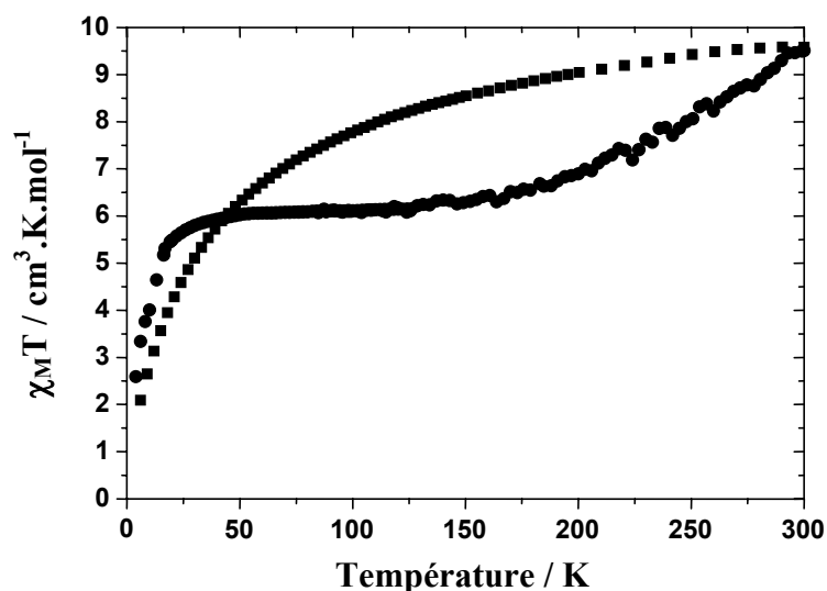
Figure III.36 : Comportements magnétiques en fonction de la température des composés trinuéaires (■) [\text{Fe}_3(p\text{-MeOptrz})_8(\text{H}_2\text{O})_4](\text{BF}_4)_6 et (●) [\text{Fe}_3(p\text{-MeOptrz})_6(\text{H}_2\text{O})_6](\text{tos})_6 .
