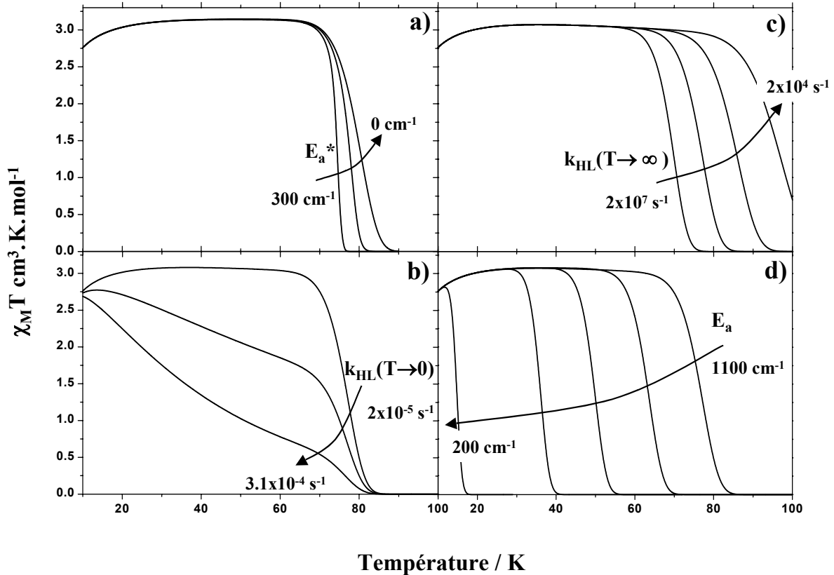
Figure II.19 : (a) Influence de la coopérativité sur le T(LIESST). Courbes simulées avec E_a^* = 0, 120 et 300\text{ cm}^{-1} . (b) Influence de k_{HL}(T \rightarrow 0) sur le T(LIESST). Courbes simulées avec k_{HL}(T \rightarrow 0) = 1,8 \cdot 10^{-5}, 1,8 \cdot 10^{-4} et 3,1 \cdot 10^{-4}\text{ s}^{-1} . (c) Influence de k_{HL}(T \rightarrow \infty) sur le T(LIESST). Courbes simulées avec k_{HL}(T \rightarrow \infty) = 2 \cdot 10^7, 2 \cdot 10^6, 2 \cdot 10^5 et 2 \cdot 10^4\text{ s}^{-1} . (d) Influence de E_a sur le T(LIESST). Courbes simulées avec E_a = 1100, 900, 700, 500 et 200\text{ cm}^{-1} .
