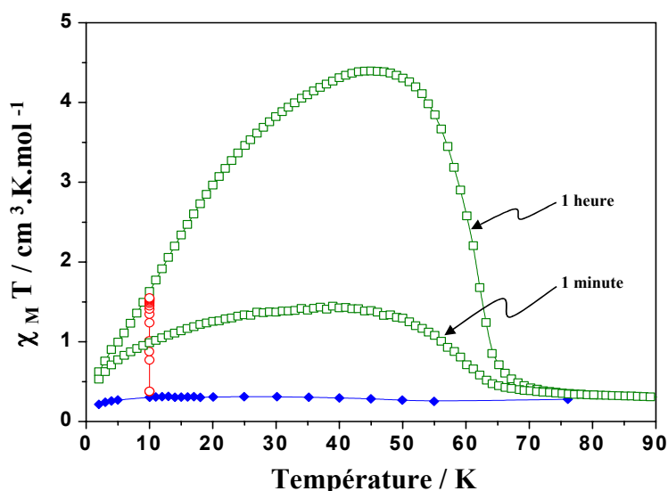
Figure III.29 : Expériences de mesure de T(LIESST) après des temps d'irradiation différents, une heure ou une minute.
