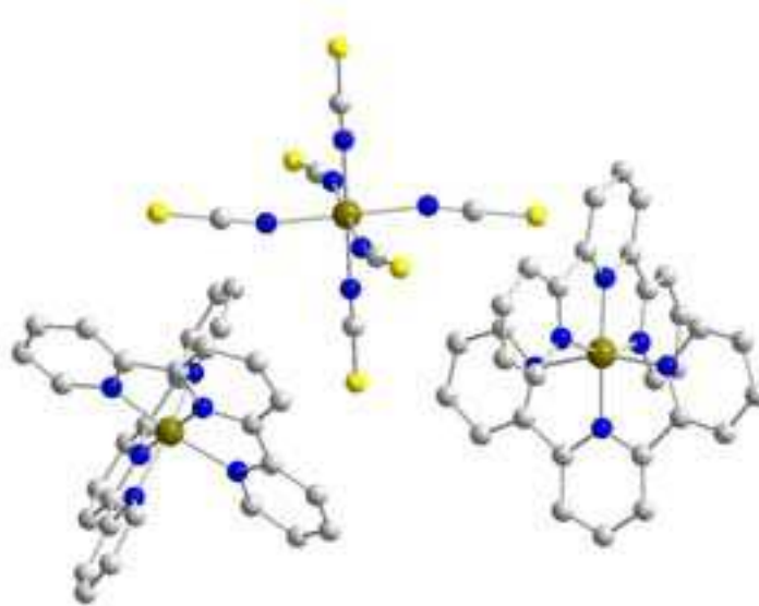
Figure III.39 : Structure de l'échantillon [Fe(tpy)_2]-[Fe(NCS)_6]-[Fe(tpy)_2] . La molécule de solvant (méthanol) a été volontairement omise.
