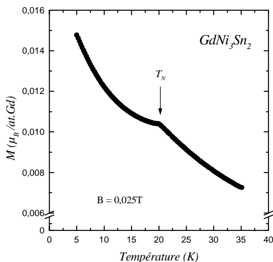
Figure III-33 : Variation thermique de l'aimantation de GdNi 3 Sn 2
