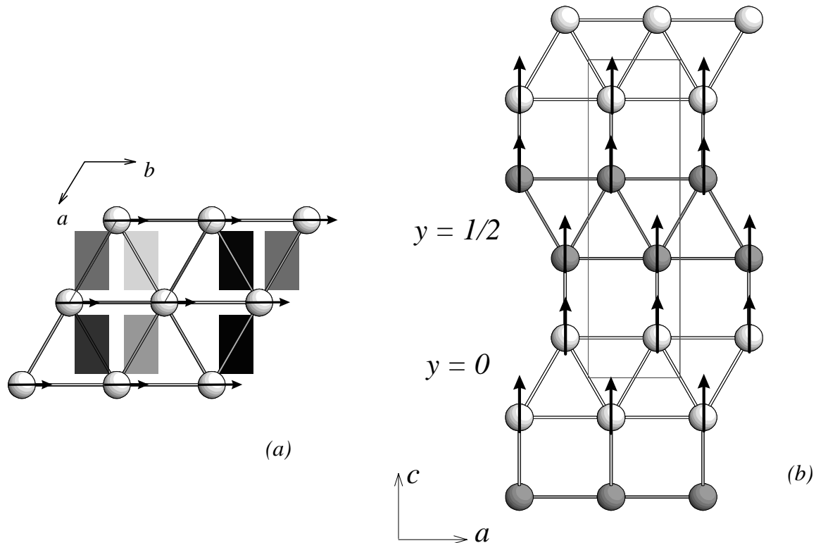
Figure II-45 : Structures ferromagnétiques des variétés \text{AlB}_2 (a) et \alpha\text{-ThSi}_2 (b) de \text{UCu}_{0,49(1)}\text{Si}_{1,51(1)}
