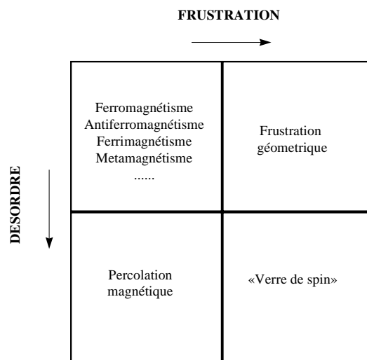
Figure I-6 : Représentation schématisée de possibles états magnétiques fondamentaux en fonction du désordre et de la frustration magnétique.
