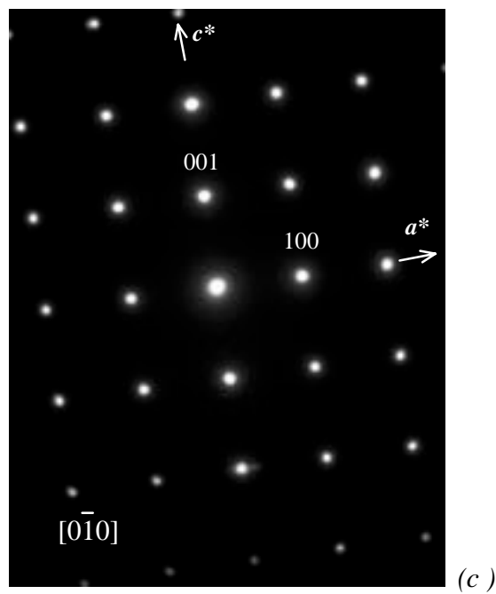
Figure III-23 : Clichés de diffraction électronique obtenus suivant les axes de zone [001] (a), [1\bar{1}0] (b) et [0\bar{1}0] (c) d'une microcristallite de \text{GdNi}_3\text{Al}_2 . Les trois plans principaux du réseau réciproque hexagonal sont indexés sur la base d'une maille de type \text{CaCu}_5 ( a = 5,058\text{\AA} , c = 4,079\text{\AA} ) et un vecteur de modulation q^* = (1/3\ 1/3\ 1/2) .
