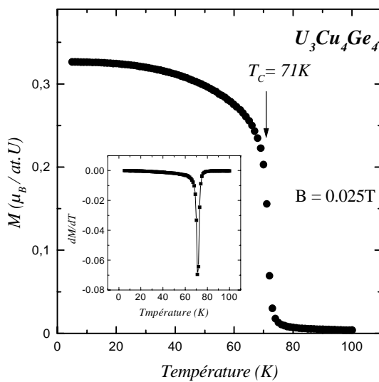
Figure II-15 : Variation thermique de l'aimantation de U_3Cu_4Ge_4
