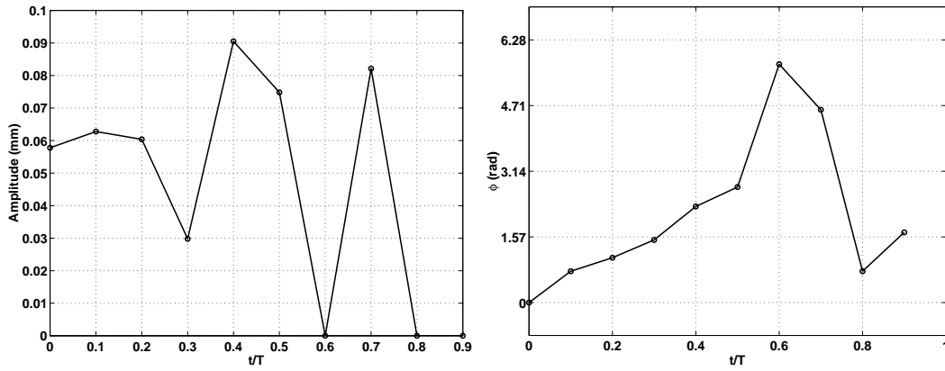
FIG. 5.10: Paramètres d'identification du troisième mode sur un cycle d'oscillations en l'absence de couplage fluide-résonant ; U_\infty = 29,8 m/s ; Amplitude moyenne identifiée : A_0=0,065 mm.
