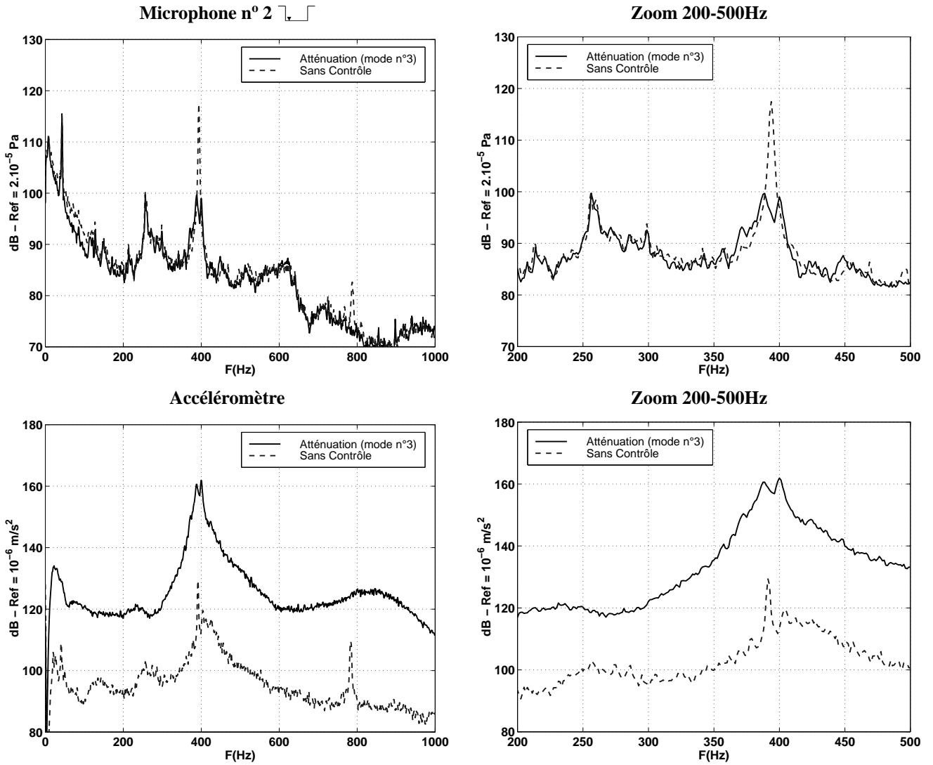
FIG. 4.33: Atténuation du couplage fluide-résonant ; Mode n° 3, U_\infty = 31 \text{ m/s} , L=150 \text{ mm} , L/D = 1 , W/L = 5, 2 , Microphone n° 2 et accéléromètre.
