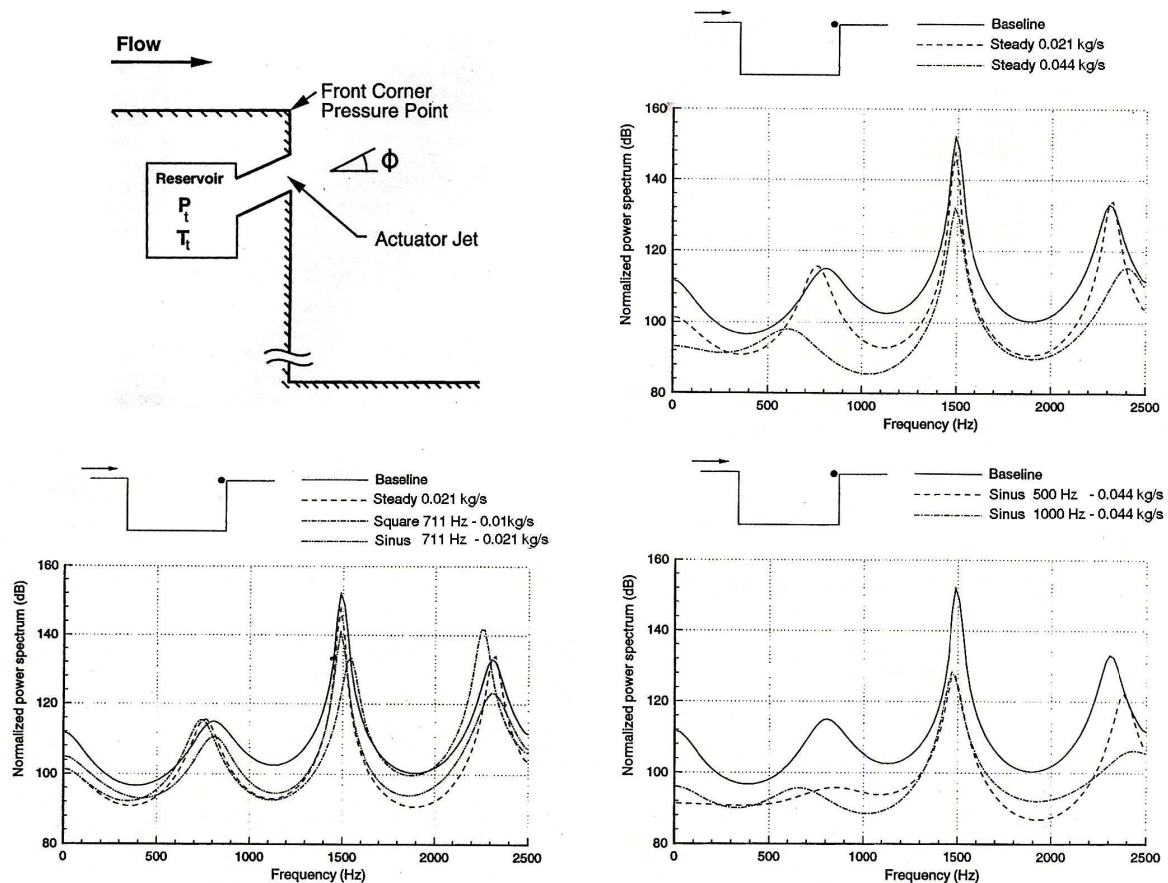
FIG. 4.9: Simulations de Lamp & Chokani [48], comparaison des performances obtenues par soufflage adapté et par forçage à basse fréquence.
