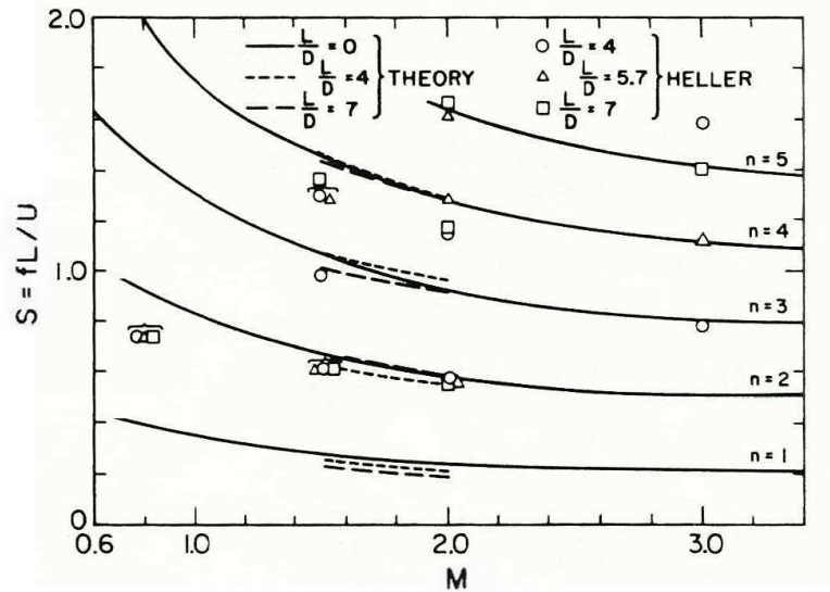
FIG. 1.25: Comparaison de l'équation 1.4 avec les données expérimentales de Heller et al. [33].
