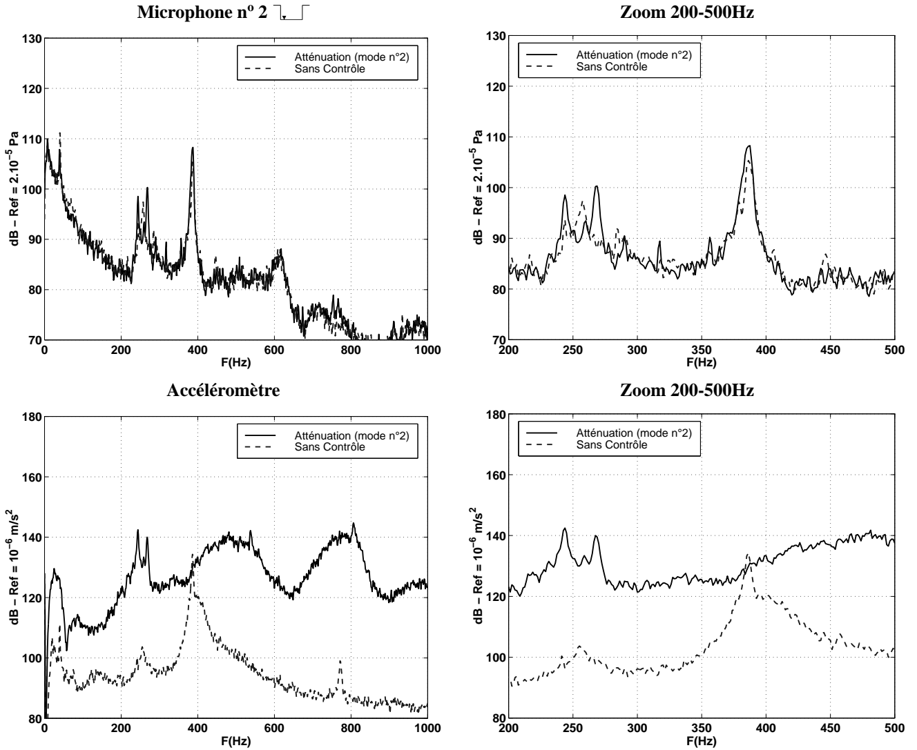
FIG. 4.31: Atténuation du couplage fluide-résonant; Mode n° 2, U_\infty = 30,1 m/s, L=150 mm, L/D = 1 , W/L = 5,2 , Microphone n° 2 et accéléromètre.
