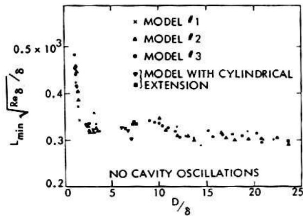
FIG. 1.13: Domaine d'apparition d'oscillations en cavité axisymétrique [70].
