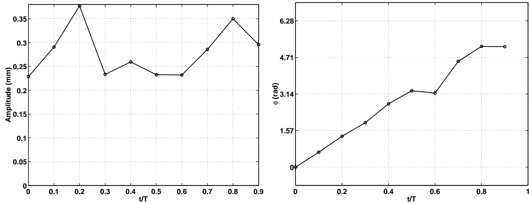
FIG. 5.31: Paramètres d'identification du troisième mode après atténuation ; U_\infty = 31 m/s ; Amplitude moyenne identifiée : A_0 = 0,279 mm.
