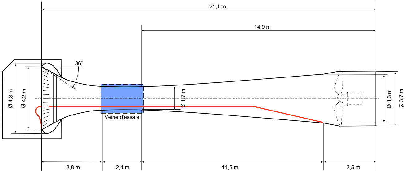
FIG. 3.1: Soufflerie Nieuport
