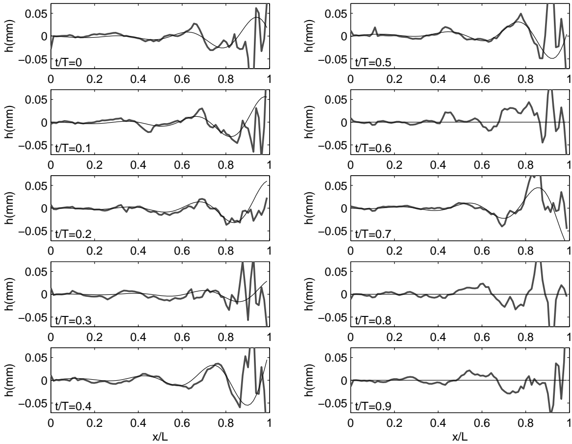
FIG. 5.11: Cycle d'oscillations du troisième mode en l'absence de couplage fluide-résonant ; U_\infty = 29,8 m/s.
