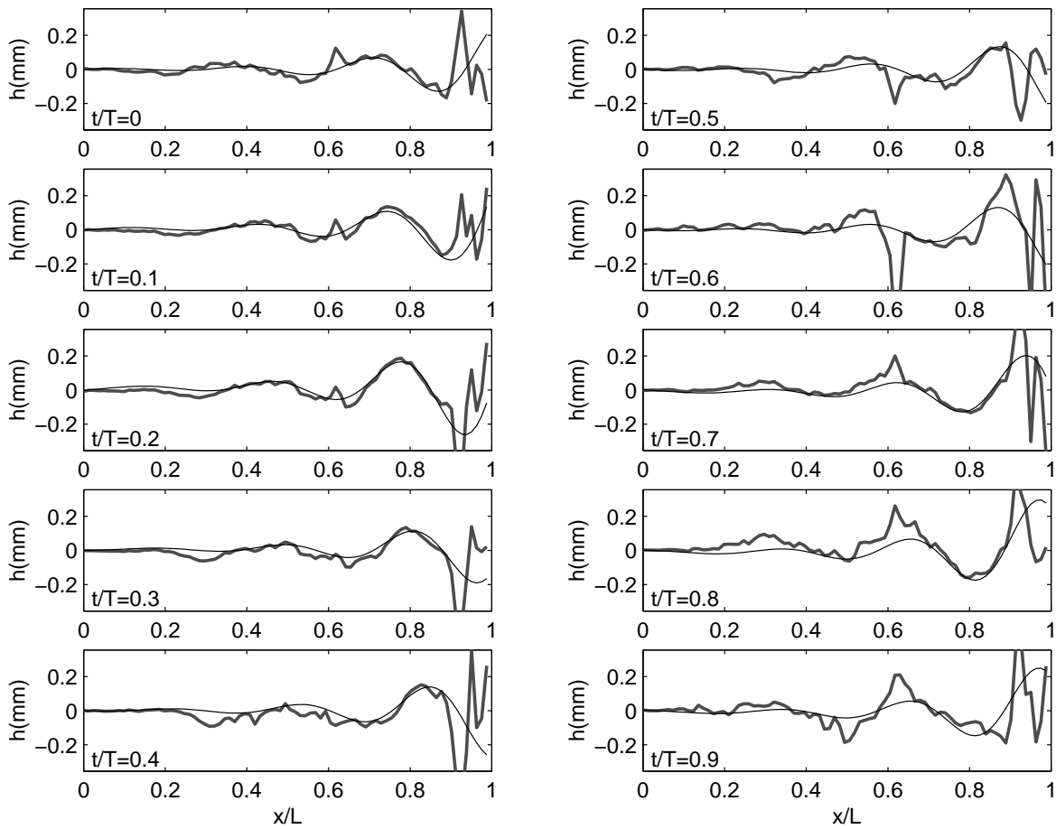
FIG. 5.32: Atténuation du troisième mode ; U_\infty = 31 m/s.
