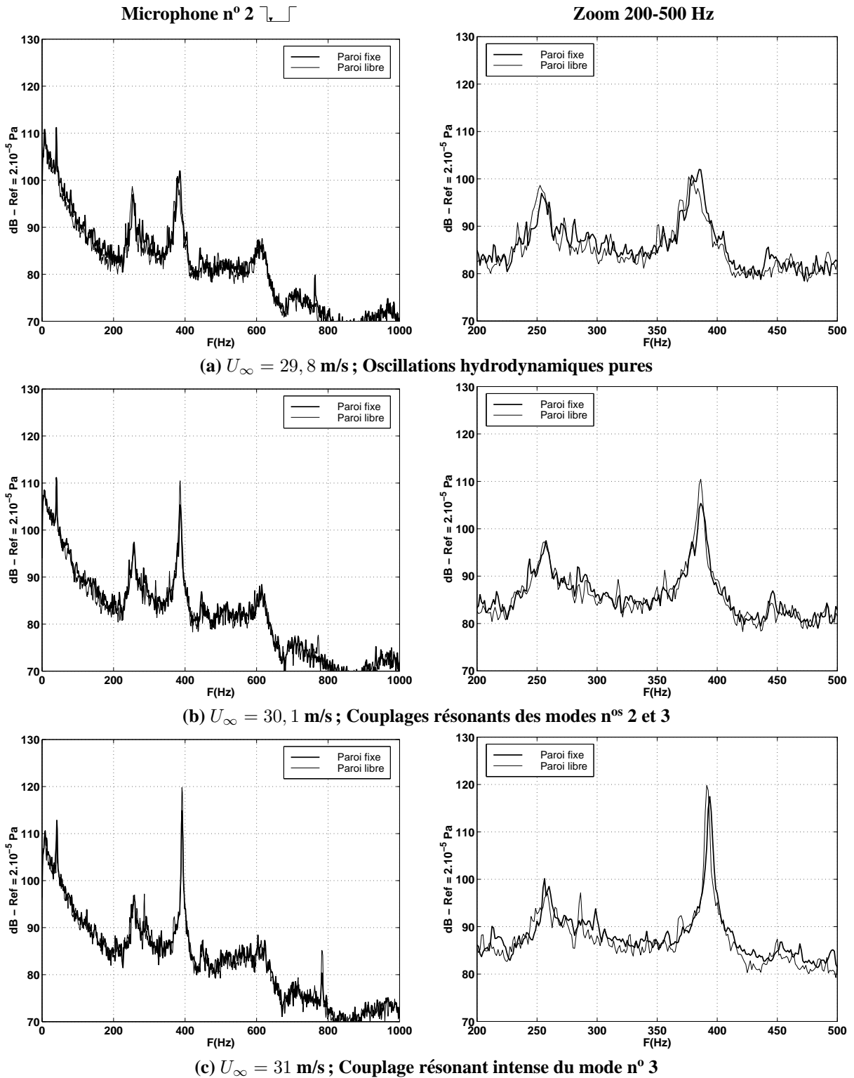
FIG. 4.18: Effet de la présence de l'actionneur libre sur les fluctuations de pression mesurées en fond de cavité pour trois régimes d'écoulement voisins, L=150 mm, L/D = 1 , W/L = 5, 2 .
