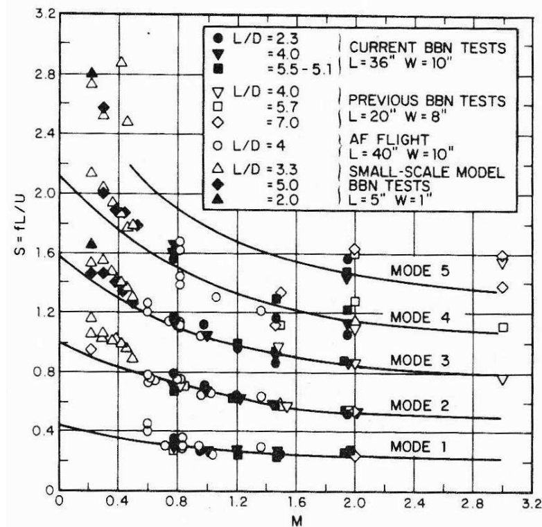
FIG. 1.22: Comparaison de l'équation 1.3 avec les données expérimentales de Heller & Bliss [32].
