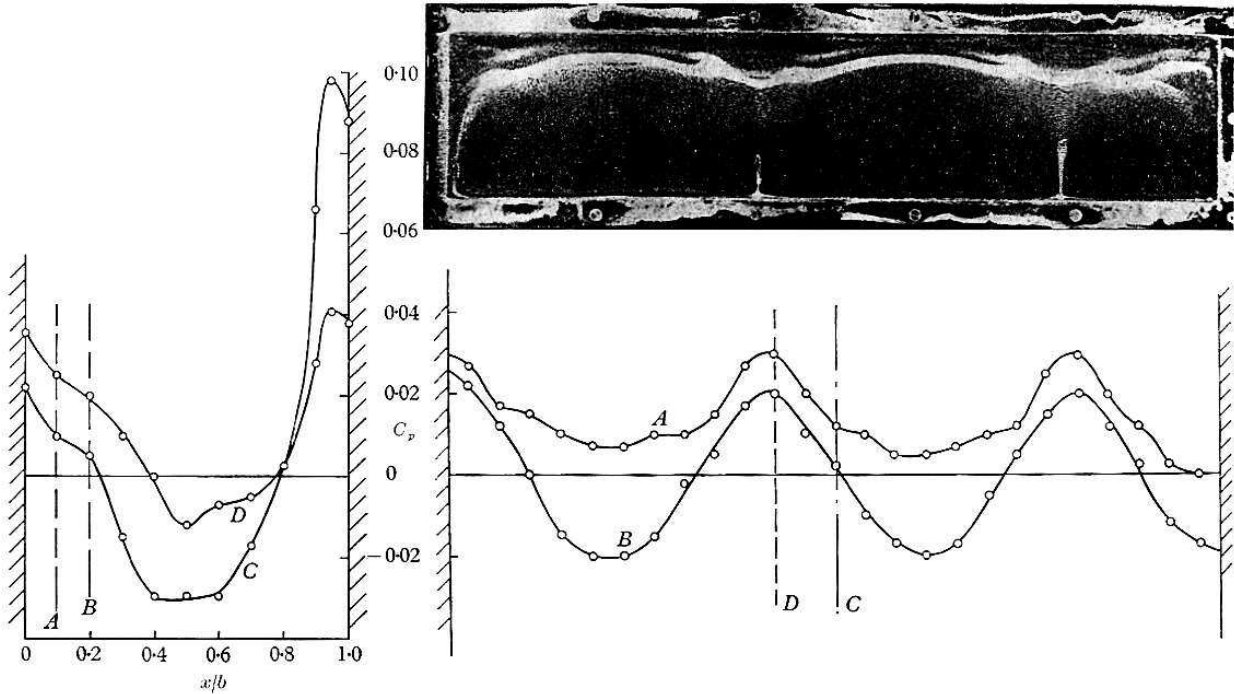
FIG. 1.10: Structures longitudinale et transversale de l' coulement, comparaison avec les mesures de pression statique [51].
