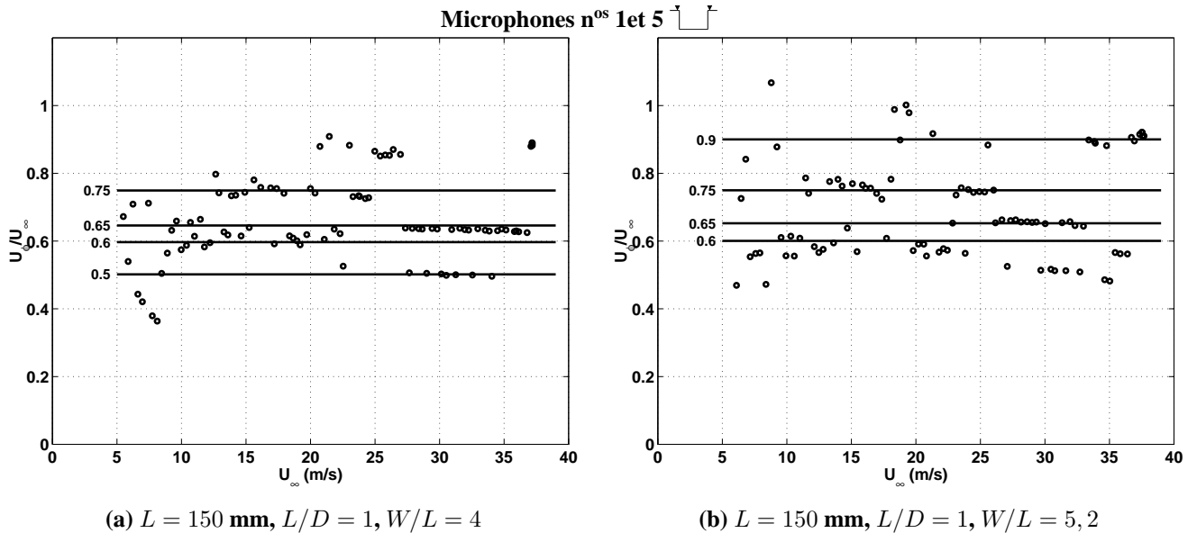
FIG. 3.24: Estimation de la vitesse de phase entre les microphones n^{OS} 1 et 5.
