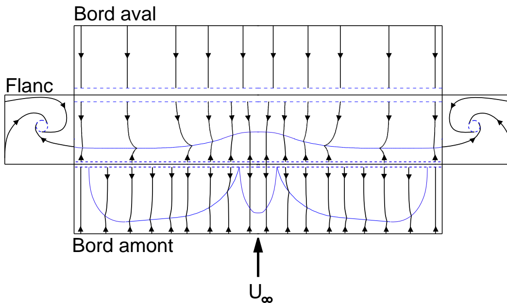
FIG. 3.15: Tracé des lignes de diffusion en paroi, maquette avec flancs ; \blacktriangleright : lignes de diffusion, \text{---} : lignes de séparation.
