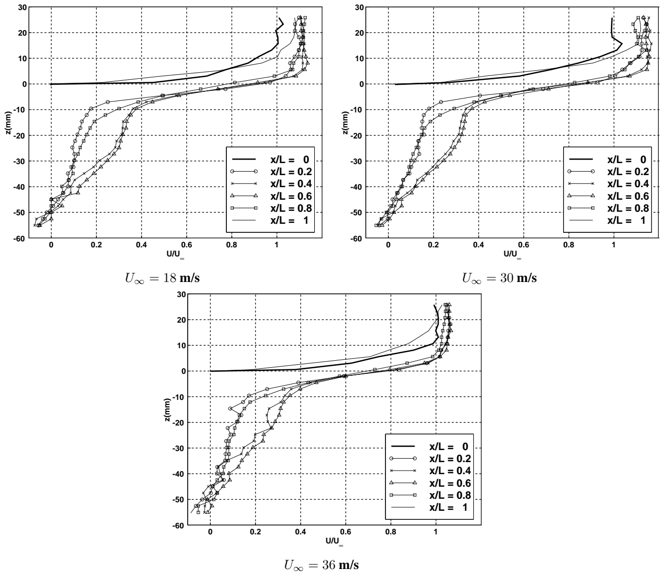
FIG. 5.5: Evolution de la couche de mélange selon la longueur de cavité pour trois régimes d'écoulement différents; L = 100 mm; L/D = 1 ; W/L = 7, 8 .
