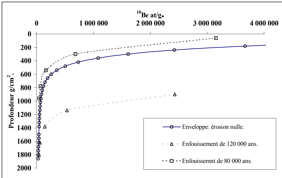
Figure 17: Comparaison des courbes concentrations en 10 Be en fonction de la profondeur pour une érosion nulle et un profil enfoui depuis 80 000 et 120 000 ans.
